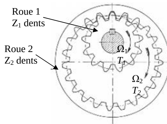
Fig. I.2 .d Engrenage en contact intérieur
