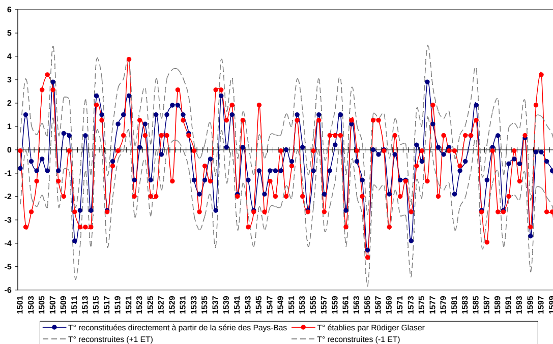
Graphique 36 – Comparaison entre les températures moyennes (en C°) allemandes des hivers (DJF) reconstruites directement à partir de celles des Pays-Bas, et la série établie par Rüdiger Glaser (1501-1600)
