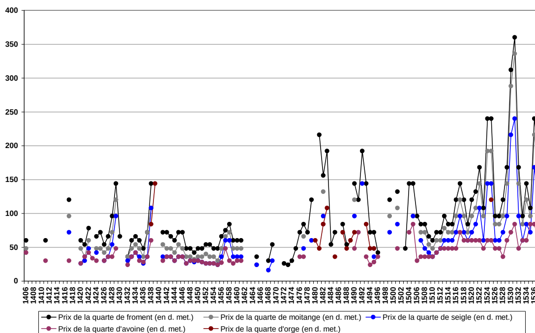
Graphique 69 – Prix annuels (post-récoltes) des céréales (froment, moitange, seigle, avoine, orge) à Metz, en d. met. par quartre, 1406-1537
