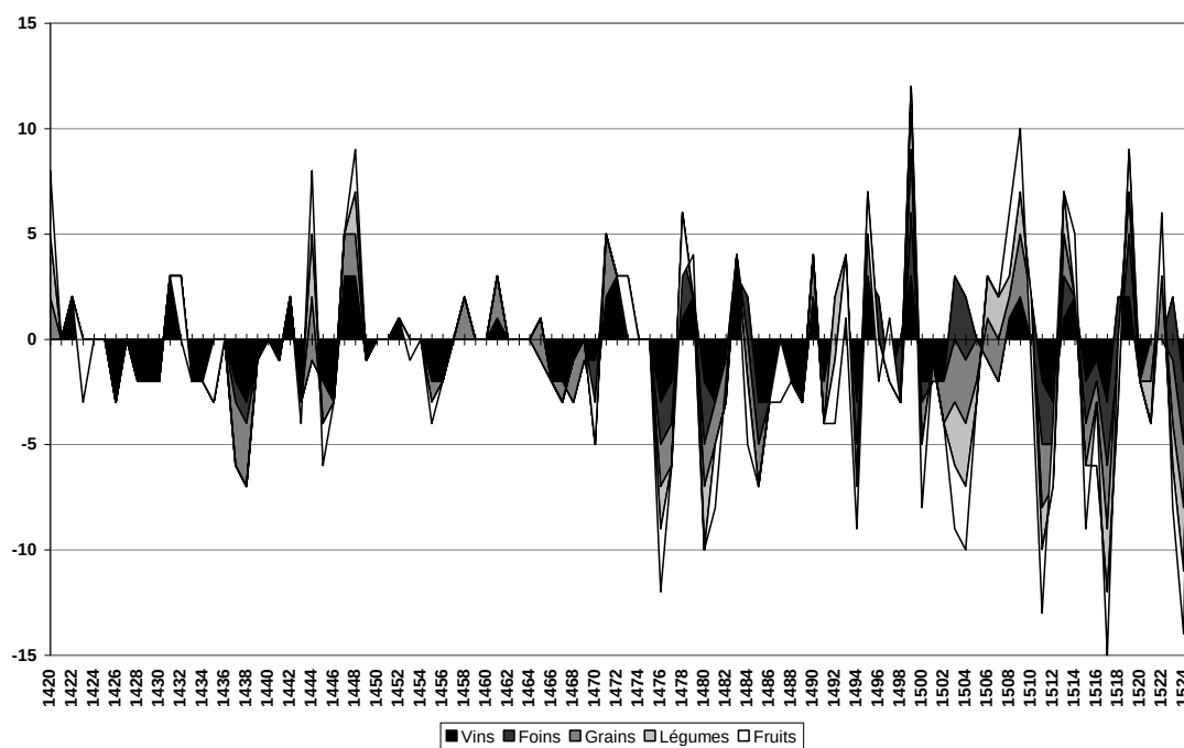
Graphique 63 – Indice global des quantités des récoltes annuelles (vins, foin, grains, légumes, fruits) dans le Pays messin (1420-1525)
