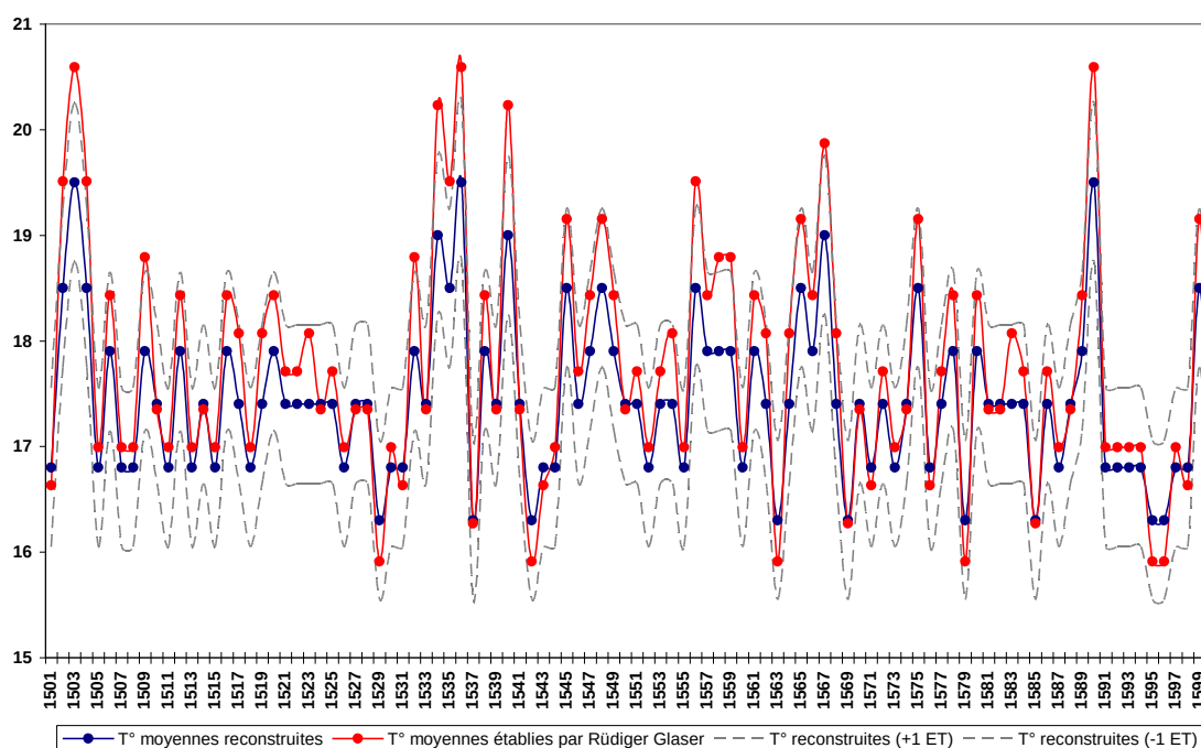
Graphique 35 – Comparaison entre les températures moyennes (en C°) allemandes des étés (JJA) reconstruites et celles établies par Rüdiger Glaser (1501-1600)
