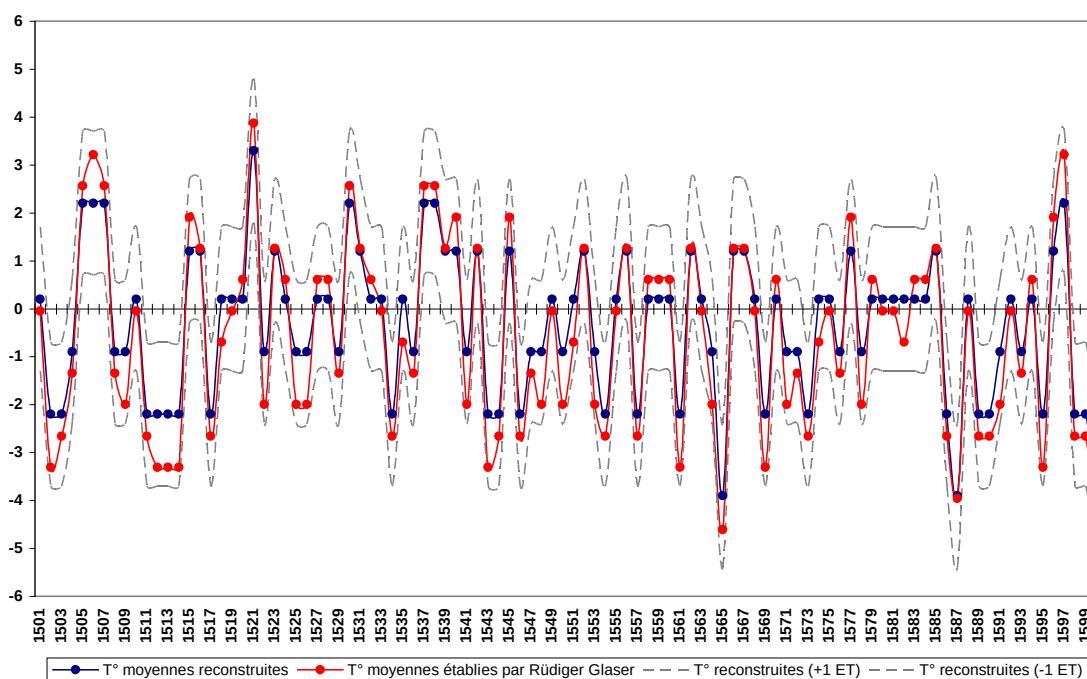
Graphique 34 – Comparaison entre les températures moyennes (en C°) allemandes des hivers (DJF) reconstruites et celles établies par Rüdiger Glaser (1501-1600)
