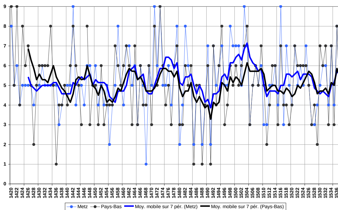
Graphique 32 – Comparaison des indices messins et hollandais des températures estivales (MJJAS), 1420-1537
