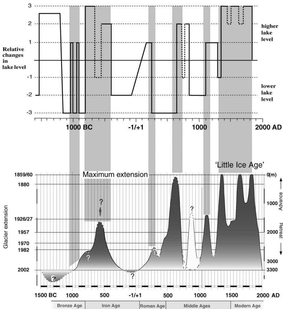
Figure 9 – Comparaison entre les fluctuations du glacier du Grand Aletsch (en bas) et les variations du niveau des lacs du Centre-Ouest européen (en haut) 655
