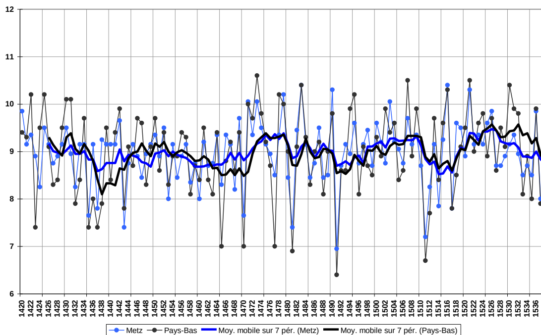
Graphique 38 – Reconstruction hypothétique (en C°) des températures annuelles moyennes à Metz, comparées aux températures moyennes annuelles des Pays-Bas (1420-1537)
