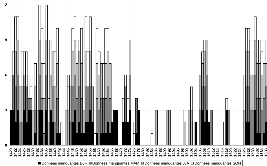
Graphique 16 – Nombre de mois non renseignés en termes de précipitations, 1420-1537
