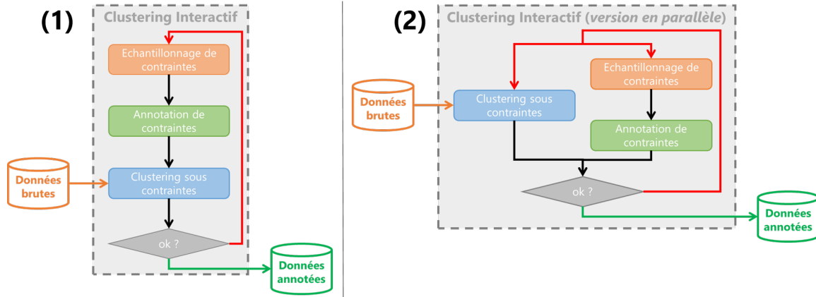
FIGURE 4.21 – Schéma comparatif des architectures du Clustering Interactif : (1) représente la version séquentielle initialement présentée en CHAPITRE 3 où le clustering s’adapte avec les annotations de l’itération en cours ; (2) représente l’évolution en mode parallèle où le clustering s’adapte avec les annotations de l’itération précédente (décalage d’une itération).
