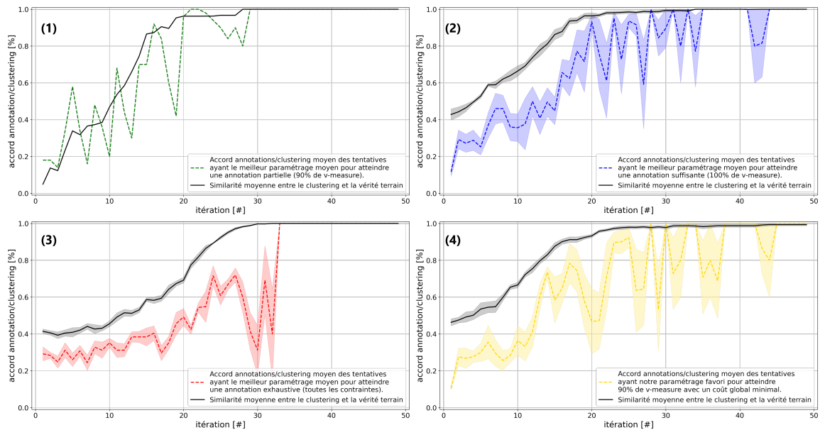
FIGURE 4.28 – Évolution au cours des itérations de l'accord entre l'annotation de contraintes d'un expert et le résultat de clustering sur lequel est basé l'échantillonnage de contraintes. Ces accords sont exprimés grâce à des lots de 50 contraintes annotées. Les évolutions moyennes de différents paramétrages de la méthode sont exposées : (1) meilleur paramétrage moyen pour atteindre une annotation partielle ; (2) meilleur paramétrage moyen pour atteindre une annotation suffisante ; (3) meilleur paramétrage moyen pour atteindre une annotation exhaustive ; et (4) paramétrage favori. À titre d'information, les courbes en noir représentent l'évolution de la v-mesure entre le clustering et la vérité terrain.
