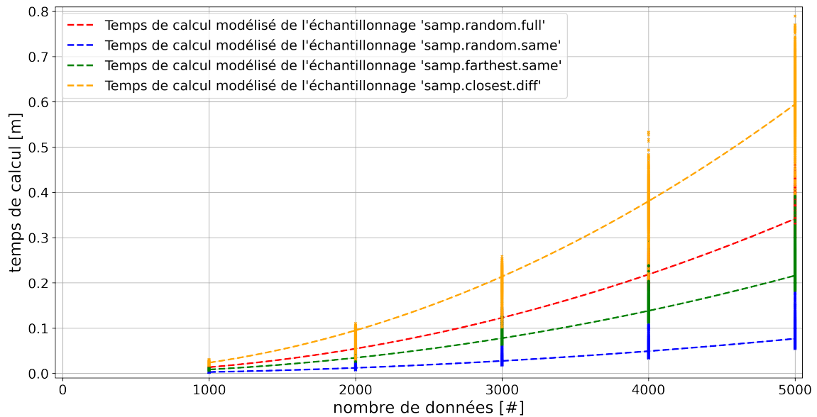
FIGURE 4.18 – Estimation du temps nécessaire (en minutes) pour effectuer une tâche d'échantillonnage de contraintes en fonction du nombre de données à traiter.
