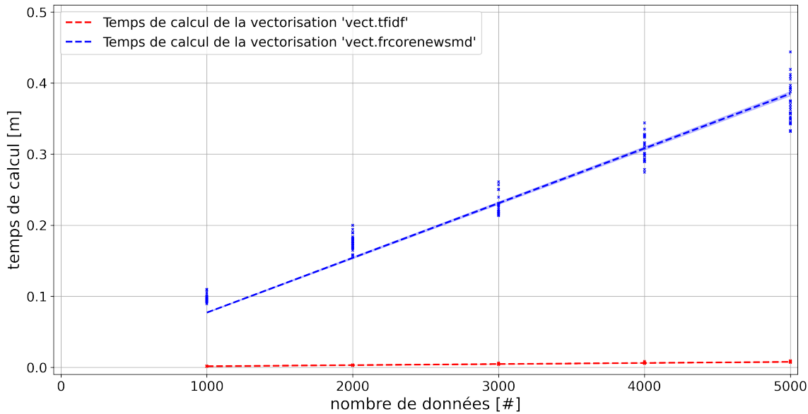
FIGURE 4.16 – Estimation du temps nécessaire (en minutes) pour effectuer une tâche de vectorisation en fonction du nombre de données à traiter.
