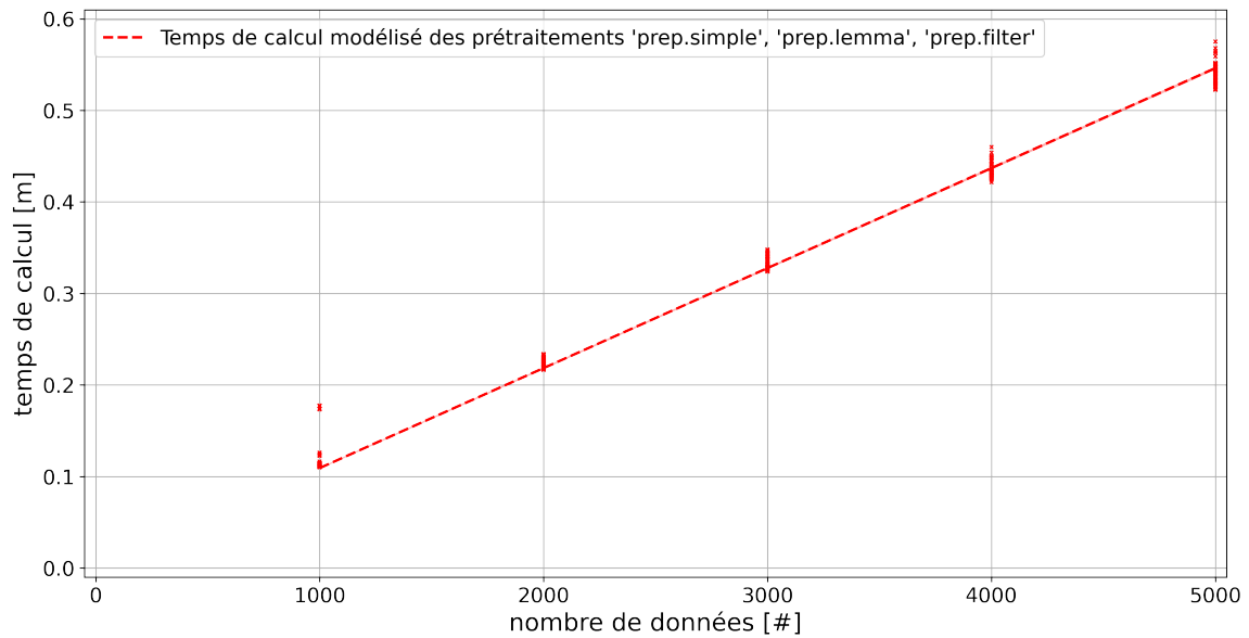
FIGURE 4.15 – Estimation du temps nécessaire (en minutes) pour effectuer une tâche de prétraitements en fonction du nombre de données à traiter. Les paramétrages prep.simple , prep.lemma et prep.filter ayant des temps de calculs similaires, leurs modélisations n'ont pas été séparées.
