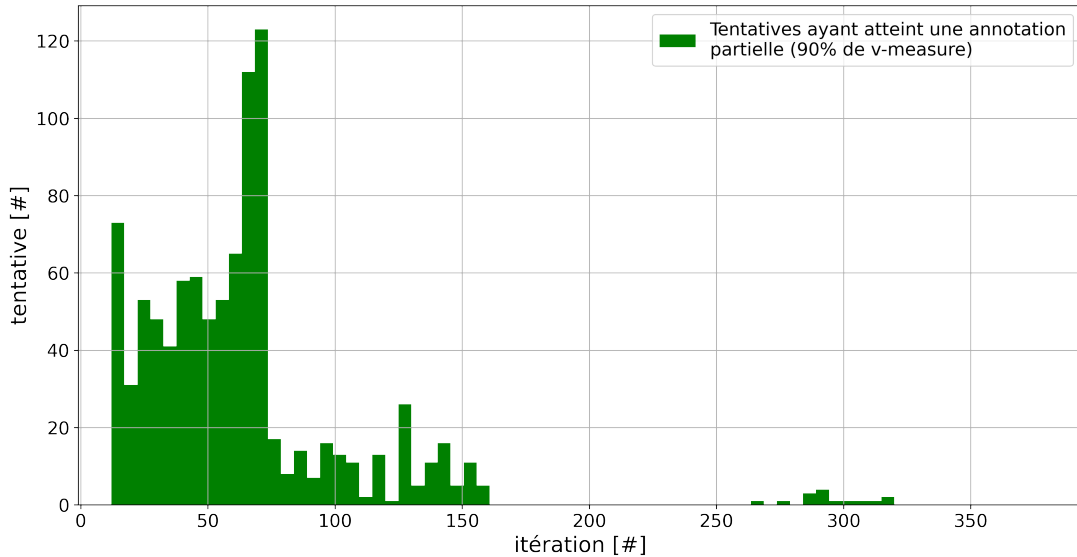
FIGURE 4.5 – Répartition des tentatives en fonction de l'itération de la méthode pour laquelle elles atteignent le seuil d'une annotation partielle, c'est-à-dire l'itération pour laquelle elles parviennent à 90% de v-mesure entre un résultat obtenu et la vérité terrain. L'histogramme est réduit à 60 pics pour simplifier l'affichage.
