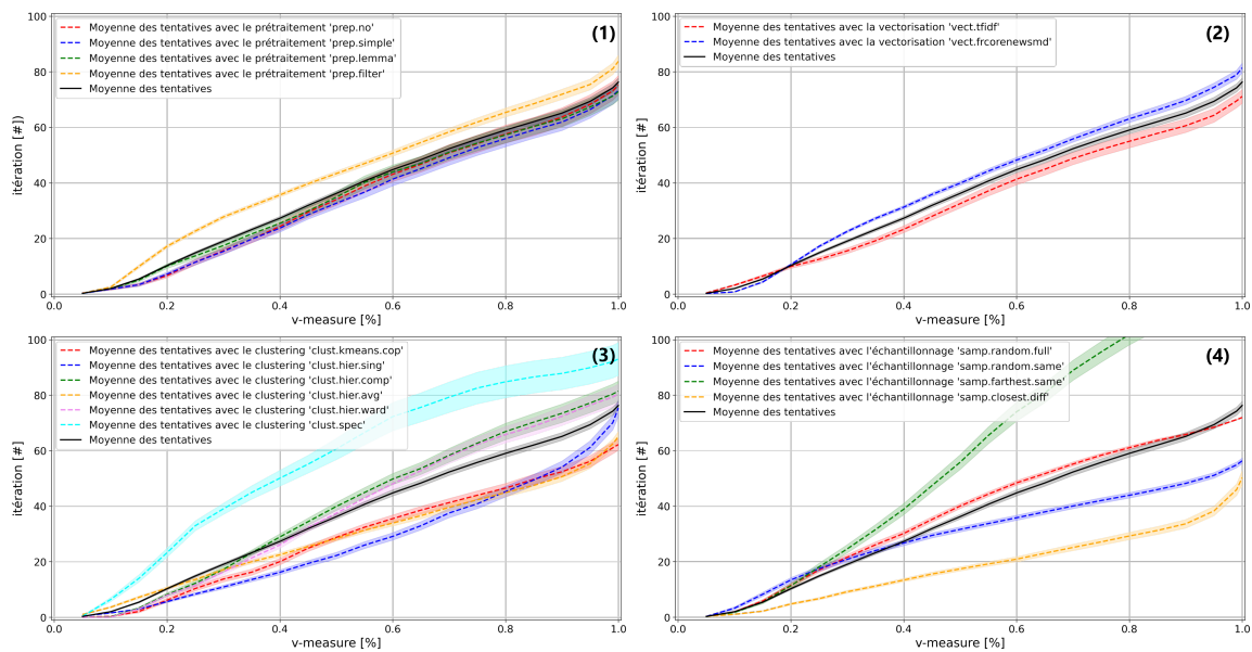
FIGURE 4.8 – Évolution des moyennes du nombre d'itérations nécessaire de la méthode de Clustering Interactif pour obtenir un seuil défini de v-measure entre un résultat obtenu et la vérité terrain, moyennes réalisées sur les différentes valeurs que peuvent prendre les facteurs analysés, affichées par facteur : (1) prétraitements, (2) vectorisation, (3) clustering et (4) échantillonnage.
