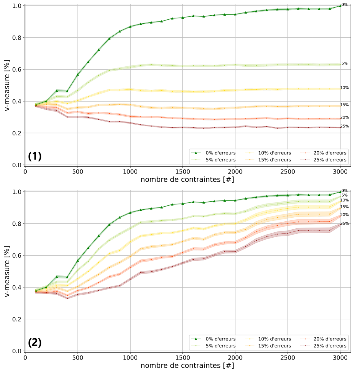
FIGURE 4.31 – Évolution des similitudes moyennes (calculées en terme de v -mesure) des résultats de clustering des tentatives introduisant des erreurs d'annotation par rapport à la vérité terrain au cours des itérations. Les dégradés de couleurs des courbes représentent les déclinaisons de ces évolutions en fonction des différents taux d'annotations erronées (allant de 0% et 25%). (1) représente l'approche naïve ignorant les conflits d'annotation et (2) représente l'approche corrigeant les conflits détectés par le gestionnaire de contraintes. Toutes les courbes sont tronquées à 3 000 contraintes (nombre maximum de contraintes nécessaires à une tentative n'introduisant pas d'erreurs pour converger vers la vérité terrain).
