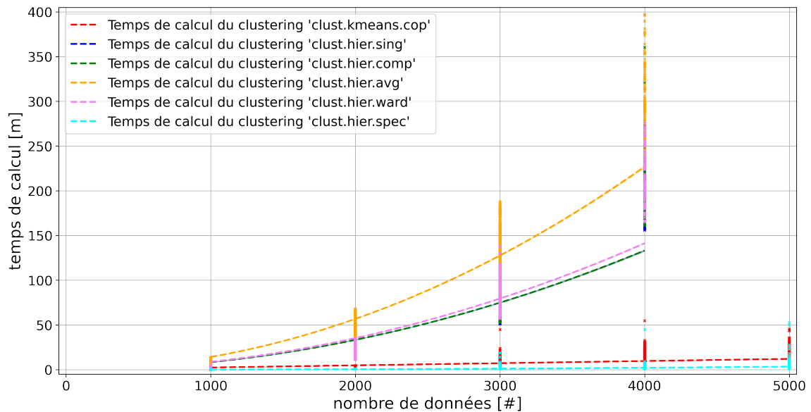
FIGURE 4.17 – Estimation du temps nécessaire (en minutes) pour effectuer une tâche de clustering en fonction du nombre de données à traiter.
