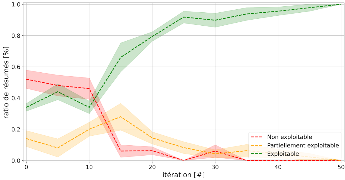
FIGURE 4.25 – Évolution de la pertinence métier moyenne en fonction du nombre d’itérations de la méthode. Cette pertinence, exprimée en proportion du nombre de clusters, est estimée sur la base du résumé automatique des clusters par un large modèle de langage et est retranscrite en trois niveaux : exploitable en vert, partiellement exploitable en orange, et non exploitable en rouge.
