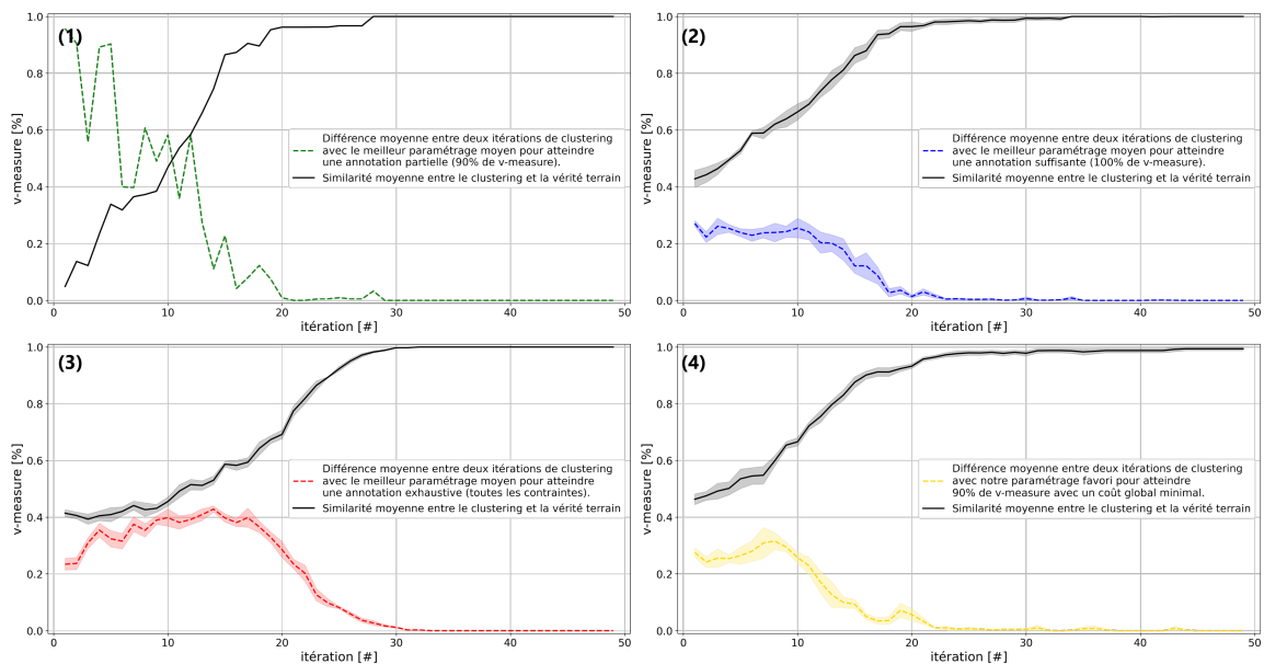
FIGURE 4.29 – Évolution de la différence de résultats entre deux itérations de clustering. Les évolutions moyennes de différents paramétrages de la méthode sont exposées : (1) meilleur paramétrage moyen pour atteindre une annotation partielle ; (2) meilleur paramétrage moyen pour atteindre une annotation suffisante ; (3) meilleur paramétrage moyen pour atteindre une annotation exhaustive ; et (4) paramétrage favori. À titre d'information, les courbes en noir représentent l'évolution de la v-mesure entre le clustering et la vérité terrain.
