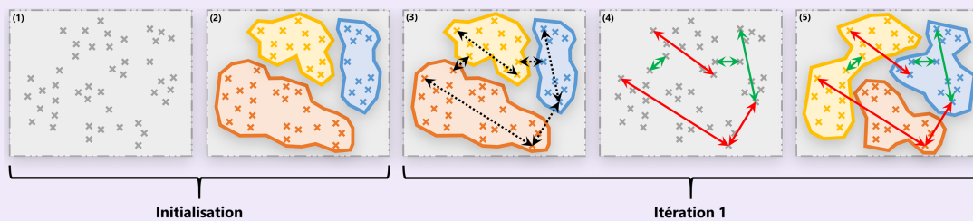
FIGURE 3.2 – Exemple d'une itération de Clustering Interactif.
