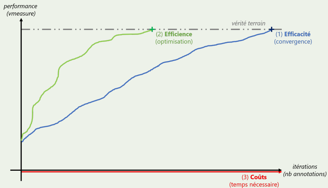
FIGURE 4.10 – Illustration des études réalisées sur le Clustering Interactif (étape 3/6) en schématisant l'évolution de la performance (accord avec la vérité terrain calculé en v-measure ) d'une base d'apprentissage en cours de construction en fonction du coût temporel de la méthode (temps nécessaire à l'expert métier et à la machine).
