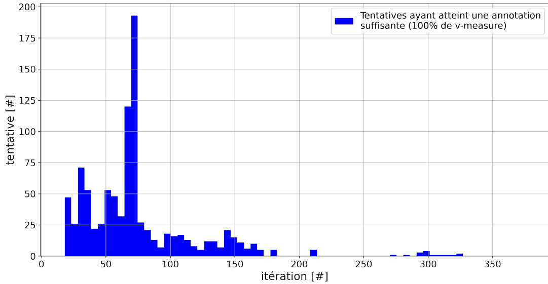
FIGURE 4.6 – Répartition des tentatives en fonction de l'itération de la méthode pour laquelle elles atteignent le seuil d'une annotation suffisante, c'est-à-dire l'itération pour laquelle elles parviennent à 100% de v -mesure entre un résultat obtenu et la vérité terrain. L'histogramme est réduit à 60 pics pour simplifier l'affichage.
