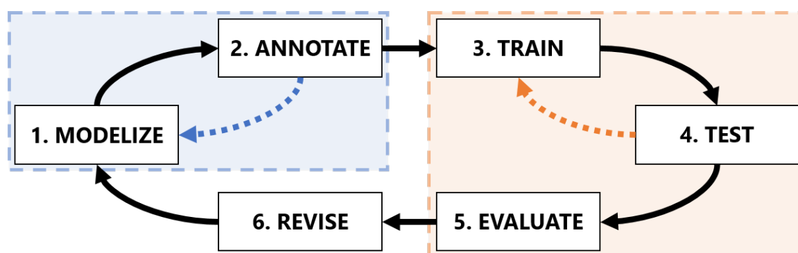
FIGURE 2.4 – Cycle MATTER structurant un projet d'annotation en six étapes principales : Modelize , Annotate , Train , Test , Evaluate et Revise .
