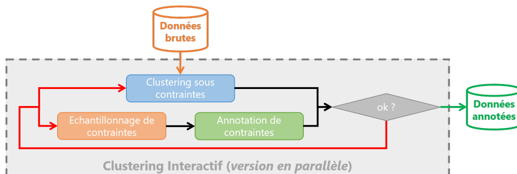
FIGURE 5.3 – Schéma illustrant l'architecture du Clustering Interactif en mode parallèle.
