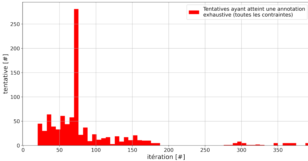
FIGURE 4.7 – Répartition des tentatives en fonction de l'itération de la méthode pour laquelle elles atteignent le seuil d'une annotation exhaustive, c'est-à-dire l'itération pour laquelle toutes les contraintes possibles entre les données ont été annotées. L'histogramme est réduit à 60 pics pour simplifier l'affichage.
