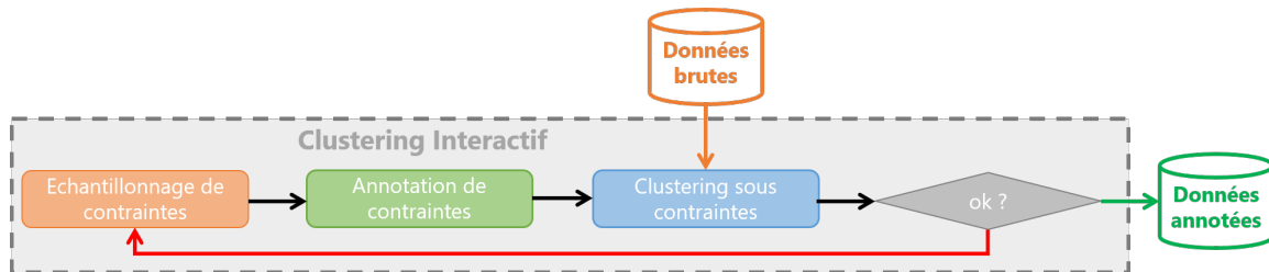
FIGURE 3.1 – Schéma illustrant l'architecture du Clustering Interactif. La boucle principale enchaîne un échantillonnage de paires de données, une annotation de contraintes, et un clustering sous contraintes.
