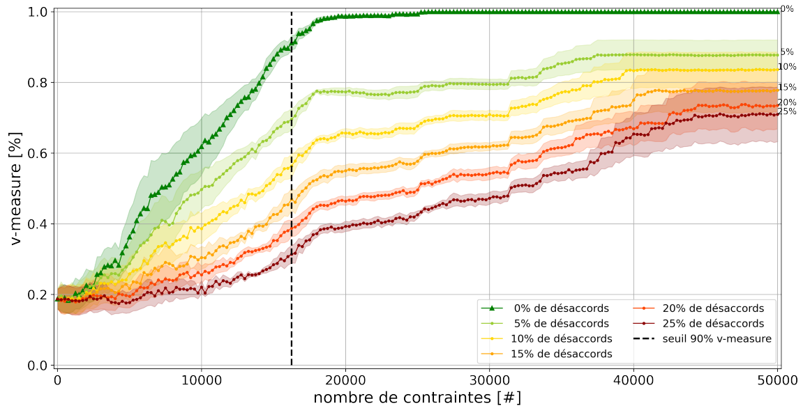
FIGURE 4.32 – Exemple d’une évolution de similitudes moyennes (calculées en terme de v-mesure ) de résultats de clustering de tentatives introduisant des différences d’annotation par rapport à la vérité terrain au cours des itérations, vérité terrain ayant ici une taille de 5 000 données. Les dégradés de couleurs des courbes représentent les déclinaisons de ces évolutions en fonction des différents taux d’annotations divergentes (allant de 0% et 25%). La barre verticale indique le nombre moyen de contraintes nécessaires aux tentatives n’introduisant pas de désaccords pour obtenir un score de 90% de v-mesure (ici : 16 250 contraintes).
