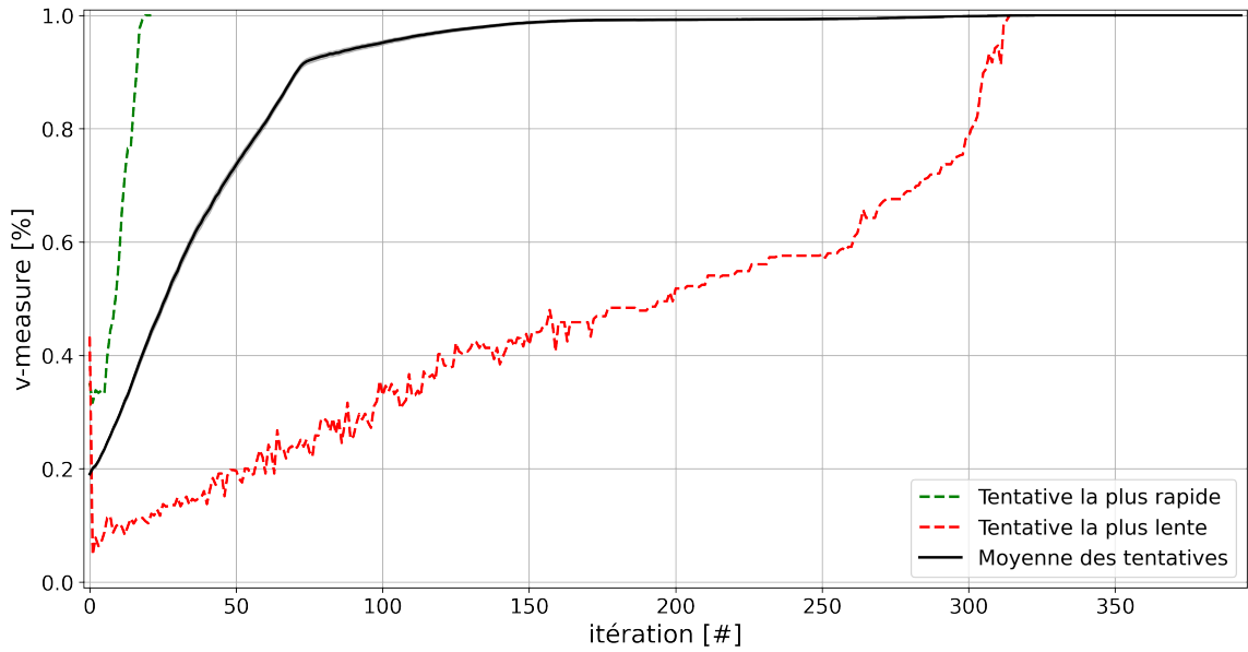
FIGURE 4.3 – Évolution de la moyenne de la v -mesure entre un résultat obtenu et la vérité terrain en fonction du nombre d'itérations de la méthode de Clustering Interactif , moyenne réalisée itération par itération sur l'ensemble des tentatives. Représentation des tentatives ayant été les plus rapides (des prétraitements prep.simple , une vectorisation vect.tfidf , un clustering clust.hier.comp ou clust.hier.ward , et un échantillonnage samp.closest.diff ) et les plus lentes (un prétraitement prep.no , une vectorisation vect.tfidf , un clustering clust.spec , et un échantillonnage de contraintes samp.farthest.same ) pour atteindre 100% de v -mesure.
