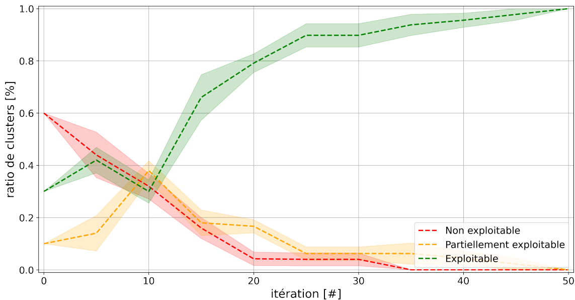
FIGURE 4.24 – Évolution de la pertinence métier moyenne estimée manuellement au cours des itérations du résultat du Clustering Interactif avec notre paramétrage favori. Cette pertinence, exprimée en proportion du nombre de clusters, est retranscrite en trois niveaux : exploitable en vert, partiellement exploitable en orange, et non exploitable en rouge.
