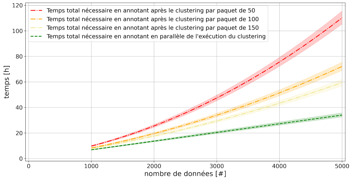
FIGURE 4.22 – Estimation du temps total nécessaire (en heures) pour modéliser un jeu de données avec notre paramétrage favori du Clustering Interactif afin d'obtenir une annotation partielle (atteindre une v-measure de 90%), en fonction de plusieurs tailles de jeu de données, plusieurs tailles de lots d'annotation, et mettant en opposition l'approche séquentielle (annotation puis le clustering) et l'approche parallèle (annotation pendant le clustering).
