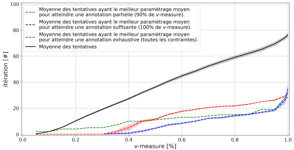
FIGURE 4.9 – Évolution des moyennes du nombre d'itérations nécessaire de la méthode de Clustering Interactif pour obtenir un seuil défini de v-mesure entre un résultat obtenu et la vérité terrain, moyennes réalisées sur les différents seuils d'annotations étudiés : l'annotation partielle (atteindre une v-mesure de 90%), l'annotation suffisante (atteindre une v-mesure de 100%) et l'annotation exhaustive (annoter toutes les contraintes possibles).
