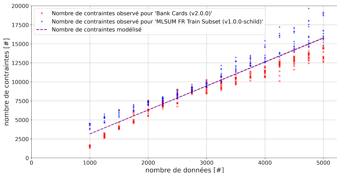
FIGURE 4.19 – Estimation du nombre moyen de contraintes nécessaires à notre paramétrage favori du Clustering Interactif afin d'obtenir une annotation partielle (atteindre une v-measure de 90%) en fonction de la taille du jeu de données à modéliser.
