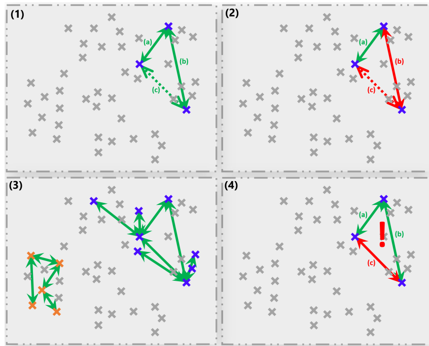
FIGURE C.1 – Exemples des propriétés de transitivité des contraintes MUST-LINK (flèches vertes) et CANNOT-LINK (flèches rouges). (1) et (2) représentent les possibilités de déduction d'une contrainte ((c)) en fonction des deux autres ((a) et (b)). (3) représente deux composants connexes définis par la transitivité des contraintes MUST-LINK . Enfin, (4) représente un cas de conflit où une contrainte ((c)) ne correspond pas à sa déduction faite à partir des autres contraintes ((a) et (b)).
