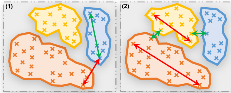
FIGURE 4.27 – Exemples d'accords et de désaccords entre les annotations d'une itération et le résultat du clustering de l'itération précédente. Des contraintes MUST-LINK (flèches vertes) et CANNOT-LINK (flèches rouges) sont représentées dans deux situations : (1) montre des cas d'accords ( MUST-LINK dans un même cluster, CANNOT-LINK entre deux clusters différents), et (2) montre des cas de désaccords ( MUST-LINK entre deux clusters différents, CANNOT-LINK dans un même cluster).
