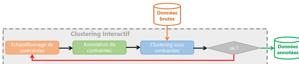
FIGURE 5.1 – Schéma illustrant l'architecture du Clustering Interactif .
