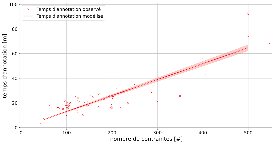
FIGURE 4.13 – Estimation du temps nécessaire (en minutes) pour annoter un lot de contraintes.
