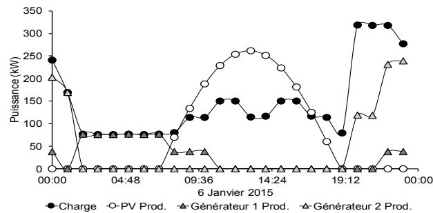
A : stratégie « Cycle Charging »
