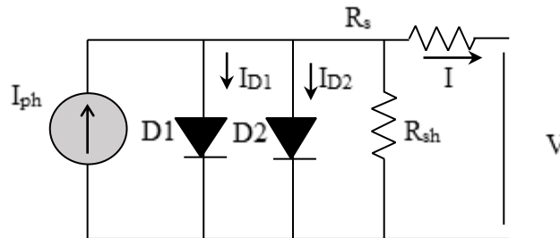
Figure 16. Modèle à deux diodes
