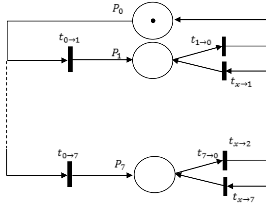
Figure 34. Réseau de Petri (PN1)
