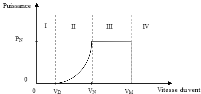
Figure 8. Caractéristique vent-puissance des éoliennes
