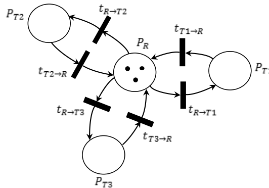
Figure 35. Réseau de Petri (PN2)
