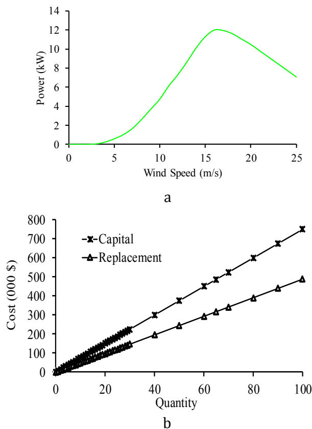
Figure 27. Courbe de puissance du SCEE (a) et Evolution du coût avec la quantité de SCEE (b)
