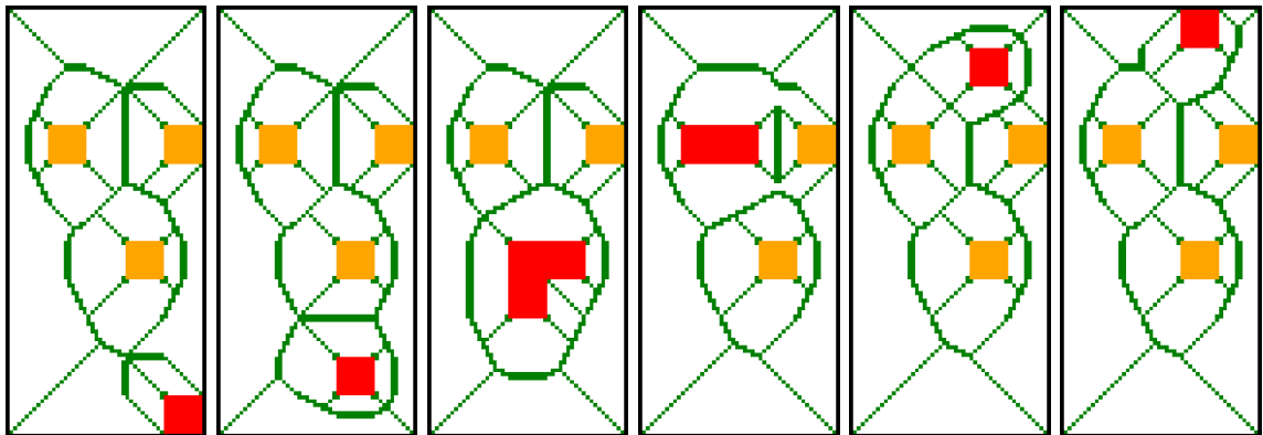
(c) Le diagramme de Voronoï extrait lorsqu'une personne entre dans la scène en bas à droite, s'assied sur une chaise, et quitte la scène par le côté en haut à droite. Les obstacles dynamiques et statiques sont représentés comme des carrés rouges et oranges, respectivement. Les chemins les plus sûrs sont indiqués en vert.
