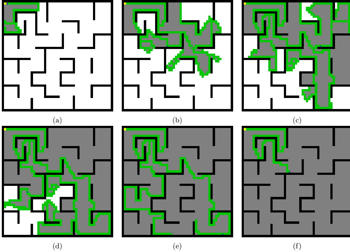
Figure A.7 – Exploration effectuée par deux agents, qui utilisent un algorithme stigmergique proposé, appelé BMILRV. Le point de rendez-vous est situé dans le coin en haut à gauche de la carte.
