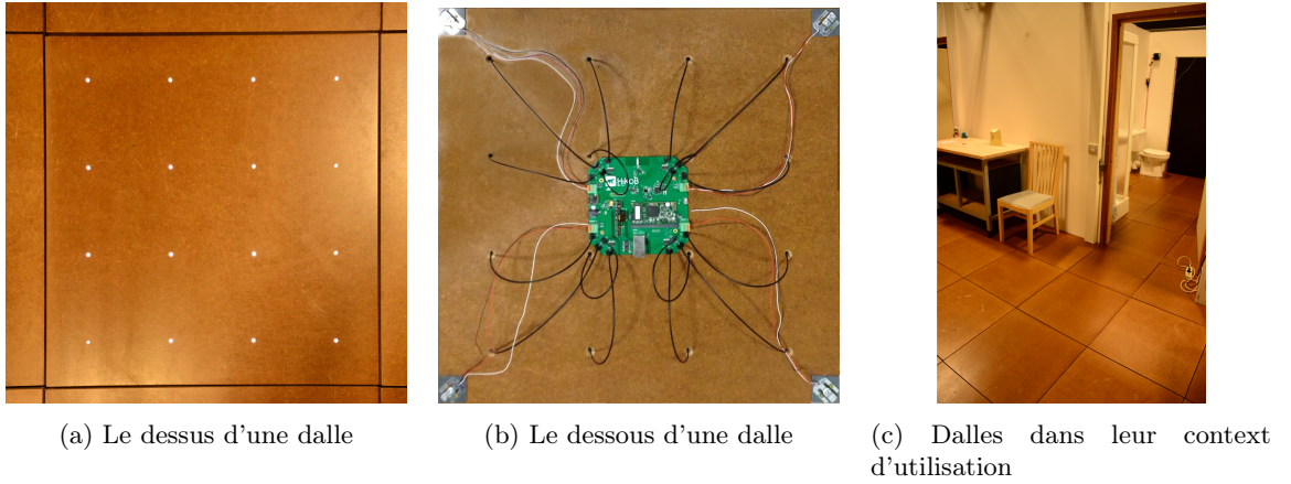
Figure A.2 – Les dalles de mesure de pression. La vue d'en bas montre les capteurs localisés dans les coins, ainsi que l'unité de calcul visible au milieu. Les câbles noirs alimentent les 16 LEDs utilisées pour fournir un retour visuel.
