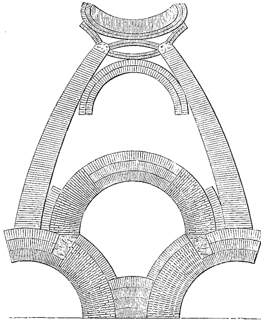
KONSTRUKTION DER KUPPEL DES PANTHEONS.
