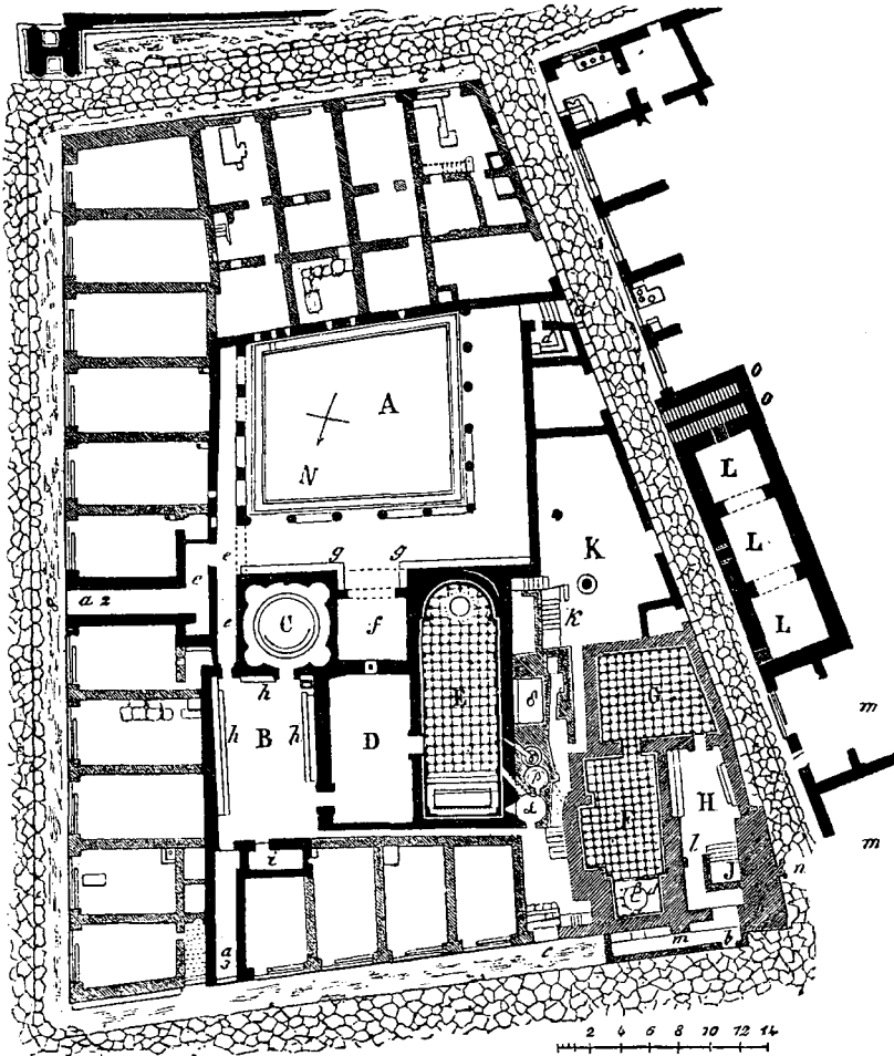
GRUNDRISS DER ÄLTEREN THERMEN ZU POMPEJI.
