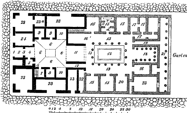
SCHEMA EINES ITALISCHEN (POMPEJANISCHEN) WOHNHAUSES.
