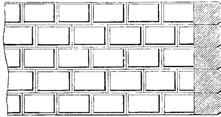
QUADERMAUERWERK.
