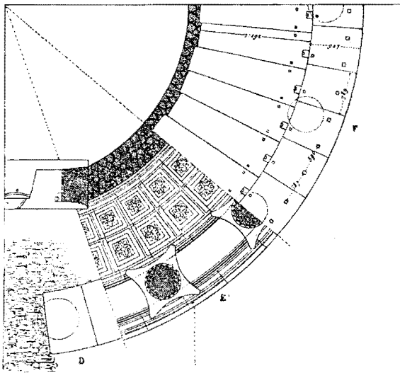
THÜR, KASSETTENBILDUNG UND STÜCK DER ANSICHT DES VESTATEMPELS VON OBEN.
