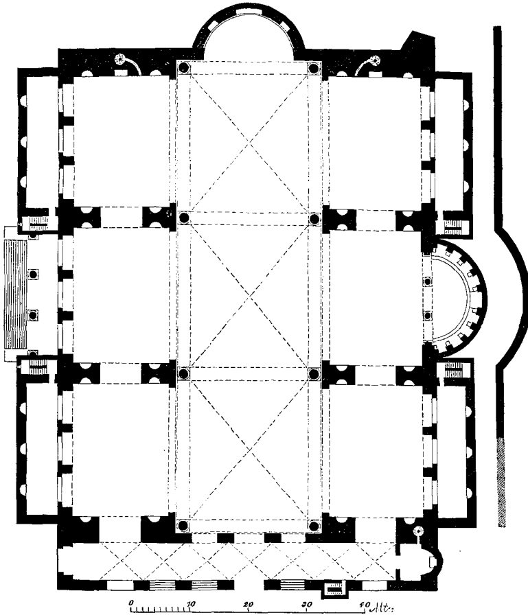
GRUNDRISS DER BASILIKA DES CONSTANTIN UND MAXENTIUS.
