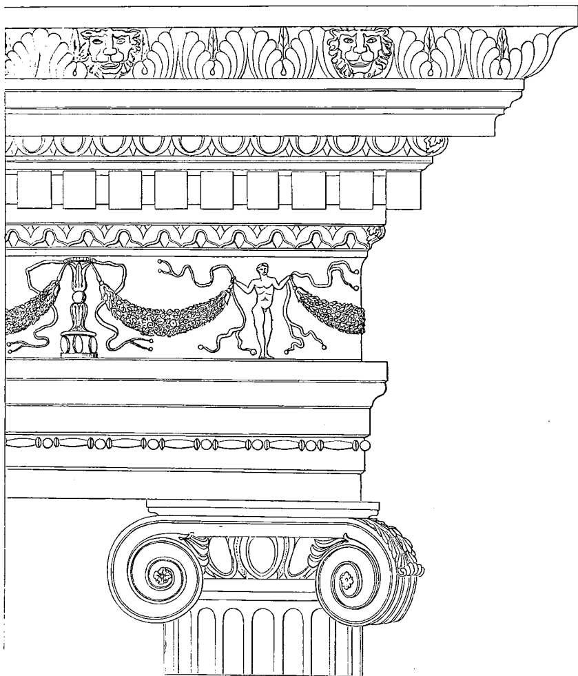
KAPITÄL UND GEBÄLK VOM TEMPEL DER FORTUNA VIRILIS ZU ROM.
