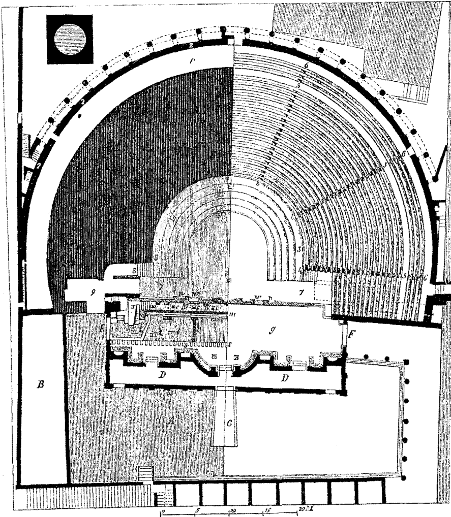
GRUNDRISS DES GROSSEN THEATERS IN POMPEJI.
