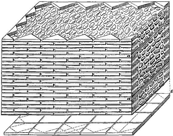
MIT ZIEGELSTEINEN VERBLENDETES EMPEKTON.
