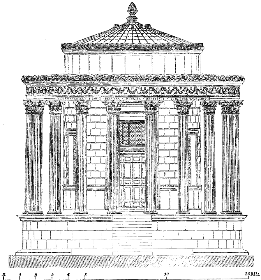
RESTAURIERTE ANSICHT DES VESTATEMPELS ZU TIVOLI.
