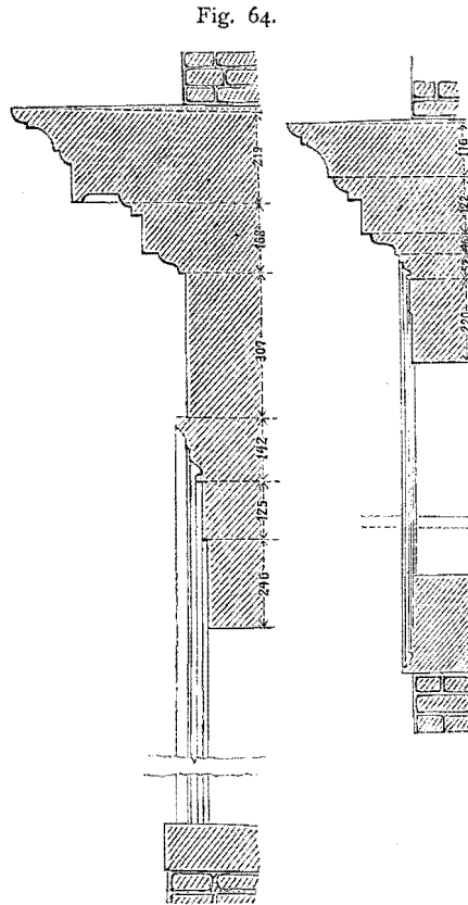
PROFILE DES THÜR- UND FENSTERRAHMENS VOM VESTATEMPEL ZU TIVOLI.
