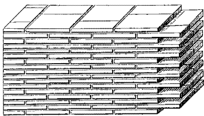
RÖMISCHE ZIEGELSTEINVERBÄNDE.
