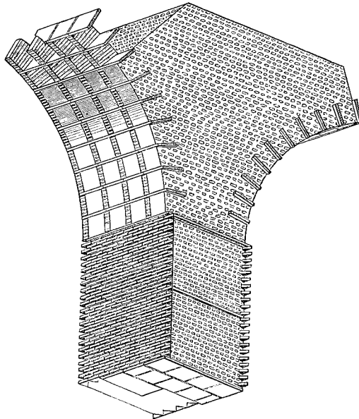
GEWÖLBE MIT ZELLENBOGEN.
