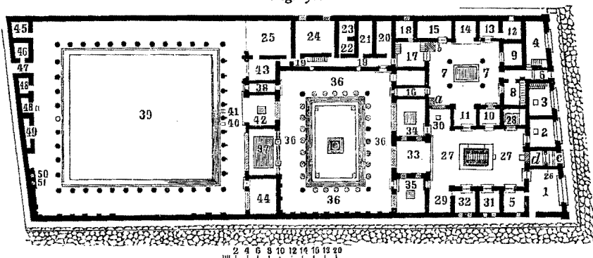
GRUNDRISS EINES PALASTARTIGEN POMPEJANISCHEN WOHNHAUSES (DER CASA DEL FAUNO).
