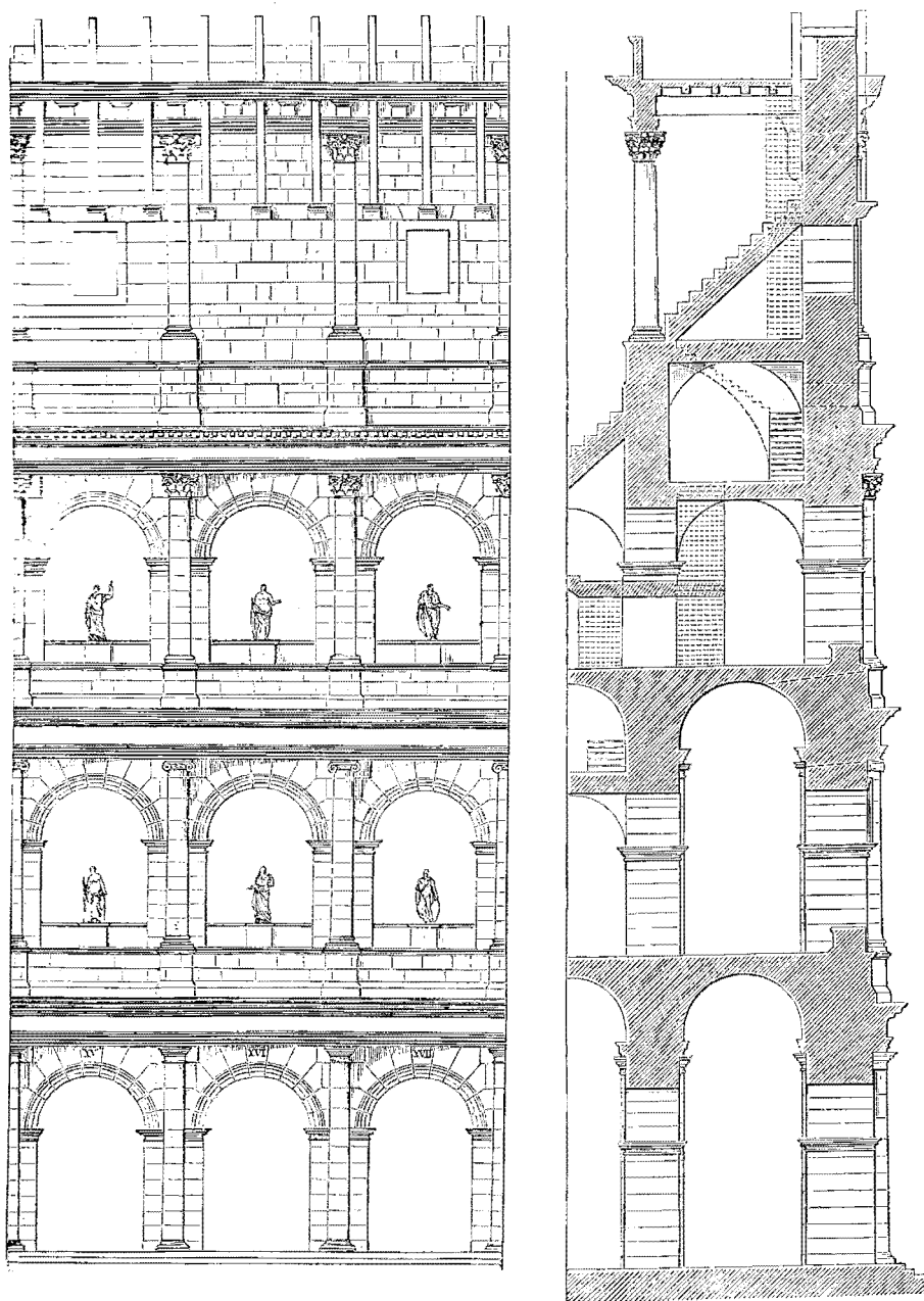
VOM SOG. COLOSSEUM.
