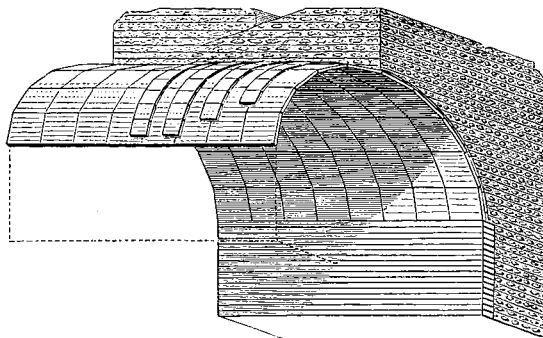
GEWÖLBE MIT STEINSCHALE.
