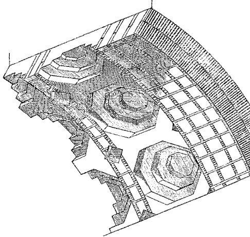
KASSETTENBILDUNGEN.
