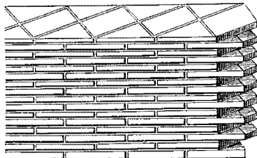
RÖMISCHE ZIEGELSTEINVERBÄNDE.
