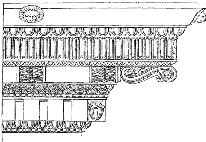
KRANZGESIMS VOM TEMPEL DER DIOSKUREN.
