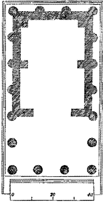
GRUNDRISS DES TEMPELS DER FORTUNA VIRILIS.
