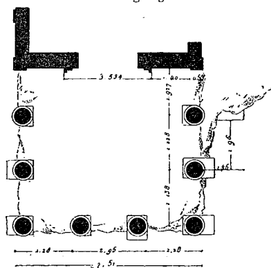
GRUNDRISS ZU FIG. 22.
