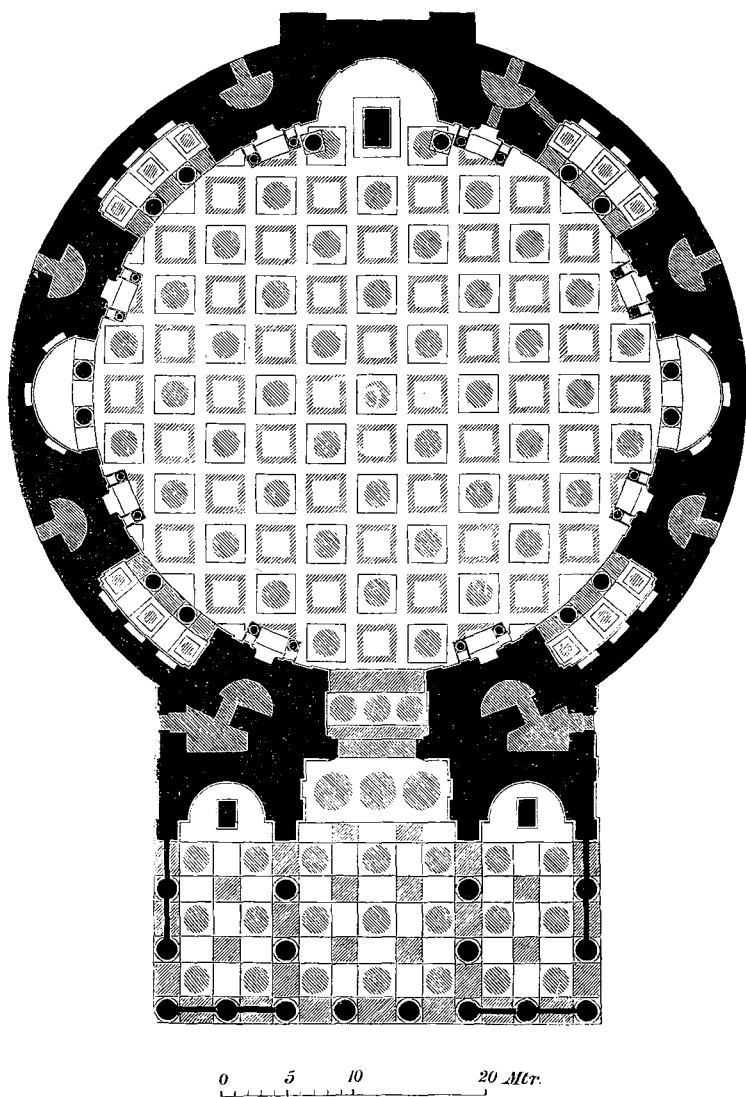
GRUNDRISS DES PANTHEONS.
