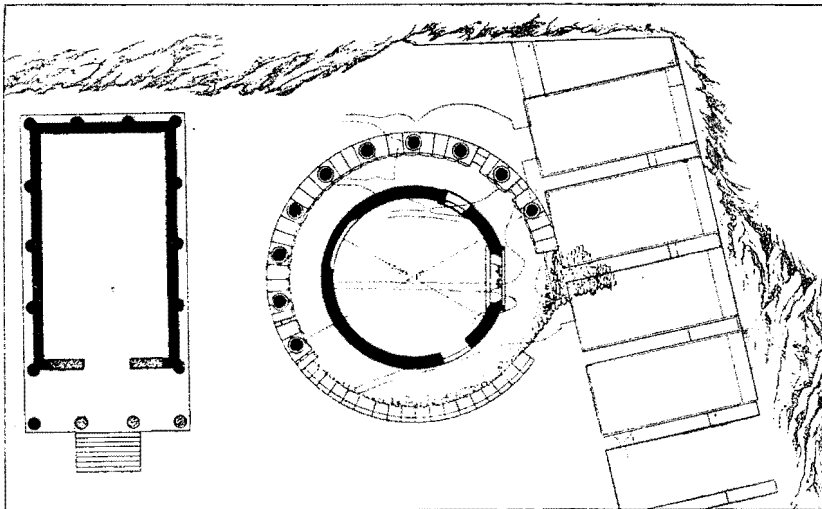
GRUNDRISS DES TEMPELS DER VESTA (UND SIBYLLA) ZU TIVOLI.
