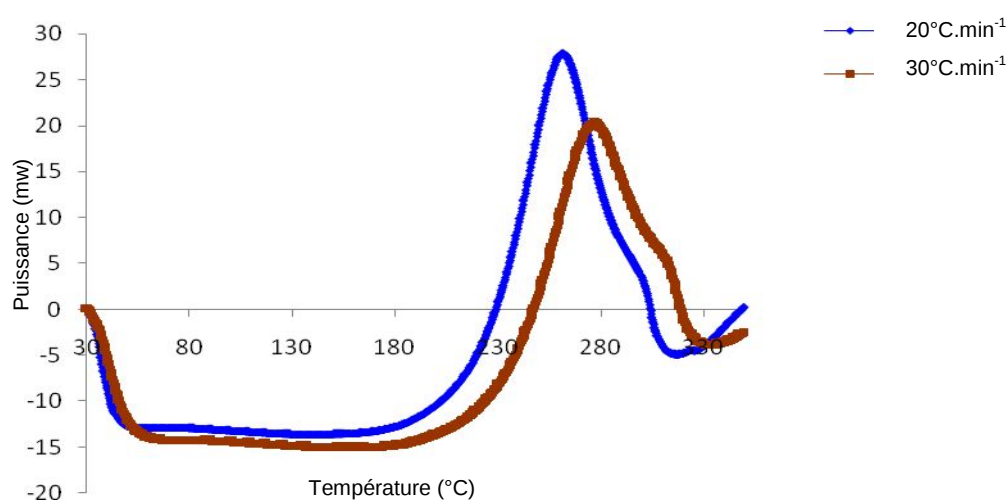
Figure IV.3 : DSC de la RTM6 à 20^{\circ}\text{C.min}^{-1} et 30^{\circ}\text{C.min}^{-1}
