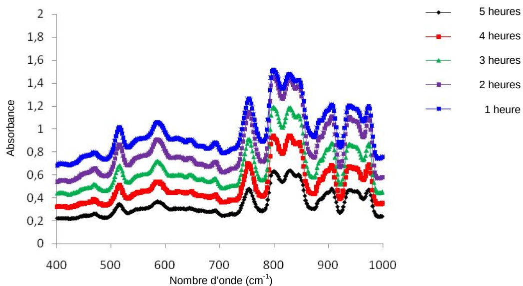
Secteur 1 (1000-400 \text{cm}^{-1} ) spectres Infra-rouge de la RTM6 à 100°C
