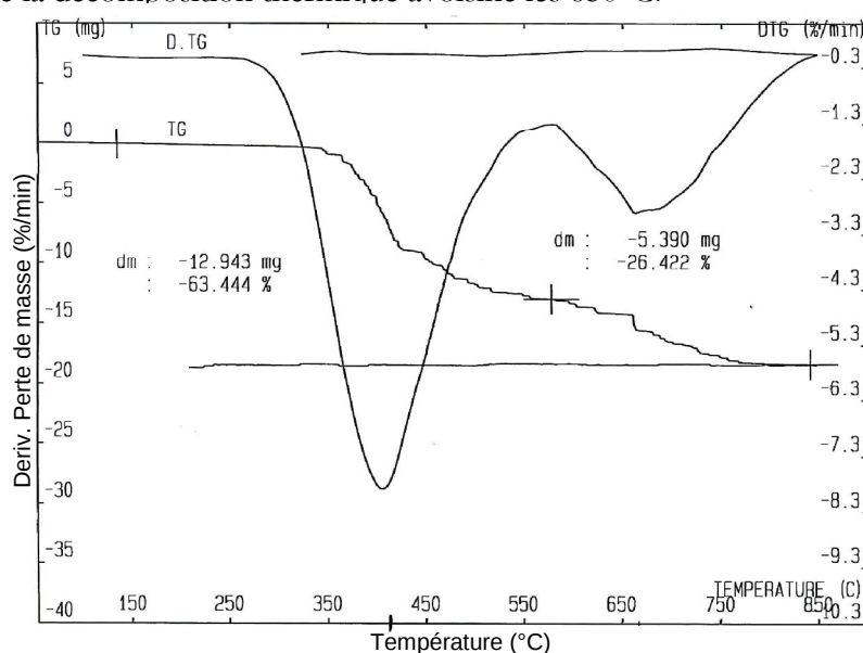
Figure IV.22 : Courbes de DTG de l'échantillon à 10^{\circ}\text{C}.\text{min}^{-1}
