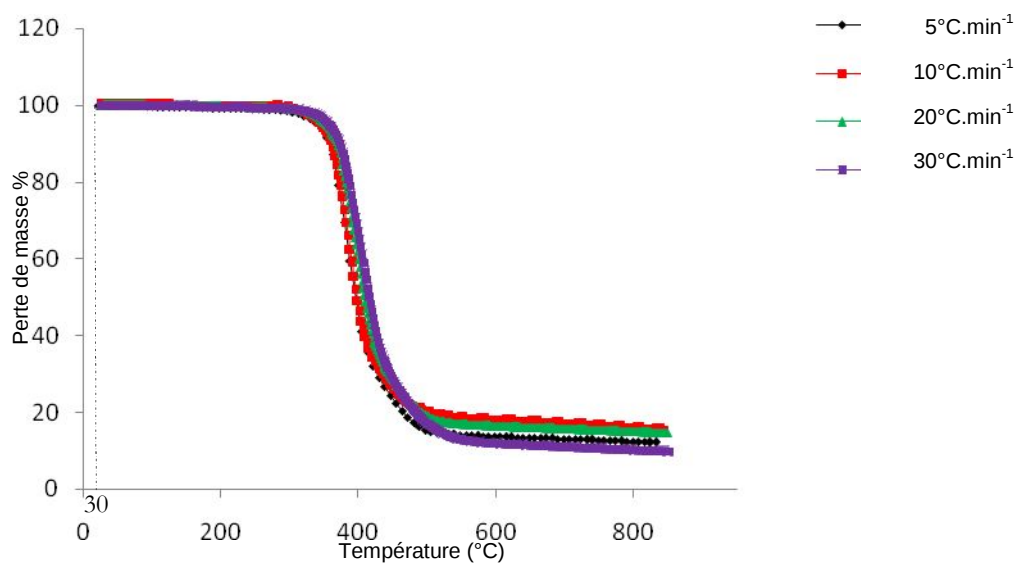
Figure IV.26 : ATG pour la RTM6 à 5% de \text{TiO}_2 à 5, 10, 20 et 30°C.min -1
