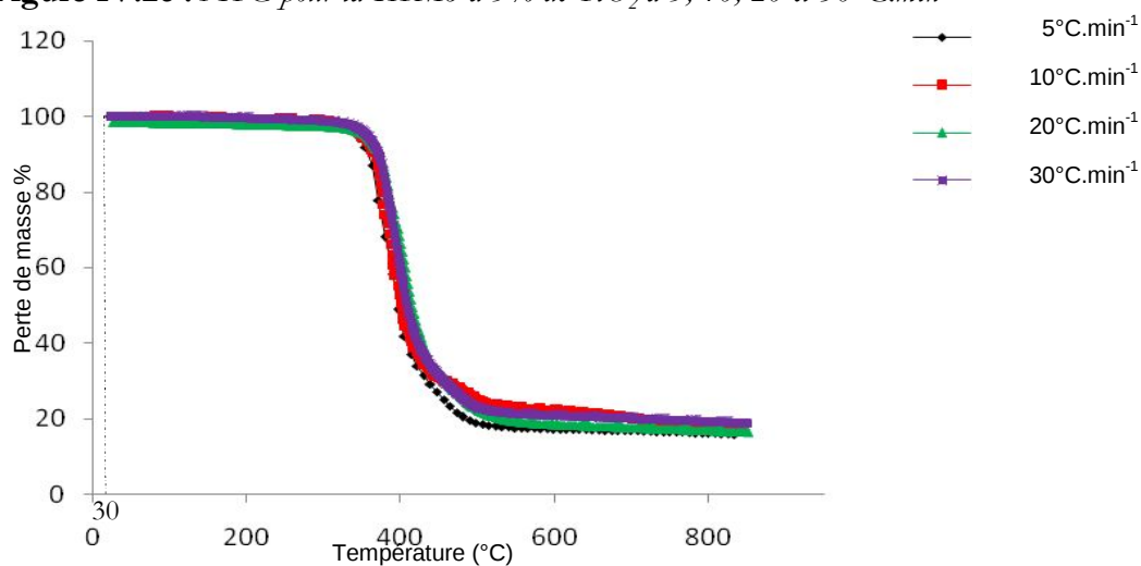
Figure IV.27 : ATG pour la RTM6 à 10% de \text{TiO}_2 à 5, 10, 20 et 30°C.min -1
