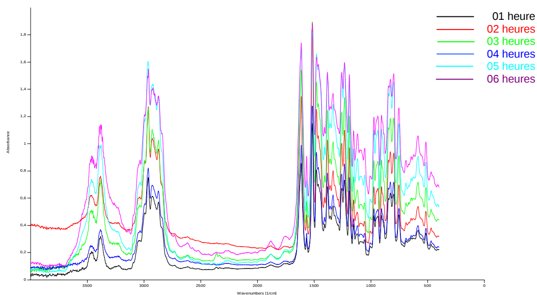
Figure IV.34 : Spectres Infra-rouge de la RTM6 de 01 à 06 heures à 100°C
