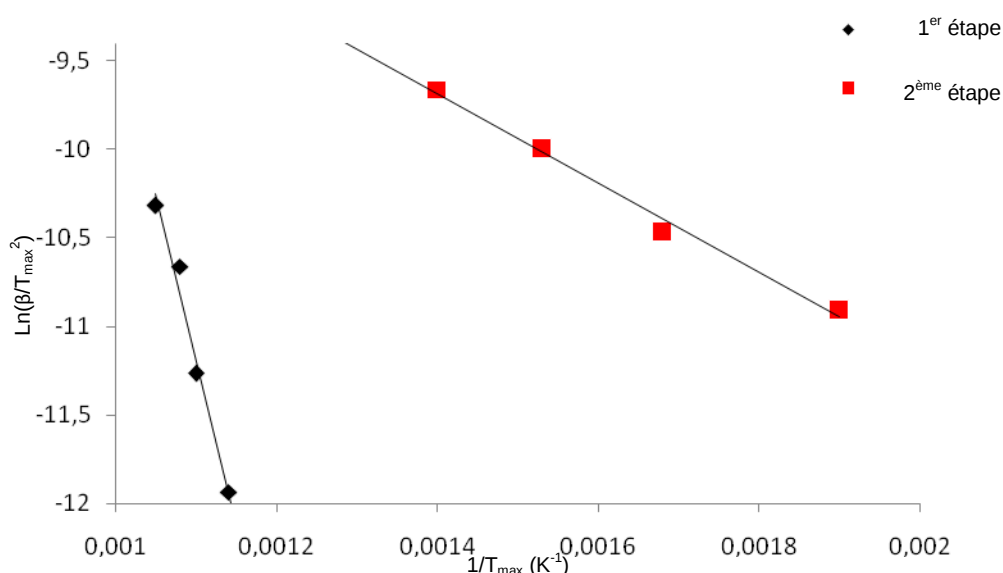
Figure IV.30 : Variation de \ln(\beta/T_{\text{max}}^2) en fonction de 1/T_{\text{max}} de la RTM6 avec \text{TiO}_2 pour le calcul de l'énergie d'activation par la méthode de Kissinger
