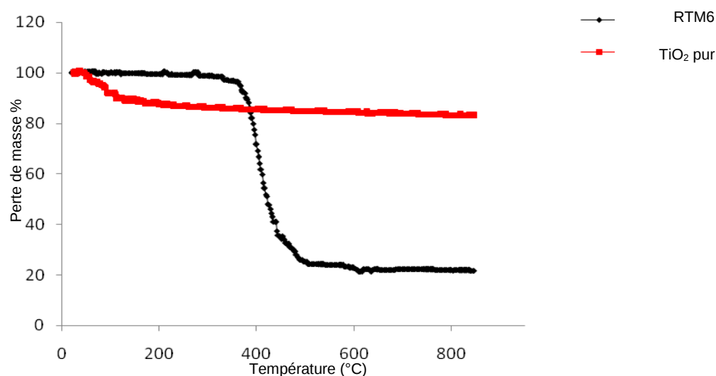
Figure IV.21 : ATG pour RTM6 et \text{TiO}_2 pur à 10^{\circ}\text{C}.\text{min}^{-1}
