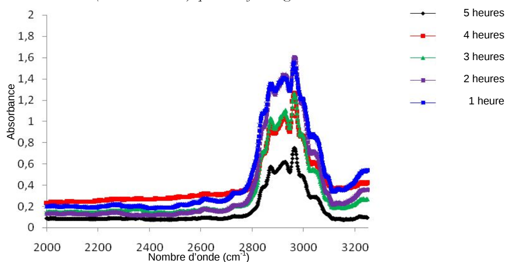
Secteur 3 (3250-2000 \text{cm}^{-1} ) spectres Infra-rouge de la RTM6 à 100°C
