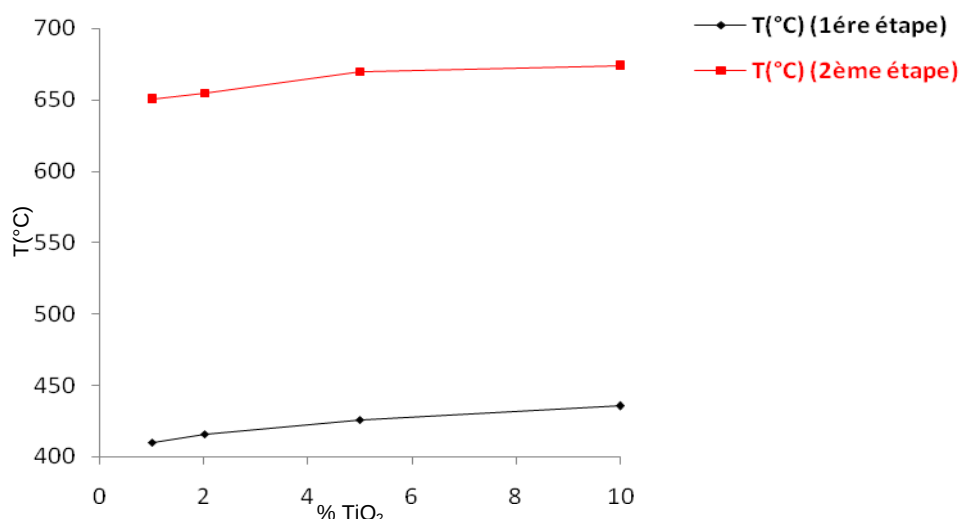
Figure IV.29 : Variation de T en fonction du taux de \text{TiO}_2
