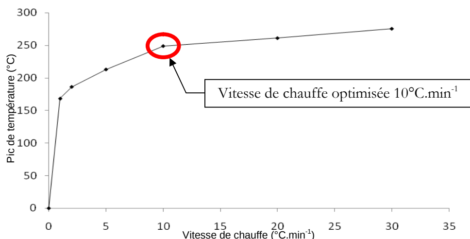
Figure IV.4 : Variation du pic de température en fonction de la vitesse de chauffe
