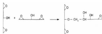
Figure II.7 : Structure chimique de la réaction 3
