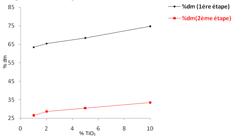
Figure IV.28 : Variation de dm en fonction du taux de \text{TiO}_2
