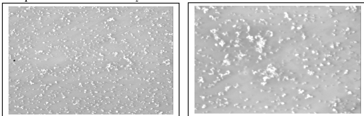
Figure IV.15 a : MEB de la RTM6 au cœur de l'échantillon à 1% de \text{TiO}_2
