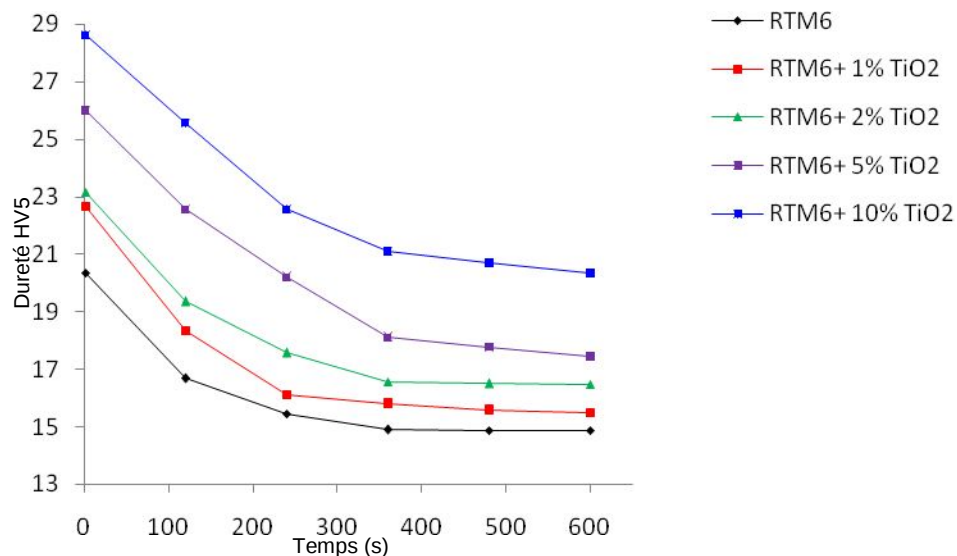
Figure IV.59 : Influence du taux de \text{TiO}_2 sur la dureté de la résine
