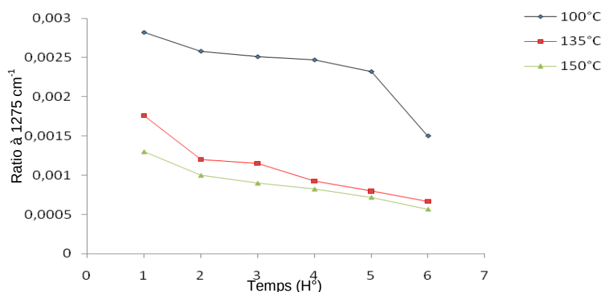
Figure IV.53 : Variation du ratio à ( A_{1275} / Aire totale du spectre) en fonction du temps à différentes températures
