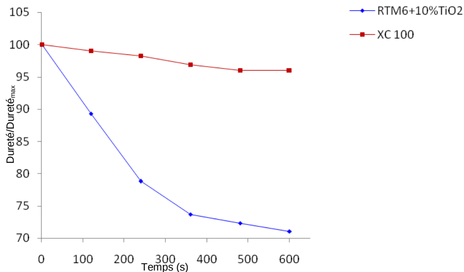
Figure IV.60 : Comparaison de l'influence du temps sur la dureté de la RTM6+10% \text{TiO}_2
