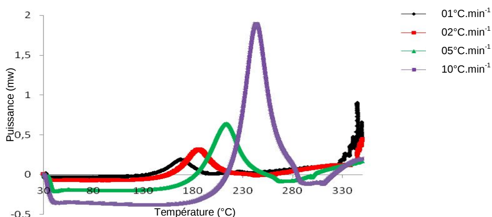
Figure IV.2 : DSC de la RTM6 à 1^{\circ}\text{C.min}^{-1} , 2^{\circ}\text{C.min}^{-1} , 5^{\circ}\text{C.min}^{-1} , 10^{\circ}\text{C.min}^{-1}
