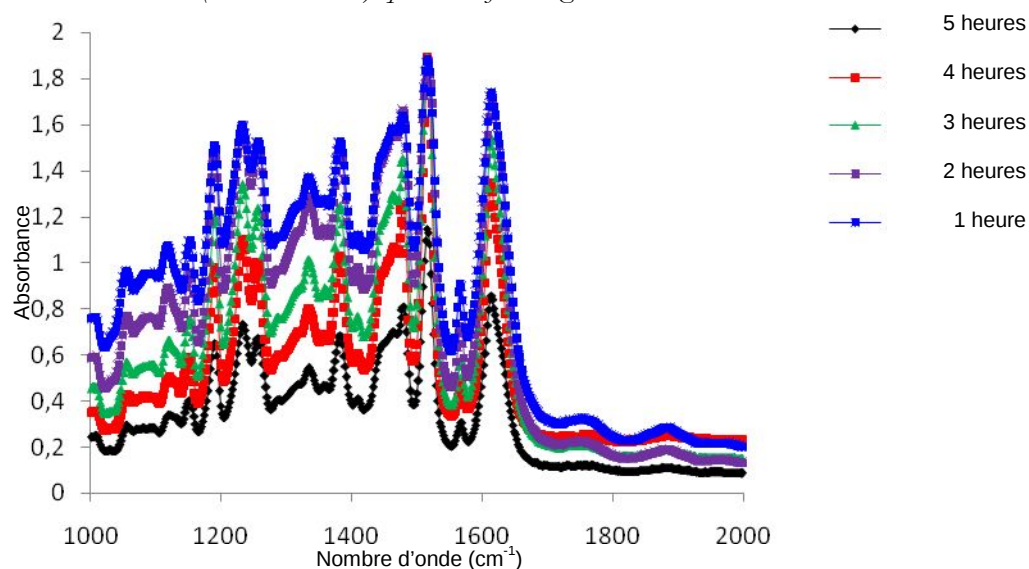
Secteur 2 (2000-1000 \text{cm}^{-1} ) spectres Infra-rouge de la RTM6 à 100°C
