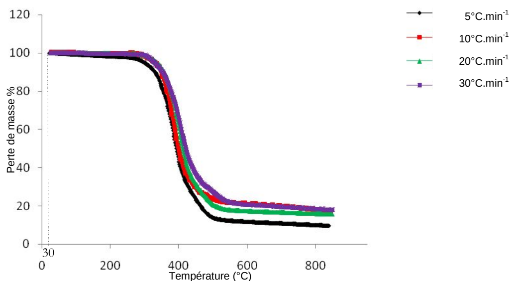
Figure IV.25 : ATG pour la RTM6 à 2% de \text{TiO}_2 à 5, 10, 20 et 30^\circ\text{C}.\text{min}^{-1}
