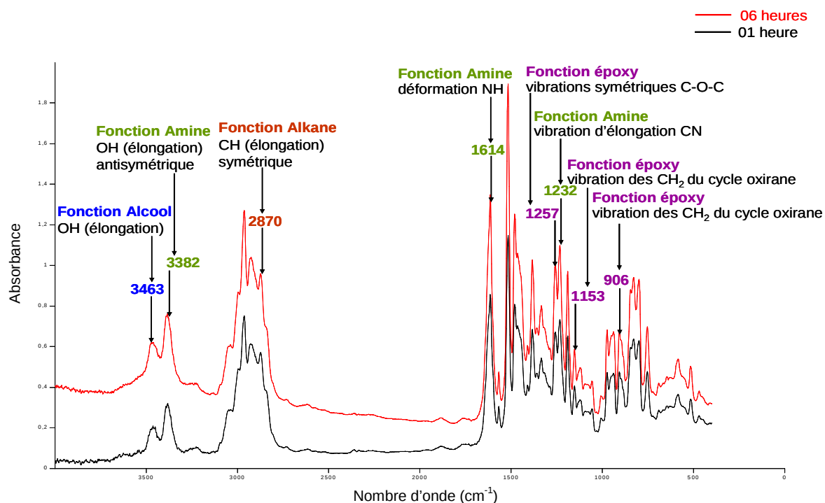
Figure IV.35 : Spectre Infra-Rouge de la RTM6 de 01 Heure et 06 Heures à 100°C
