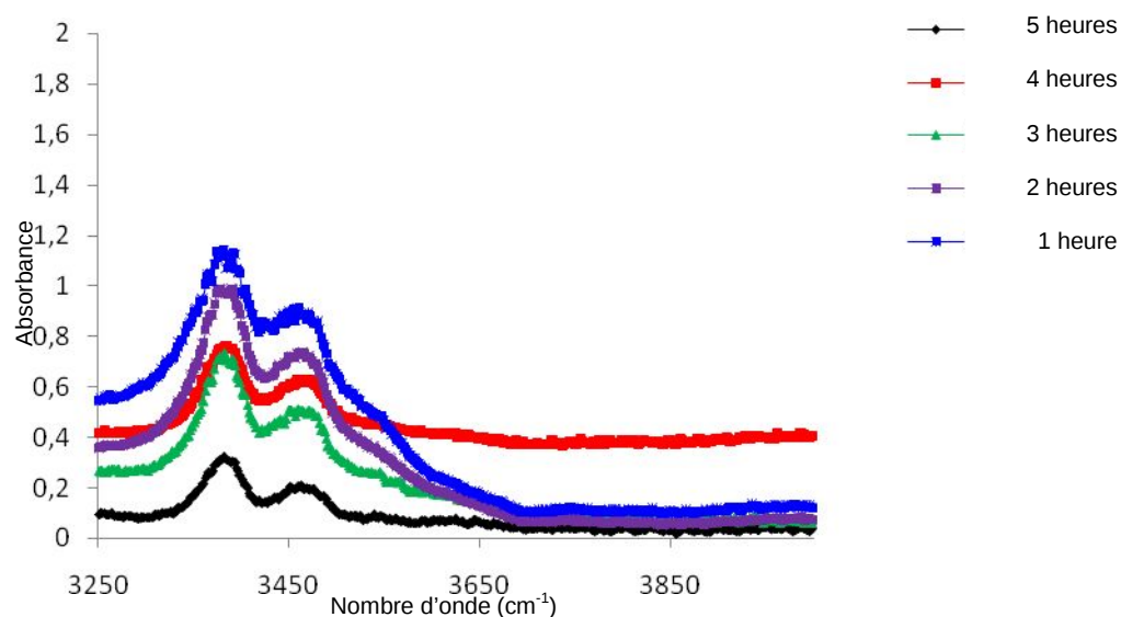
Figure IV.34 : Spectres Infra-rouge de la RTM6 à 100°C
