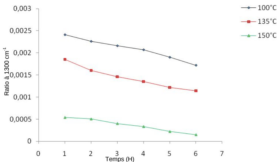
Figure IV.58 : Variation du ratio à ( A_{1300}/\text{Aire totale du spectre} ) par rapport au temps à différentes températures
