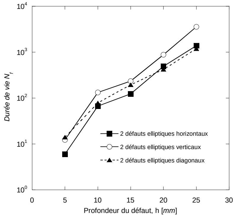
Figure 3-80. Durée de vie en fonction de la profondeur pour les trois configurations de défauts elliptiques ( F = 12\text{ MN / m} ).
