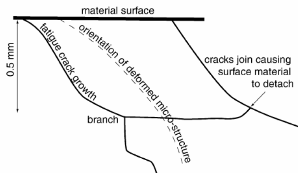
Figure 1-5. Représentation schématisée de la propagation de fissures de fatigue amorcées en surface dans les roues. Un fois amorcée, la fissure dévient vers une direction presque radiale.
