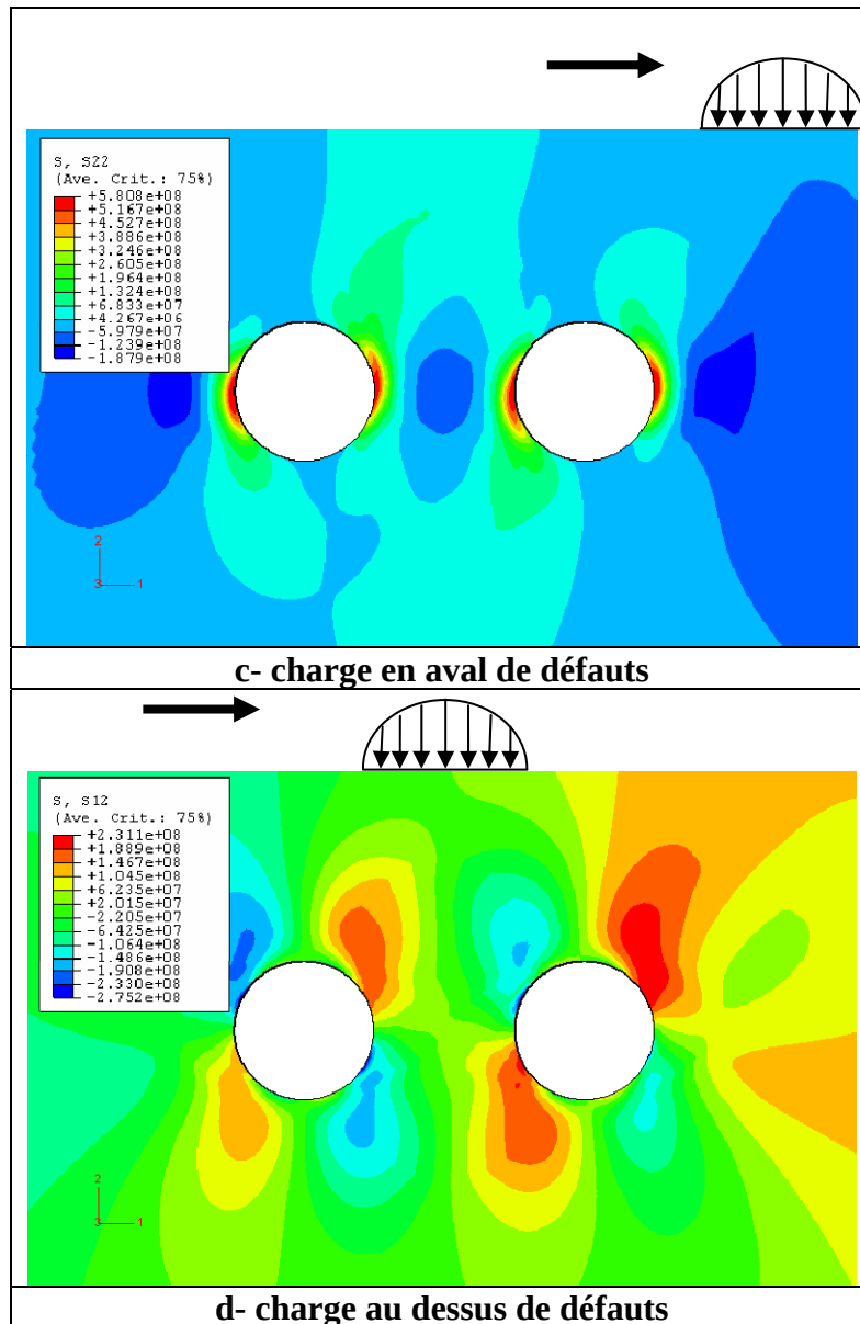
Figure 3-45. Répartition des contraintes normale et de cisaillement autour des deux défauts circulaires alignés horizontalement, F = 12 \text{ MN} / \text{m} et h = 15 \text{ mm} .
