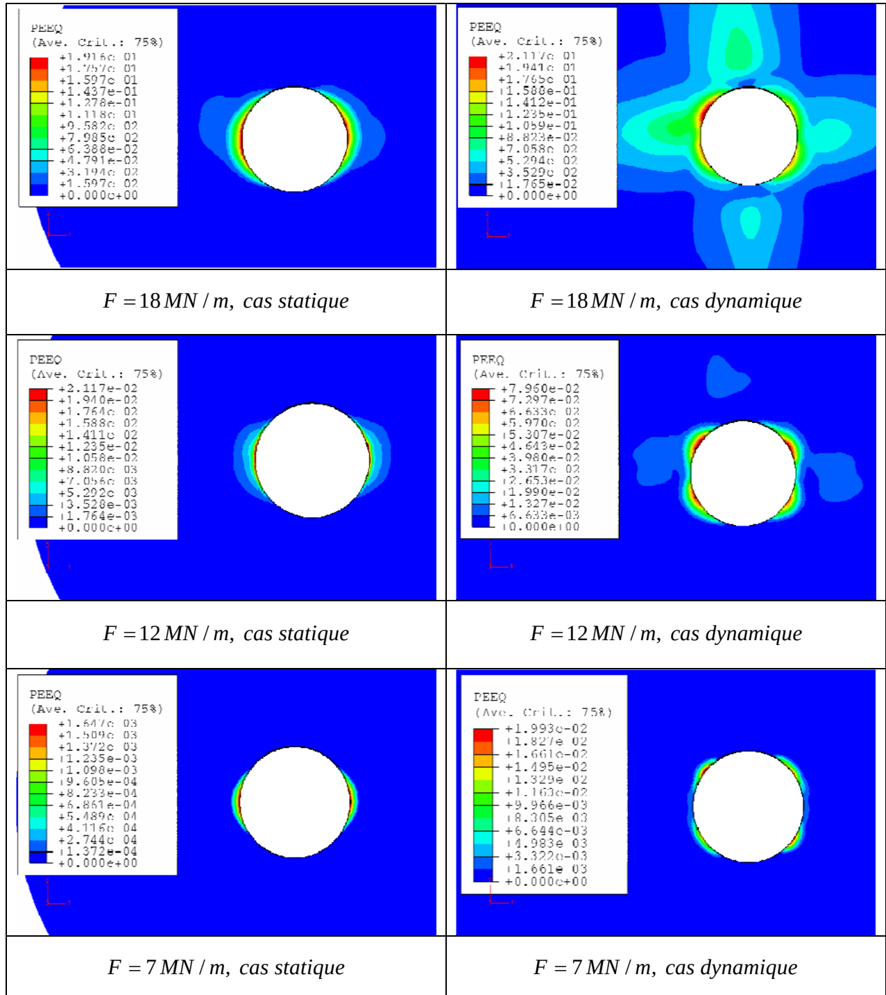
Figure 5-4. Comparaison de la répartition de la déformation plastique équivalente autour du défaut entre le cas statique et dynamique à V = 160 \text{ km/h} .
