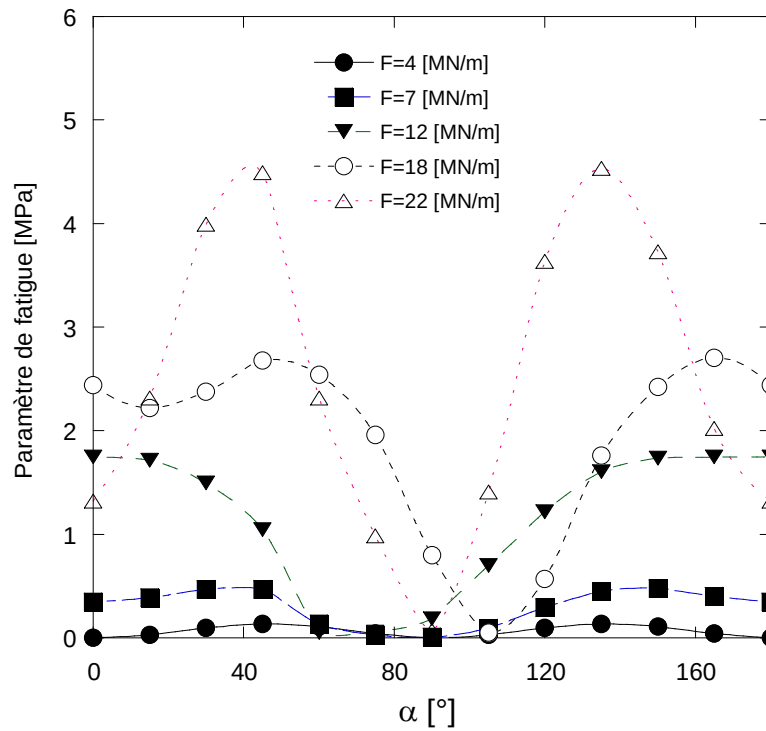
Figure 3-3. Paramètre de fatigue en fonction de l'angle \alpha pour différentes charges linéiques à h = 15mm .
