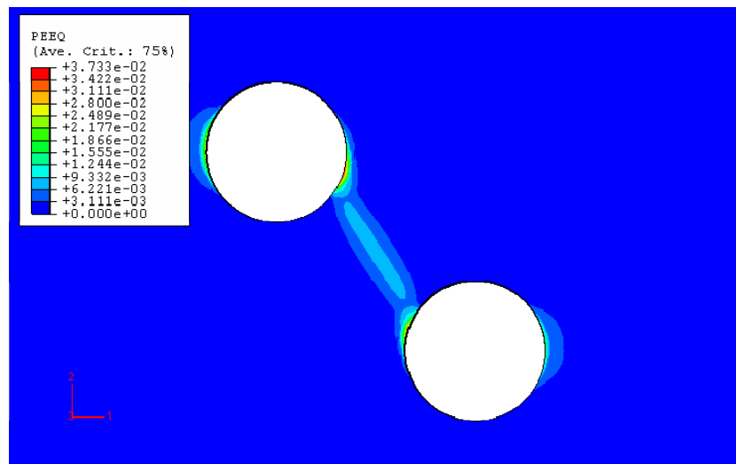
Figure 3-52. Répartition de la déformation plastique équivalente de von-Mises au 6 ème cycle de chargement, F = 12\text{MN} / \text{m} , h = 15\text{mm} .
