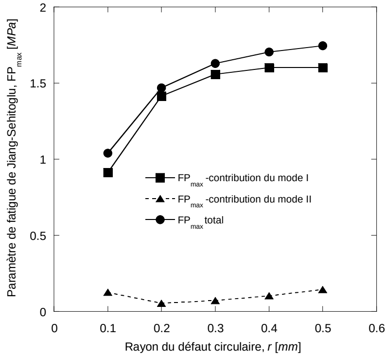
Figure 3-21. FP_{\max} en fonction du rayon du défaut à h = 15\text{ mm} et F = 12\text{ MN} / \text{m} .
