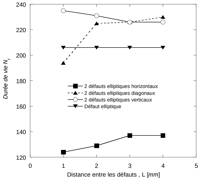
Figure 3-81. Durée de vie en fonction de la distance entre défauts pour les trois configurations de défauts elliptiques ( h = 15\text{ mm} , F = 12\text{ MN / m} ).
