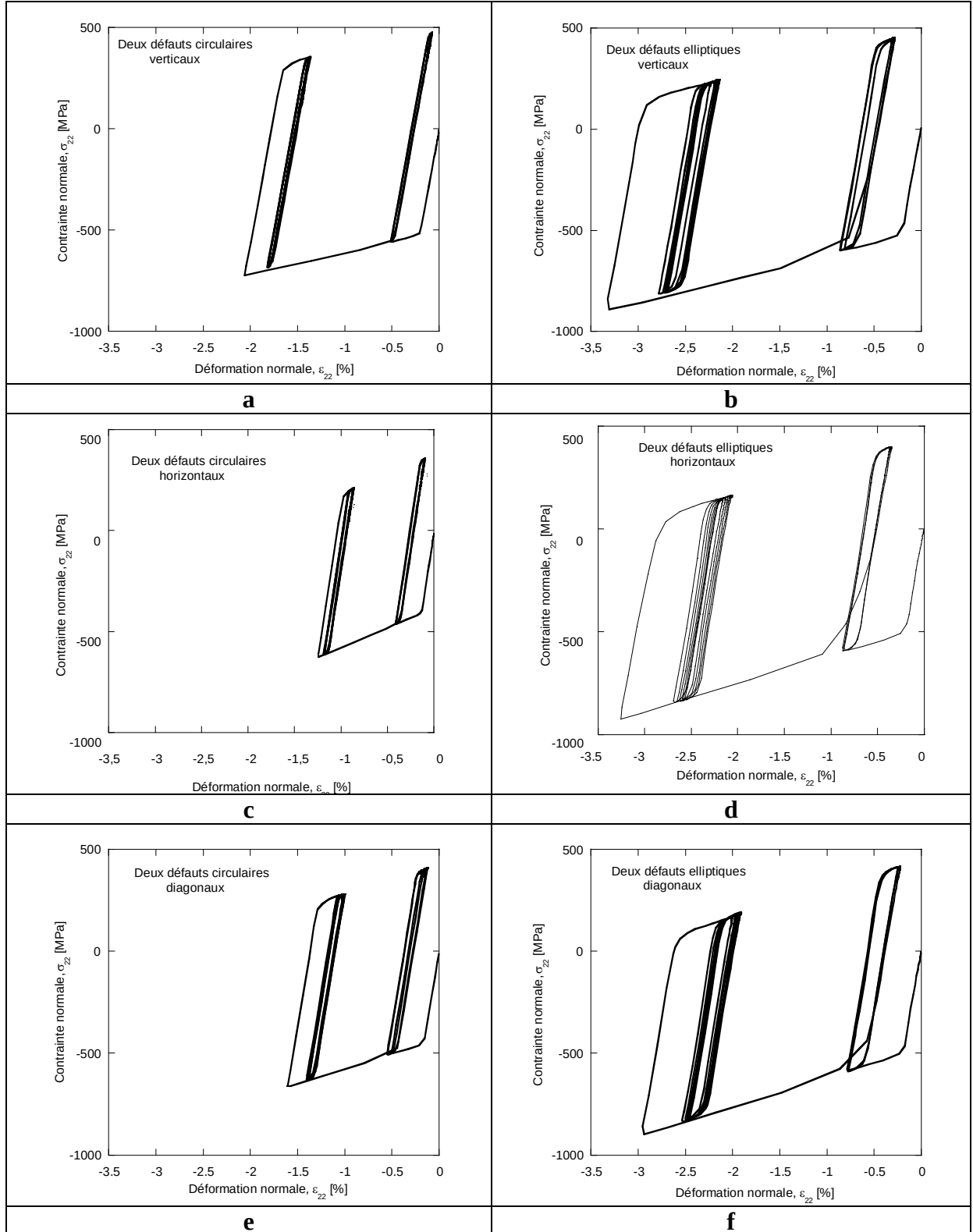
Figure 4-11. Boucles \sigma_{zz} - \epsilon_{zz} , chargement Bloc A (a) 2DCV (b) 2DEV (c) 2DCH (d) 2DEH, (e) 2DCD, (f) 2DED, R_s = 1,5 .
