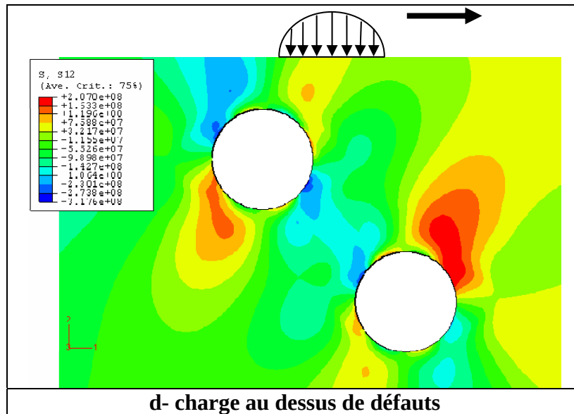
Figure 3-51. Distribution des contraintes normale, \sigma_{22} , et de cisaillement, \sigma_{12} autour des deux défauts circulaires alignés diagonalement.
