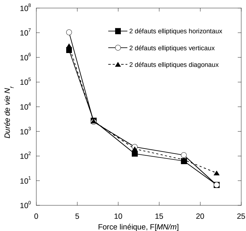
Figure 3-79. Durée de vie en fonction de la charge pour les trois configurations de défauts elliptiques ( h = 15\text{mm} ).
