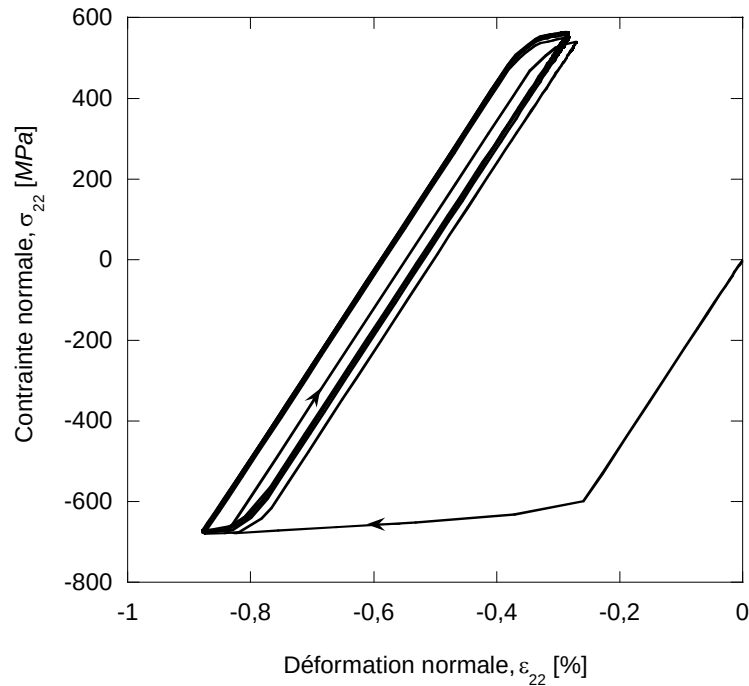
Figure 3-6. Accommodation plastique du matériau au chargement cyclique à h = 15 \text{ mm} et F = 12 \text{ MN} / \text{m} .
