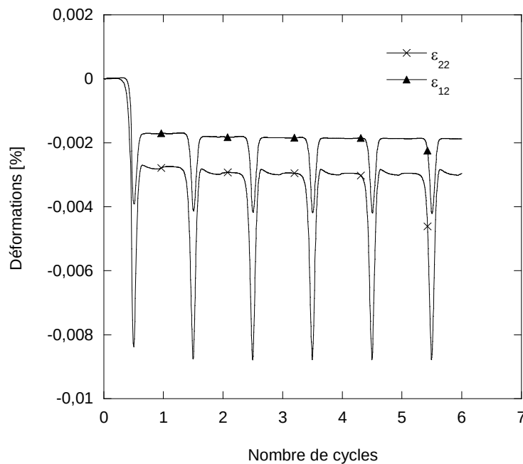
Figure 2-15. Déformations au cours des cycles de chargement pour un défaut de section circulaire situé à h = 15\text{mm} et chargé à F = 12\text{MN/m}
