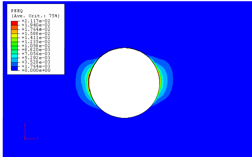
Figure 3-4. Répartition de la déformation plastique équivalente au voisinage immédiat du défaut circulaire, h = 15 \text{ mm} et F = 12 \text{ MN} / \text{m} .
