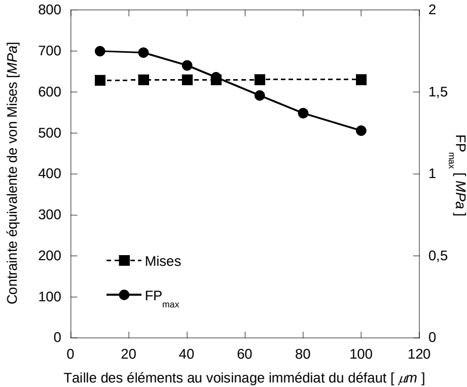
Figure 2-11. Evolution de FP_{\max} et de la contrainte équivalente de von Mises en fonction de la taille des éléments autour du défaut
