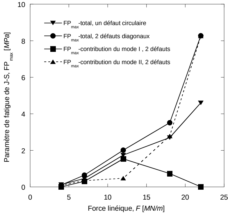
Figure 3-53. FP_{\max} en fonction de la charge linéique pour un défaut circulaire unique et pour deux défauts circulaires alignés diagonalement, h = 15 \text{ mm} .
