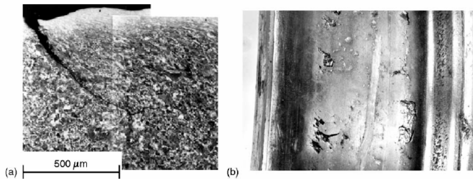
Figure 1-4. (a) Microstructure déformée et propagation de fissure dans un contact de roulement. (b) Endommagement superficiel dû à la fatigue amorcée en surface [3].
