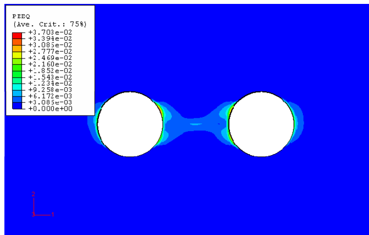
Figure 3-46. Répartition de la déformation plastique équivalente de von Mises au 6 ème cycle de chargement, F = 12 \text{ MN/m} , h = 15 \text{ mm} .
