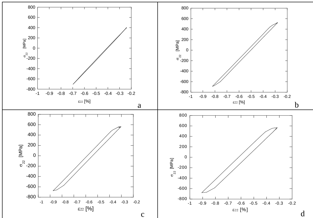
Figure 3-20. Influence de la taille du défaut sur la réponse du matériau - cycle stabilisé à h = 15\text{ mm} et F = 12\text{ MN} / \text{m} a) r = 0,1\text{ mm} , b) r = 0,2\text{ mm} , c) r = 0,4\text{ mm} , d) r = 0,5\text{ mm} .
