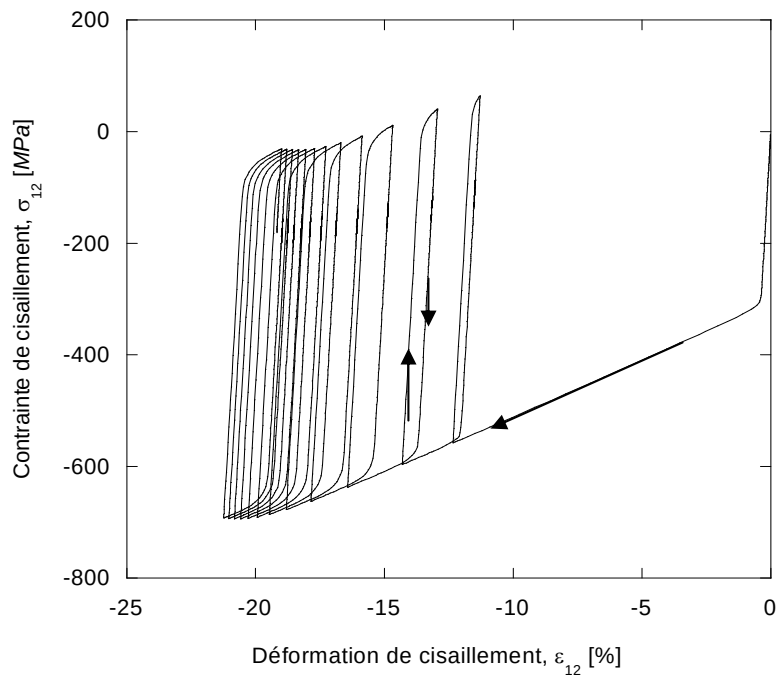
Figure 3-7. Effet de rochet lors du chargement cyclique à h = 15 \text{ mm} et F = 22 \text{ MN} / \text{m} .
