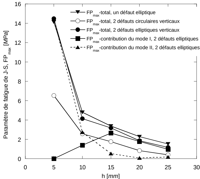
Figure 3-63. FP_{\max} en fonction de la profondeur à F = 12 \text{ MN} / m .
