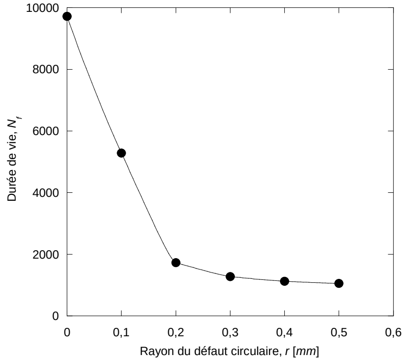
Figure 3-19. Durées de vie à l'amorçage en fonction du rayon du défaut à h = 15\text{ mm} et F = 12\text{ MN} / \text{m} .
