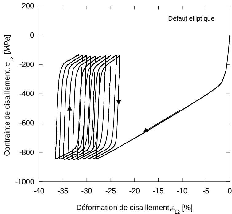
Figure 3-31. Fort effet de rochet à F = 22 \text{ MN} / \text{m} ( h = 15 \text{ mm} ).
