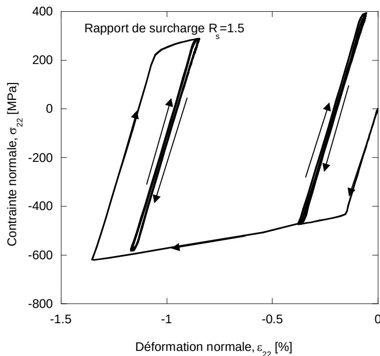
Figure 4-2. Boucles \sigma_{22} - \varepsilon_{22} avant et après surcharge à R_s = 1,5 .
