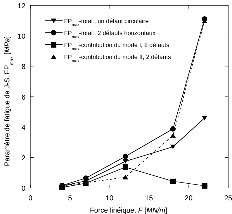
Figure 3-47. FP_{\max} en fonction de la charge linéique pour un défaut circulaire et deux défauts circulaires alignés horizontalement, h = 15 \text{ mm} .
