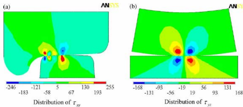
Figure 1-14. Distribution des contraintes de cisaillement dans le plan d'un contact roue/rail [131].
