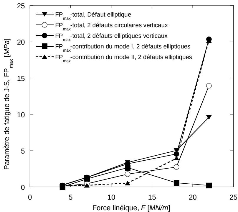
Figure 3-61. FP_{\max} en fonction de la force linéique à h = 15 \text{ mm} .
