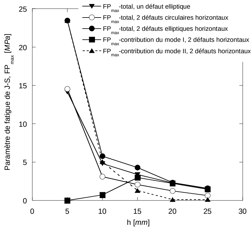
Figure 3-70. FP_{max} en fonction de la profondeur à F = 12 \text{ MN} / \text{m} .
