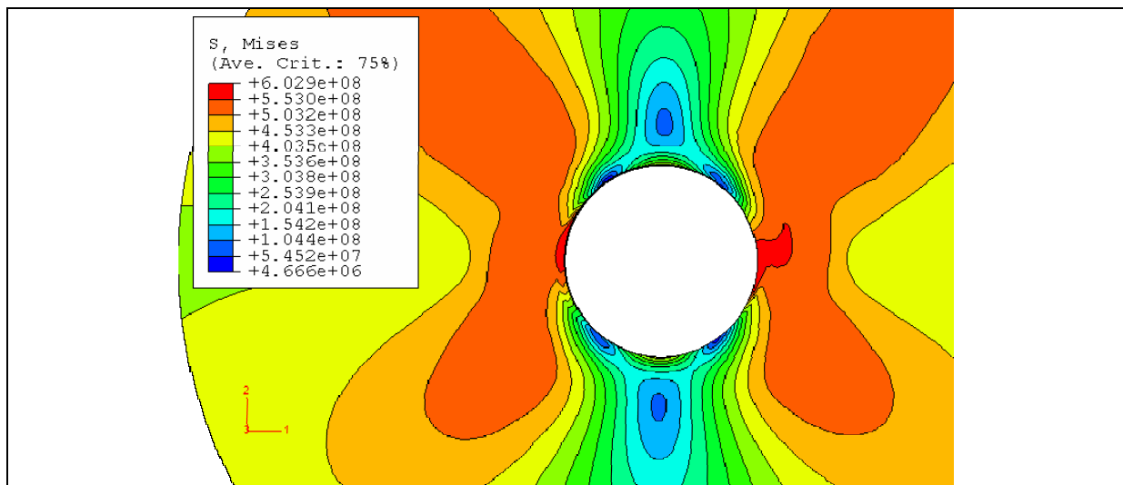
Figure 2-12. Distribution au sixième cycle du chargement, des contraintes de von Mises autour d'un défaut circulaire situé à h = 15\text{mm} et pour F = 12\text{ MN/m}
