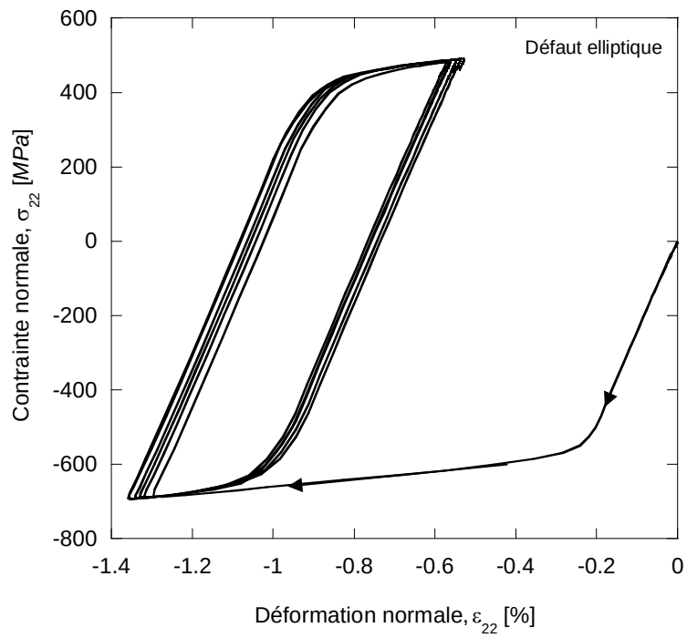
Figure 3-30. Faible effet de rochet à F = 12 \text{ MN} / \text{m} ( h = 15 \text{ mm} ) .
