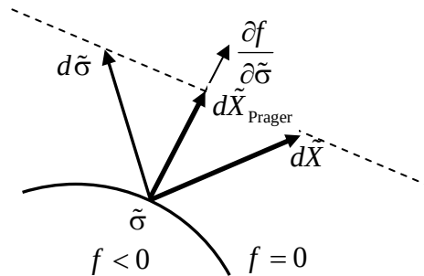
Figure 2-2. Représentation géométrique de l'écrouissage cinématique
