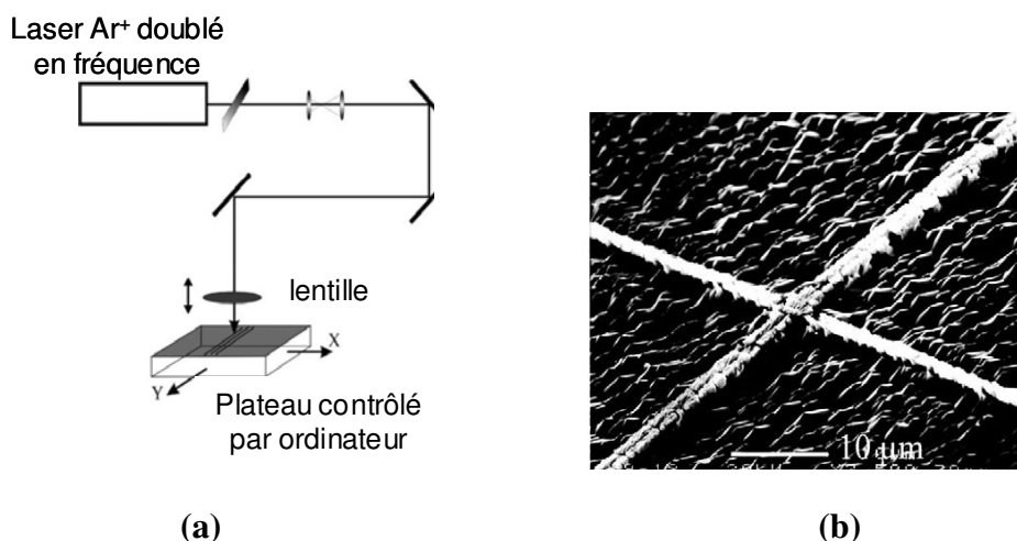
Figure 2.14 : (a) Montage expérimental utilisé par Mailis. (b) Image MEB d'un réseau de lignes gravées sur la surface z- d'un cristal de \text{LiNbO}_3
