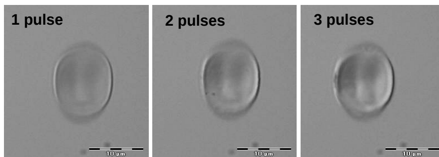
Figure 3.18 : trous ablatés sur le cristal implanté avec 1.9 \text{ J/cm}^2 et 1, 2 et 3 pulses.
