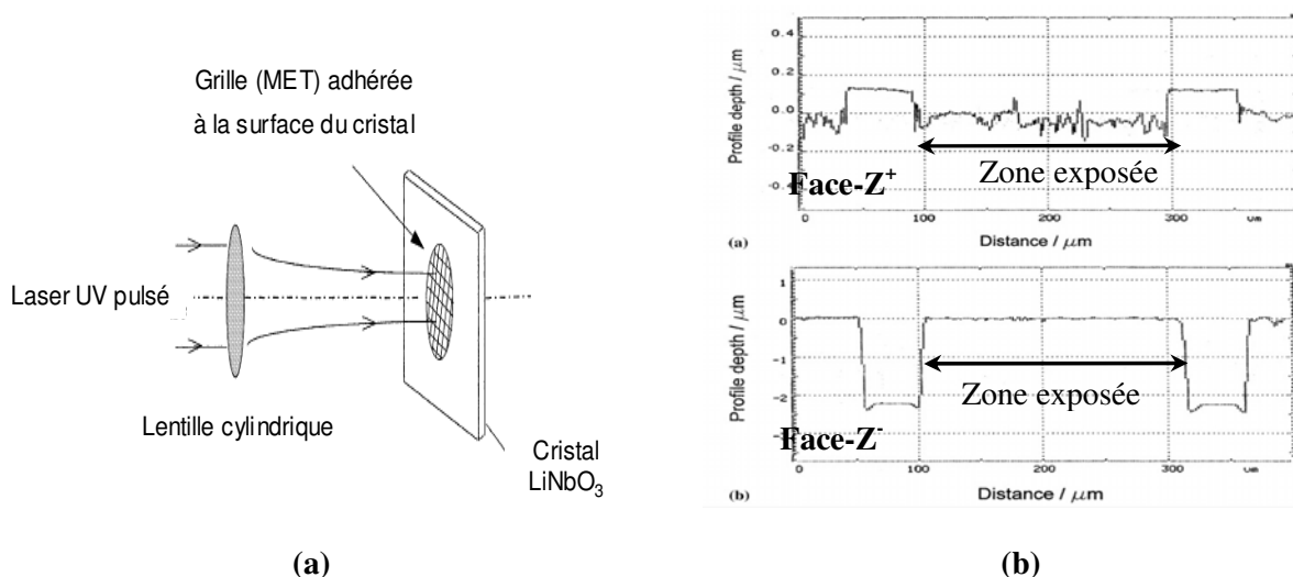
Figure 2.15 : (a) Montage expérimental utilisé par Brown. (b) Les reliefs obtenus sur la surface z^+ et z^- du cristal \text{LiNbO}_3 avec les mêmes conditions d'exposition : 1000 tirs à 248 nm et 5h de gravure dans un bain de \text{HF}:\text{HNO}_3 .
