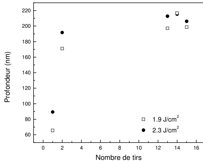
Figure 4.11 : Profondeur ablatée en fonction du nombre de tirs pour deux fluences : 1.9 et 2.3 \text{J}/\text{cm}^2 .
