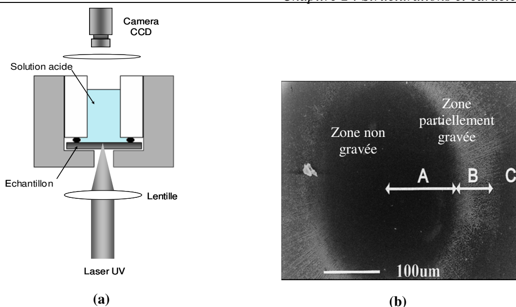
Figure 2.13 : (a) Cellule utilisée pour la gravure LIFE (illumination + acide). (b) Photographie MEB des trois régions obtenues lors d'une gravure LIFE d'un cristal de \text{LiNbO}_3 [141].
