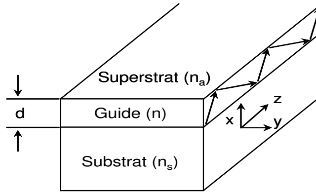
Figure 1.1 : Schéma d'un guide d'onde plan
