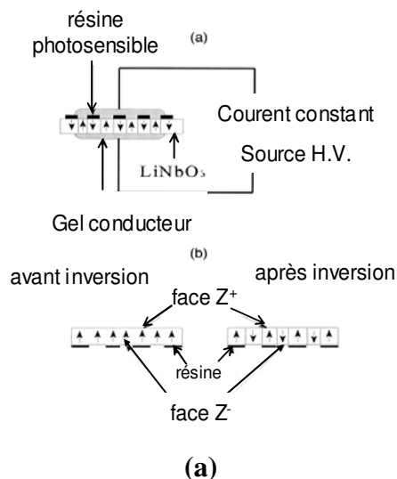
Figure 2.7: (a) Vue schématisée du processus d'inversion. (b) Tableau de carrés de 150 \mu\text{m} de hauteur.
