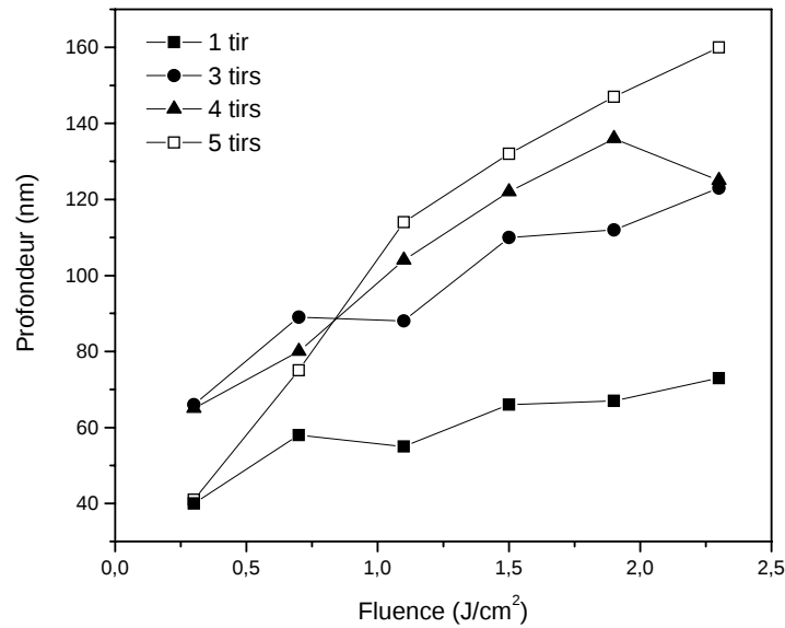
Figure 3.10 : Profondeur d'ablation ( \mu\text{m} ) des couches minces de \text{LiNbO}_3 en fonction de la fluence du laser ( \text{J/cm}^2 ) pour 1, 3, 4 et 5 tirs. La fluence pour chaque nombre de tir varie de 0.3 à 2.3 \text{J/cm}^2 .
