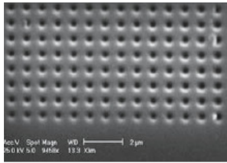
Figure 2.6 : Photographie MEB d'un réseau carré de trous gravé sur un crystal z-cut de \text{LiNbO}_3 par la technique EBL : diamètre des trous D=170 nm, période a=650 nm.
