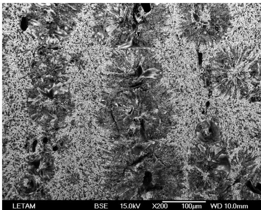
图 3-4 5 次轰击 D2 模具钢表面典型的背散射电子（BSE）形貌像 Fig. 3-4 Typical BSE surface micrograph of the D2 sample treated with 5 pulses.
