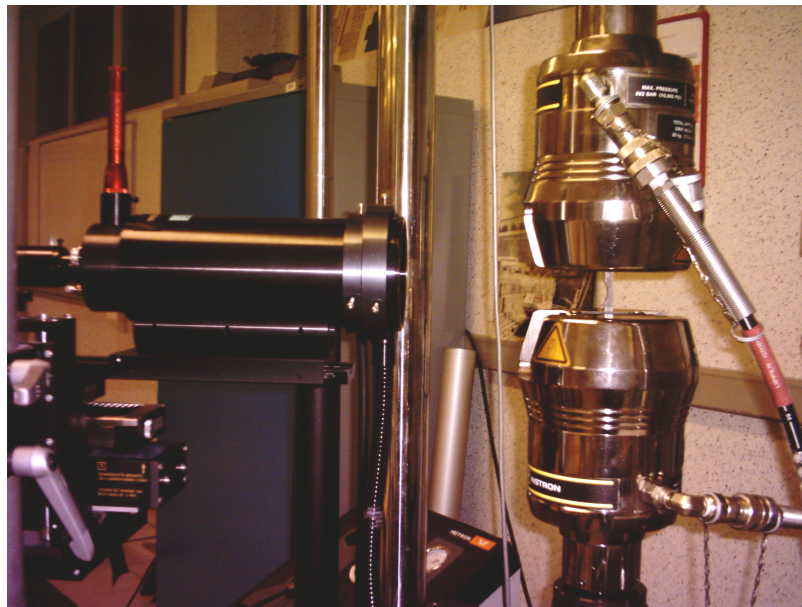
Figure V-4 : Microscope à longue distance focale
