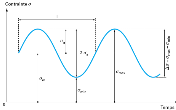
Figure V-8 : Sollicitation sinusoïdale appliquée (amplitude constante)
