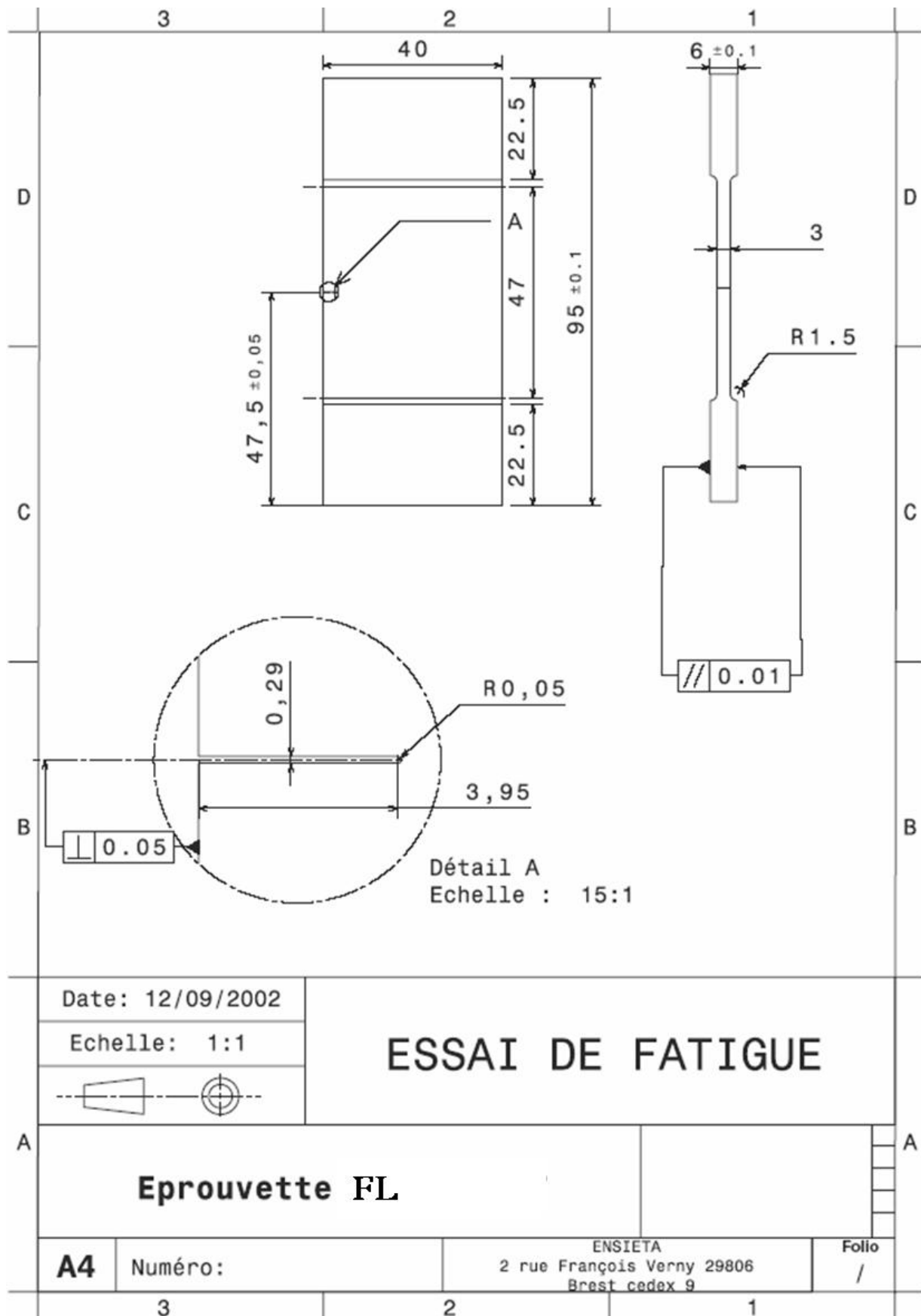
Figure V-3: Eprouvette destinée à l'étude des fissures longues
