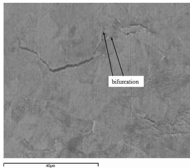
Figure XI-15 : Arrêt de la fissuration dû au phénomène de bifurcation
