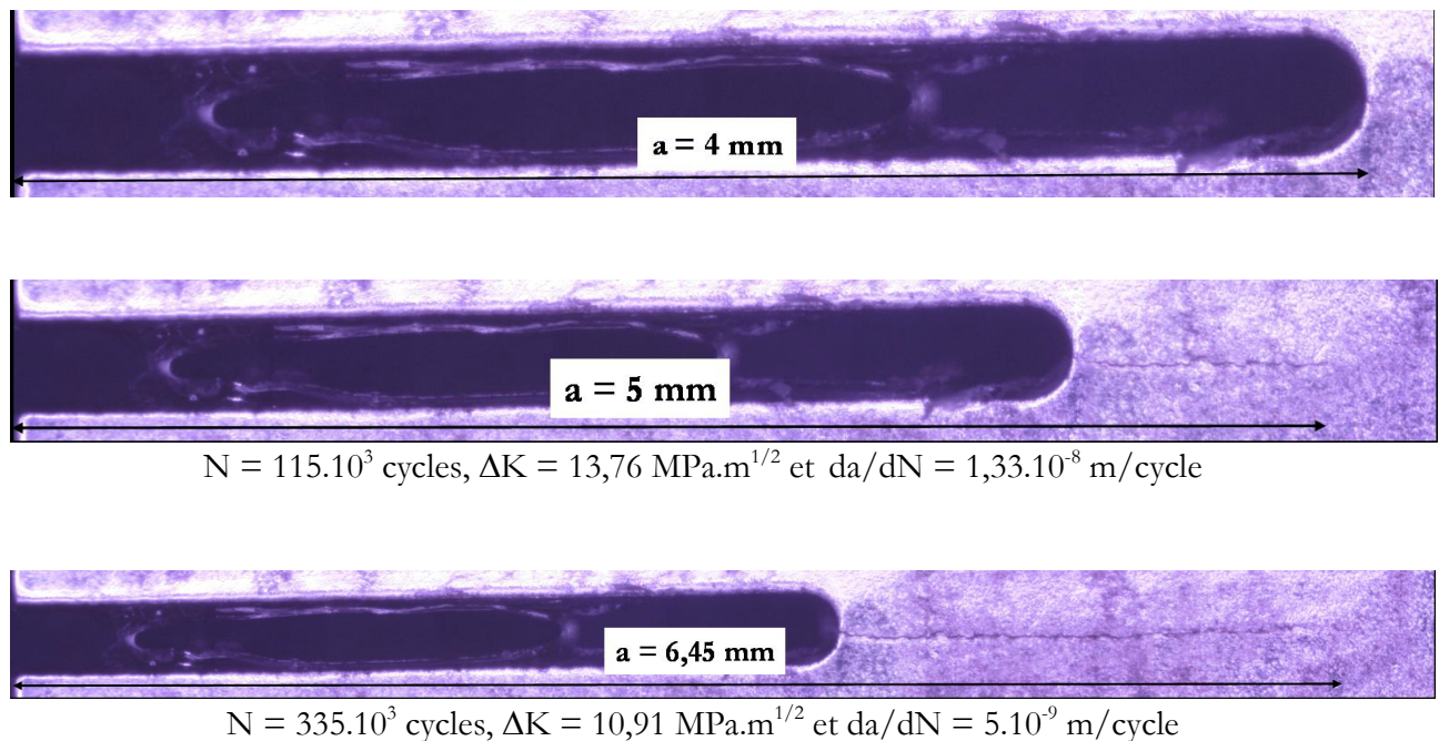
Figure V-5 : Exemple de suivi de fissure longue par microscope à longue distance en utilisant la méthode à \Delta K décroissant ( R = 0,5 )
