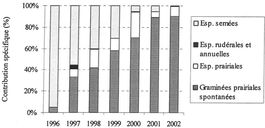
Figure 1 : Evolution des contributions spécifiques sur la parcelle SC de 1996 à 2002
