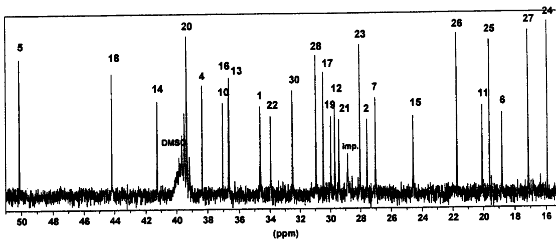
Figure 52: Spectre de RMN ^{13}\text{C} d'Anis 27 = acide bryonolique enregistré dans DMSO- \text{d}_6 à 125.76 MHz
