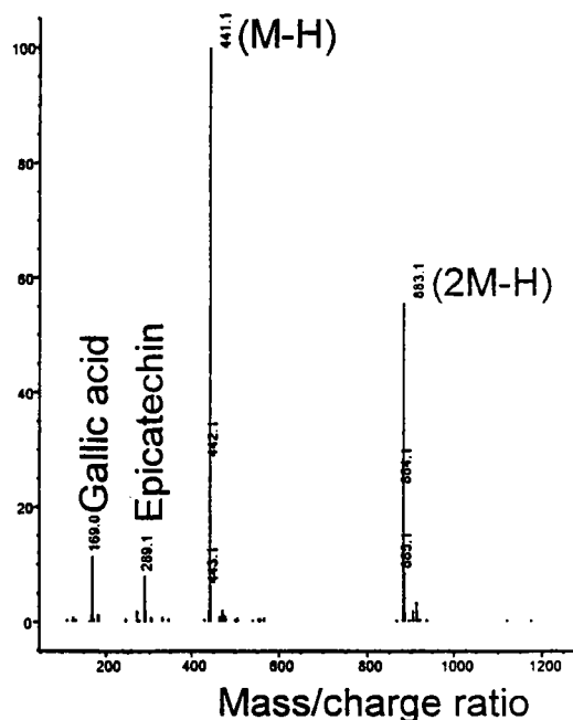
Figure 20: Spectre de Masse en ESI/MS (mode négatif) du produit Anis 6
