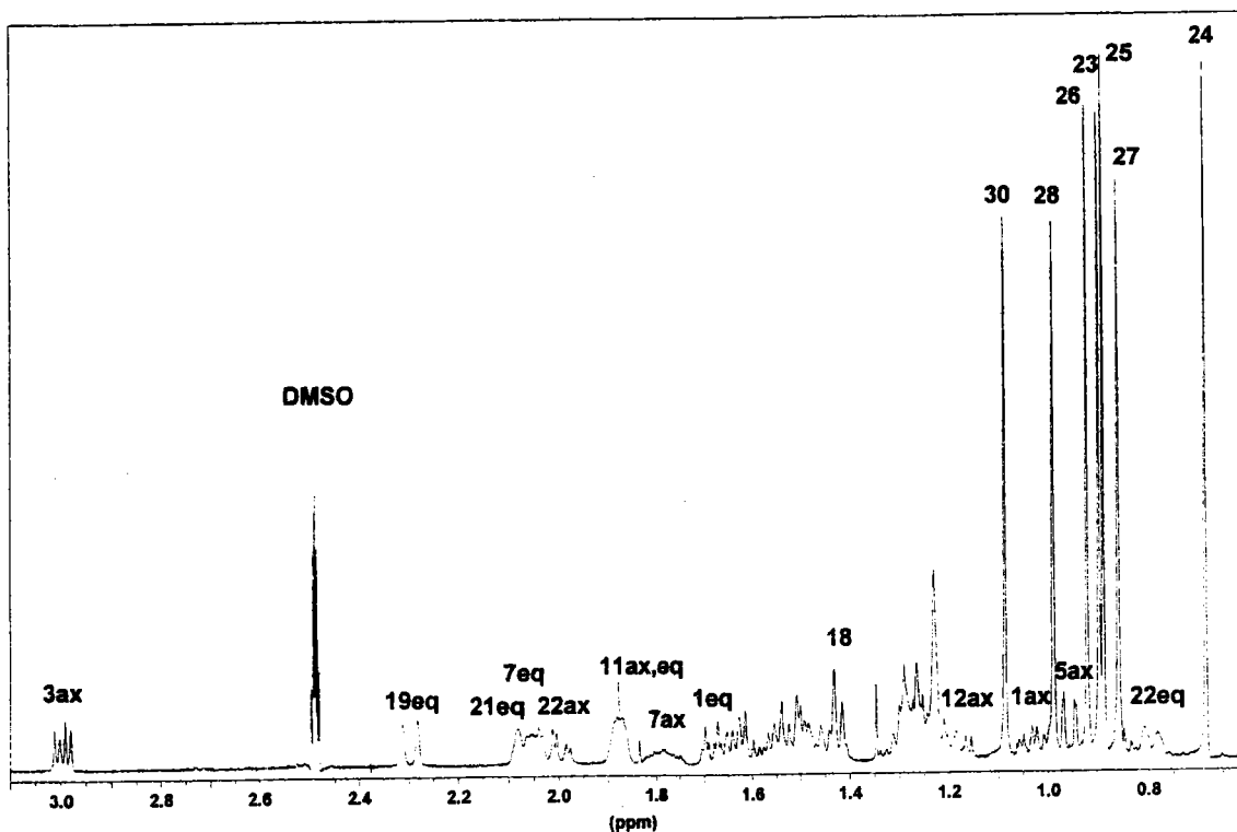
Figure 51: Spectre de RMN ^1\text{H} d'Anis 27 = acide bryonolique enregistré dans DMSO- \text{d}_6 à 500 MHz
