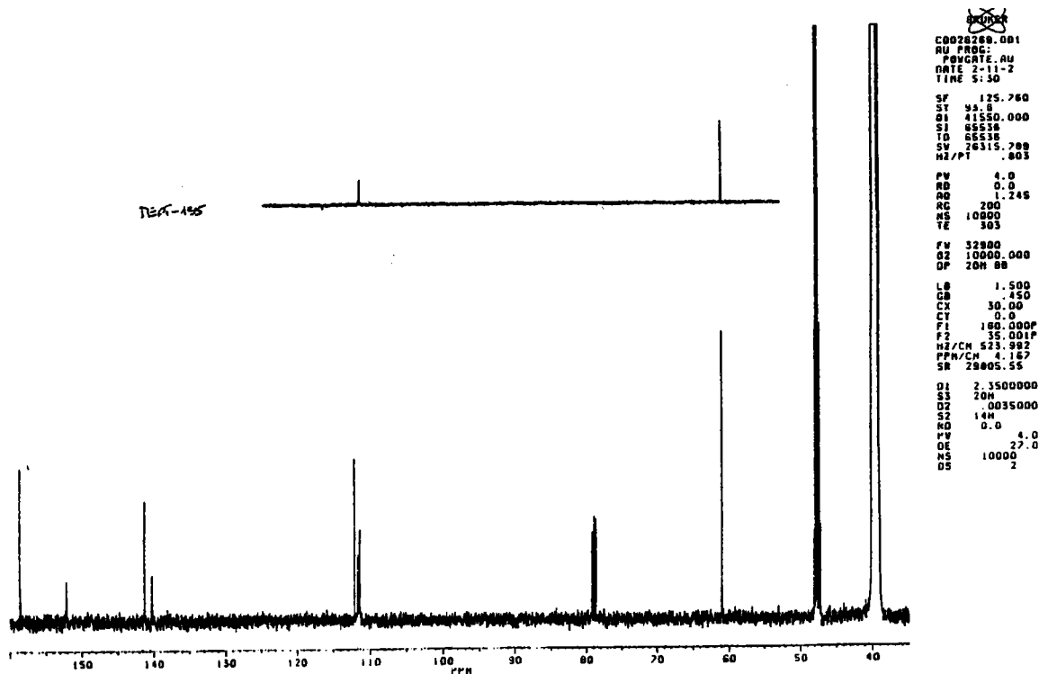
Figure 50: Spectre de RMN ^{13}\text{C} dans (DMSO- \text{d}_6 , 5% de \text{CD}_3\text{OD} ) à 125,6 MHz d'Anis 15
