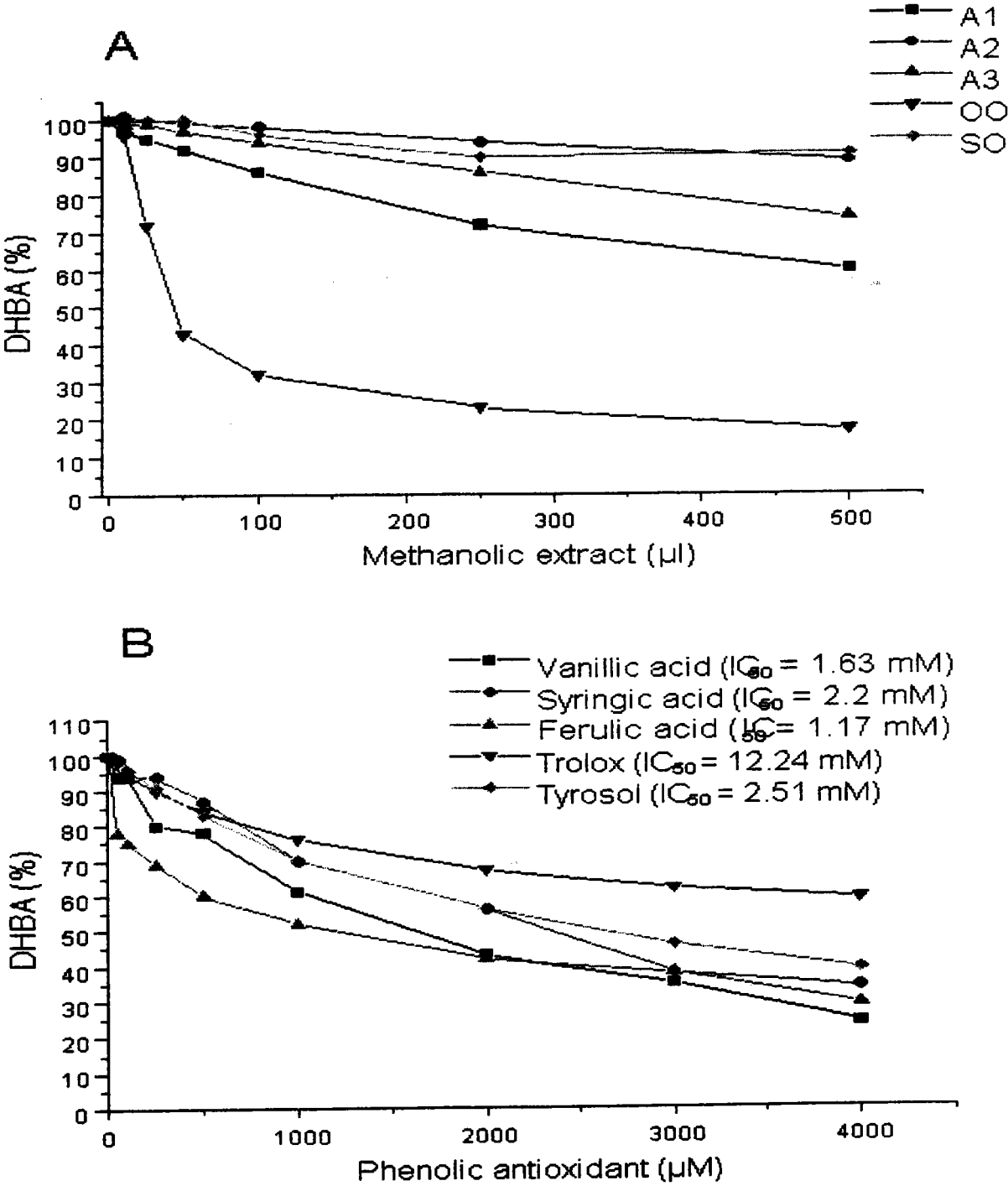
Figures 98: Détection de l'atténuation des espèces réactives d'oxygène par A: les différents extraits méthanoliques des huiles étudiées: A 1 . Argan alimentaire, A 2 . Argan esthétique, A 3 . Argan commerciale, OO. Huile d'olive, SO. Huile de tournesol, B: les différents acides phénols majoritaires détectés dans l'huile d'argan. Le TROLOX a été utilisé comme antioxydant témoin dans cette étude
