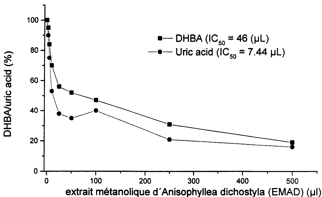
Figure 97: Inhibition de la xanthine oxydase par l'extrait méthanolique EMAD (en \mu l) obtenu de l'écorce des racines d' A. dichostyla
