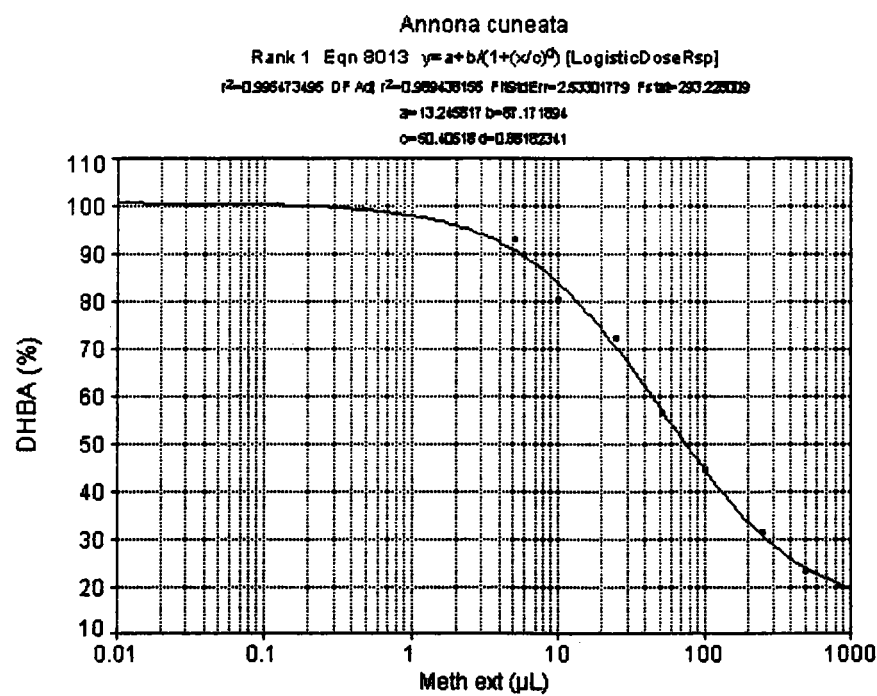
Figure 96: Signal montrant l'inhibition des espèces réactives d'oxygène dans le système HX/XO par EMAC (IC 50 =72 µl)
