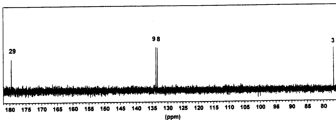
Figure 51: Spectre de RMN ^1\text{H} d'Anis 27 = acide bryonolique enregistré dans DMSO- \text{d}_6 à 500 MHz
