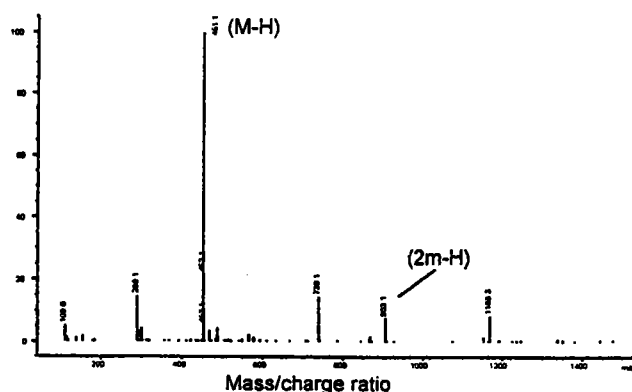
Figure 10: Spectre de Masse en ESI /MS (mode négatif) du composé Anis 1
