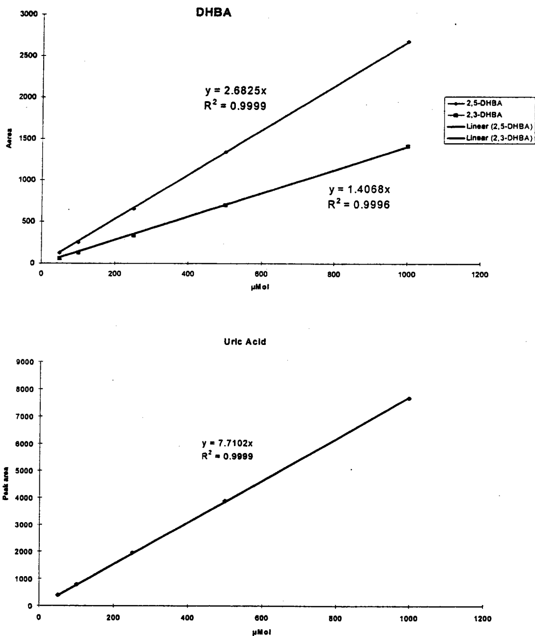
Figure 94: Courbes de calibration (analyse par CLHP en duplicat) des acides benzoïque (2,5-DHBA et 2,3-DHBA) et de l'acide urique
