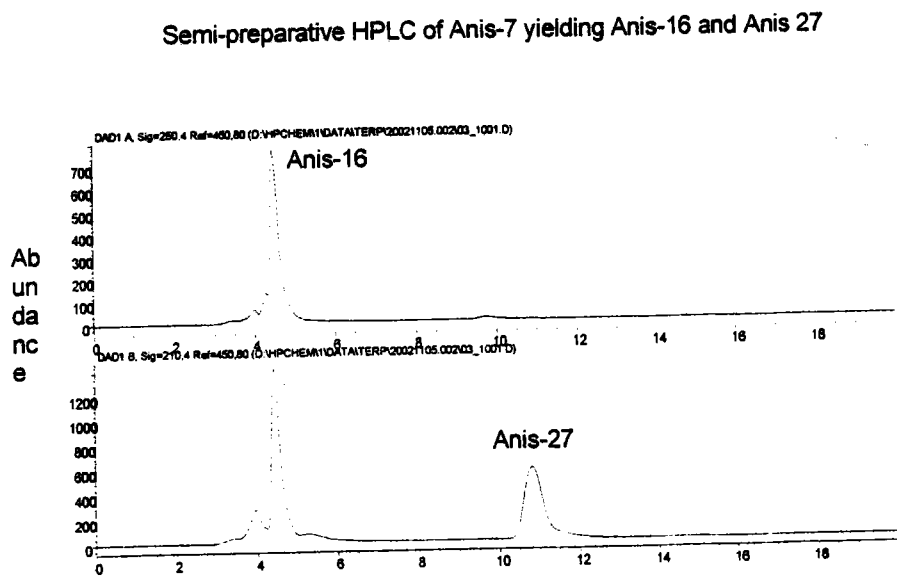
Figure 41: Profil CLHP du produit Anis 16 mélangé avec le produit Anis 27 , colonne Latek C-18, gradient d'élution MeOH, 2% acide acétique dans l'eau bidistillée, Débit: 3 ml/l, détection à 210 nm.
