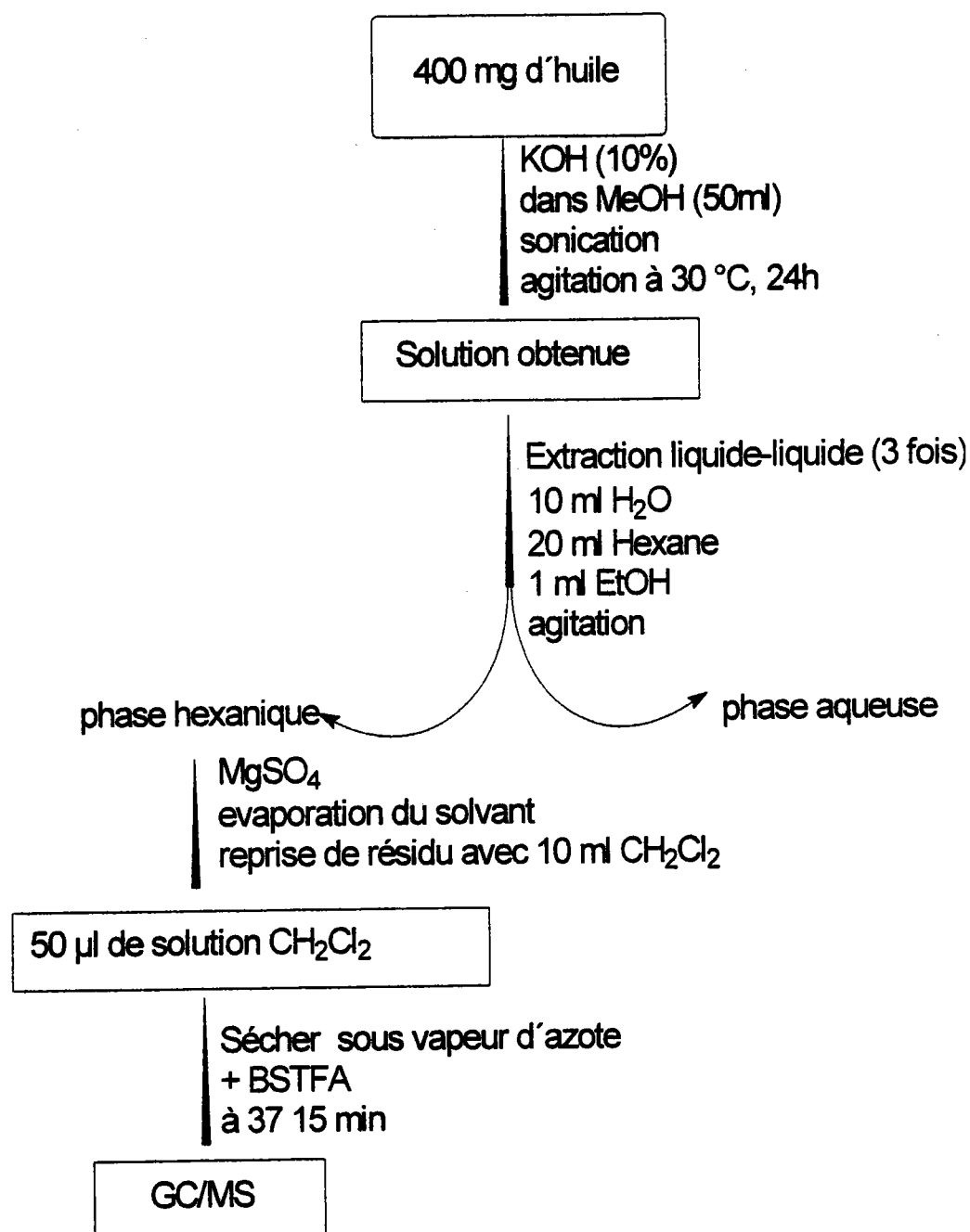
Schéma 3: Obtention de l'insaponifiable enrichi de squalène et de stéroïdes de l'huile d'argan esthétique
