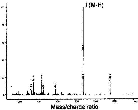
Figure 15: Spectre de masse en ESI/MS (en mode négatif) d'Anis 4
