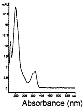
Figure 22: Spectre en UV du composé Anis 8
