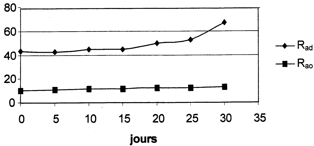
Figure 83: Changement des rapports entre les intégrales des protons aliphatiques et protons diallylméthylènes et les intégrales des protons aliphatiques et oléfiniques ( R_{ad} et R_{ao} respectivement), évoluant à 63,5 °C
