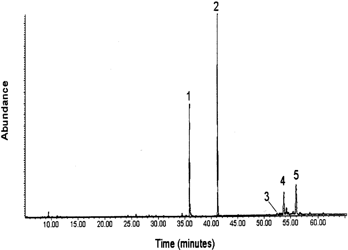
Figure 70: Profil des stérols et de squalène de la variété esthétique de l'huile d'argan déterminé à partir de l'insaponifiable par GC/MS
