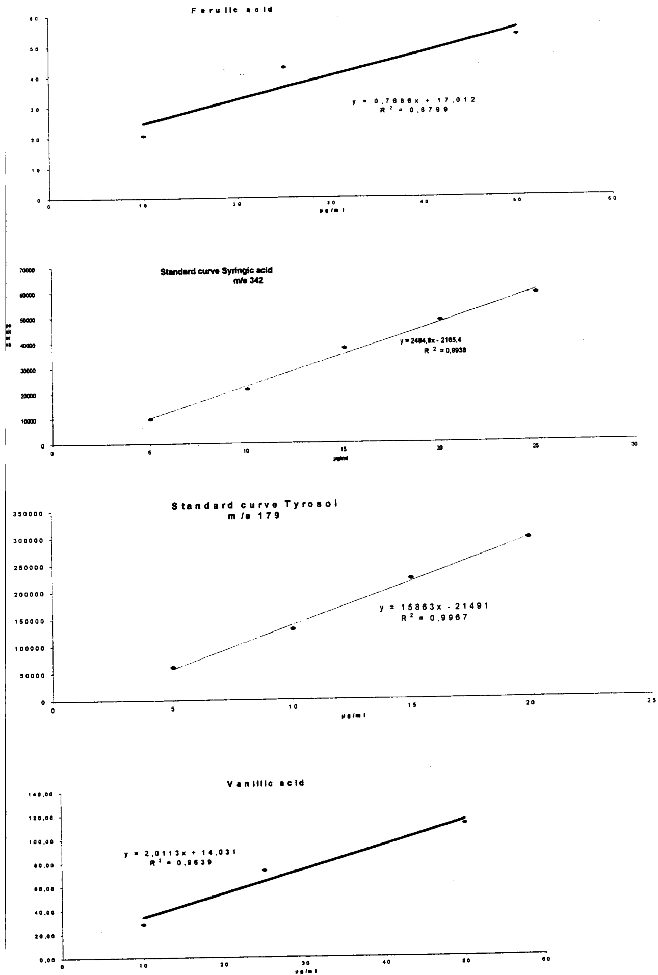
Figure 87: Courbes d'étalonnage externes obtenues par GC/MS (en duplicat) des phénols simples détectés dans l'huile d'argan
