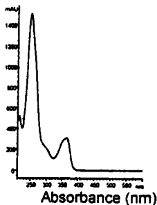
Figure 30: Spectre en UV du produit Anis 12
