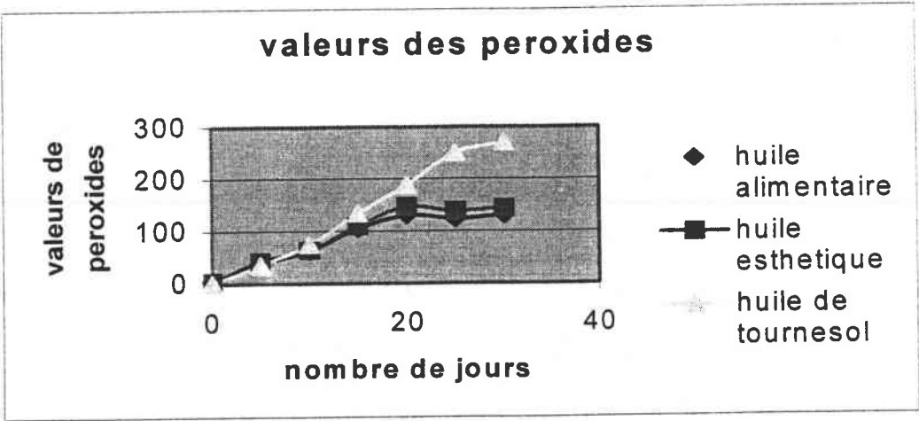
Figure 81: Cinétique de valeurs des peroxydes formés dans l'huile d'argan à 63,5 °C
