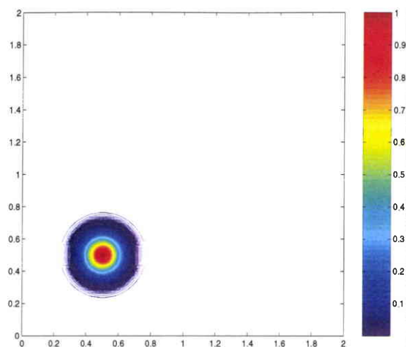
FIG. 4.36 – Test 1 : Isolignes de la solution initiale.
