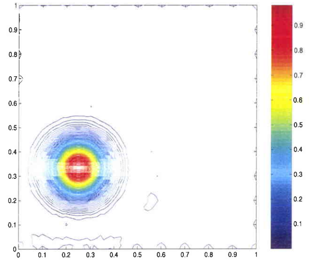
FIG. 2.24 – Test 4 : Isolignes de la solution u_h \in P_{nc,0}^2 calculée par le schéma P_{nc,0}^2 \times (RT^1 + \Phi) .
