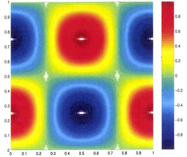
FIG. 2.14 – Test 1 : Isolignes de la solution u_h \in P^2_{nc,0} calculée par le schéma P^2_{nc,0} \times (RT^1 + \Phi) .
