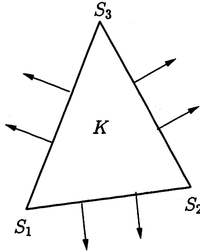
FIG. 2.9 – Représentation des degrés de liberté de l'espace BDM_1 .
