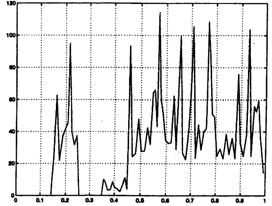
FIG. 4.33 – Représentation de \mu pour ce test
