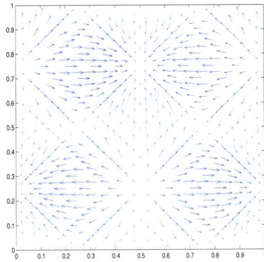
FIG. 2.15 – Test 1 : Flux p_h \in (RT^1 + \Phi) calculé par le schéma P^2_{nc,0} \times (RT^1 + \Phi) .
