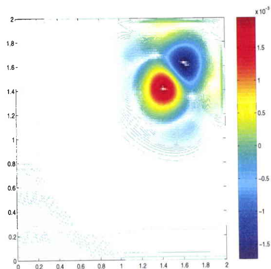
FIG. 4.44 – Test 1 : Isolignes de la différence entre la solution exacte et la solution ADI, T = 1.25 , Maillage 3.
