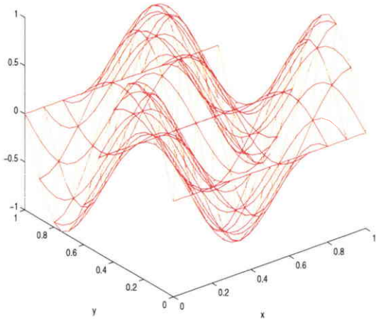
FIG. 2.13 – Test 1 : Solution u_h \in P^2_{nc,0} calculée par le schéma boîte P^2_{nc,0} \times (RT^1 + \Phi) .
