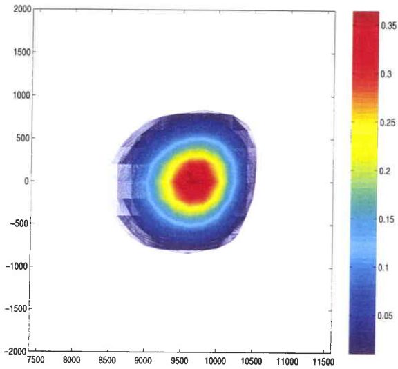
FIG. 4.49 – Test 2 : Isolignes de la solution calculée ADI, T = 4800 , Maillage 1.
