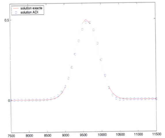
FIG. 4.48 – Test 2 : Coupe selon y = 0 des solutions exacte et calculée ADI, T = 4800 , Maillage 2
