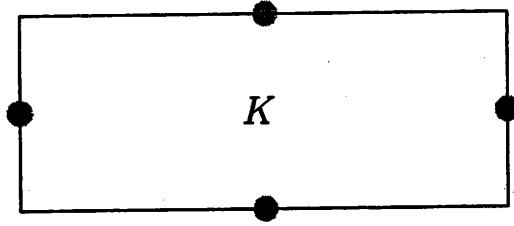
FIG. 3.17 – Les degrés de liberté de Q^1_{\text{rot}} dans le rectangle K
