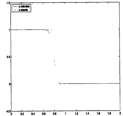
FIG. 4.5 – Test 2 : Décentrement D_u = 0.18 donné par (4.81). Le schéma est d'ordre 1. On observe la diffusion artificielle.
