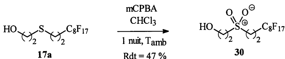
Figure II-54 : Oxydation du 2-perfluorooctyl-éthyl 3-hydroxy-propyl thioéther : 30 .
