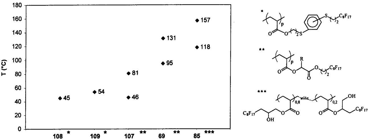
Figure IV-30 : Températures de transition de phases ( T g ) des polyacrylates comportant un groupement organique non soufré (fonction ester, groupements aromatique et hydroxyle).
