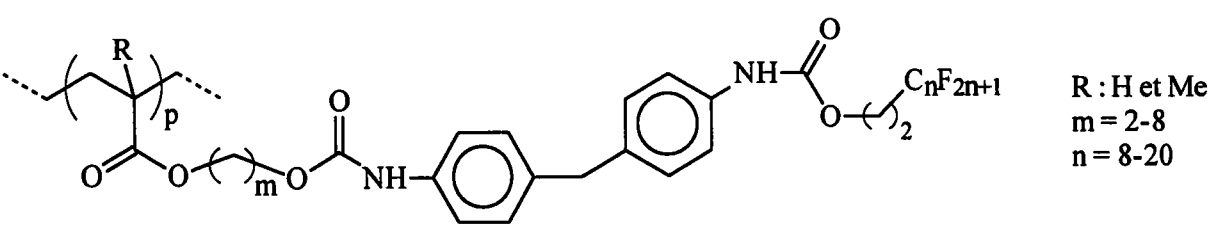
Figure I-43 : Poly(méth)acrylate perfluoré porteur d’un groupement di-uréthane aromatique [122,123].
