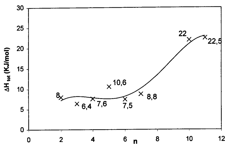
Figure IV-13 : Evolution des variations d'enthalpie associées aux différentes transitions de phases des polyacrylates de ω-perfluorooctyl-alkyle en fonction de la taille de l'espaceur (n).
