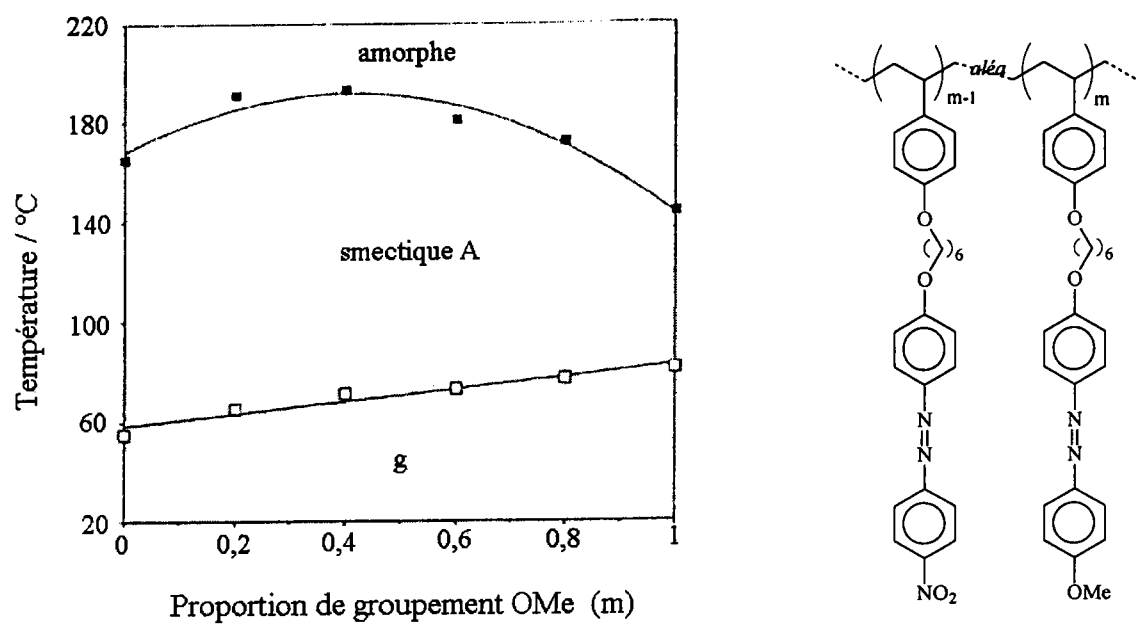
Figure I-42 : Dépendance des températures de transition de phases en fonction de la proportion en comonomère porteur du groupement méthoxyle [121].
