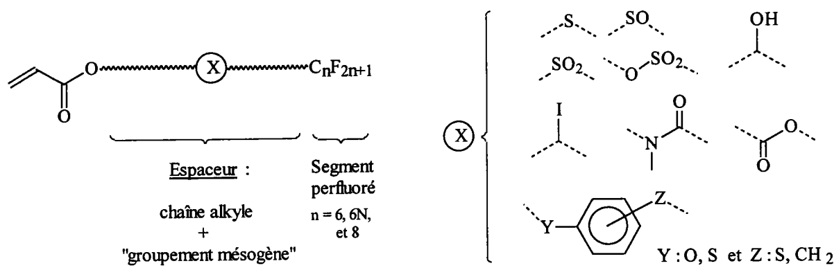
Figure II-1 : Structure générale des monomères à préparer.
