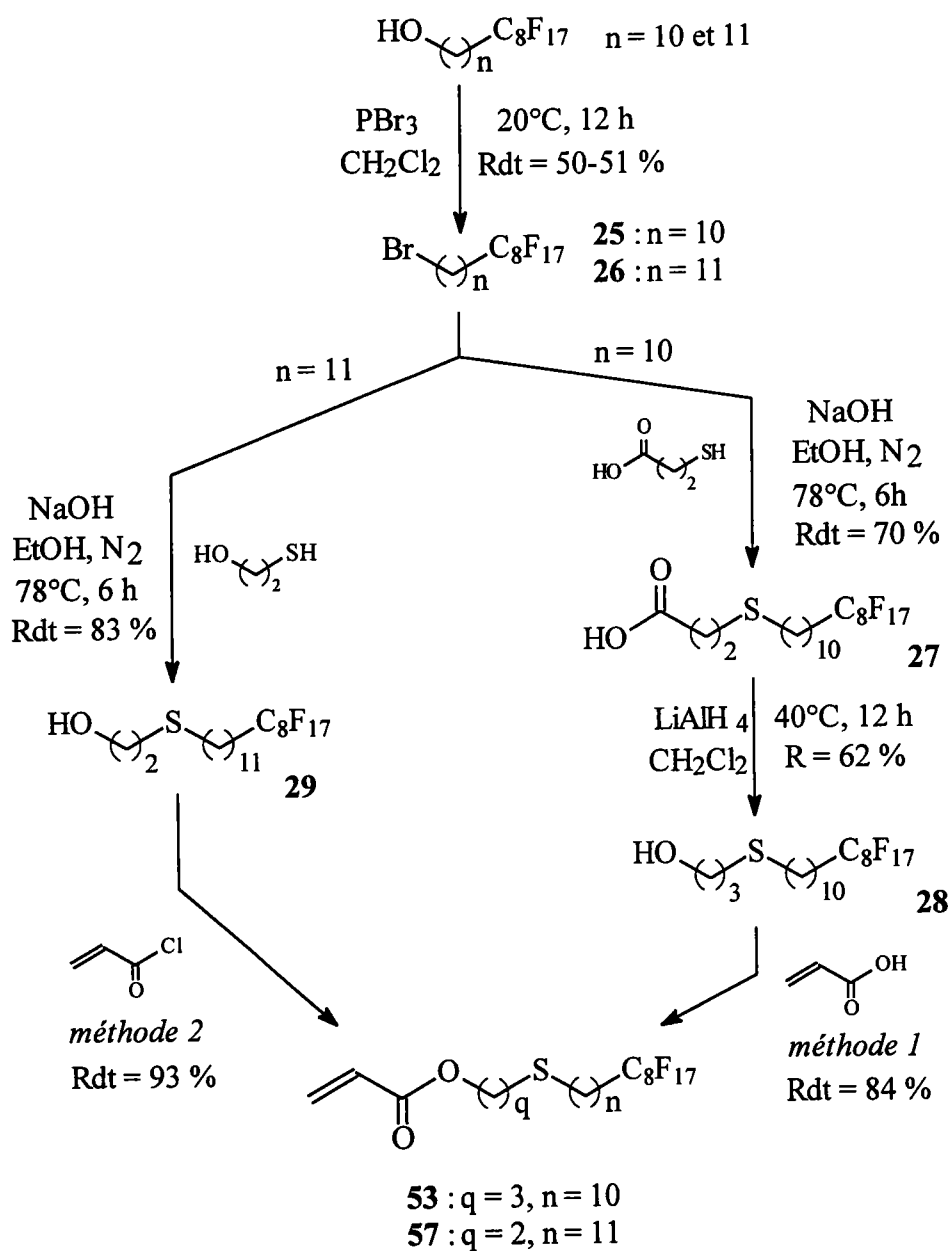
Figure II-52 : Schéma général de synthèse des acrylates de 14-perfluorooctyl-x-thia-tétradécyle ( x = 3 et 4 ) : 53 et 57.
