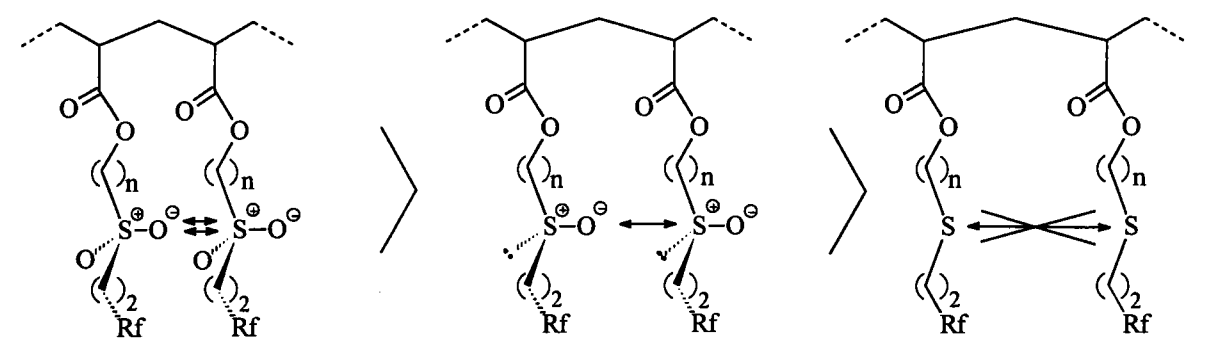
Figure IV-26 : Effet structurant des groupements organiques polaires : fonctions sulfoxyde et sulfone.
