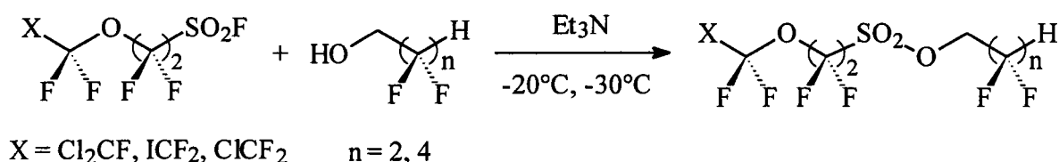
Figure II-62 : Synthèse de sulfonates perfluorés selon Q.Y. Chen [206].
