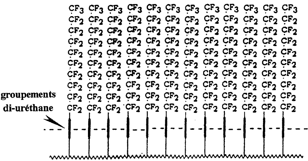
Figure I-44 : Arrangement idéal des chaînes latérales d'un poly(méth)acrylate perfluoré porteur d'un groupement di-urthane aromatique [122].
