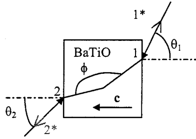
FIG. 3.1 – Double conjugaison de phase : cas général
