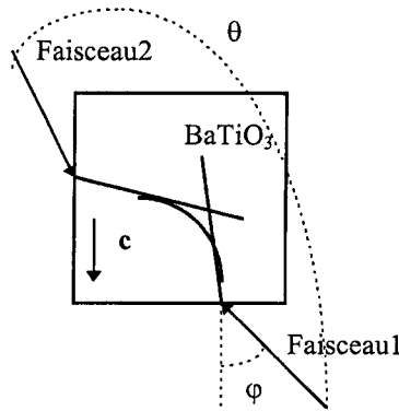
FIG. 3.11 – Modified Bridge dans \text{BaTiO}_3 présenté par Wang et al. [45]
