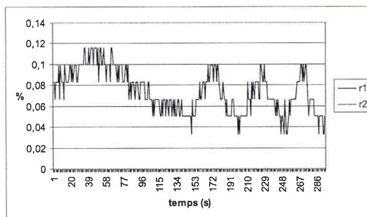
FIG. 5.67 – Evolution des rendements du DPCM dans le cristal dopé en faisceaux fins, d = 840 \mu m
