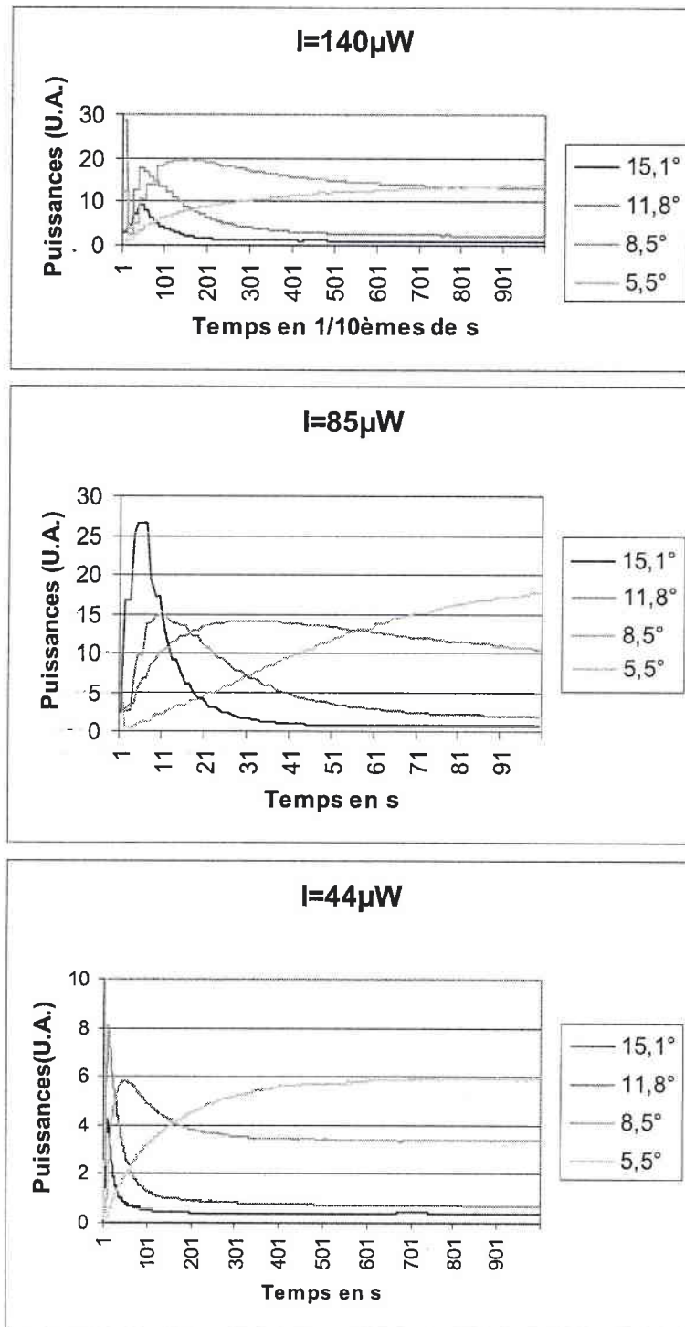
FIG. 4.24 – Evolution du fanning dans le cristal dopé pour un angle d'incidence de 18.6° dans les directions principales prévues par le modèle développé en 4.5.1 pour diverses puissances incidentes.
