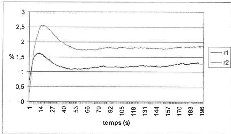
FIG. 5.63 – Evolution des rendements du DPCM pour un angle de fanning du faisceau 2 compris entre \theta_{f,1}^{(1)} et \theta_{f,1}^{(2)} , d = 360 \mu m
