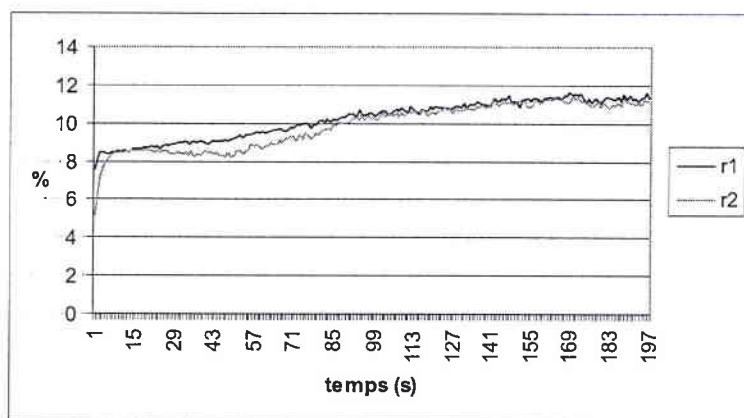
FIG. 5.23 – Evolution temporelle des rendements du DPCM dans le cristal non dopé avec deux faisceaux fins pour h = 60 \mu m
