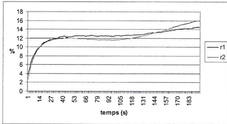
FIG. 5.62 – Evolution des rendements du DPCM pour un angle de fanning du faisceau 2 compris entre \theta_{f,1}^{(1)} et \theta_{f,1}^{(2)} , d = 240 \mu m
