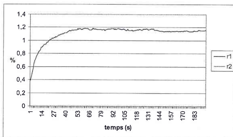
FIG. 5.38 – Evolution des rendements du DPCM avec un faisceau large et un faisceau fin dans le cristal non dopé d = -840 \mu m
