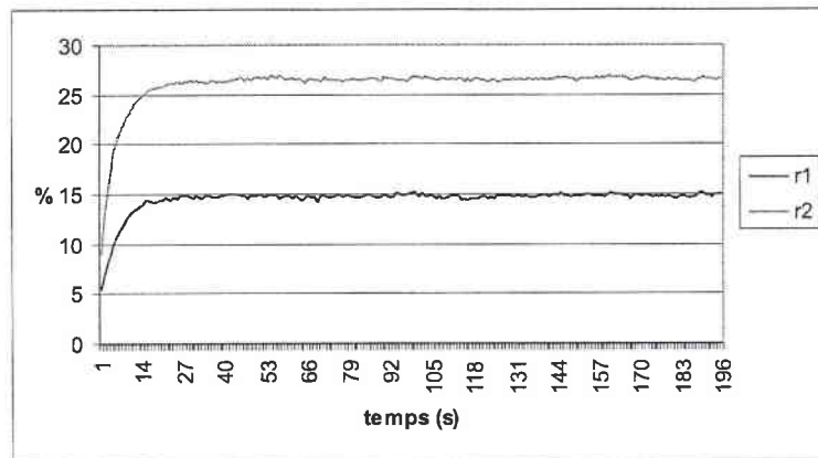
FIG. 5.8 – Evolution temporelle des rendements du DPCM dans le cristal non dopé avec deux faisceaux fins pour d = 240 \mu m
