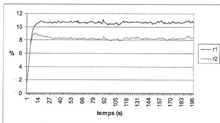
FIG. 5.11 – Evolution temporelle des rendements du DPCM dans le cristal non dopé avec deux faisceaux fins pour d = -480 \mu m
