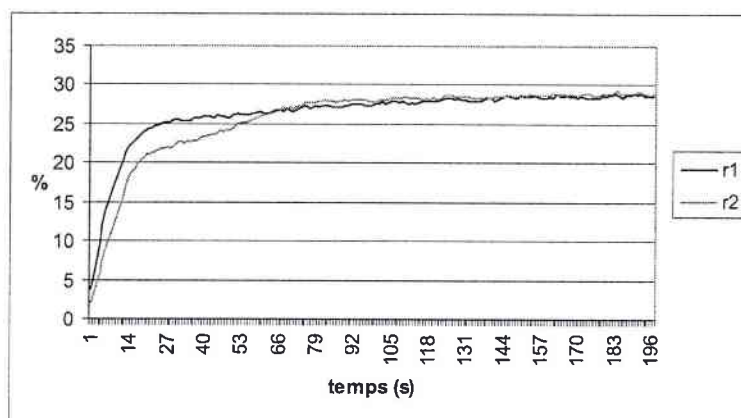
FIG. 5.10 – Evolution temporelle des rendements du DPCM dans le cristal non dopé avec deux faisceaux fins pour d = -240 \mu m
