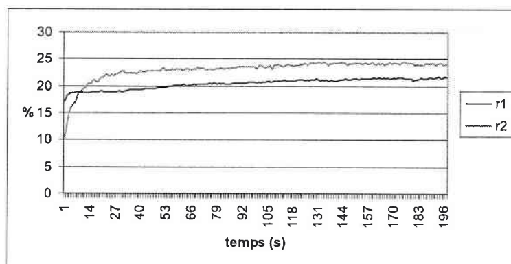
FIG. 5.22 – Evolution temporelle des rendements du DPCM dans le cristal non dopé avec deux faisceaux fins pour h = 40 \mu m
