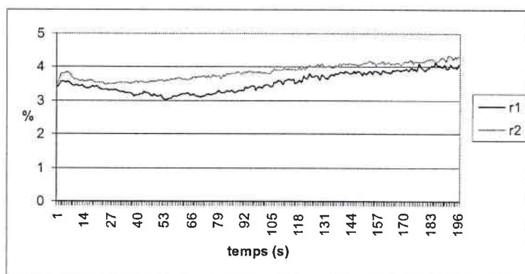
FIG. 5.24 – Evolution temporelle des rendements du DPCM dans le cristal non dopé avec deux faisceaux fins pour h = 80 \mu m
