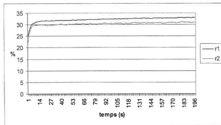
FIG. 5.9 – Evolution temporelle des rendements du DPCM dans le cristal non dopé avec deux faisceaux fins pour d = 0 \mu m
