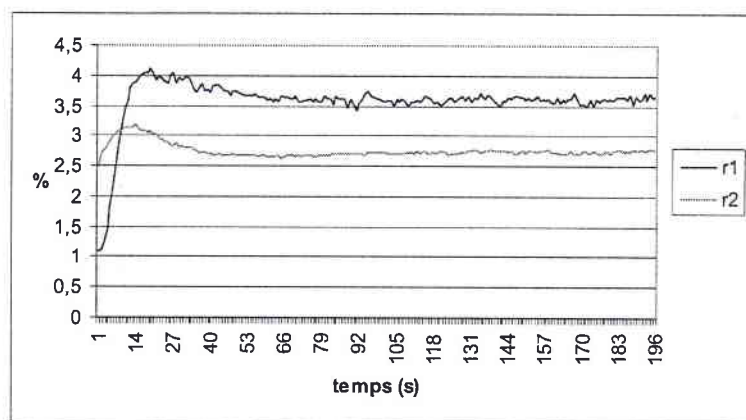
FIG. 5.12 – Evolution temporelle des rendements du DPCM dans le cristal non dopé avec deux faisceaux fins pour d = -721 \mu m
