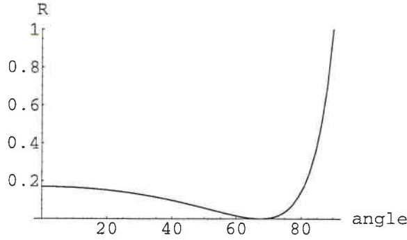
FIG. 5.2 – Evolution du rapport de l'intensité lumineuse réfléchie par rapport à celle incidente calculée en fonction de l'angle d'incidence en degrés pour un faisceau passant de l'air dans le cristal de BaTiO 3
