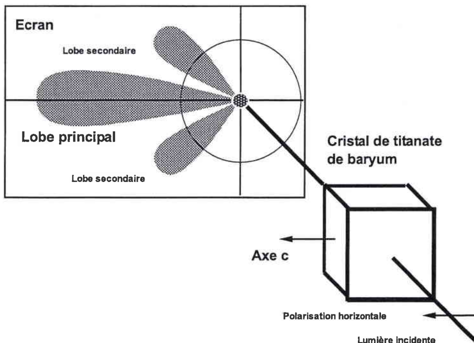
FIG. 4.2 – Figure de fanning pour un cristal de \text{BaTiO}_3
