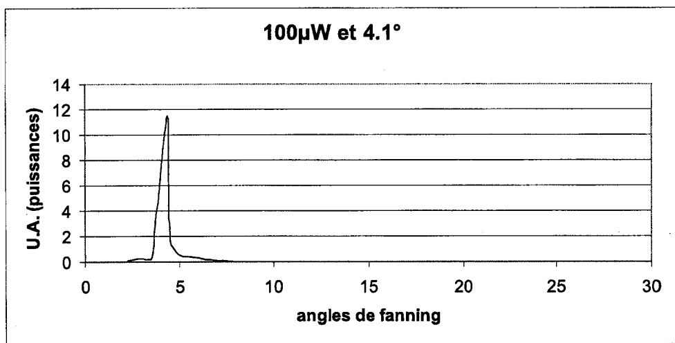
FIG. 4.10 – Figure de fanning typique obtenue dans le cristal non dopé pour une face d'entrée -c , et un angle d'incidence 4.1^\circ
