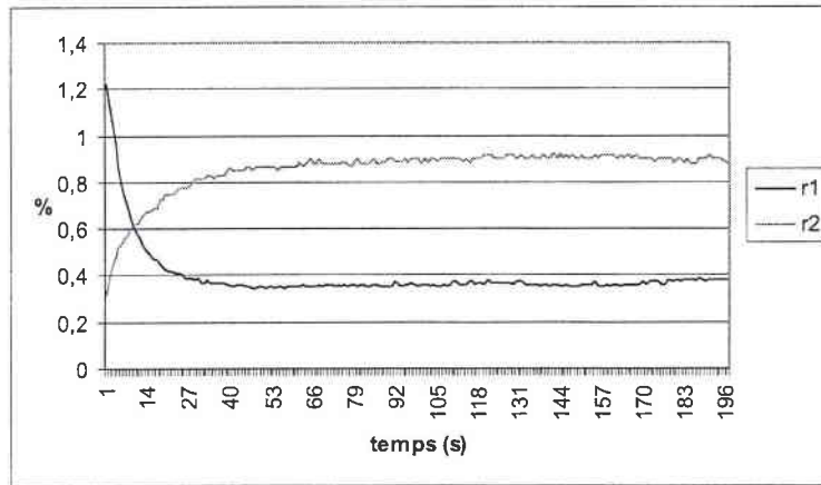
FIG. 5.65 – Evolution des rendements du DPCM pour un angle de fanning du faisceau 2 compris entre \theta_{f,1}^{(1)} et \theta_{f,1}^{(2)} , d = 600 \mu m
