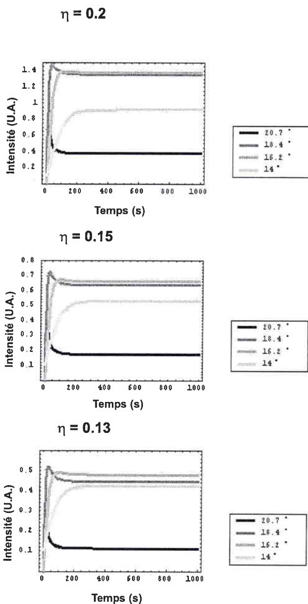
FIG. 4.27 – Evolution calculée du fanning dans les directions principales prévues pour différentes valeurs du paramètre \eta . Courbes obtenues avec les paramètres du cristal non dopé.
