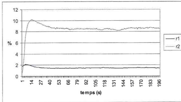
FIG. 5.7 – Evolution temporelle des rendements du DPCM dans le cristal non dopé avec deux faisceaux fins pour d = 480 \mu m
