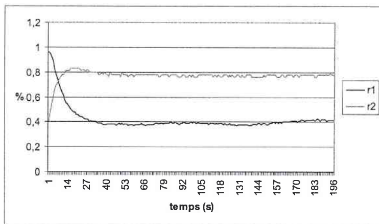
FIG. 5.64 – Evolution des rendements du DPCM pour un angle de fanning du faisceau 2 compris entre \theta_{f,1}^{(1)} et \theta_{f,1}^{(2)} , d = 480 \mu m
