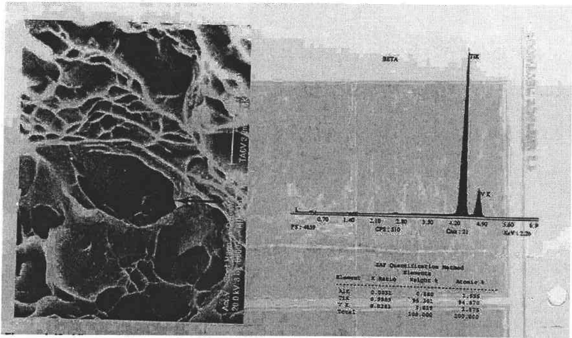
Figure 4-2 : Analyse chimique en fond de cupule. On peut voir que l'aluminium (élément alphas) est inférieur à 2%. Ce qui peut être un grain \beta .
