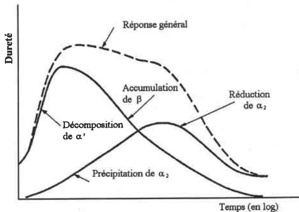
Abbildung 8-1 Ausscheidung der \alpha_2 -Phase. Härtesteigerung während einer Anlassglühung bei 500°C
