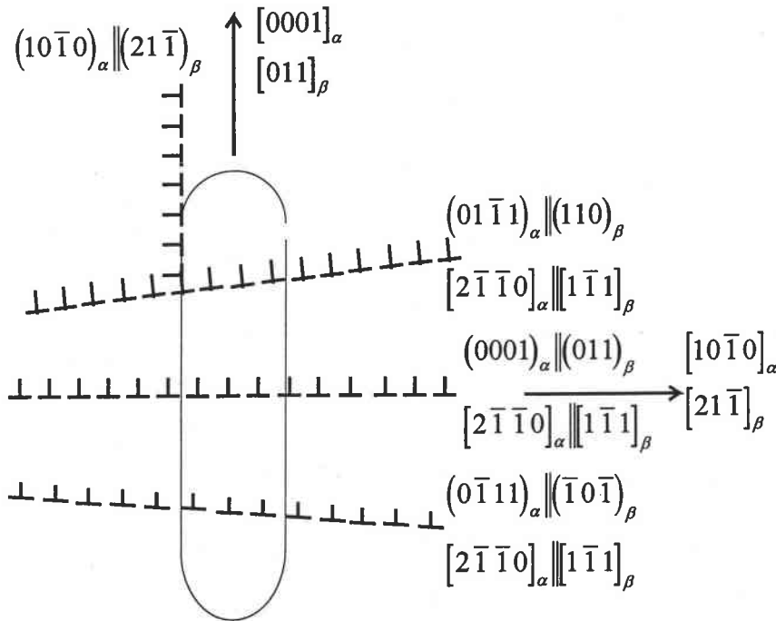
Figure 2-1 : Coïncidence entre systèmes de glissement
