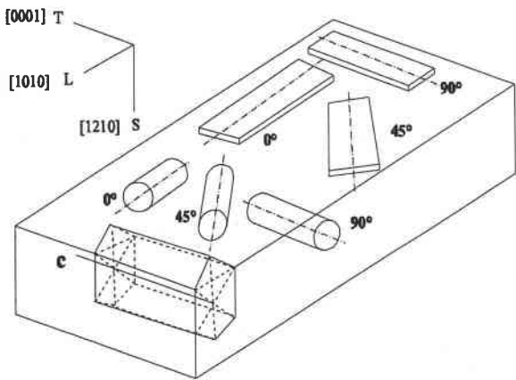
Figure 4-1 : Représentation schématique de la tôle et du monocristal (0°, 90°, 0°) ainsi que les éprouvettes de traction et de compression et leurs sens de prélèvement.
