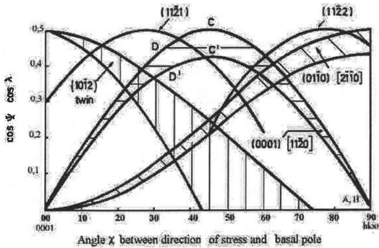
Figure 4-1 : Facteur de Schmid de chacun des systèmes de glissement en fonction de l'angle entre l'axe de contrainte et l'axe \langle c \rangle
