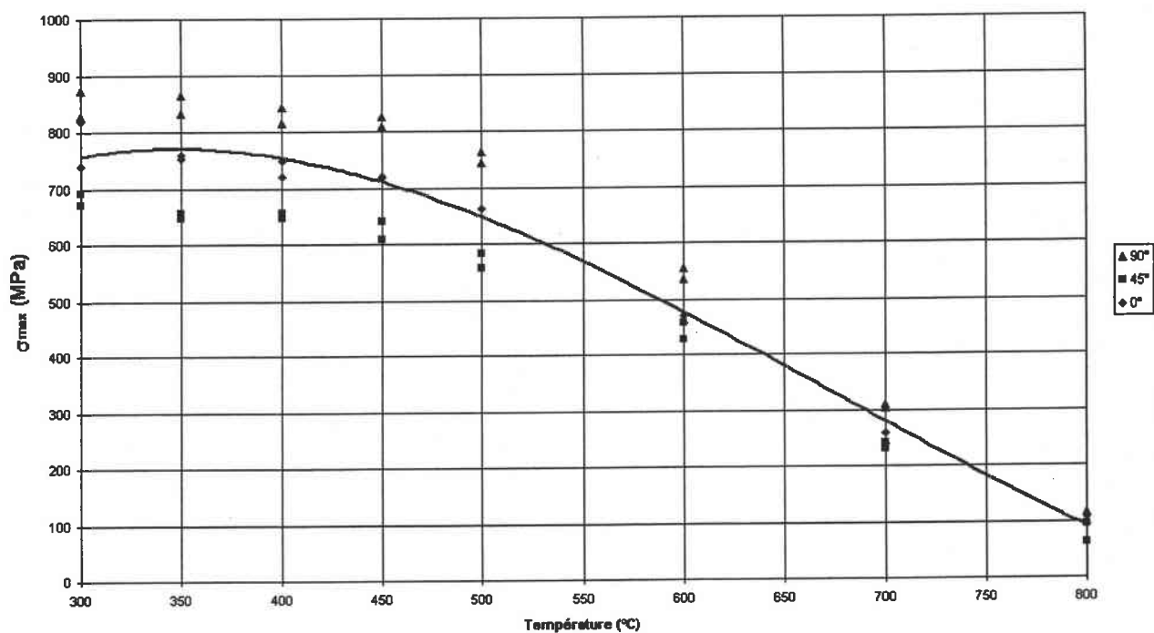
Figure 4-6 Graphe \sigma_{max} = f(T) pour une vitesse de \dot{\epsilon} = 10^{-3} \text{ s}^{-1} et pour les trois directions de prélèvement.
