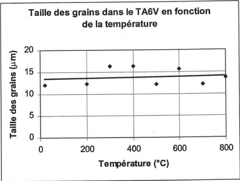
Figure 4-1 La taille de grains \alpha en fonction de la température dans le TA6V
