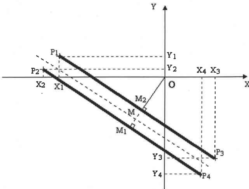
Figure 3-3 : Les quatre points ( P_1 , P_2 , P_3 , P_4 ) forment la paire de lignes de Kikuchi
