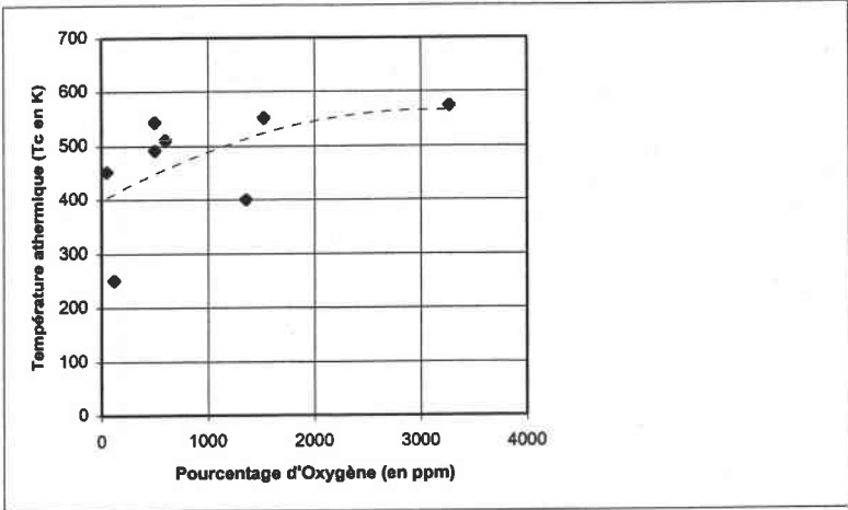
Abbildung 8-1 Einfluß der Sauerstoffkonzentration auf die « athermische » Temperatur
