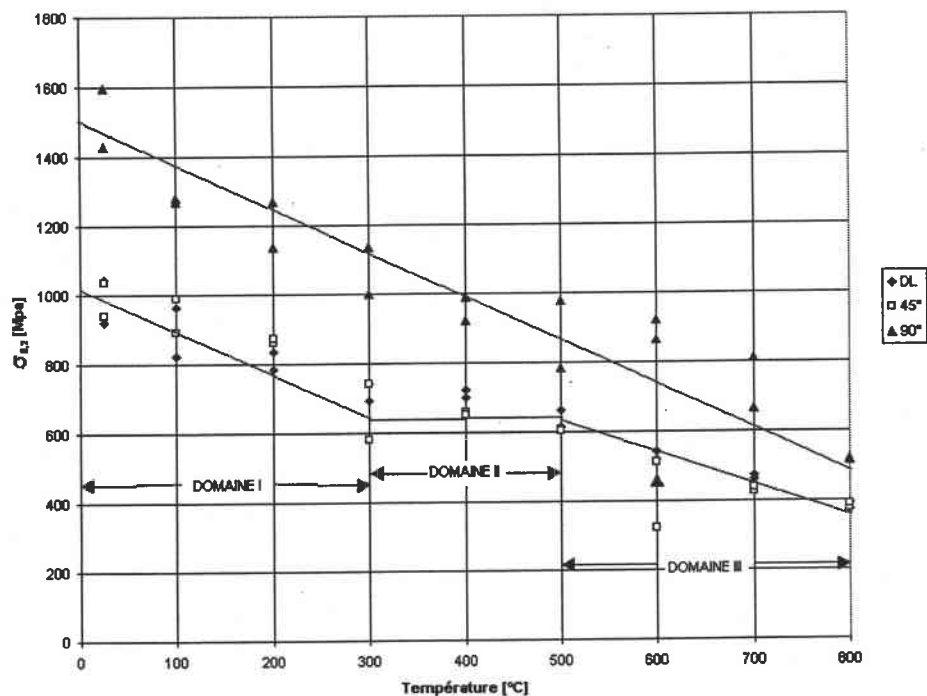
Figure 4-1 Courbe \sigma_{0.2\%} = f(T) pour une vitesse de \dot{\epsilon} = 1 \text{ s}^{-1} et pour les trois directions de prélèvement pour les essais de compression.
