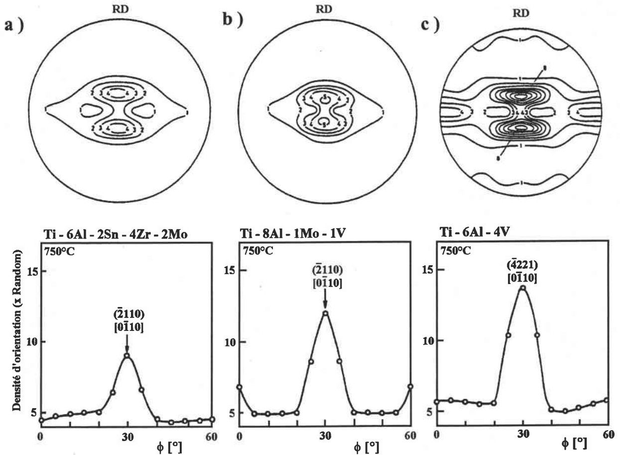
Figure 2-1 : Figures de Pôles (0002) avec le maximum de densité d'orientation pour les sections \phi de l'espace FDO ( \psi\theta\phi ). a) Ti-6Al-2Sn-4Zr-2Mo b) Ti-8Al-1Mo-1V c) Ti-6Al-4V. Laminage à chaud à 750°C, réduction de 94% et refroidi à l'air
