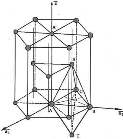
Figure 2-1 : Vecteurs de Burgers dans le réseau hexagonal compact
