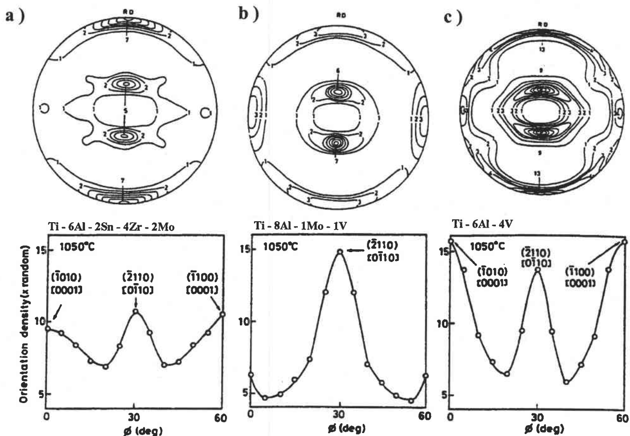
Figure 2-1 Figures de Pôles (0002) avec le maximum de densité d'orientation pour les sections \phi de l'espace FDO ( \psi\theta\phi ). a) Ti-6Al-2Sn-4Zr-2Mo b) Ti-8Al-1Mo-1V c) Ti-6Al-4V. Laminage à chaud à 1050°C, réduction de 94% et refroidi à l'air
