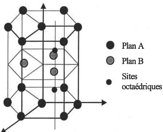
Abbildung 8-1 Hexagonal-kompakte Kristallstruktur
