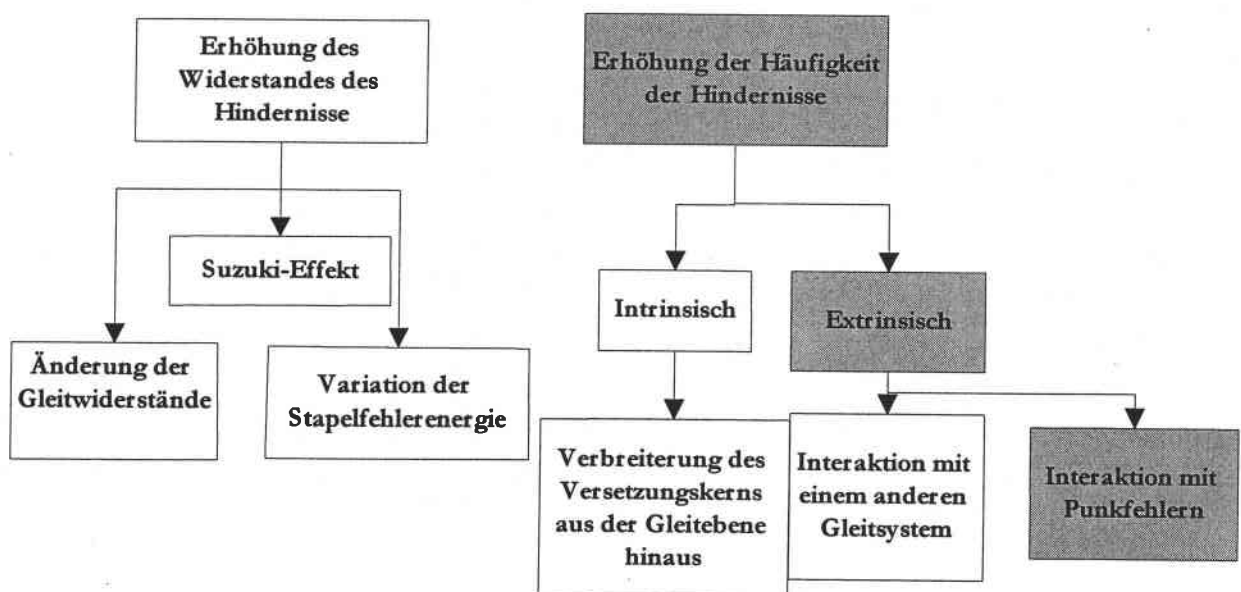
Abbildung 10-1 : Annahmen über das athermische Plateau der Streckgrenze
