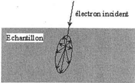
Figure 3-1 : Représentation schématique de la diffusion inélastique localisée sur un seul point de l'éprouvette
