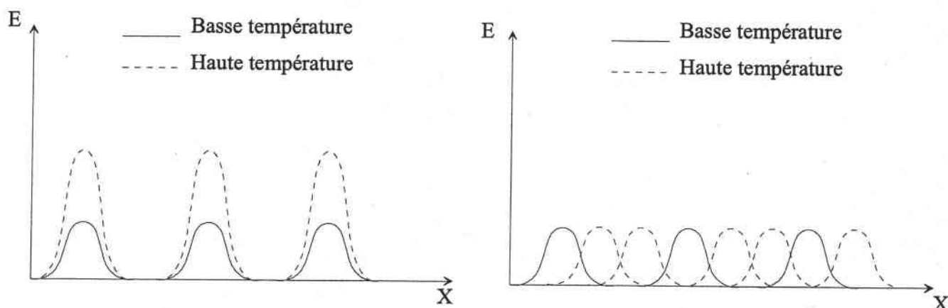
Figure 5-1: Schéma de l'énergie d'interaction (E) de la dislocation avec les obstacles en fonction du déplacement (X); a) cas de l'augmentation de la force des obstacles; b) cas de l'augmentation de la fréquence d'apparition des obstacles.
