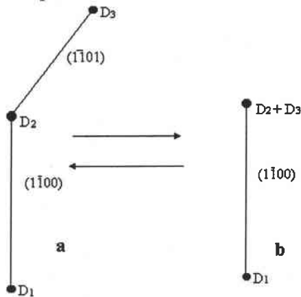
Abbildung 8-1 Versetzungsreaktion
