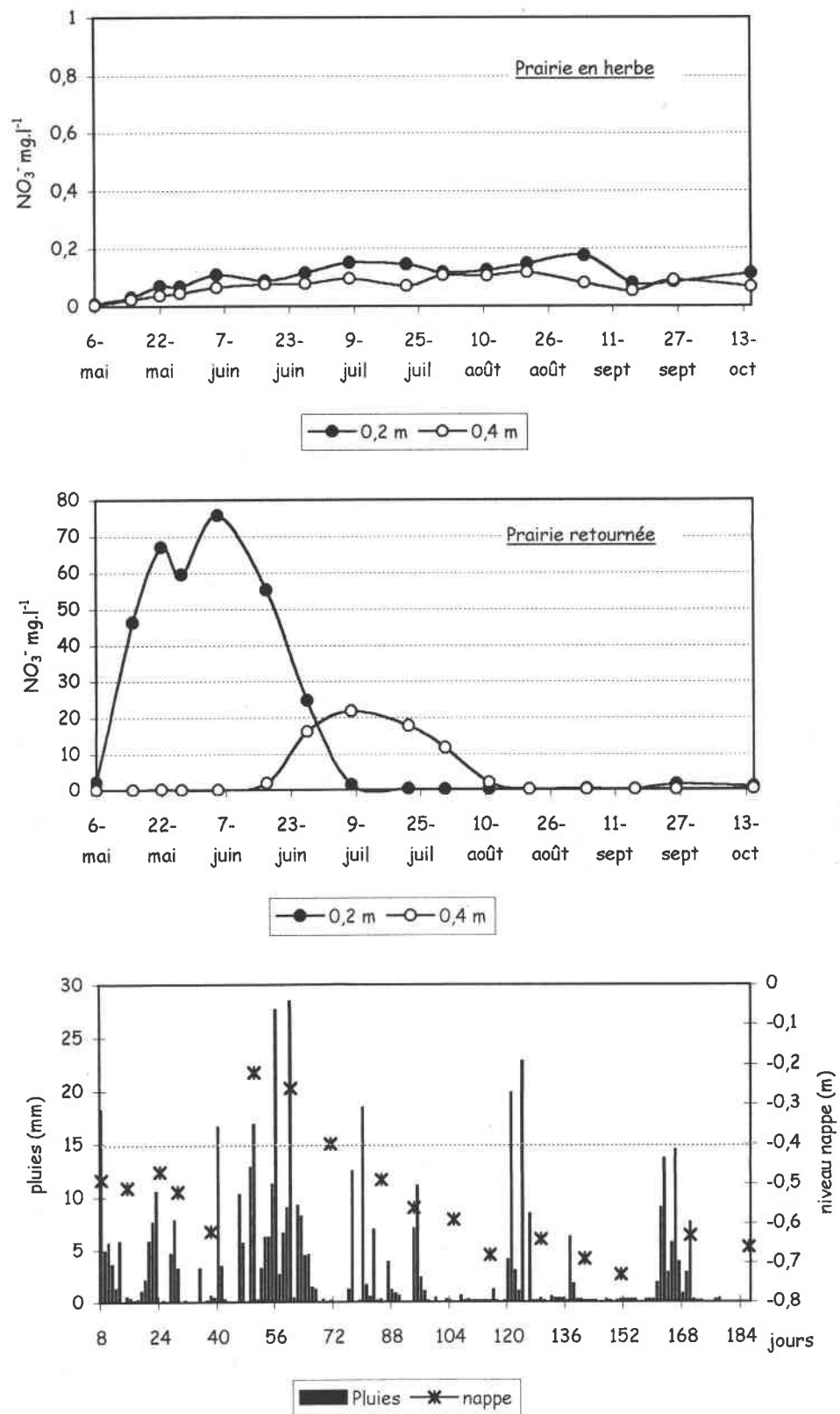
Figure IX.6. Distribution verticale des nitrates dans la solution du sol (0,2 et 0,4 m) dans les micro-parcelles C enherbée et D retournée. Les micro-parcelles subissent une fertilisation azotée mixte le 28 avril 1997 (jour 0) et le suivi couvre la période du 6 mai au 31 octobre 1997 (jours 8 à 186)
