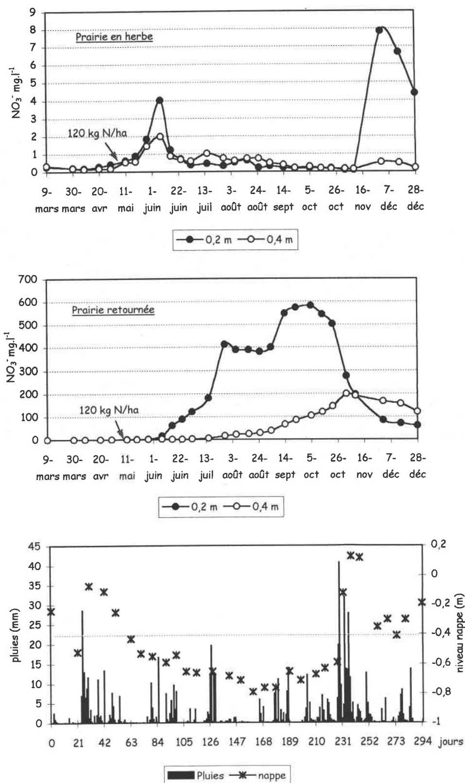
Figure IX.9. Distribution verticale des nitrates dans la solution du sol (0,2 et 0,4 m) dans les micro-parcelles C enherbée et D retournée. Les micro-parcelles subissent une fertilisation azotée mixte le 7 mai 1998 (jour 59) et le suivi couvre la période du 9 mars au 28 décembre 1998 (jours 0 à 296)
