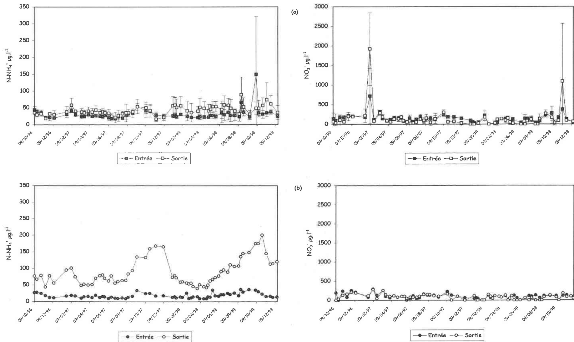
Figure VI.23. Variation des concentrations en azote ammoniacal et en nitrate à l'entrée et à la sortie du carré permanent E (MEG) dans la nappe superficielle (a) et profonde (b)
