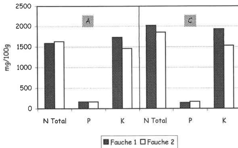
Figure VIII.12. Teneurs moyennes en N, P et K dans les fourrages lors des deux coupes dans les micro-parcelles A témoin et C fertilisée (Apport de 120 kg d'N/ha le 7 mai 1998)
