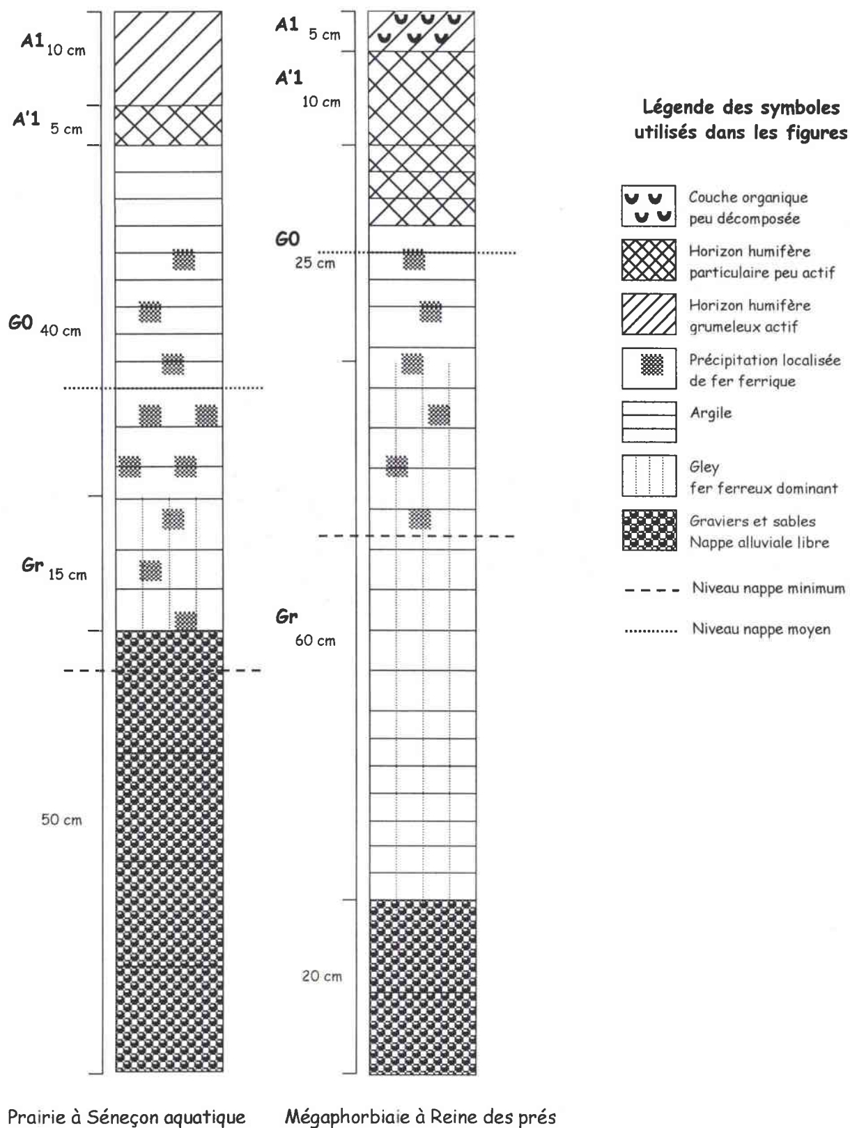
Figure IV.1. Profils de sol (1,20 m de profondeur) réalisés dans les deux prairies
