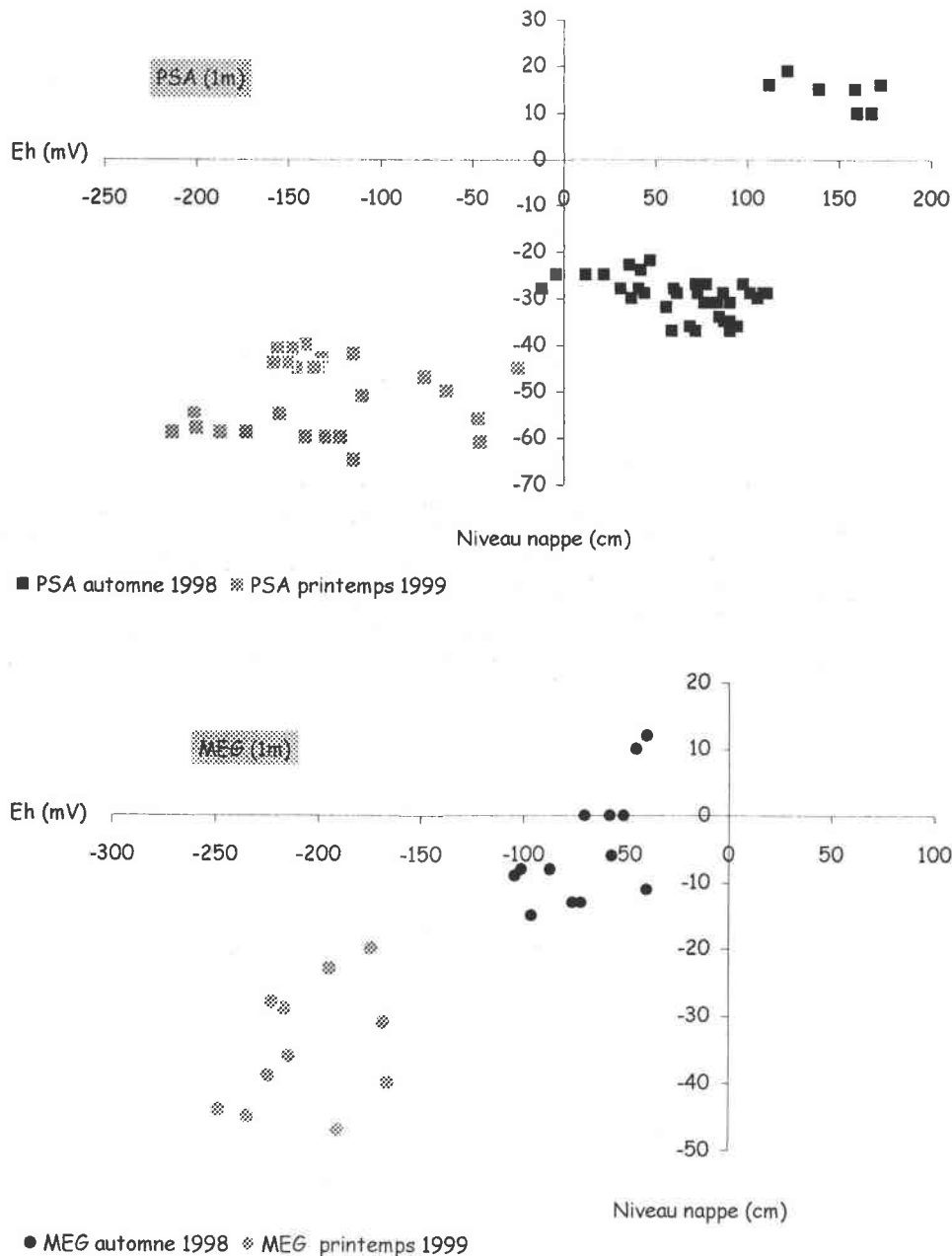
Figure VII.5. Variation du potentiel rédox dans la nappe superficielle en fonction du type de végétation, de la saison et du niveau hydrique
