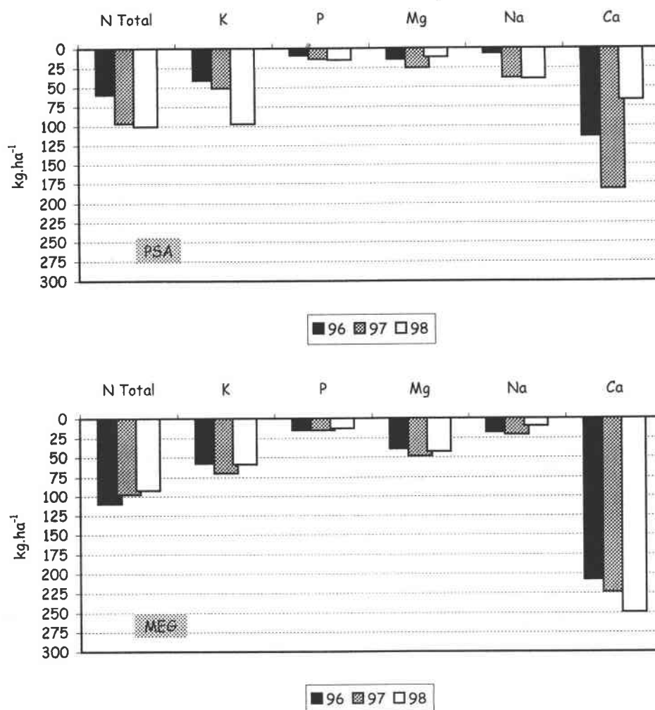
Figure VIII.4. Comparaison des quantités de nutriments stockées (en \text{kg.ha}^{-1} ) dans les organes souterrains des deux prairies une semaine après la fauche en 1996 et après les saisons de végétation de 1997 et 1998
