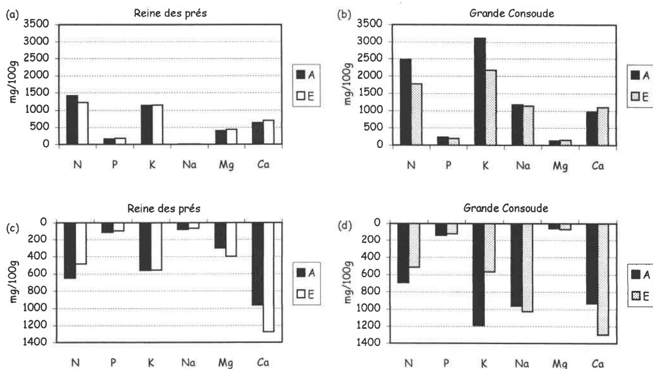
Figure VIII.7. Teneurs en nutriments des parties épigées (a, b) et hypogées (c, d) de deux espèces prélevées dans des prairies différentes (micro-parcelles A et E)
