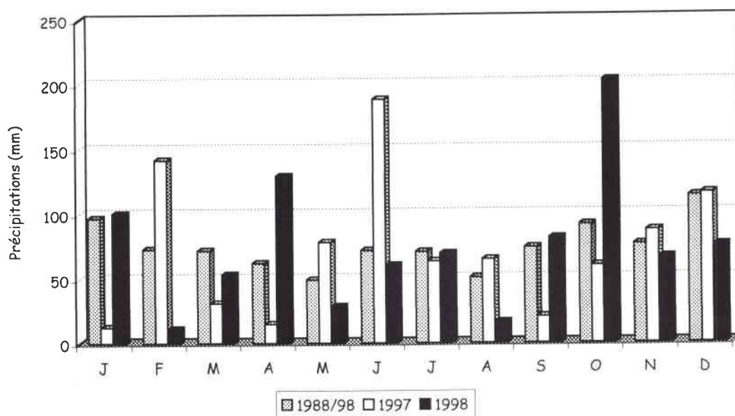
Figure II.8. Précipitations moyennes mensuelles à Stenay, période 1988/98 et les années 1997 et 1998
