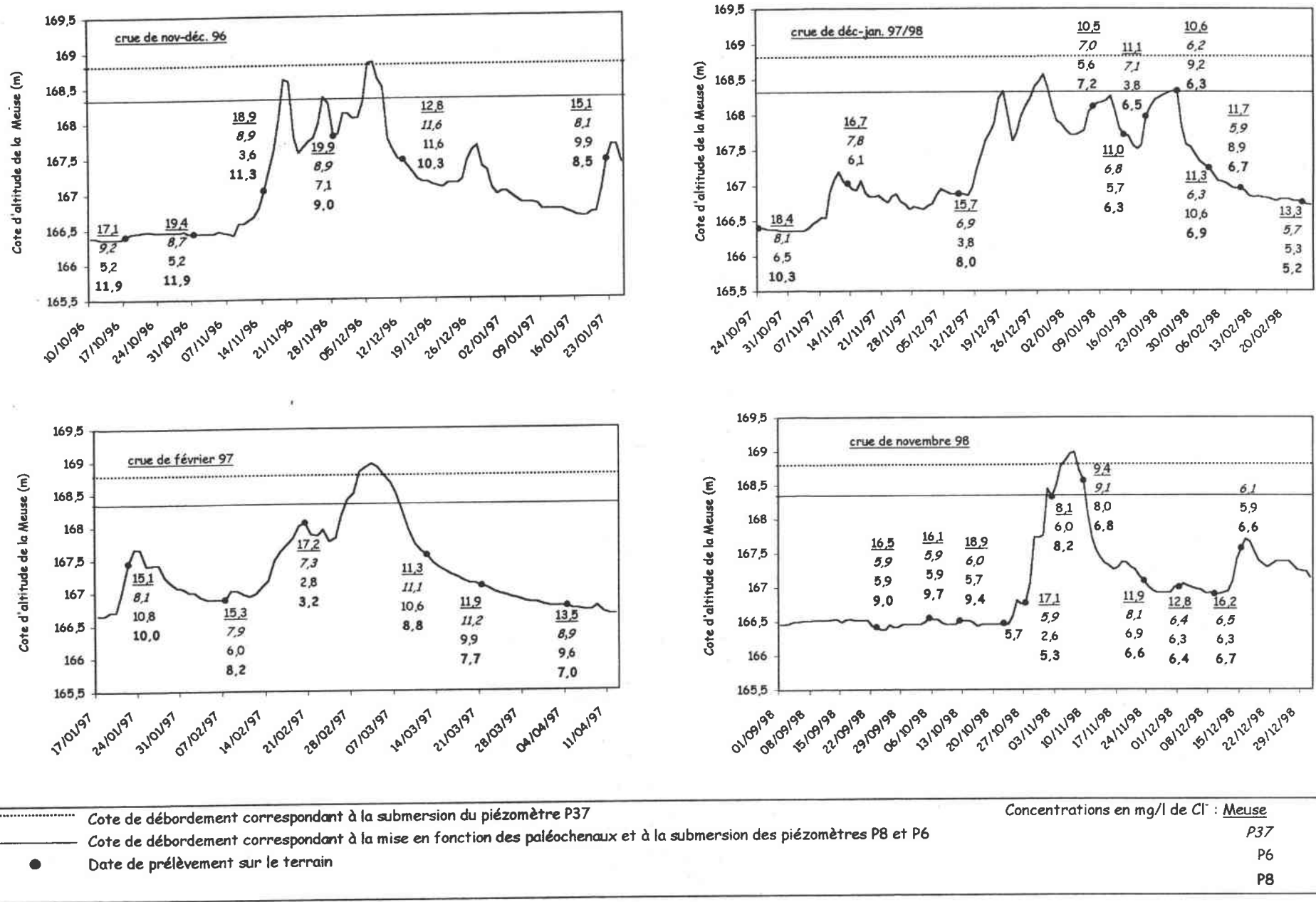
Figure V.10. Evolution des teneurs en chlorure dans la nappe et la Meuse lors de 4 événements hydro-climatologiques observés pendant la période d'étude
