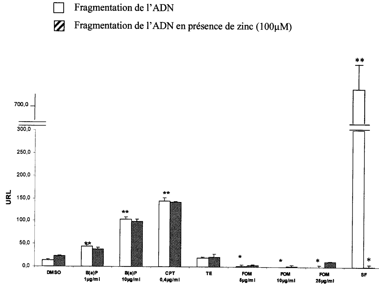
Figure 28. Fragmentation de l'ADN, mesurée à l'aide du kit 'Cellular DNA Fragmentation ELISA', dans les cellules SHE exposées au BaP, à la camptothécine (CPT), par rapport au témoin DMSO ; au fomesafen (FOM) et à un milieu sans sérum (SF), par rapport au témoin (TE) sans traitement. Les substances ont été appliquées en présence ou non de ZnCl 2 (100μM). ** Résultats significativement différents des cellules traitées au DMSO ( p < 0.01 ), * résultats significativement différents des cellules témoins ( p < 0.05 ), * résultats significativement différents par rapport au traitement sans zinc ( p < 0.01 ).
