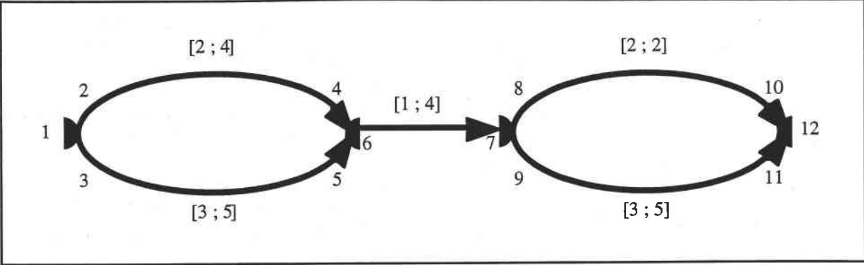
Figure IV- 6 : Représentation du produit à fabriquer
