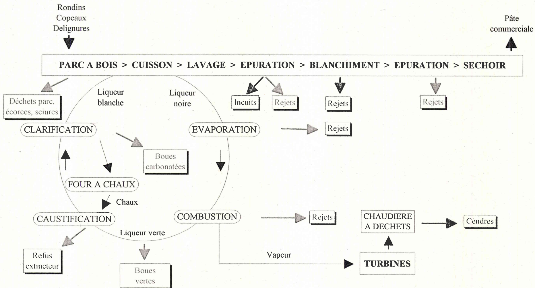
Figure 1.6 : Formation de déchets lors de la fabrication de la pâte à papier par le procédé Kraft (d'après Centre Technique du Papier, 1995).
