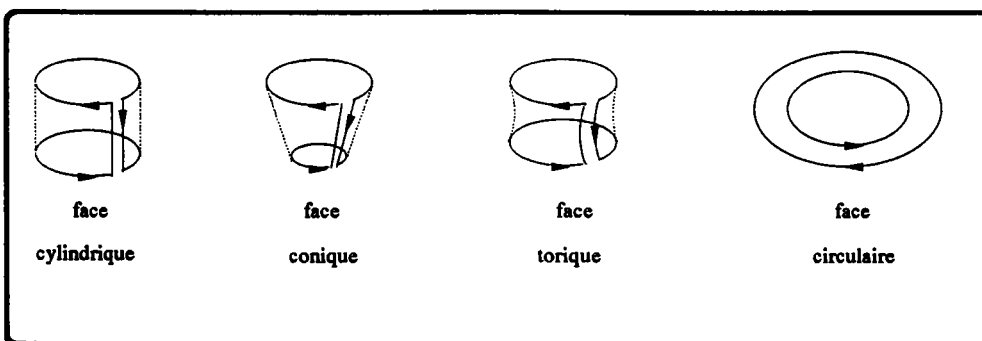
figure 4.7: faces autorisées dans un trou
