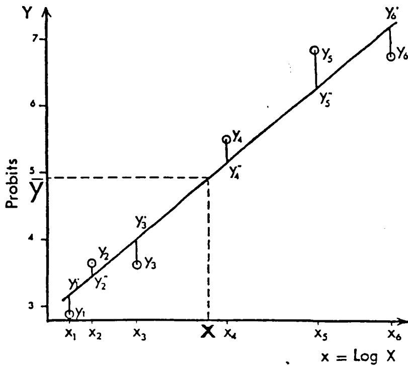
Fig. 12 : Droite de régression : Probit = f(\text{Log } X) (d'après RAMADE, 1977). X = élément toxique testé.
