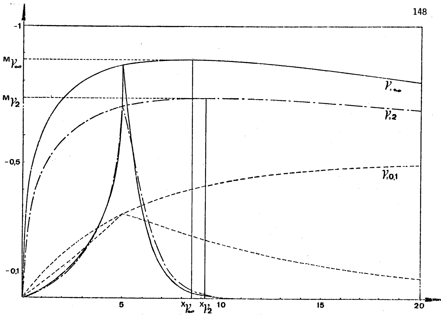
Fig. 11 : Evolution de l'onde de contrainte pour différentes longueurs de pénétration, lieu des extrémums.
