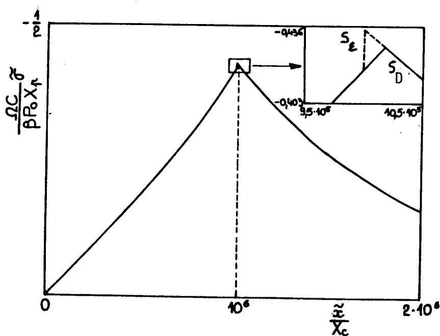
FIG. 8 : Comparaison des deux solutions approchées S_e et S_{e1} pour t = \frac{\tilde{t}}{T_c} = 10^6
