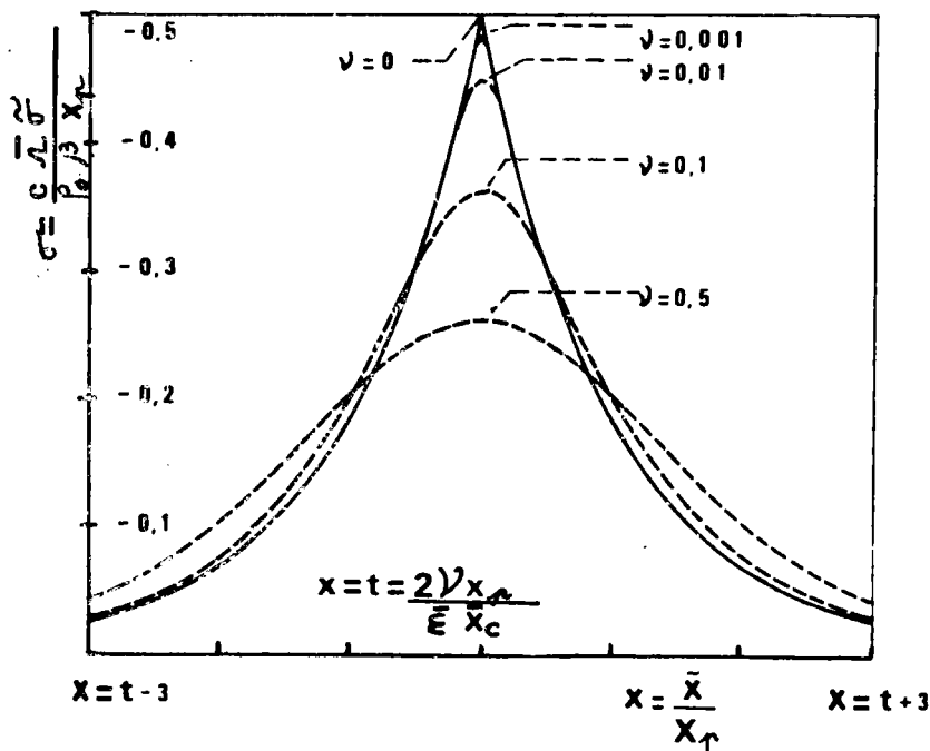
FIG. 7 : Amortissement du pic de contrainte en fonction de \nu = \frac{\varepsilon \bar{X}_c \bar{\Omega}}{2 X_p^2} \tilde{t}
