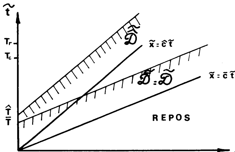
Fig : 1 Domaines de validité des ondes \hat{S} et \bar{S} Deuxième cas ( T_r \leq T_c )
