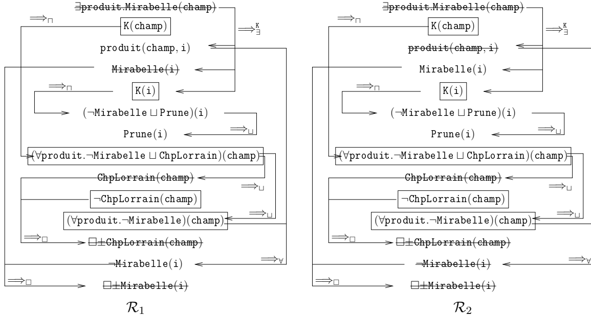
FIGURE 2.6 – AGraph obtenu après application des règles \Rightarrow , y compris \Rightarrow_{\square} , sur l'union des AGraph \mathcal{G}_1 et \mathcal{H}_1 obtenus dans l'exemple 2.5.5. Les formules impliquées par \mathcal{A}_{\mu} et \mathcal{T} sont encadrées pour symboliser le fait qu'elles ne seront pas remises en cause lors de la révision.
