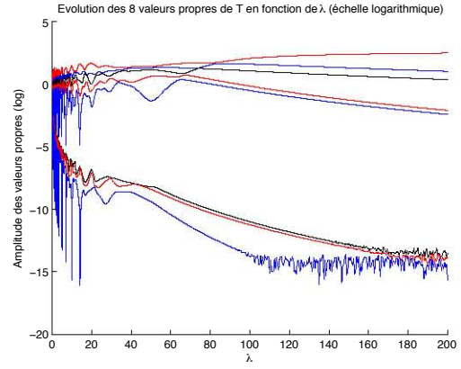
(b) Echelle logarithmique de l'amplitude des 8 valeurs propres de \mathbb{T}
