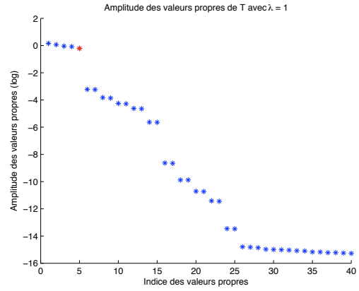
(d) \lambda = 1 (= 50\delta = d/20)
