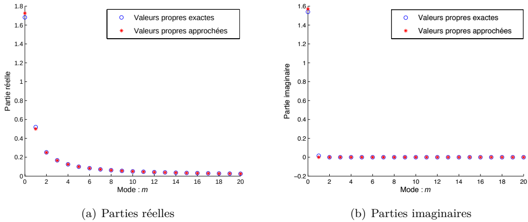
FIGURE 5.1 – Comparaison entre les valeurs propres exactes (5.14) et approchées (5.16) de L , pour ka = 0.2 et N = 20 modes (positifs).
