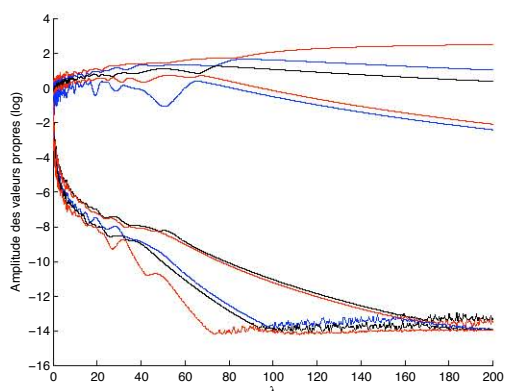
(c) Echelle logarithmique de l'amplitude des 10 plus grandes valeurs propres de \mathbb{T}
