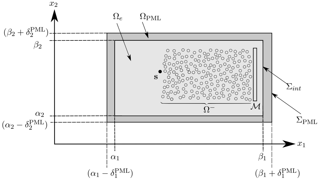
FIGURE 3.8 – Représentation du domaine \Omega_T , composé des sous-domaines \Omega_e et \Omega_{\text{PML}} ainsi que de leurs frontières \Sigma_{\text{int}} et \Sigma_{\text{PML}} . Le domaine \Omega_e est le domaine d'étude sur lequel une approximation de la solution est calculée. Il contient notamment le miroir à retournement temporel \mathcal{M} , les obstacles \Omega^- et la source \mathbf{s} . L'épaisseur de la PML dans la direction x_1 est \delta_1^{\text{PML}} , et \delta_2^{\text{PML}} dans la direction x_2 .
