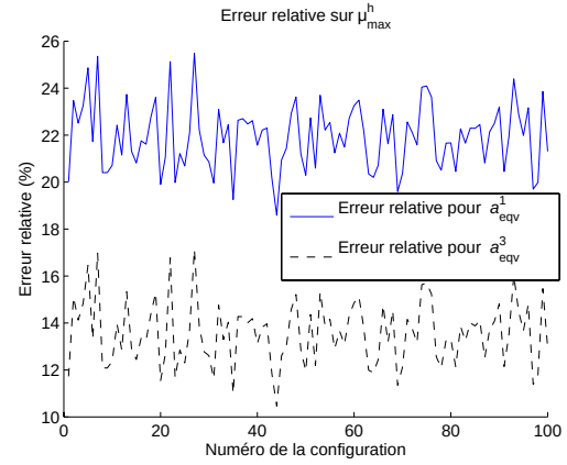
(d) Erreur relative sur de \mu_{max}
