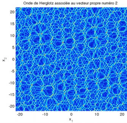
(c) Module de l'onde de Herglotz associée au deuxième vecteur propre de \mathbb{T}
