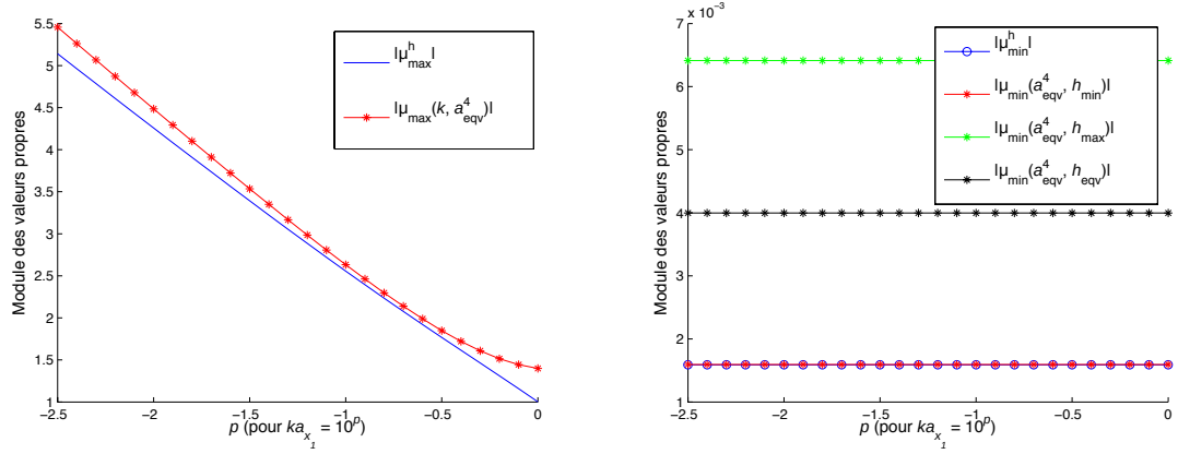
(a) Plus grandes valeurs propres numérique et estimée. (b) Plus petites valeurs propres numérique et estimées.
