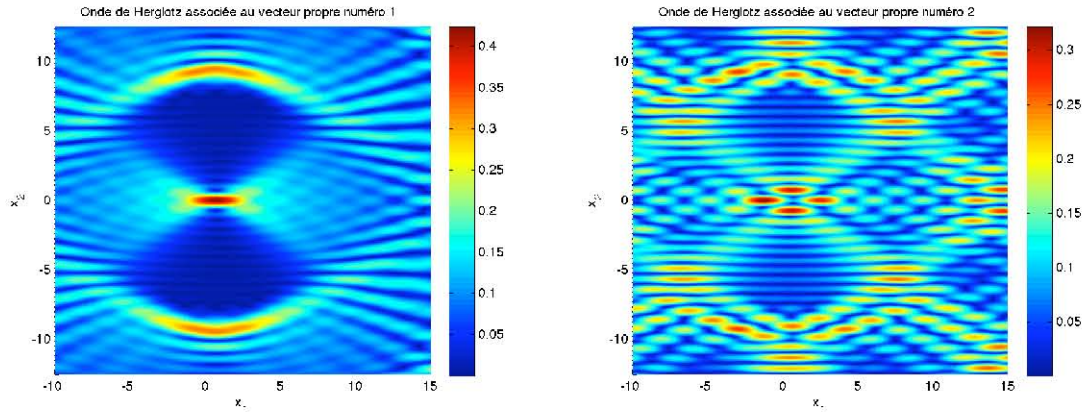
(b) Module de l'onde de Herglotz associée au premier vecteur propre de \mathbb{T} (c) Module de l'onde de Herglotz associée au deuxième vecteur propre de \mathbb{T}
