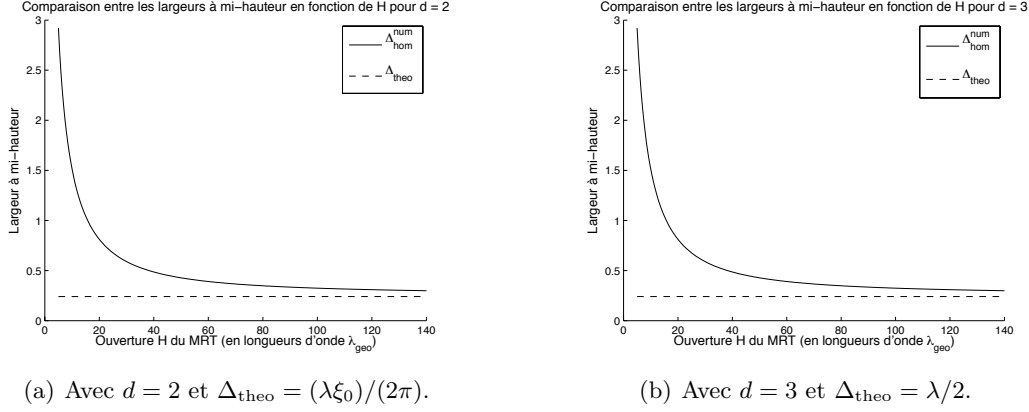
FIGURE 3.14 – Évolution de la largeur à mi-hauteur \Delta_{\text{hom}}^{\text{num}} en fonction de l'ouverture H du miroir à retournement temporel et comparaison avec la valeur limite \Delta_{\text{theo}} , donnée par (3.29). La dimension du problème est d = 2 sur la figure (a) et d = 3 sur la figure (b). Dans les deux cas, nous avons k = k_{\text{geo}} , \lambda = \lambda_{\text{geo}} et D = 20\lambda_{\text{geo}} .
