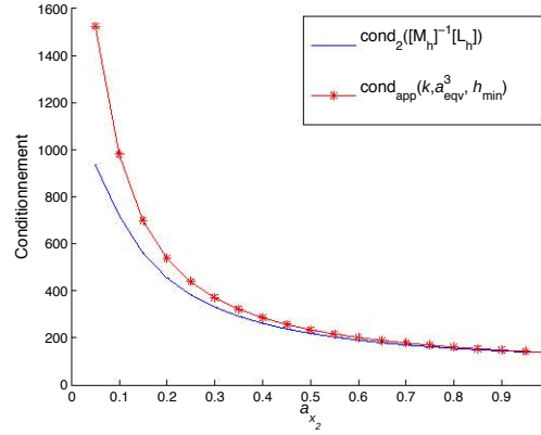
(c) Ellipse ( a_{x_1} = 1 et k = 0.2 ) : conditionnements numériques et estimé en fonction du demi-axe a_{x_2} , avec N_h = 60 .
