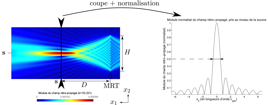
FIGURE 3.12 – Coupe au niveau de la source du module du champ rétro-propagé (figure de gauche). Après normalisation, nous calculons la largeur à mi-hauteur correspondant à la largeur du pic central (figure de droite).
