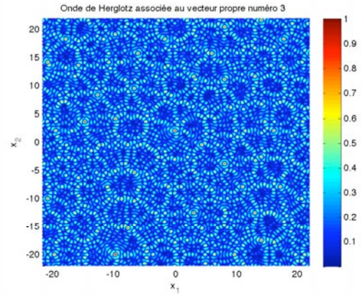
(d) Module de l'onde de Herglotz associée au troisième vecteur propre de \mathbb{T}
