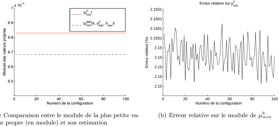
FIGURE 5.26 – Comparaison entre la valeur propre de plus petit module \mu_{\min}^h de la matrice [M_h]^{-1}[L_h] et son estimation (5.106) pour des petits rectangles de demi-côtés a_{x_1} = 0.1 et a_{x_2} = 0.025 . Chaque rectangle est discrétisé à l'aide de N_h = 48 segments (12 par arrête). Pour chacune des 100 configurations différentes, nous plaçons M = 30 petits rectangles aléatoirement dans la boîte [0, 4] \times [0, 4] , avec k = 0.1 et b \geq 0.3 (= 3a_{x_1}) .
