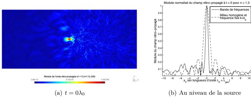
FIGURE 3.31 – Module de l'onde rétro-propagée à l'instant t = 0 de la focalisation, dans le domaine de calcul \Omega_e (figure (a)) et au niveau de la source, après normalisation (figure (b)). L'indice à l'intérieur des obstacles est de n = 1.3 . Ces deux images font suite à la figure 3.30.
