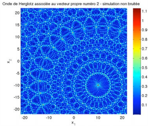
(d) Module de l'onde de Herglotz associée au deuxième vecteur propre de \mathbb{T} (e) Simulation bruitée - Module de l'onde de Herglotz associée au deuxième vecteur propre de \tilde{\mathbb{T}}
