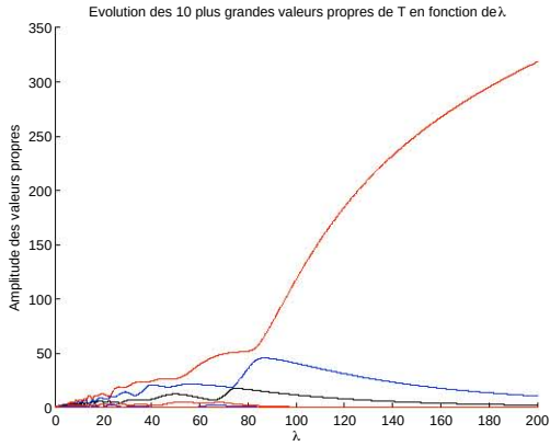
(a) Amplitude des 10 plus grandes valeurs propres de \mathbb{T}
