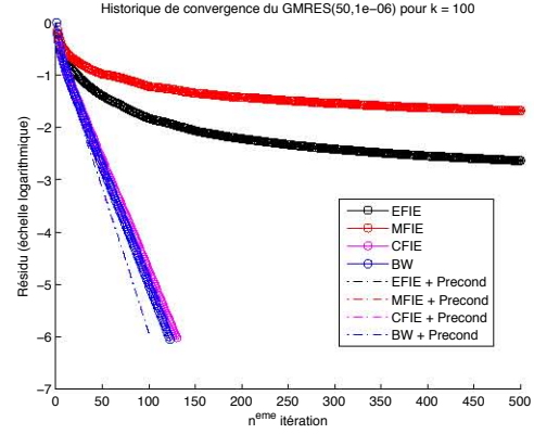
(b) Historique de convergence du GMRES(50,10 -6 )
