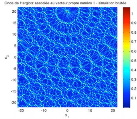
(b) Module de l'onde de Herglotz associée au premier vecteur propre de \mathbb{T} (c) Simulation bruitée - Module de l'onde de Herglotz associée au premier vecteur propre de \tilde{\mathbb{T}}
