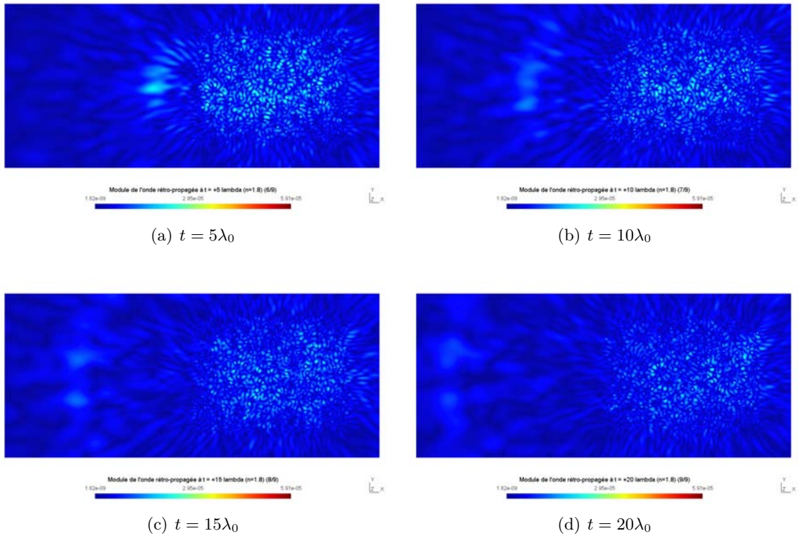
FIGURE 3.35 – Module de l'onde rétro-propagée par le MRT dans un milieu construit avec un contraste n = 1.8 . Les instants t sont ici positifs et correspondent à la propagation de l'onde après la focalisation sur le point source, présentée sur la figure 3.34.
