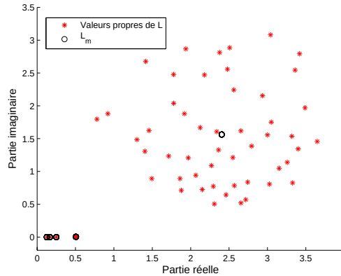
FIGURE 5.8 – Valeurs propres de la matrice \mathbb{L} pour M = 50 disques unitaires répartis aléatoirement dans la boîte [0, 1000] \times [0, 1000] , pour ka = 0.1 , kb = 10 et N = 4 . Les cercles représentent les \widehat{\mathbb{L}}_m , pour m = 0, \dots, N et les étoiles les valeurs propres de \mathbb{L} .
