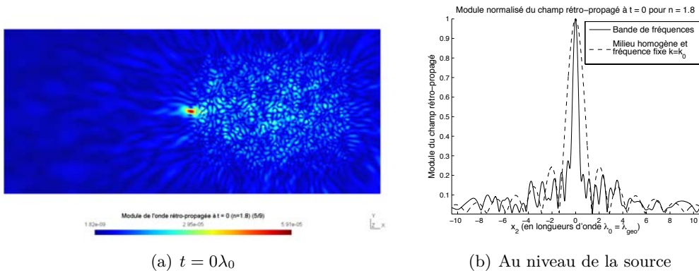
FIGURE 3.34 – Suite de la figure 3.33 à l'instant t = 0 de la focalisation. Le module du champ rétro-propagé est représenté dans le domaine de calcul \Omega_e sur la figure (a) et au niveau de la source (après normalisation) sur la figure (b).
