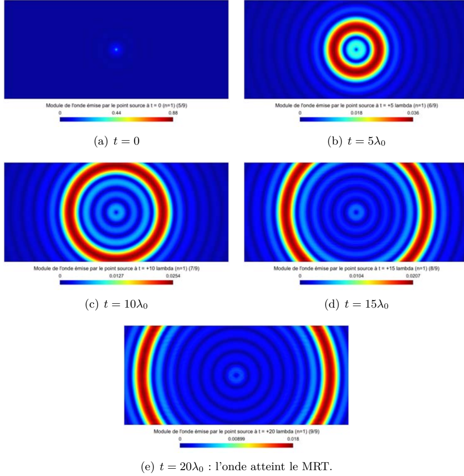
FIGURE 3.23 – Module de l'onde \mathcal{U}_E émise par le point source sur le domaine de calcul \Omega_e à différents instants t et dans un milieu homogène ( n = 1 ). La bande de fréquences utilisée étant [k_0 - k_0/5, k_0 + k_0/5] . Pour une meilleure lisibilité, l'échelle est adaptée à chaque pas de temps.
