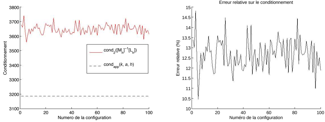
(a) Comparaison entre le conditionnement exact et approché
