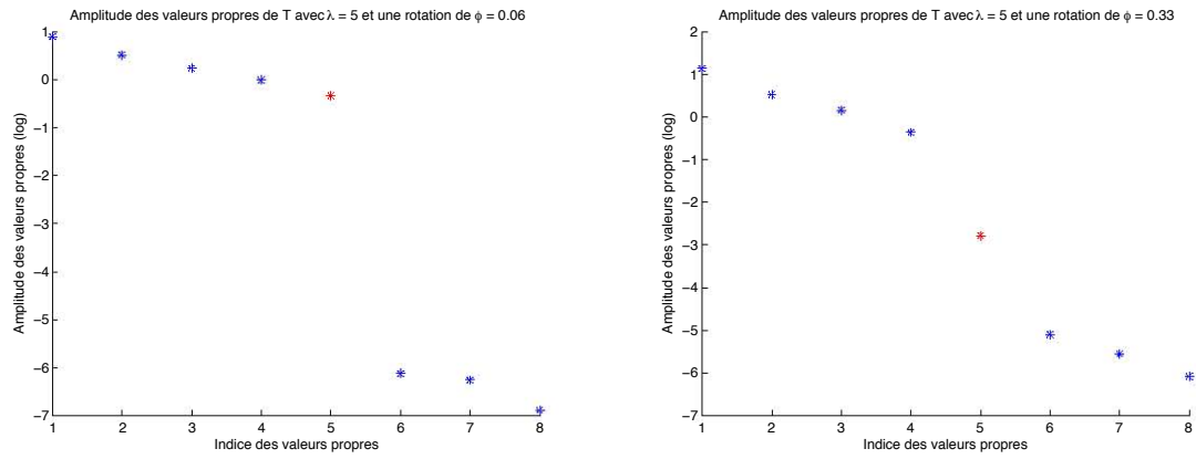
(a) Angle de déphasage \varphi = 0.06\text{rad} .
