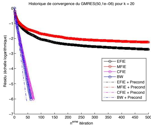
(c) Historique de convergence du GMRES(50,10 -6 )
