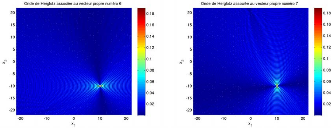
(c) Module de l'onde de Herglotz associée au sixième vecteur propre de \mathbb{T} (d) Module de l'onde de Herglotz associée au septième vecteur propre de \mathbb{T}
