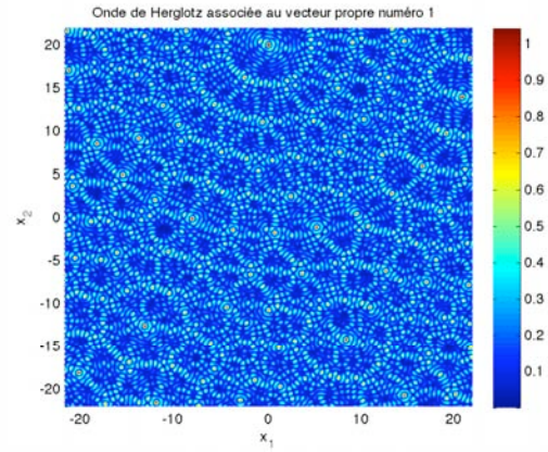
(b) Module de l'onde de Herglotz associée au premier vecteur propre de \mathbb{T}
