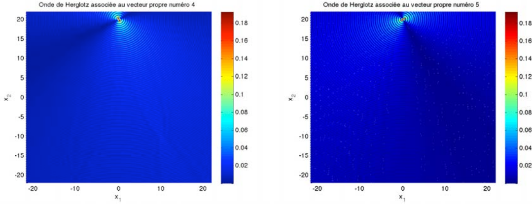
(a) Module de l'onde de Herglotz associée au quatrième vecteur propre de \mathbb{T} (b) Module de l'onde de Herglotz associée au cinquième vecteur propre de \mathbb{T}
