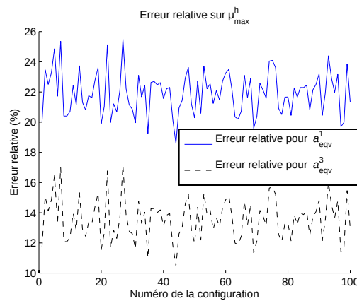
(e) Erreur relative sur le module de \mu_{max}
