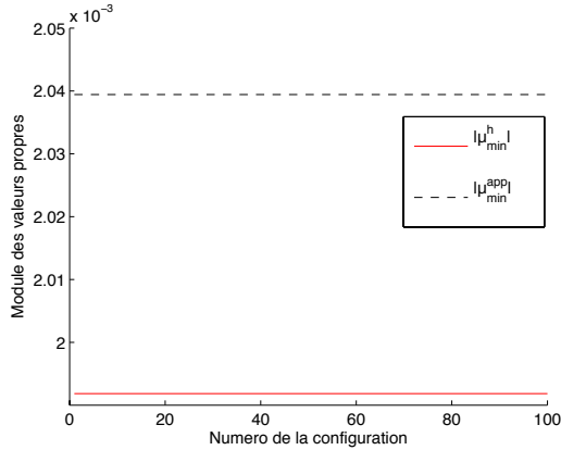
(a) Comparaison entre le module de la plus petite valeur propre (en module) et son estimation (5.106)
