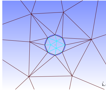
(c) Agrandissement au niveau du point source \mathbf{s} . En bleu turquoise le maillage du disque B_{\varepsilon_{\mathbf{s}}} supportant \eta_{\mathbf{s}} .
