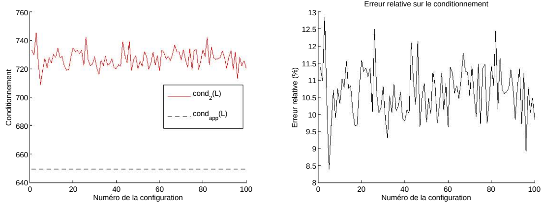
(a) Comparaison entre le conditionnement exact et ap- (b) Erreur relative sur le conditionnement en pourcen- proché tage (voir relation (5.105))
