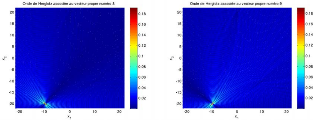
(e) Module de l'onde de Herglotz associée au huitième vecteur propre de \mathbb{T} (f) Module de l'onde de Herglotz associée au neuvième vecteur propre de \mathbb{T}
