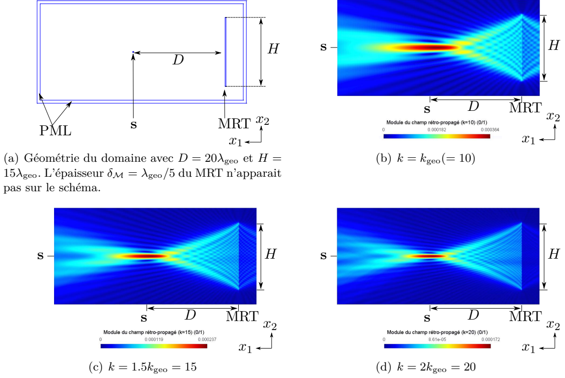
FIGURE 3.11 – Géométrie du domaine (fig. (a)) et module du champ rétro-propagé dans le milieu homogène pour k = k_{\text{geo}} (= 10) , k = 1.5k_{\text{geo}} (= 15) et k = 2k_{\text{geo}} (= 20) . Les paramètres géométriques sont les suivants : D = 20\lambda_{\text{geo}} , H = 15\lambda_{\text{geo}} et \delta_{\mathcal{M}} = \lambda_{\text{geo}}/5 (non indiqué sur les figures).
