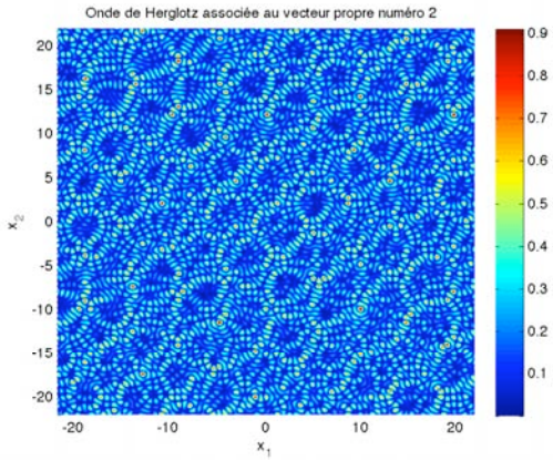
(c) Module de l'onde de Herglotz associée au deuxième vecteur propre de \mathbb{T}
