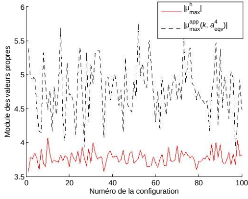
(c) Comparaison entre le module de la plus grande valeur propre (en module) et son estimation
