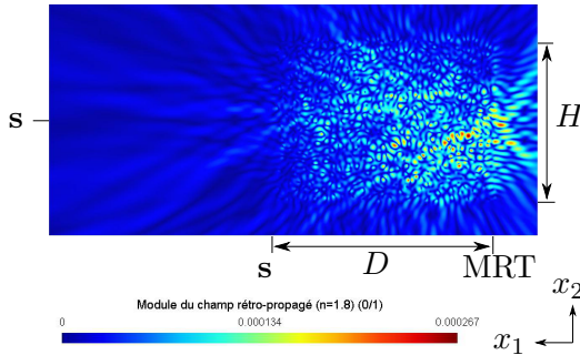
(e) n = 1.8 : module du champ rétro-propagé dans le domaine d'étude \Omega_e .
