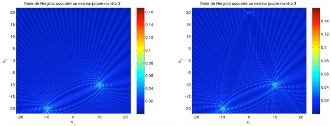
(c) Module de l'onde de Herglotz associée au deuxième vecteur propre de \mathbb{T} (d) Module de l'onde de Herglotz associée au troisième vecteur propre de \mathbb{T}
