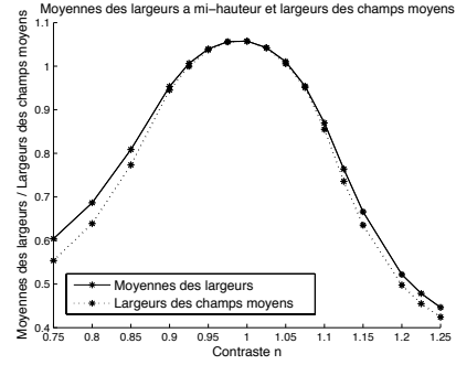
(b) Comparaison entre les largeurs à mi-hauteurs des champs moyens et la moyenne des largeurs à mi-hauteurs des champs rétro-propagés.
