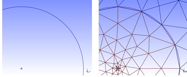
(a) Les deux cercles concentriques centrés sur \mathbf{s} . Le disque B_{\varepsilon_{\mathbf{s}}} étant situé en bas à gauche. (b) Maillage du domaine présenté sur la figure (a).
