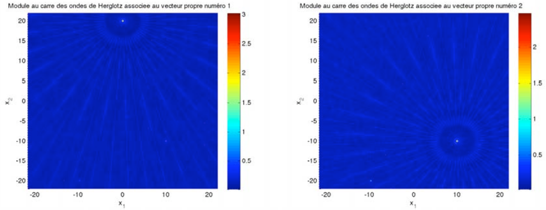
(a) Module de l'onde de Herglotz associée au premier vecteur propre de \mathbb{T} (b) Module de l'onde de Herglotz associée au deuxième vecteur propre de \mathbb{T}
