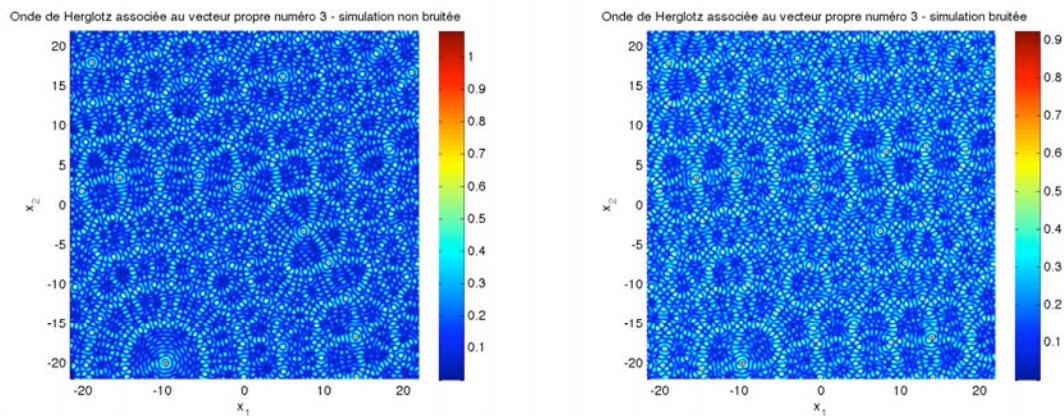
(a) Module de l'onde de Herglotz associée au troisième vecteur propre de \mathbb{T} (b) Simulation bruitée - Module de l'onde de Herglotz associée au troisième vecteur propre de \tilde{\mathbb{T}}
