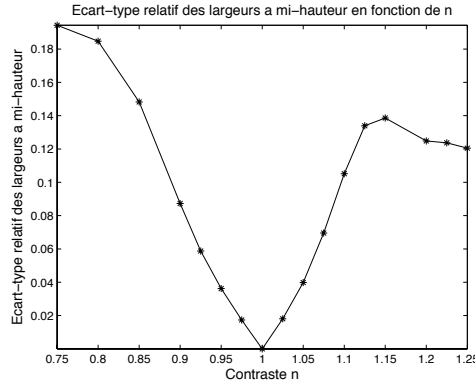
(c) Ecart-type relatif \frac{\sigma(n)}{\mu(n)} des largeurs à mi-hauteur.
