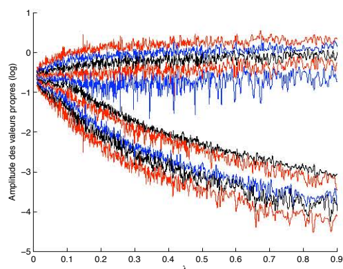
(d) Agrandissement de la figure (c) dans la zone 0 < \lambda \leq 0.9
