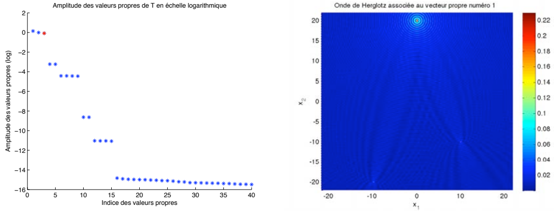
(a) Quarante plus grandes valeurs propres de \mathbb{T} (échelle logarithmique) (b) Module de l'onde de Herglotz associée au premier vecteur propre de \mathbb{T}
