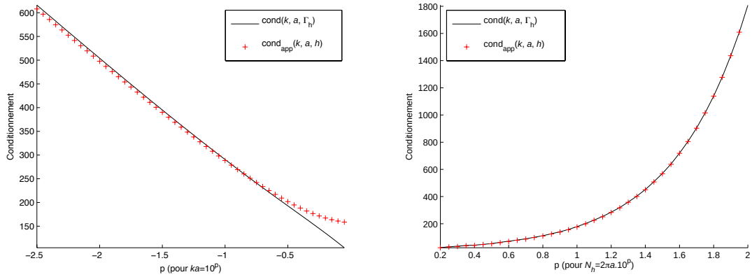
(a) Conditionnements en fonction de ka , N_h = 100 (discrétisation uniforme)
