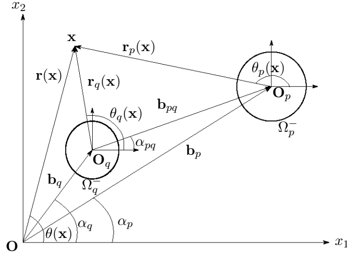
FIGURE 4.1 – Illustration des notations pour deux disques \Omega_p^- et \Omega_q^- et un point \mathbf{x} de \Omega^+ .
