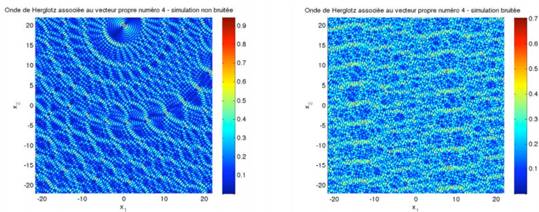
(c) Module de l'onde de Herglotz au quatrième vecteur propre de \mathbb{T} (d) Simulation bruitée - Module de l'onde de Herglotz au quatrième vecteur propre de \tilde{\mathbb{T}}
