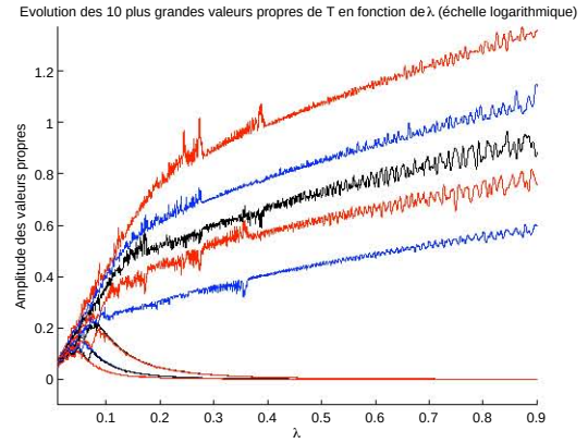
(b) Agrandissement de la figure (a) dans la zone 0 < \lambda \leq 0.9
