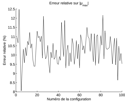
(e) Erreur relative en pourcentage, donnée par la relation (5.103), sur le module de \mu_{max}
