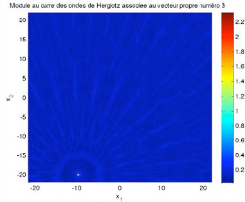
(c) Module de l'onde de Herglotz associée au troisième vecteur propre de \mathbb{T}
