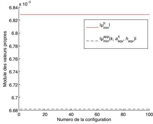
(a) Comparaison entre le module de la plus petite valeur propre (en module) et son estimation
