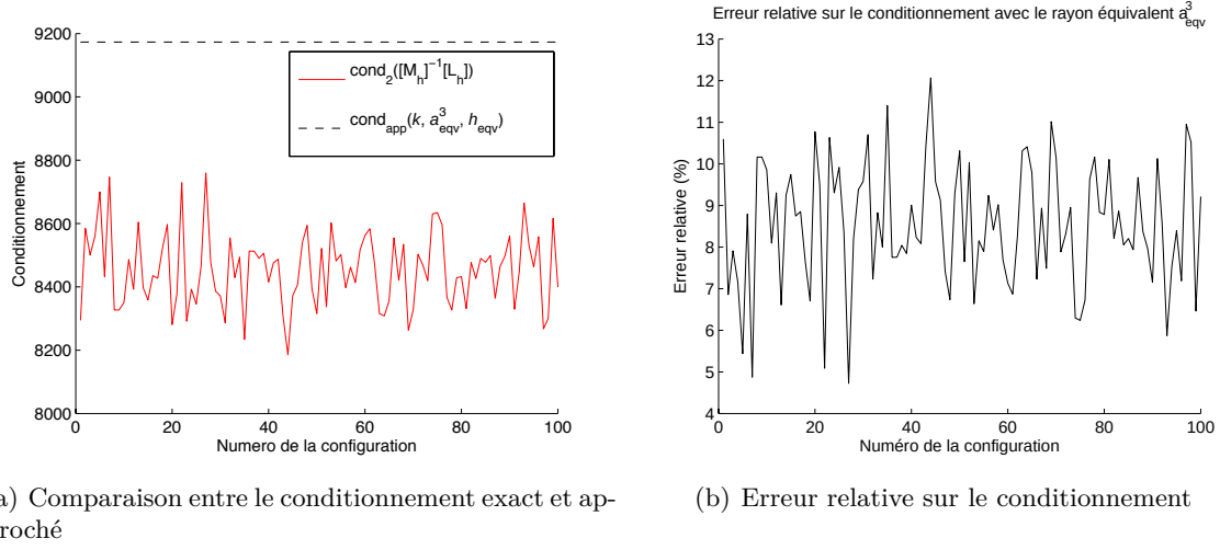
FIGURE 5.25 – Comparaison entre le conditionnement de la matrice [M_h]^{-1}[L_h] et son estimation avec le rayon équivalent a_{\text{eqv}}^3 . Les obstacles sont des petites ellipses de demi-grands axes a_{x_1} = 0.1 et a_{x_2} = 0.025 , discrétisées à l'aide de N_h = 50 segments. Pour chacune des 100 configurations différentes, nous plaçons M = 30 ellipses aléatoirement dans la boîte [0, 4] \times [0, 4] , avec k = 0.1 et b \geq 0.3 (= 3a_{x_1}) .
