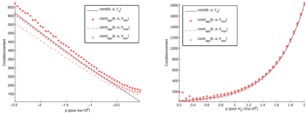
(c) Conditionnements en fonction de ka , N_h = 100 (discrétisation non uniforme)
