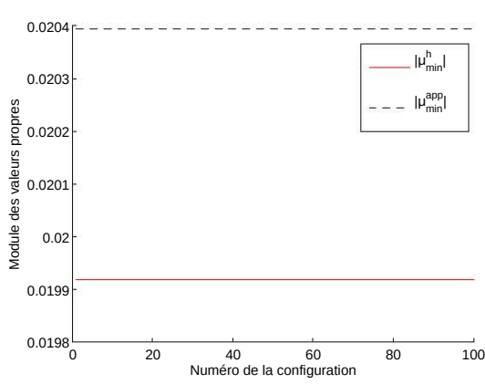
(a) Comparaison entre le module de la plus petite valeur propre (en module) et son estimation (5.69)
