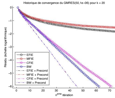
(d) Agrandissement de la figure (b)
