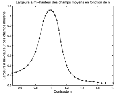
(a) Largeurs à mi-hauteur des champs moyens
