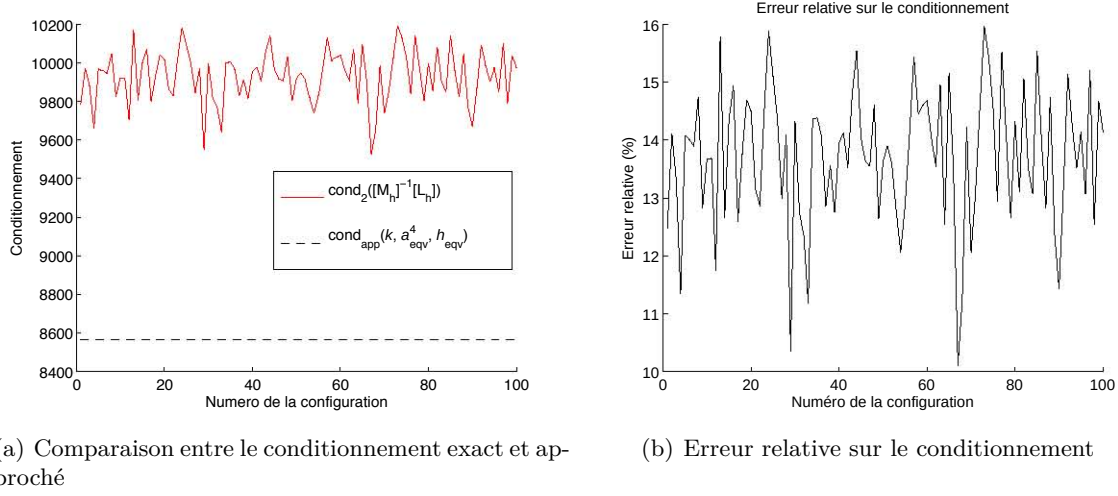
FIGURE 5.28 – Comparaison entre le conditionnement de la matrice [M_h]^{-1}[L_h] et son estimation. Les obstacles sont des petits rectangles de demi-côtés a_{x_1} = 0.1 et a_{x_2} = 0.025 , chacun étant discrétisé à l'aide de N_h = 48 segments (12 par arête). Pour chacune des 100 configurations différentes, nous plaçons M = 30 rectangles aléatoirement dans la boîte [0, 4] \times [0, 4] , avec k = 0.1 et b \geq 0.3 (= 3a_{x_1}) .
