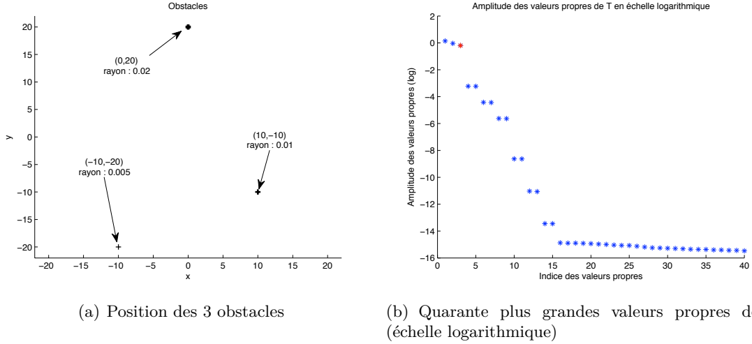
FIGURE 1.10 – Contexte dans lequel la focalisation est vérifiée
