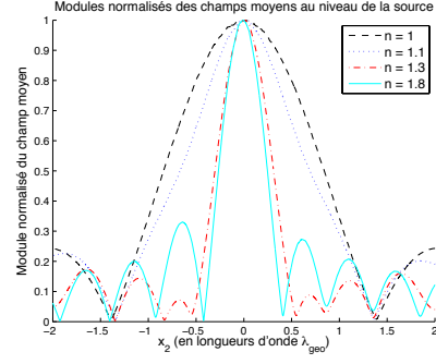
(b) Agrandissement de la figure (a).
