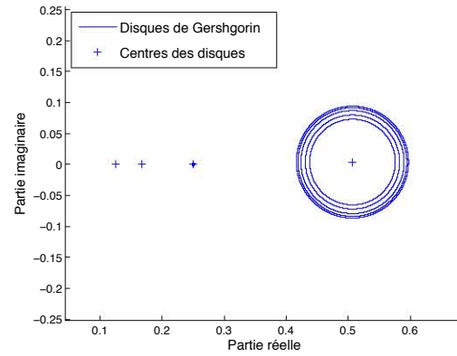
(d) kb = 7.8 (agrandissement près de l'origine)
