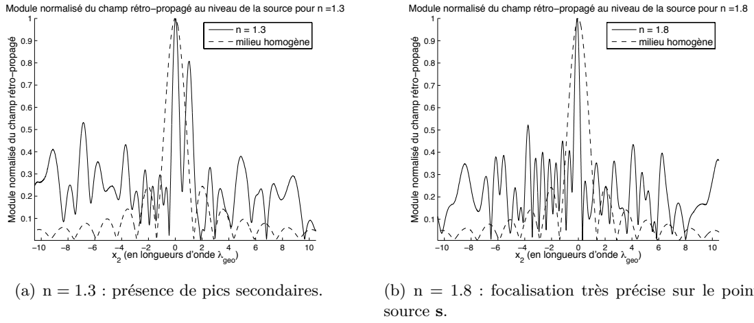
FIGURE 3.17 – Module du champ rétro-propagé au niveau de la source, normalisé par rapport à son maximum. Sur la figure (a), obtenue avec n = 1.3 , des pics secondaires d'amplitude importante apparaissent. En revanche, sur la figure (b), la focalisation est très précise, malgré le contraste élevé n = 1.8 .
