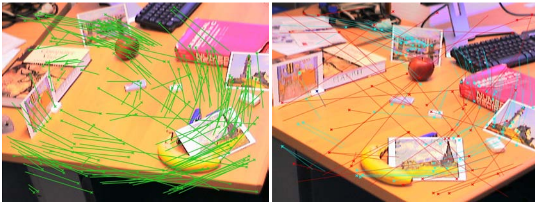
FIGURE 5.20 – Bureau, contrainte épipolaire - Mise en correspondance entre deux vues avec un fort changement de point de vue. Sur la gauche, on peut voir le mouvement apparent de 182 appariements (dont 126 sont premiers proches voisins pour la distance entre descripteurs). Sur la droite, 72 appariements avec NNT+F. Le seuil du rapport pour NNT est ici fixé à 0.8 (seulement 34 appariements sont obtenus avec un rapport de 0.6). Bien que quelques appariements incorrects soient visibles sur la gauche (à cause de points proches par hasard de leur droite épipolaire correspondante), la distribution des points est plus dense que sur l'image de droite, ce qui permet habituellement une estimation plus précise de la structure et du mouvement de la caméra.
