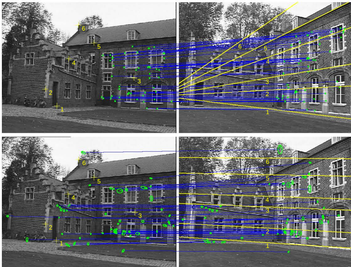
FIGURE 6.7 – Château de Leuven : deux images distantes de la séquence de M. Pollefeys. Haut : ASIFT. 94 appariements, dont seulement quelques-uns sont sur une façade différente. Bas : I-ASIFT+F. 118 appariements (24% ne sont pas plus proches voisins), distribués sur la totalité du bâtiment. Excepté 2, tous les autres sont corrects. La matrice fondamentale est alors estimée sur l'ensemble d'appariements obtenus. Les droites épipolaires (en jaune dans l'image de droite) correspondant à quelques points saisis à la main (dans l'image de gauche) prouve que I-ASIFT permet d'estimer le mouvement de la caméra de façon fiable. Les points associés aux points choisis à la main sont en effet à moins de 1 pixel de leur droite épipolaire correspondante. Au contraire, le mouvement de la caméra n'est pas restitué correctement à partir d'ASIFT. Remarquons que M_{SER} donne 5 appariements, et les détecteurs Harris/Hessien Affine donnent 20-30 appariements principalement entre motifs répétés incorrectement associés. (code d'extraction de featurespace.org )
