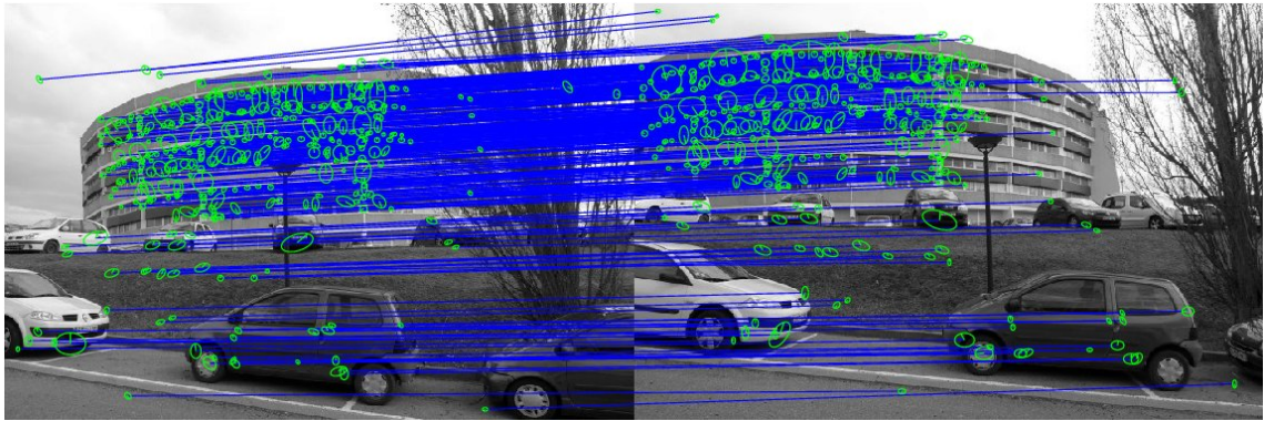
FIGURE 6.9 – Bâtiment du second-cycle : I-ASIFT permet ici de couvrir la scène d'appariements sur une grande profondeur. Il faut noter cependant que quelques points sont incorrectement mis en correspondance, en particulier ceux sur l'arbre à droite et ceux dans le ciel. Cela s'explique car ceux-ci sont cohérents avec une homographie locale, ainsi qu'avec le mouvement global donné par la géométrie épipolaire.
