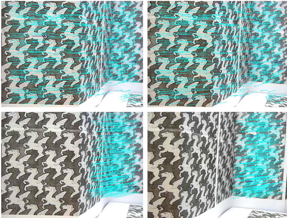
FIGURE 5.5 – pegase , homographie - En haut, faible mouvement de translation. En bas, mouvement de translation plus important. Pour une faible translation, l'homographie est approximée par une rotation équivalente, et permet d'obtenir un appariement fiable sur toute l'image. Pour une translation plus grande, l'homographie retrouvée permet la mise en correspondance des points qui sont situés sur le plan avec le plus grand support.
