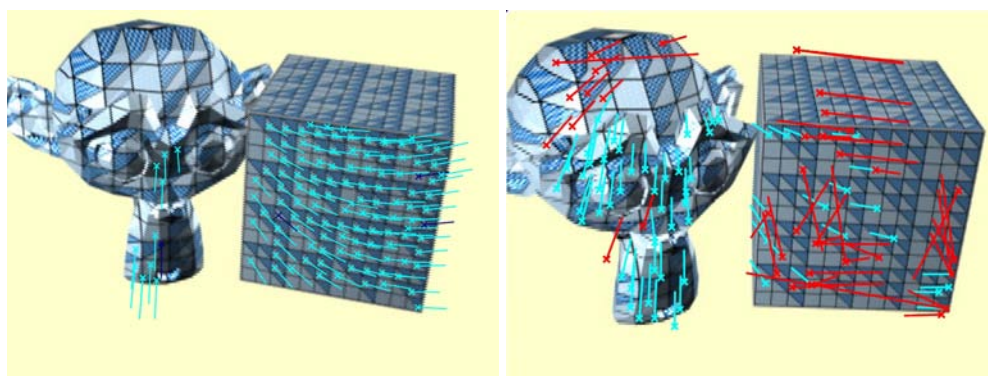
FIGURE 5.12 – Monkey , contrainte homographique. Deux images avec des motifs répétés. Sur la gauche, le modèle ACM proposé, la plupart des motifs sur le plan dominant sont détectés (les segments représentent le mouvement apparent entre les deux vues). Sur la droite, la seconde image avec les appariements obtenus avec NNT (les deux couleurs) et NNT+H (les inliers sont en bleu, les outliers en rouge). Beaucoup d’autres appariements sont obtenus avec l’algorithme ACM.
