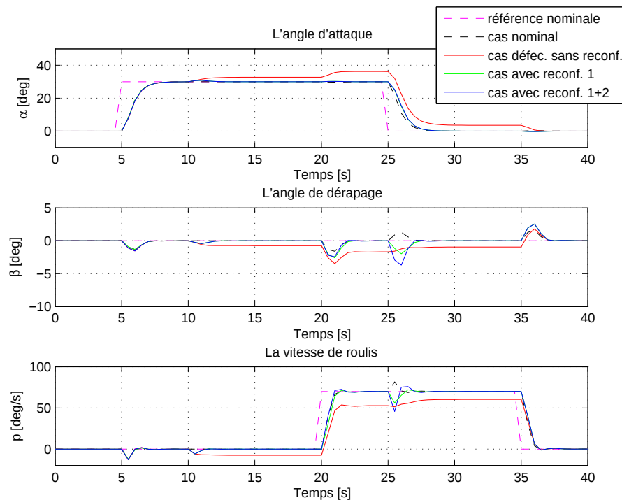
FIGURE 4.36 – Défaut actionneur 3 ( \gamma_3 = 0.5 ) : les sorties.
