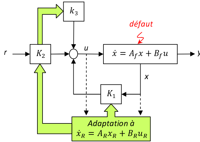
FIGURE 1.10 – Principe de la méthode AMF
