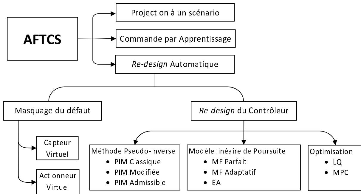
FIGURE 1.3 – Classification des approches utilisées en AFTC
