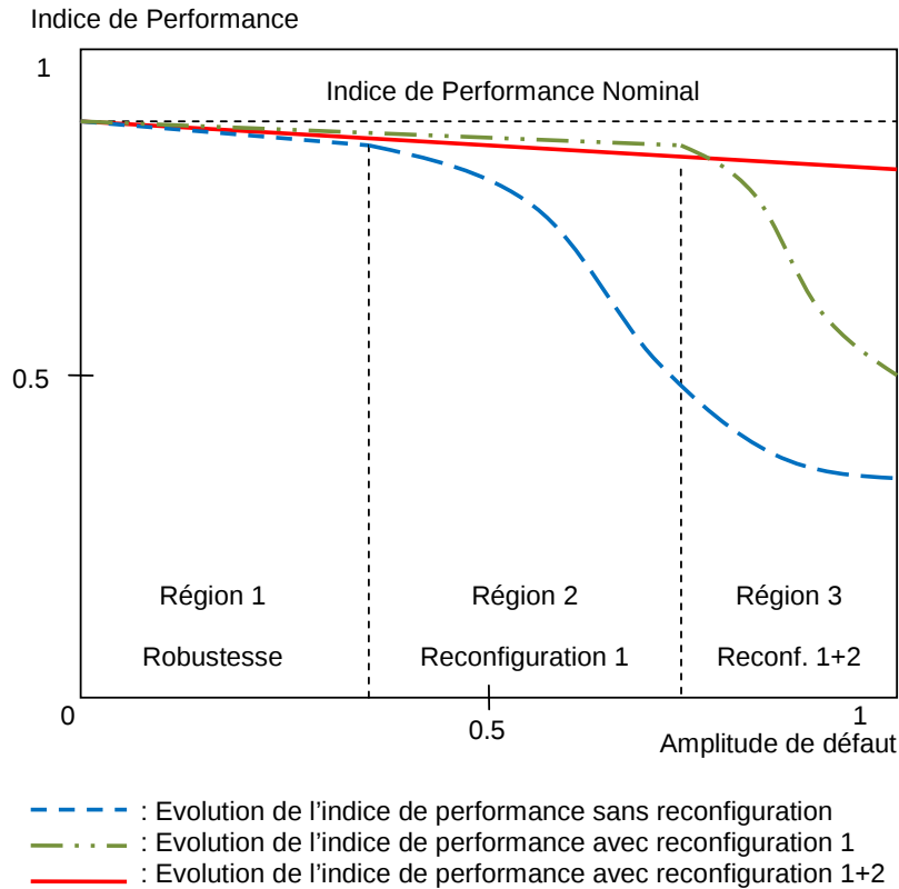
FIGURE 4.1 – Principe de dégradation de performance en fonction de sévérité du défaut
