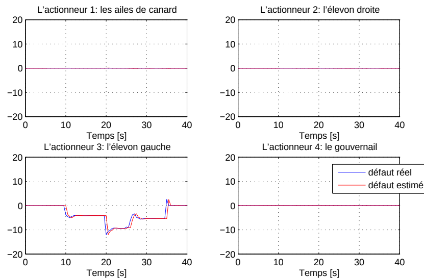
FIGURE 4.38 – Défaut actionneur 3 ( \gamma_3 = 0.5 ) : estimation du défaut \hat{f}_3 .
