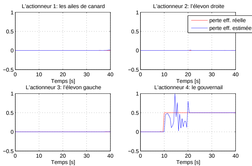
FIGURE 4.52 – Défaut actionneur 4 ( \gamma_4 = 0.5 ) : estimation de perte \hat{\gamma}_4 .
