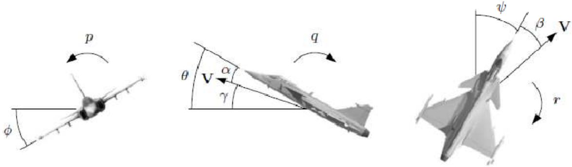
FIGURE 4.1 – Les angles d'orientation d'aéronef \phi , \theta et \psi , les angles aérodynamiques \alpha et \beta , et les vitesses angulaires p , q et r .
