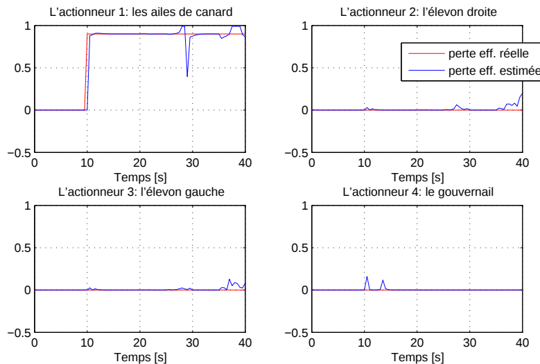
FIGURE 4.18 – Défaut actionneur 1 ( \gamma_1 = 0.9 ) : estimation de perte \hat{\gamma}_1 .
