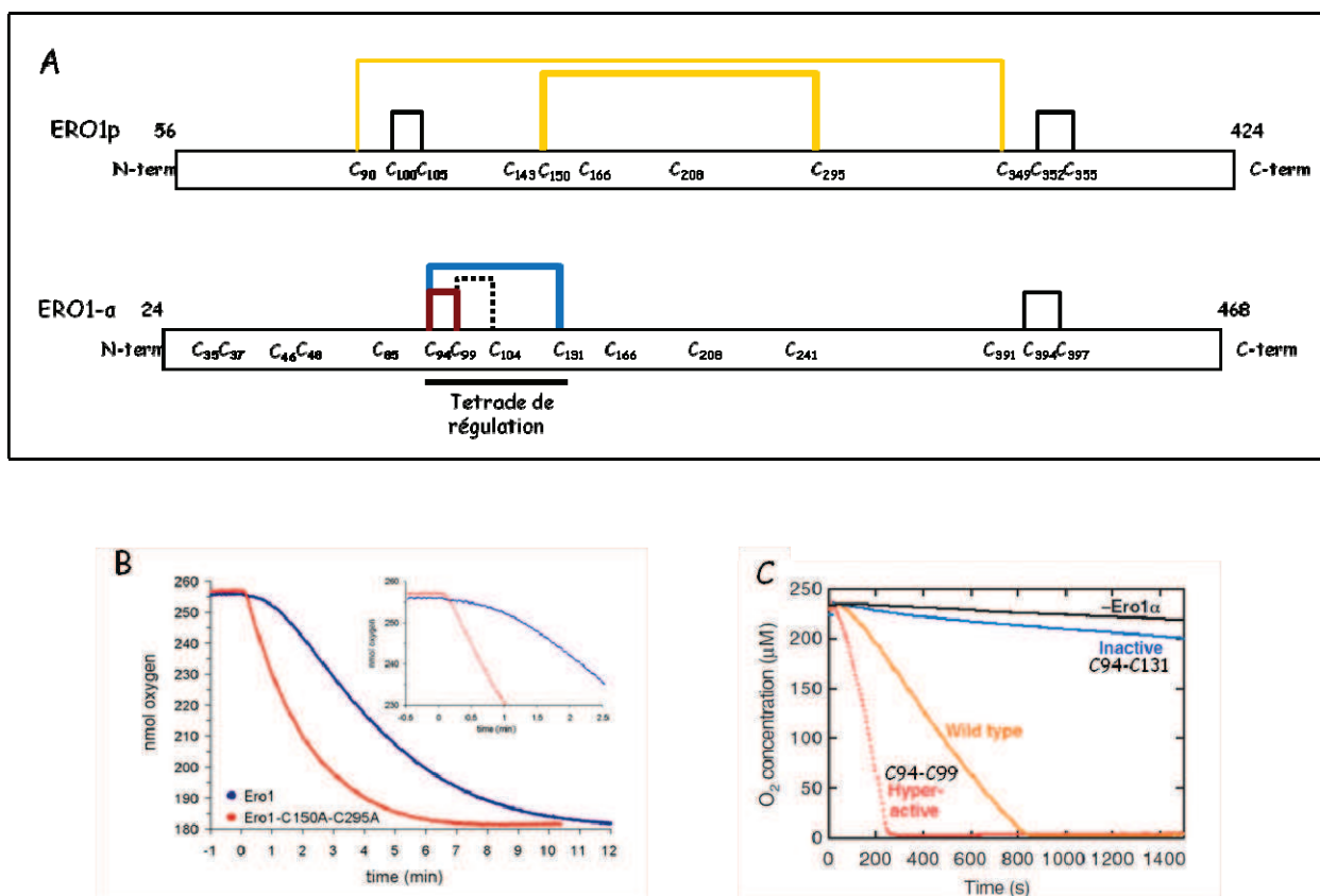
Figure 44. Rôles des cystéines régulatrices des protéines ERO1.
