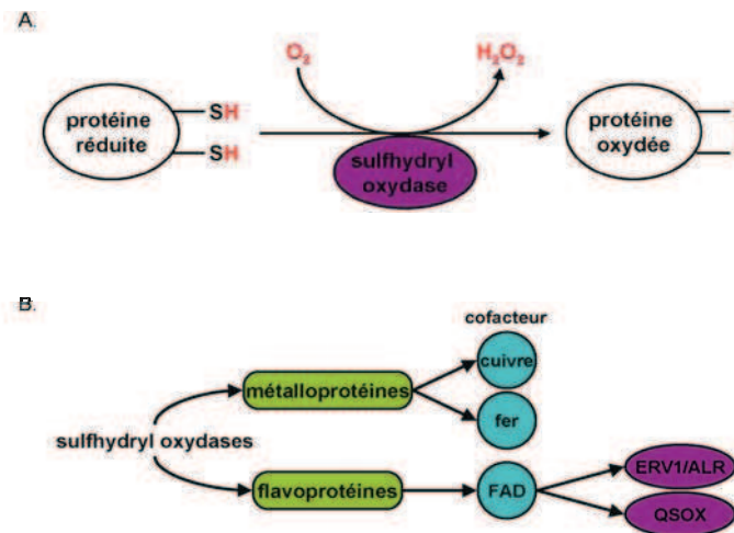
Figure 35. Les sulfhydryl oxydases.
