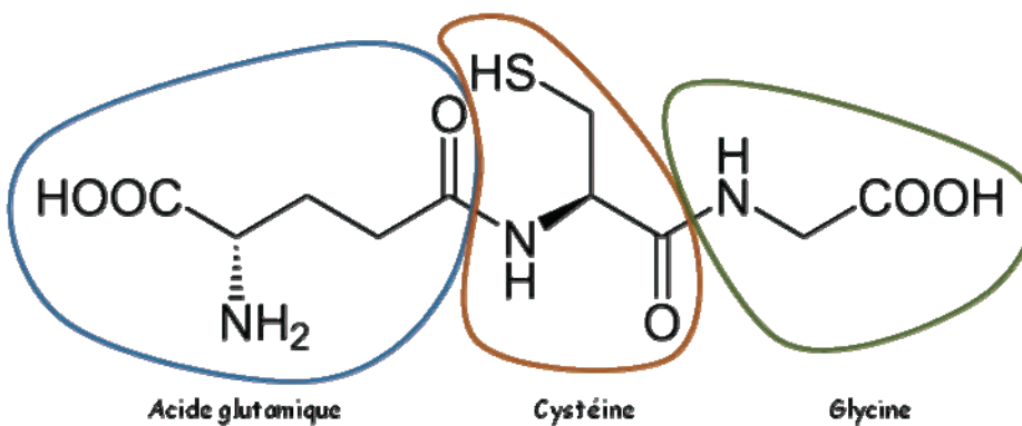
Figure 21. Structure chimique du tripeptide γ-L-glutamyl-L-cystéinyglycine.
