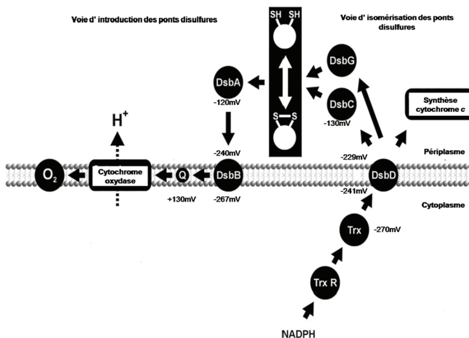
Figure 32. Trajet des électrons lors des voies d'introduction (partie gauche) et d'isomérisation (partie droite) des ponts disulfure dans le périplasmique des bactéries.
