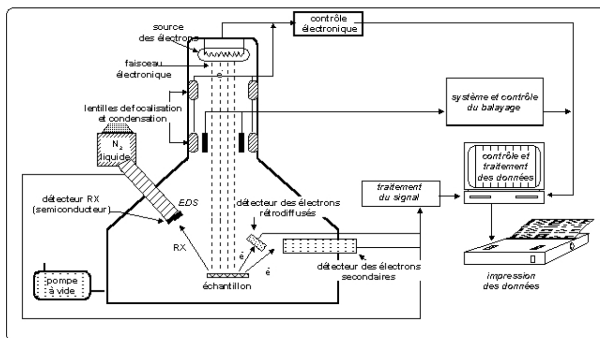
Figure a.2. : fonctionnement du MEB ( http://www.lrmh.fr/lrmh/images/meb_schema.jpg )
