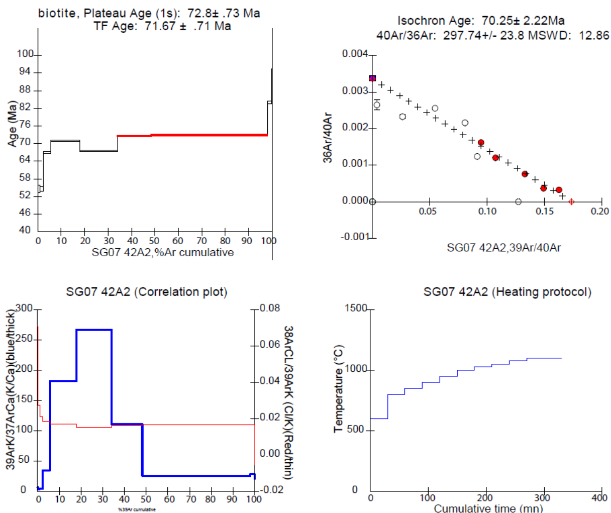
Figure 4.60 : Résultats des analyses de la population de biotites de l'échantillon SG 07 42A2.
