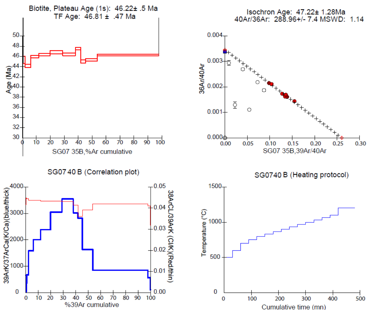
Figure 4.57 : Résultats des analyses de la population de biotites de l'échantillon SG 07 40 B.
