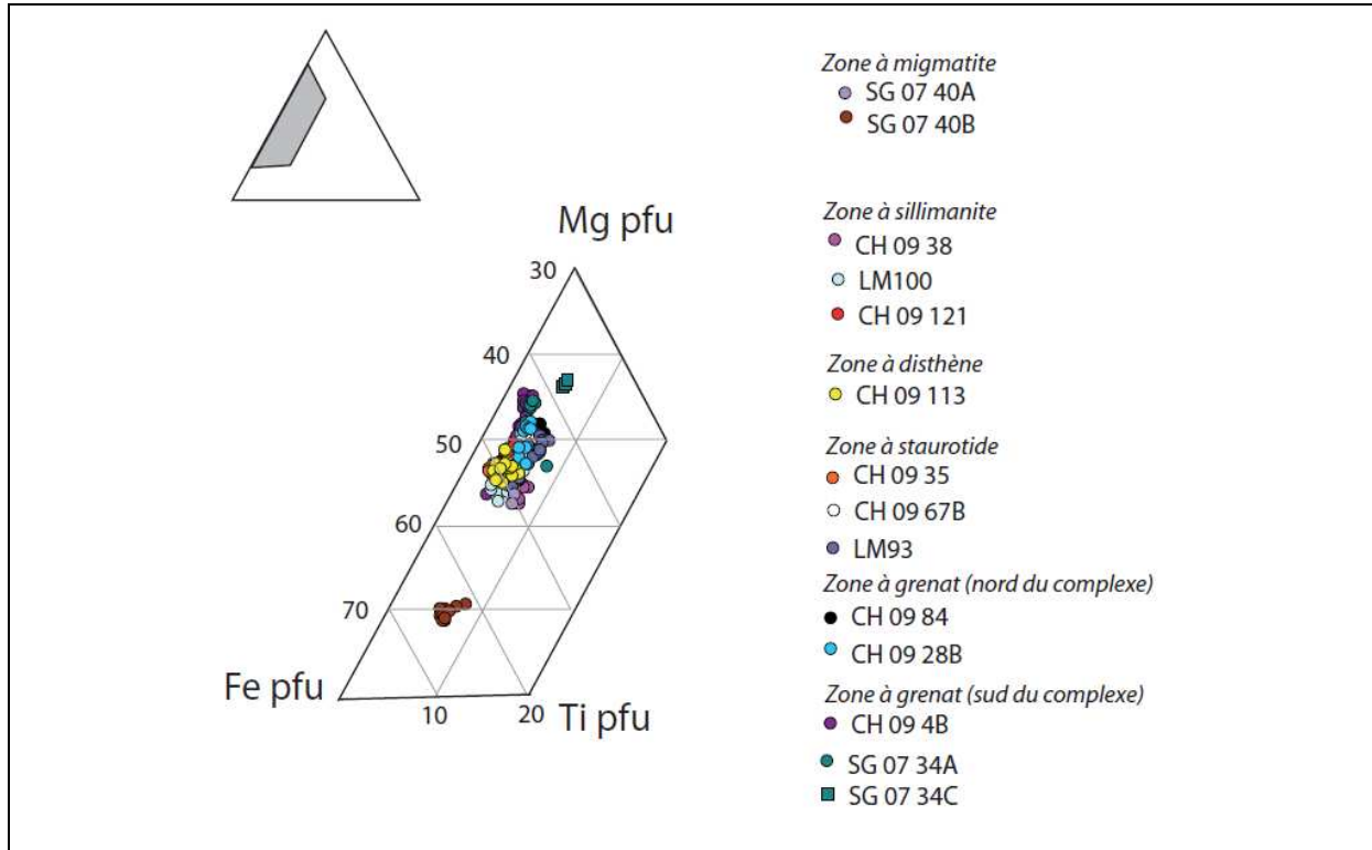
Figure 4.32 : Diagramme triangulaire montrant la composition en Fe, Mg et Ti des biotites des roches métamorphiques des différentes zones du complexe métamorphique de Danba. Les symboles ronds représentent des métasédiments et les symboles carrés représentent des metabasites.
