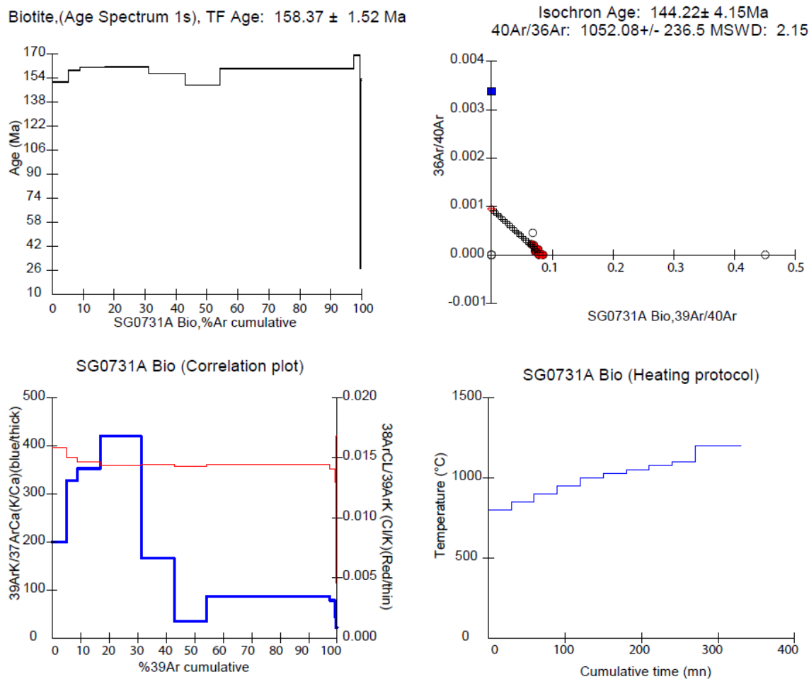
Figure 4.53 : Résultats des analyses de la population de biotites de l'échantillon SG 07 31A.
