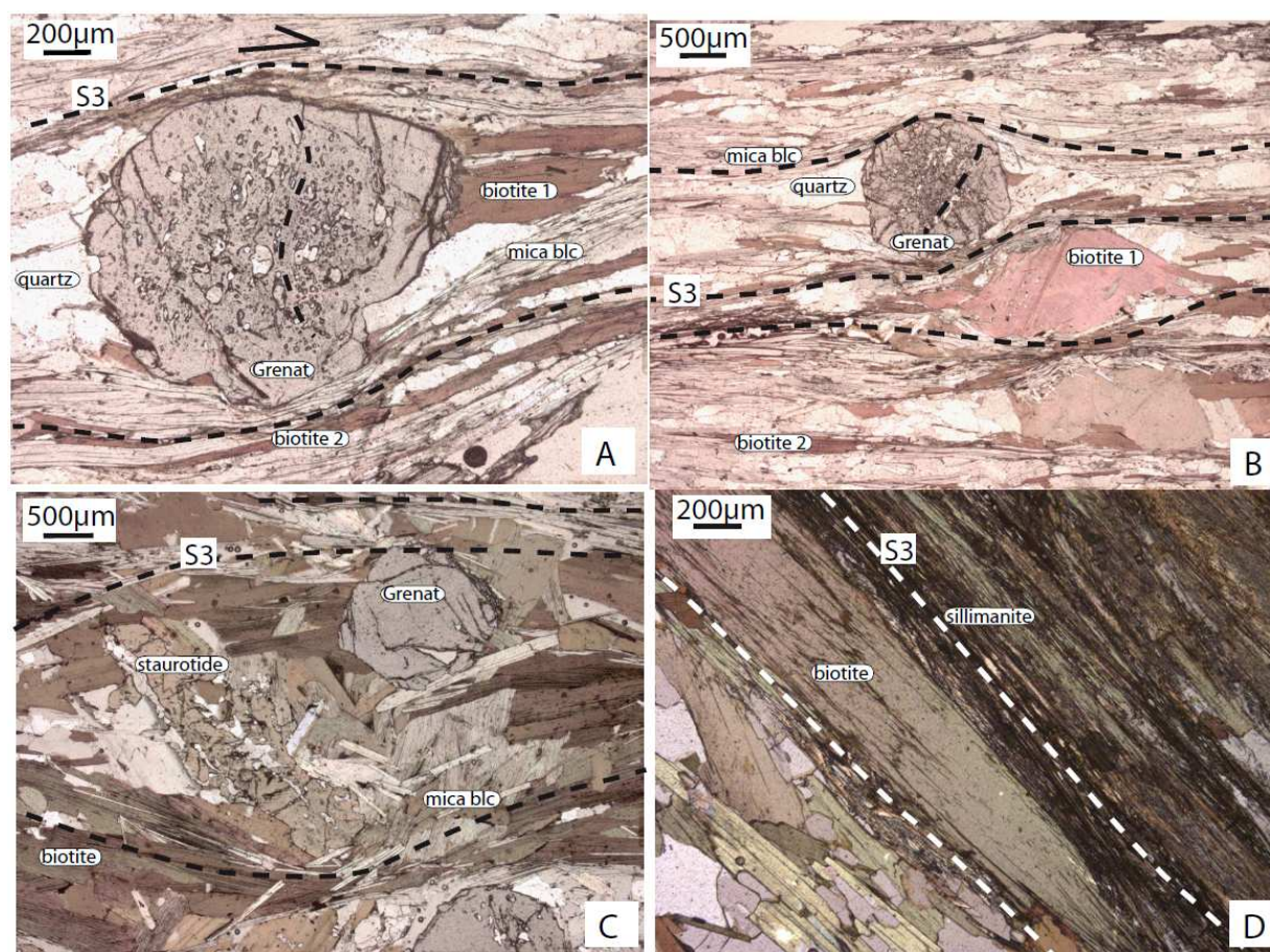
Figure 4.21 : Relations entre la S3 et les minéraux du métamorphisme. A) grenat avec schistosité interne hélicitique, moulé dans la S3 soulignée par des néoblastes de mica blanc (mica blc) et de biotite recrystallisés (biotite 2) (échantillon CH 09 84, S3=N20, 60W). B) Porphyroblaste de grenat moulé dans la S3 et porphyroclaste de biotite sigmoïde moulé dans la S3, soulignée par des néoblastes de mica blanc (mica blc) et de biotite (biotite 2) (échantillon CH 09 84, S3=N20, 60W). C) Porphyroclastes de staurotide et de grenat moulés dans la S3 portée par des néoblastes de biotite et de mica blanc (CH 09 67B, S3=N120, 55N). D) biotite et sillimanite soulignant la S3 (échantillon SG 07 40A, S3=N28, 75E).
