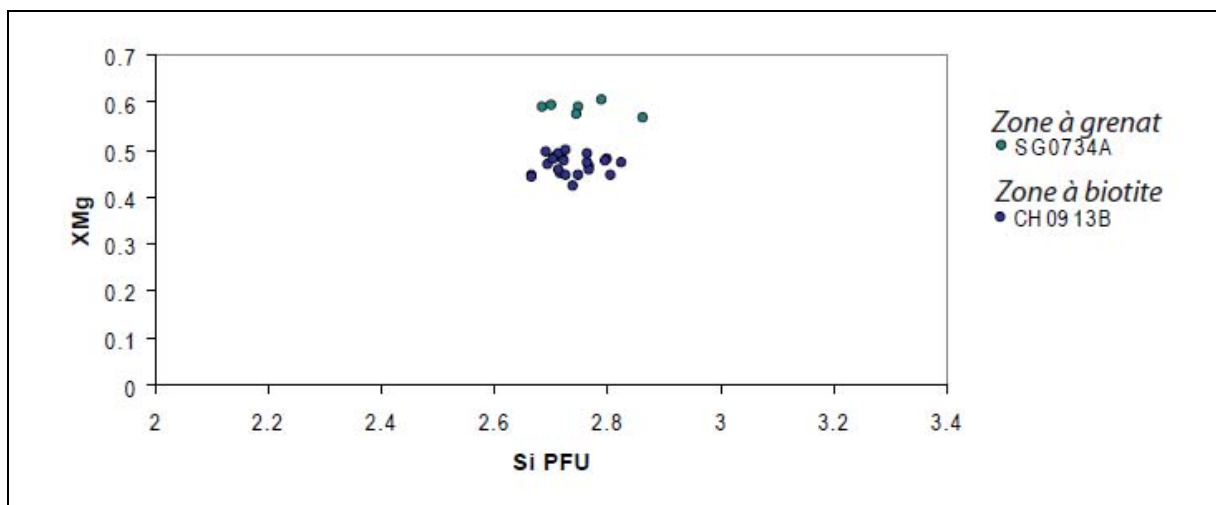
Figure 4.35 : Diagramme X_{Mg} versus Si pfu pour les chlorites des métasédiments de la couverture du massif de Gezong, dans la partie Sud du complexe métamorphique de Danba.
