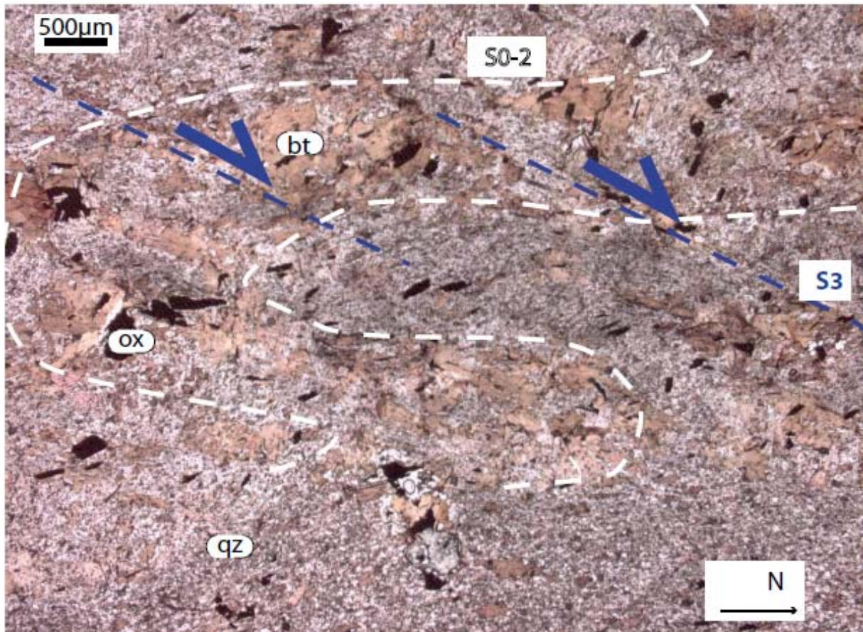
Figure 4.7: Microphotographie de l'échantillon CH 09 32 (figure 4.3) montrant la relation entre la foliation composite S_0-1/2 et la schistosité S_3 , qui correspond à des bandes de cisaillement du haut vers le nord sur la bordure nord-est du complexe métamorphique de Danba. Les pointillés blancs soulignent la foliation S_0-1/2 et les pointillés bleus soulignent la schistosité S_3 . A noter que la biotite apparaît à la fois en clastes repris par S_3 et en néoblastes syncinématiques soulignant S_4 . bt=biotite, ox=oxyde, qz=quartz.
