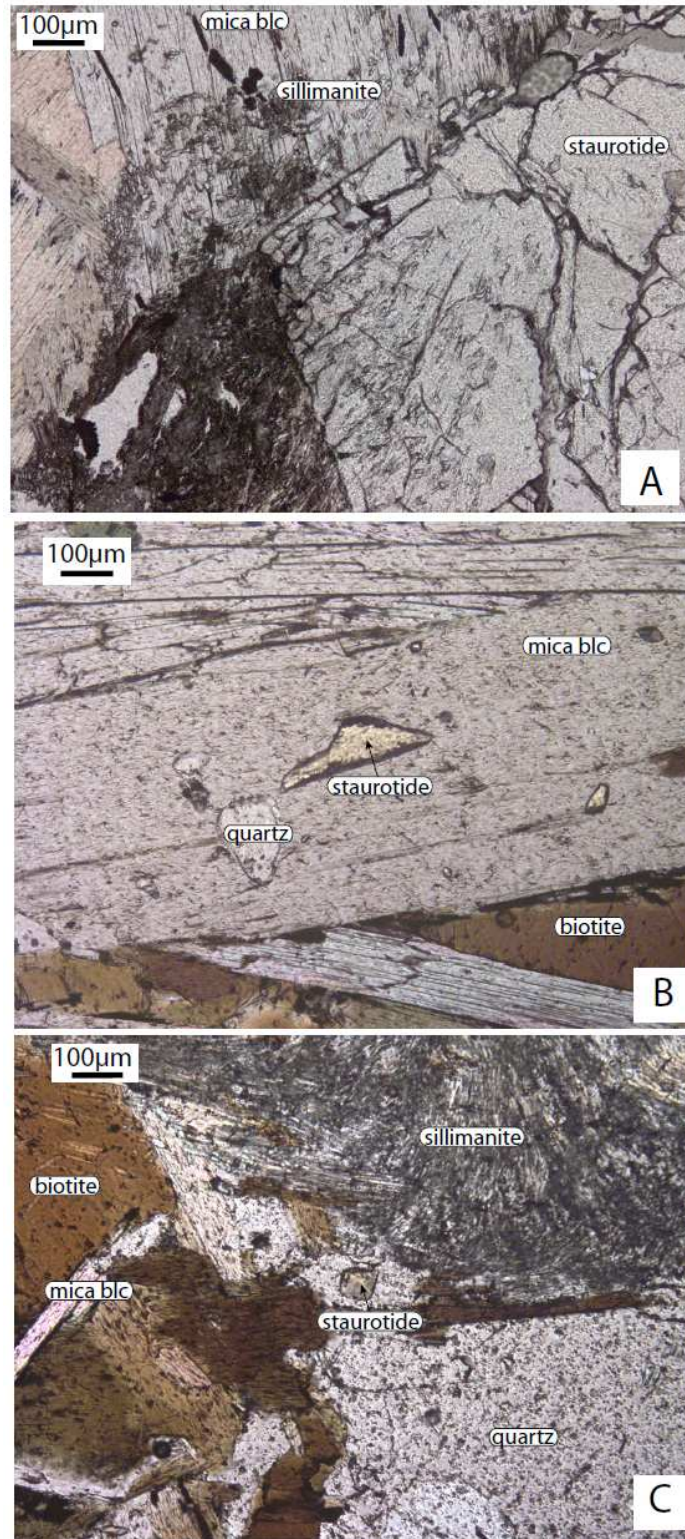
Figure 4.38 : Microphotographies montrant les relations texturales entre les minéraux dans les échantillons CH 09 121 et CH 09 38. A) Sillimanite se développant à partir d'un cristal de staurotite (échantillon CH 09 121). B) Relique de staurotite incluse dans un mica blanc (échantillon CH 09 38). C) relique de staurotite associée à des cristaux de biotite, mica blanc et sillimanite (échantillon CH 09 38).
