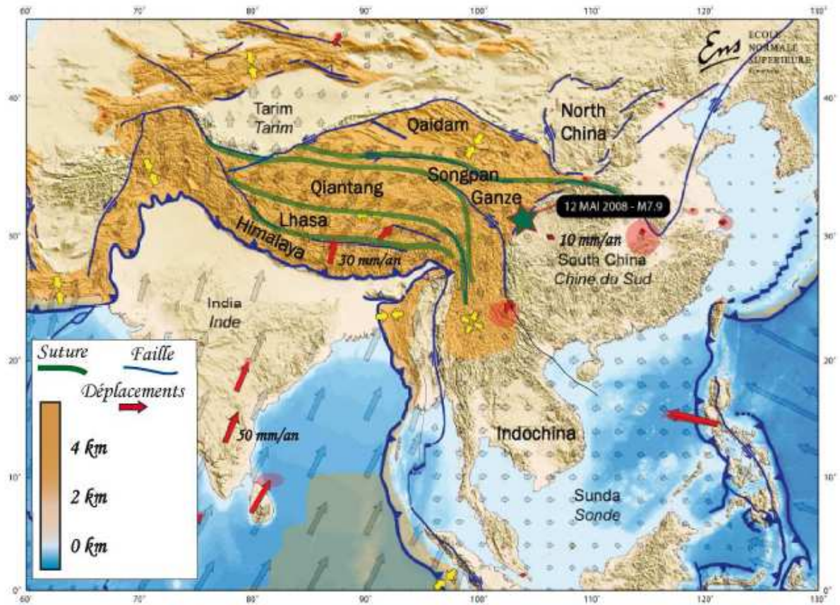
Figure 1.1: Contexte géodynamique actuel du plateau Tibétain. Les parties de hautes altitudes sont représentées en marron. Plusieurs sutures océaniques délimitent les anciens terrains qui se sont accrétés à l'Asie au cours du Mésozoïque et du Cénozoïque (Yin et Harrison 2000). Il y a environ 50 Ma, le craton Indien est venu poinçonner l'Asie, ce qui a provoqué la surrection du plateau (Yin et Harrison 2000, Molnar et Tapponier 1975). Les vitesses de déplacements mesurées actuellement sont de plus en plus faibles vers le Nord-est (Chen et al. 2000). En mai 2009 s'est produit dans la chaîne bordière Est du plateau du Tibet (la chaîne des Longmen Shan) un séisme de magnitude 7.9 dont l'épicentre est marqué par une étoile verte.
