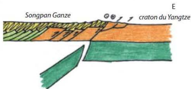
Figure 6.5 : Schémas de l'évolution de la lithosphère de l'unité lithotectonique du Songpan Ganze durant le Paléozoïque supérieur et le Trias.
