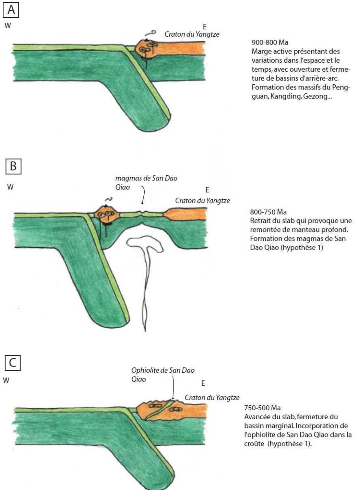
Figure 6.3: Schémas de l'évolution de la marge active de la bordure Ouest du craton du Yangtze durant le Néoprotérozoïque, considérant la genèse des magmas de San Dao Qiao au Néoprotérozoïque.
