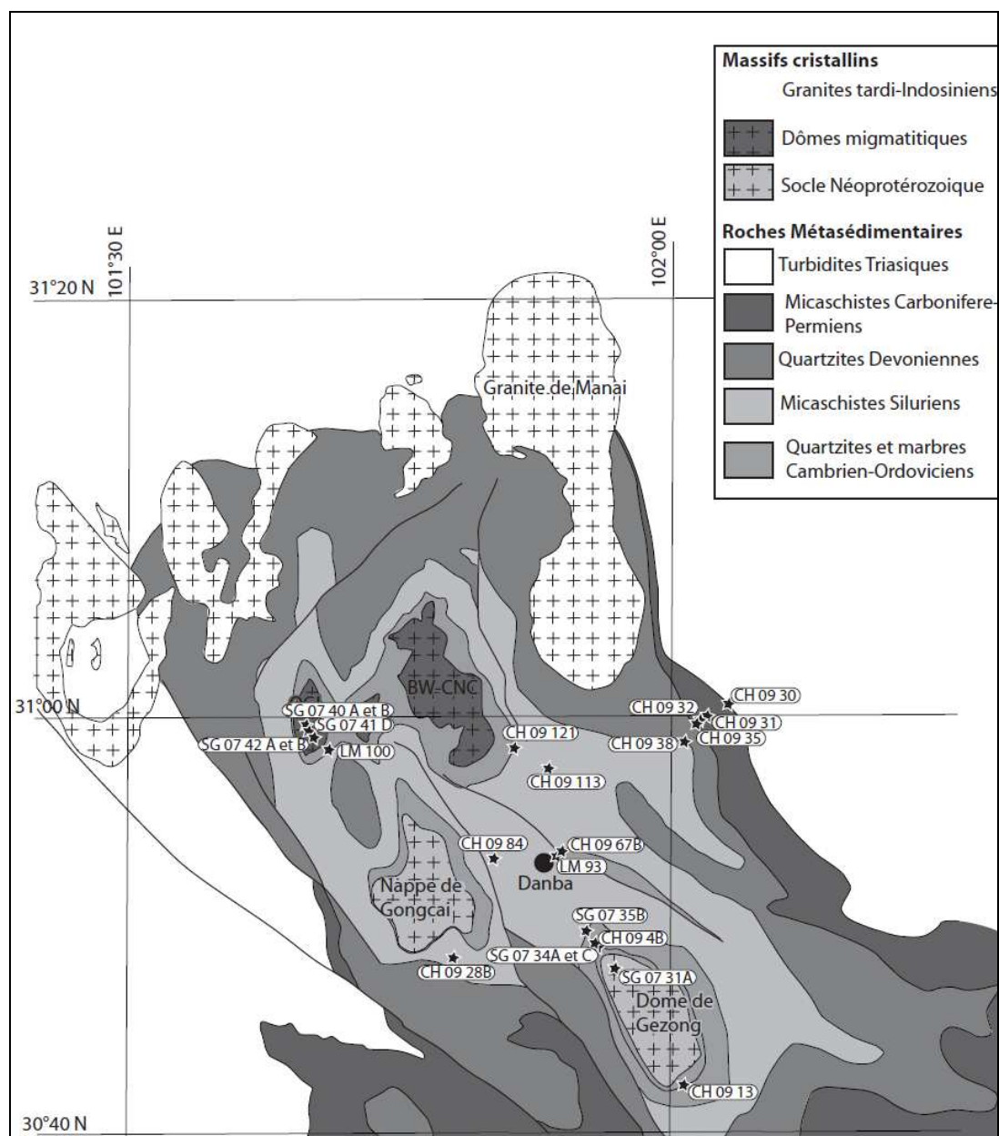
Figure 4.3 : Carte de localisation des échantillons cités.
