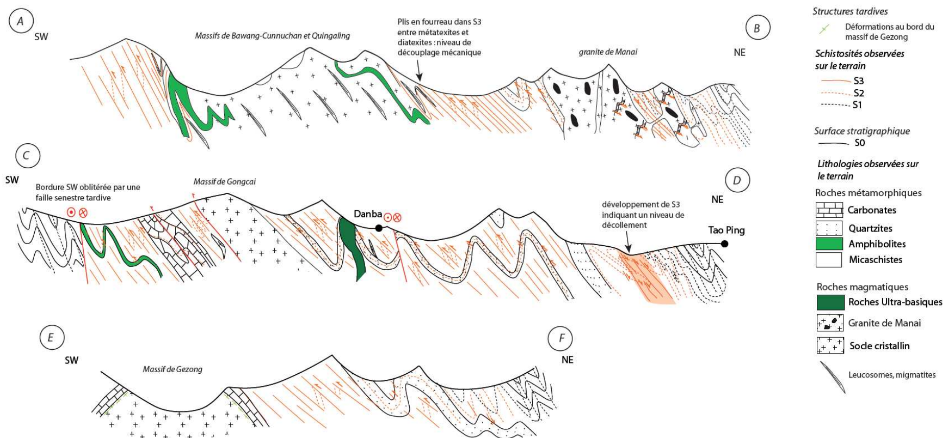
Figure 4.4 : Trois coupes NE-SW dans le complexe métamorphique de Danba montrant les principales structures et leurs relations (figure 4.2). AB : coupe au niveau des massifs migmatitiques ; CD : coupe au niveau de la nappe déversée de Gongcai ; EF : coupe au niveau du massif de Gezong. La schistosité S3 marque la bordure du complexe métamorphique. Le développement de cette schistosité correspond à un niveau de décollement entre les métasédiments turbiditiques et ceux du cœur du complexe. Au NE, la S3 correspond à des cisaillements du haut vers le nord-est. Au SW et au cœur du complexe métamorphique, la S3 correspond à des cisaillements du haut vers le sud-ouest. Les critères cinématiques tels que l'obliquité de la S3 par rapport à la S0-1/2 préservée dans les lithologies compétentes, et le déversement des plis P3 indiquent un mouvement général du haut vers le sud-ouest. AB=50Km
