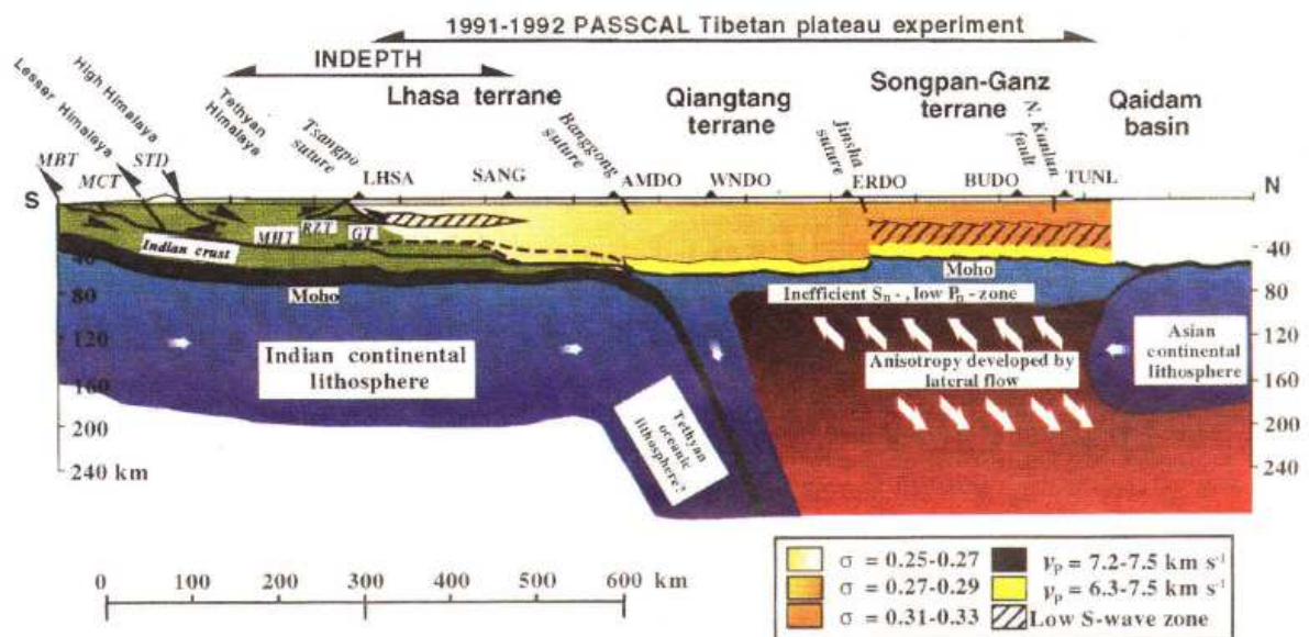
Figure 6.7 : Extrait d'Owens et Zandt, 1997. La croûte d'affinité Indienne est représentée en vert. Les diverses teintes de orange représentent les variations du rapport de Poisson ( \sigma ) dans la croûte tibétaine. Les parties coloriées en noir en base de croûte correspondent à des zones où les vitesses d'ondes P sont très élevées. Les parties coloriées en jaune en base de croûte correspondent à des zones où les vitesses d'ondes P sont comprises entre 6.3 et 7.5 km/s. Les parties hachurées représentent des zones de faible vitesse d'ondes S. Sous le Moho, les parties bleues représentent la lithosphère et les parties rouges représentent des zones où les données suggèrent que le manteau présente des vitesses d'ondes sismiques plus faibles qu'au Sud du plateau, en particulier au niveau de l'unité du Songpan Ganze.
