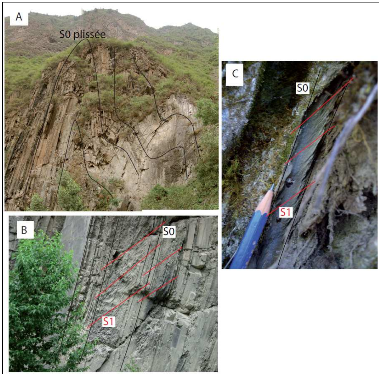
Figure 4.5 : Relation macroscopique entre la stratigraphie et la schistosité S1 de plan axial dans les turbidites Triasiques de l'unité lithotectonique du Songpan Ganze. A) La stratigraphie plissée (en noir), déformation typique de l'unité du Songpan Ganze ; B) et C) Relation entre la stratigraphie (en noir) et la schistosité S1 de plan axial (en rouge) à deux échelles différentes.
