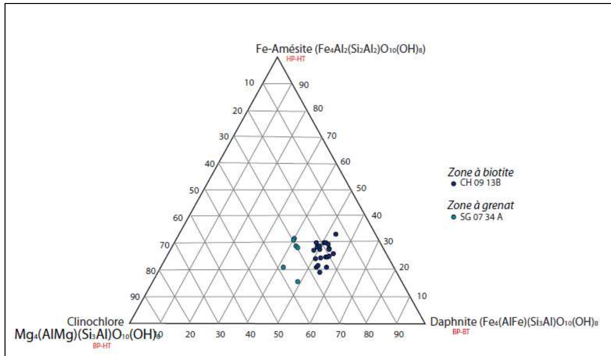
Figure 4.36 : Diagramme amésite-clinocllore-daphnite montrant la composition des cristaux de chlorite des métasédiments de la couverture du dôme de Gezong, au Sud du complexe métamorphique de Danba.
