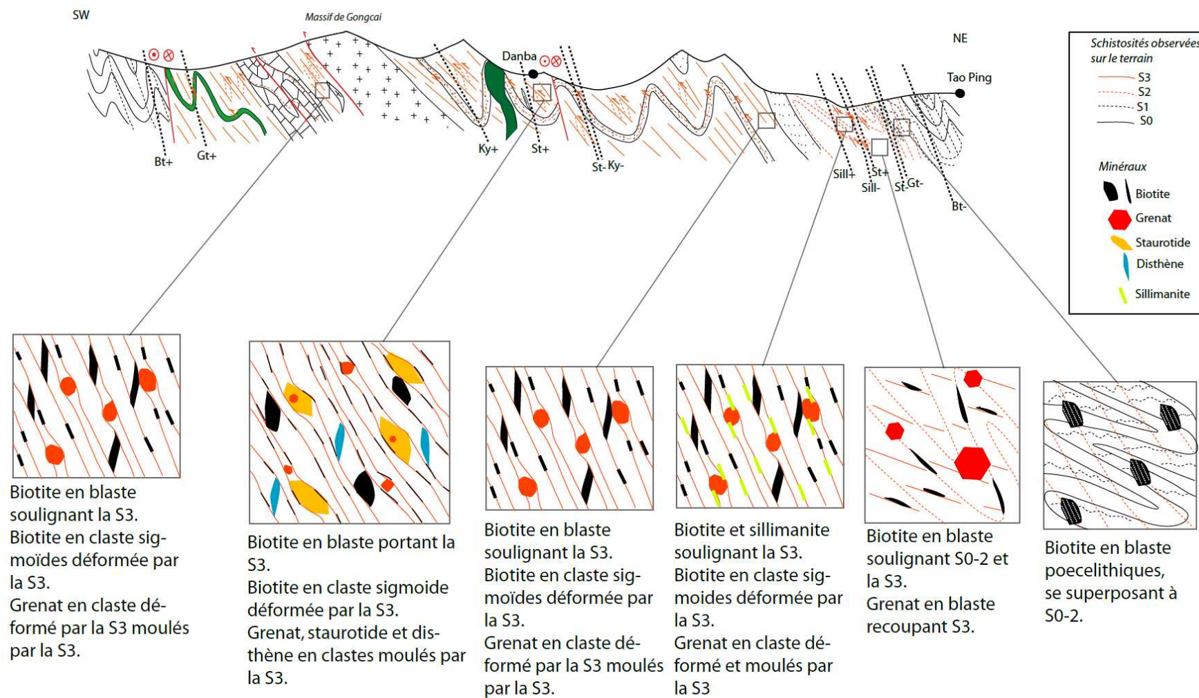
Figure 4.22 : Coupe NE-SW passant par Danba (coupe CD de la figure 4.2) et montrant les relations entre schistosités et minéraux marqueurs du métamorphisme dans le complexe métamorphique de Danba, ainsi que la position des isogrades (la présence et l'absence des minéraux le long de la coupe est décrite d'ouest en est).
