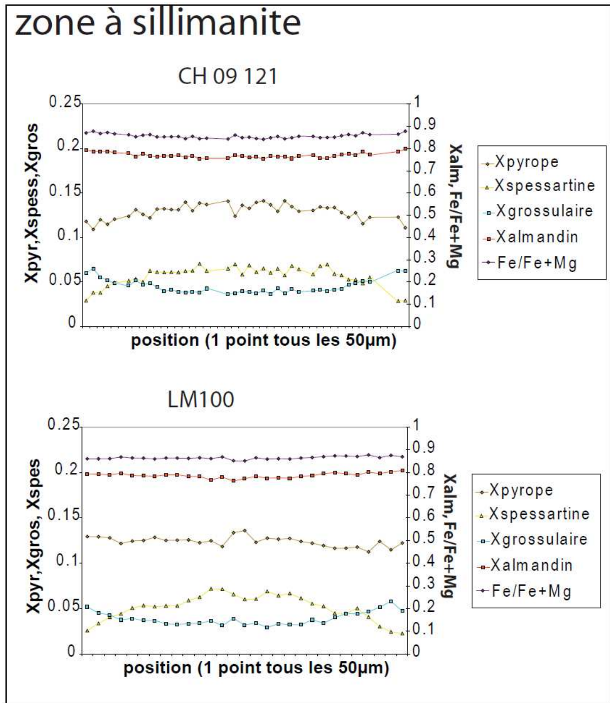
Figure 4.30 : Profils de composition de grenats issus d'échantillons représentatifs de la zone à sillimanite (CH 09 121 et LM 100, figure 4.3 pour localisation, figure 4.29 B et C pour aspect des grenats)
