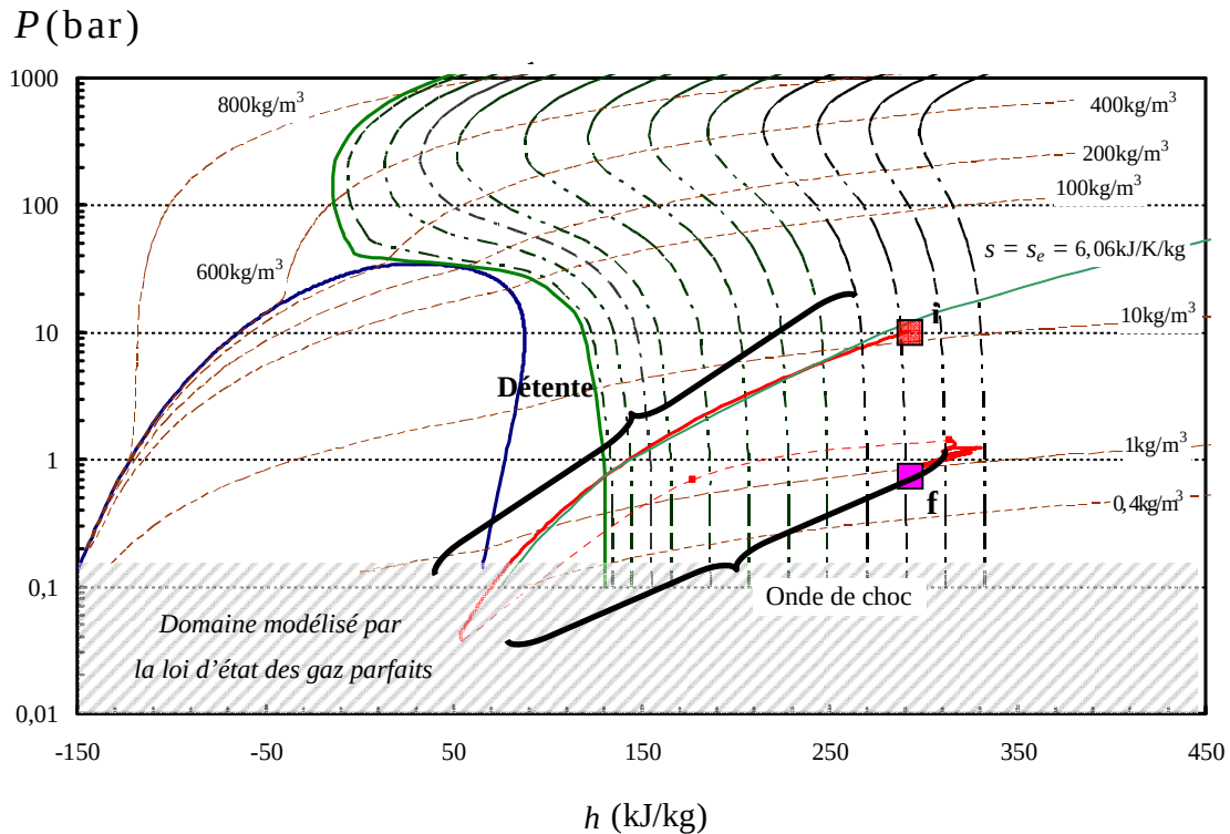
Figure 4.24 : Chemin thermodynamique suivi sur l'axe du jet dans le jet fortement sous détendu de fluide réel à NPR=10 ; i: état initial du fluide sur la section de sortie du jet, f: état final du fluide sur l'axe du jet à une distance x/D_e=250 ; Courbes de saturation liquide et gazeuse (—) ; isothermes de 130K à 350K par pas de 20K de gauche à droite (---) ; isotherme critique (—) ; isentrope S=6,06 \text{ J.kg}^{-1}.\text{K}^{-1} (—) ; courbes de masse volumique constante (---).
