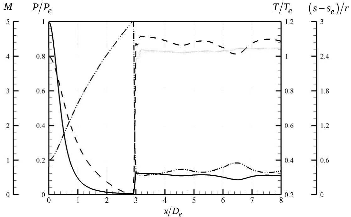
Figure 4.21 : Variations de la pression statique P/P_e (—), du nombre de Mach M (---), de la température T/T_e (---) et de l'entropie (S-S_e)/r (—) en fonction de la position x/D_e sur l'axe du jet obtenus pour le cas test de jet fortement sous détendu de fluide réel à NPR=10 .
