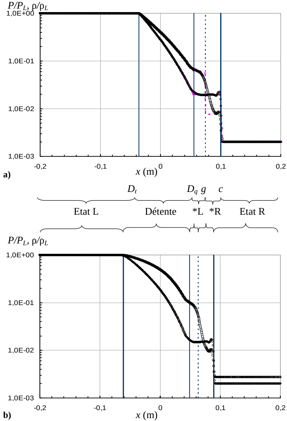
Figure 4.12 : Courbes représentant les rapports P/P_L ( \diamond ) et \rho/\rho_L ( \square ) à t=0.1 ms pour : a) le gaz parfait, b) le fluide réel. Distinction des différents états dans le tube à choc (voir légende de la Figure 4.5).
