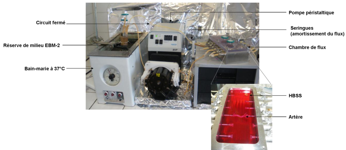
Figure 39 : Photographie de l'ensemble des éléments constitutifs du circuit permettant de soumettre les artères au cisaillement.
