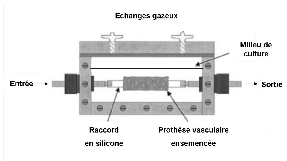
Figure 38 : Schéma de la chambre d'écoulement.
