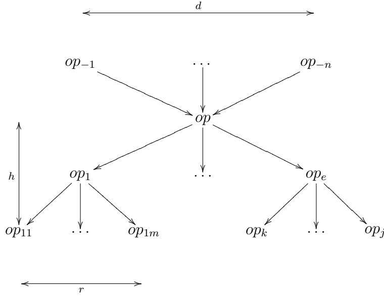
FIGURE 5.5 – Dépendances pour l'opération op .
