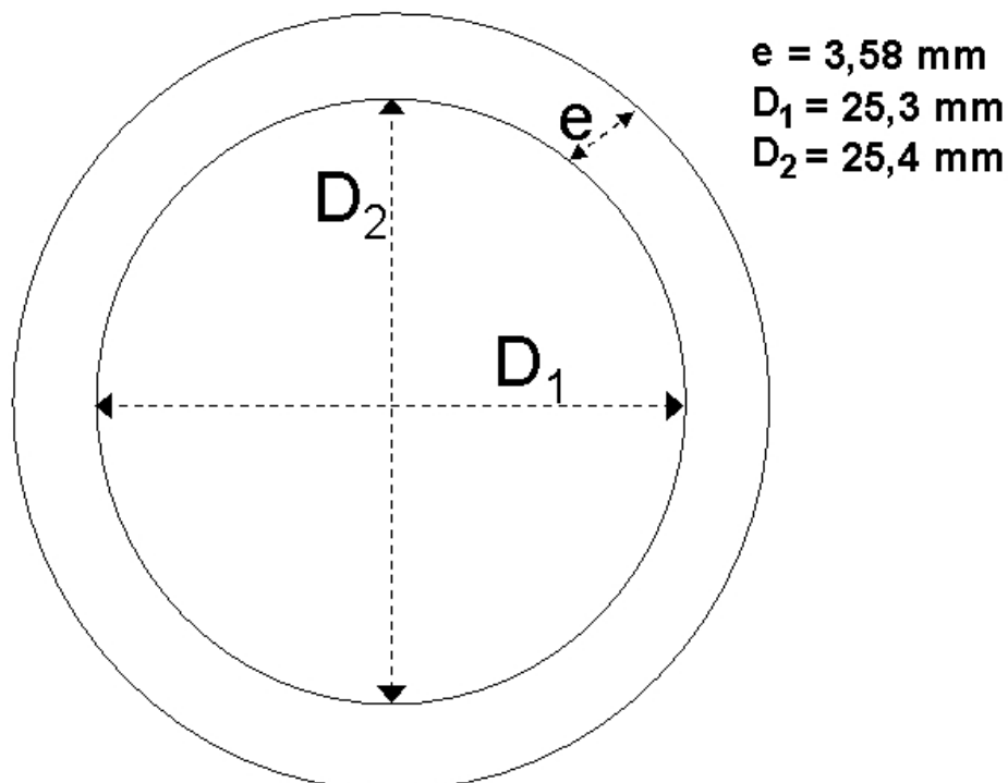
FIG. 4.29 – Introduction d'un défaut de circularité de 0,1 mm dans une bague de serrage d'épaisseur moyenne
