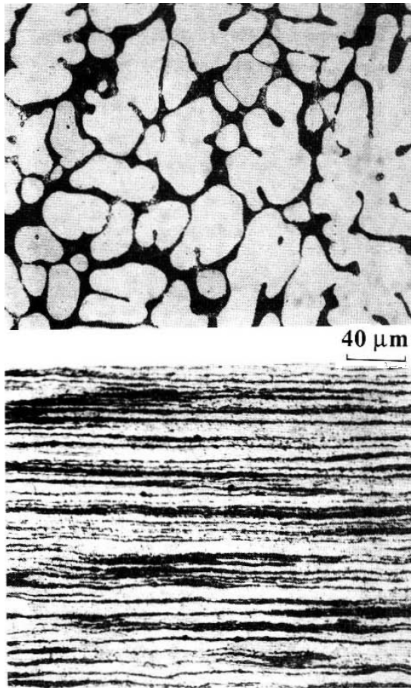
FIG. 2.10 – Structure du \text{Ni}_{47}\text{Ti}_{44}\text{Nb}_9 juste après la coulée (a) et après une déformation à chaud (b) (Melton et al. 1989)
