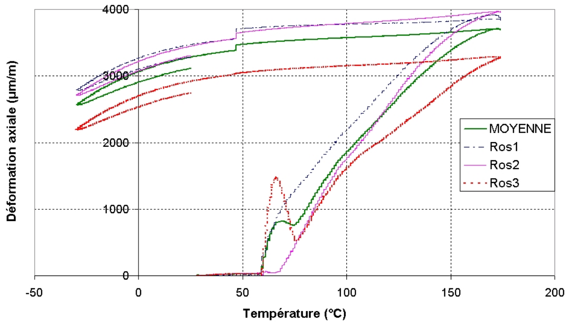
FIG. A.14 – Évolution des déformations axiales relevées sur les rosettes de la bague épaisse lors du cycle A2
