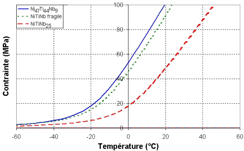
FIG. 5.3 – Augmentation de la température A_s par prédéformation - Comparaison entre le \text{Ni}_{47}\text{Ti}_{44}\text{Nb}_9 et deux composites avec la même matrice, le premier avec 10 % d'inclusions fragiles et le second avec 25 % d'inclusions de comportement analogue à celui du \text{Ni}_{47}\text{Ti}_{44}\text{Nb}_9
