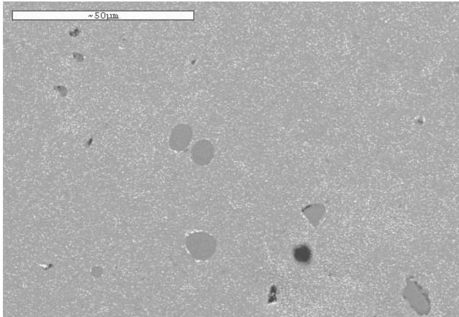
FIG. 2.5 – Micrographie du \text{Ni}_{47}\text{Ti}_{44}\text{Nb}_9 dans le sens transverse - Échelle 50 \mu\text{m} .
