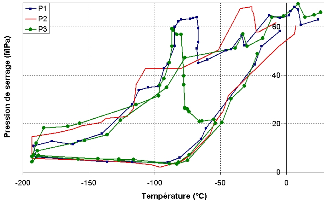
FIG. 4.15 – Évolution de la pression de serrage dans la bague moyenne lors de la trempe dans l'azote liquide
