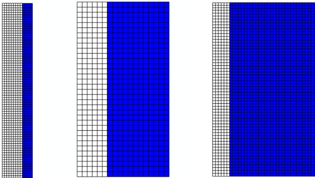
FIG. 4.17 – Maillage des trois configurations simulées avec une bague en NiTiNb fine, moyenne et épaisse - Éléments de longueur respective 0,22, 0,3 et 0,3 mm
