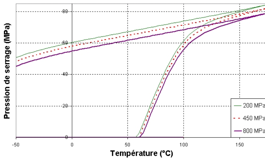
FIG. 3.16 – Influence de l'écroutissage des inclusions sur la pression de serrage - H_{iso} = 200 ; 450 et 800 MPa
