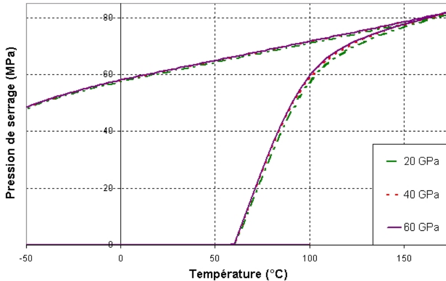
FIG. 3.14 – Influence du paramètre H_{twin} sur la pression de serrage - H_{twin} = 20 ; 40 et 60 GPa
