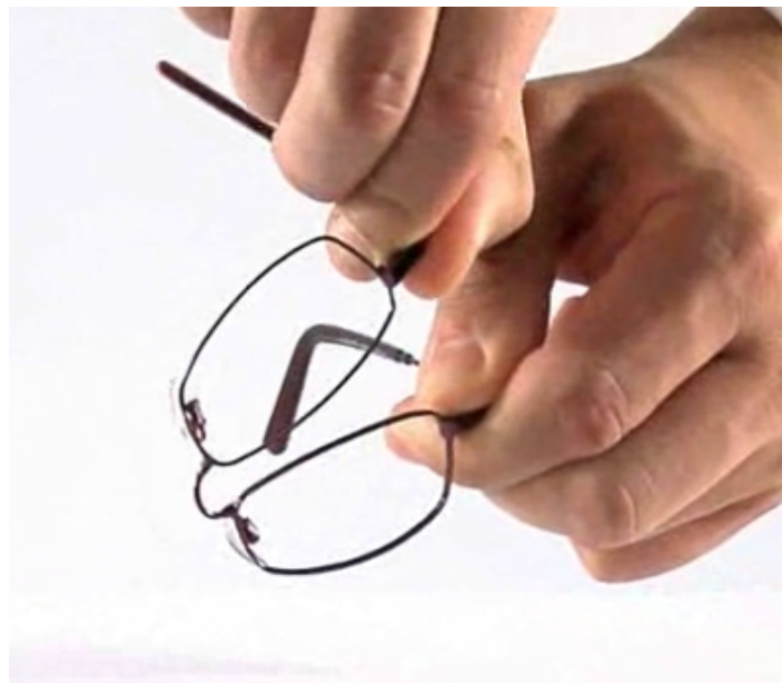
FIG. 1.5 – Exemple d'utilisation de la propriété superélastique des AMF dans l'habillement - Monture de lunettes superélastique (Aspex)
