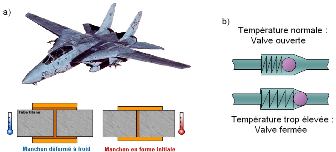
FIG. 1.7 – Exemples d'utilisation de la propriété mémoire de forme des AMF - a) Bague de serrage (Kauffman et Mayo 1996) ; b) Valve de sécurité
