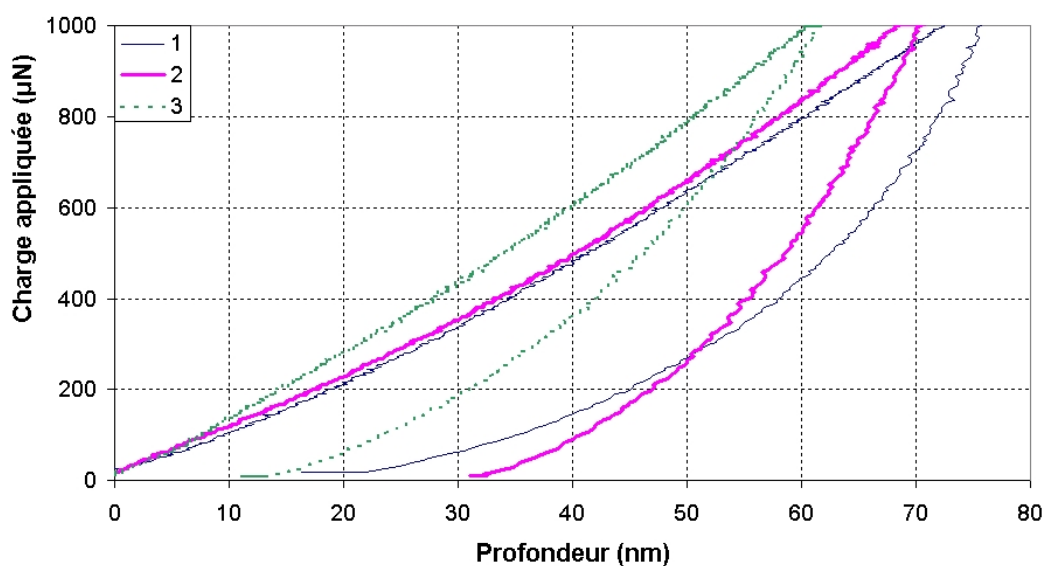
FIG. A.1 – Résultats de nanoindentation sur des échantillons de \text{Ni}_{47}\text{Ti}_{44}\text{Nb}_9 avec une charge appliquée de 1000\ \mu\text{N} et une vitesse de 65\ \mu\text{N/s}
