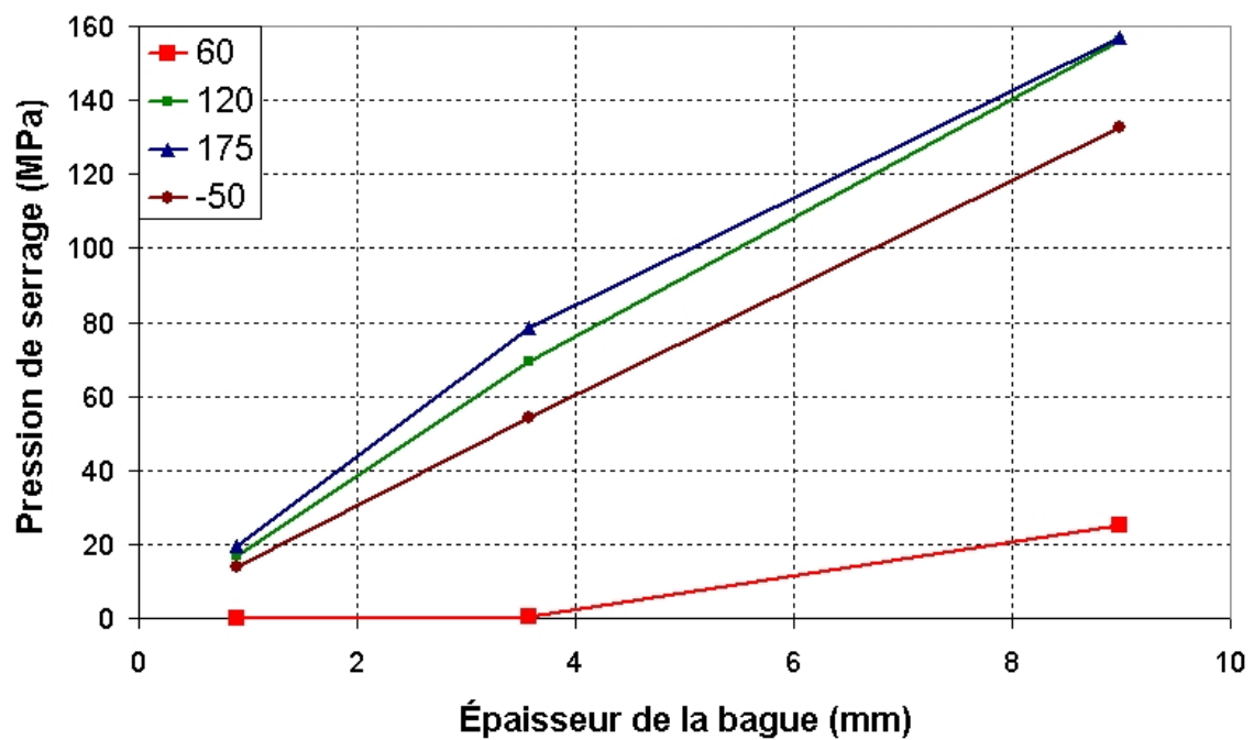
FIG. 4.21 – Évolution de la pression de serrage en fonction de l'épaisseur de la bague à différentes températures : 60 et 120 °C (pendant le chauffage), 175 °C (fin du chauffage) et -55 °C (fin du refroidissement)
