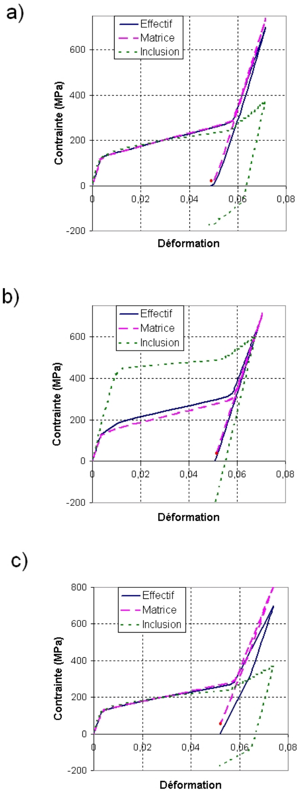
FIG. 5.4 – Évolution de la contrainte effective de chacune des phases lors de la prédéformation - Comparaison entre le \text{Ni}_{47}\text{Ti}_{44}\text{Nb}_9 et deux composites avec la même matrice, le premier avec 10 % d'inclusions fragiles et le second avec 25 % d'inclusions de comportement analogue à celui du \text{Ni}_{47}\text{Ti}_{44}\text{Nb}_9
