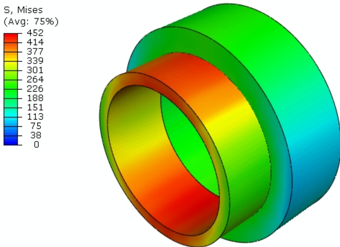
FIG. 4.30 – Répartition hétérogène de la contrainte dans la bague de serrage due au défaut de circularité
