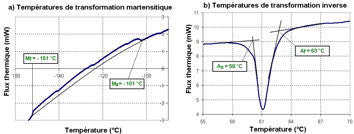
FIG. 2.14 – Résultats de l'analyse par DSC sur les échantillons prédéformés – a) Températures de transformation martensitique b) Températures de transformation inverse
