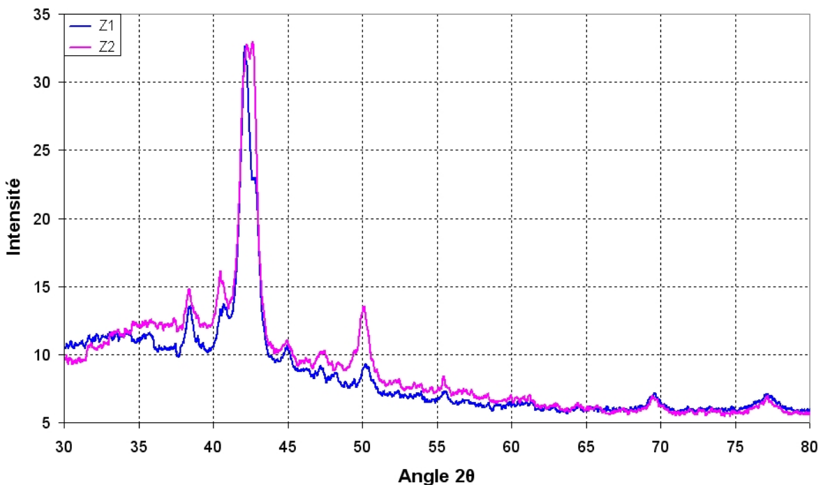
FIG. 2.16 – Comparaison de deux diffractogrammes obtenus sur deux zones différentes Z1 et Z2 appartenant au même échantillon martensitique
