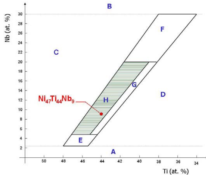
FIG. 1.16 – Influence de la teneur en niobium sur les propriétés mécaniques du NiTiNb (Simpson et al. 1988). Zone H : ensemble des compositions répondant aux contraintes de l'application considérée
