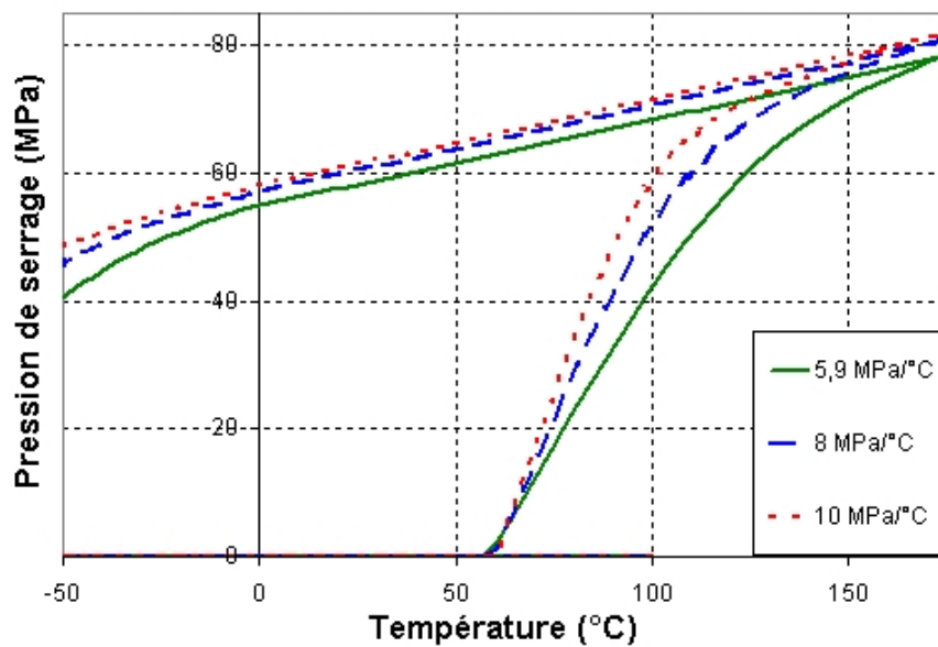
FIG. 3.11 – Influence du paramètre b sur la pression de serrage - b = 5,9 ; 8 et 10 MPa/°C
