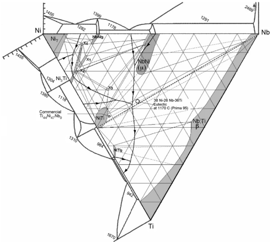
FIG. 1.13 – Diagramme de phase ternaire du NiTiNb (Grummon et al. 2006)
