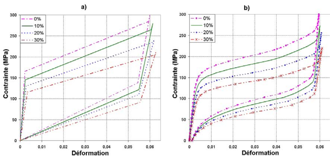
FIG. 5.6 – Évolution de la contrainte en fonction de la déformation pour un AMF poreux - a) Résultats de Entchev et Lagoudas (2002), b) Résultats avec le modèle présenté
