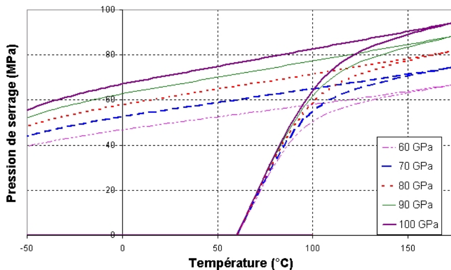
FIG. 3.6 – Influence du module de Young de la matrice sur la pression de serrage - E = 60 ; 70 ; 80 ; 90 et 100 GPa
