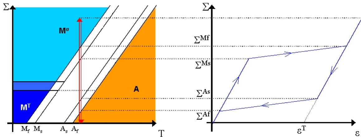
FIG. 1.3 – Évolution de la contrainte en fonction de la déformation lors d'un chargement superélastique et sa représentation dans le diagramme de transformation.
