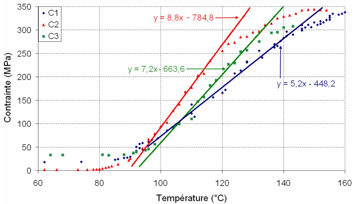
FIG. 2.25 – Évolution de la contrainte en fonction de la déformation lors du chauffage des bagues S1, en bloquant le déplacement de leur diamètre interne
