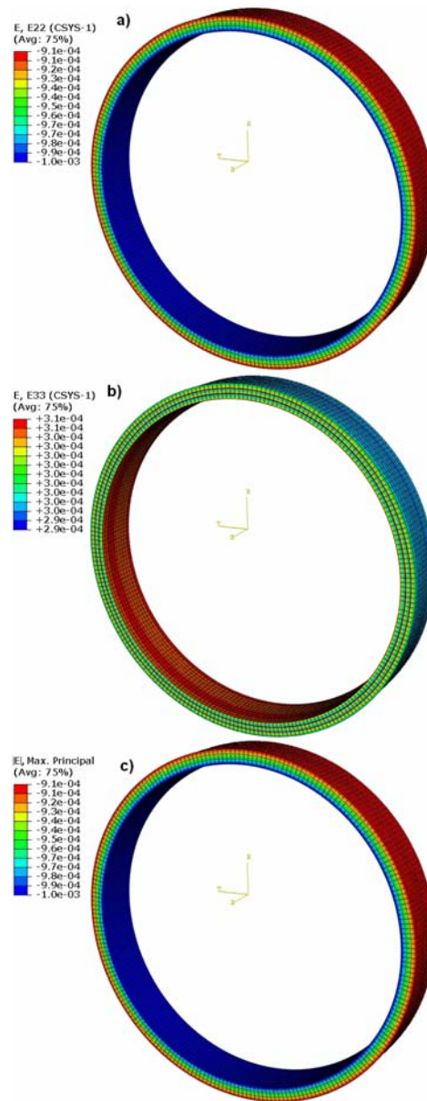
FIG. A.9 – Résultat d'une simulation par éléments finis vérifiant que les déformations principales coïncident avec les déformations \varepsilon_\theta et \varepsilon_z dans le cas axisymétrique - a) \varepsilon_\theta b) \varepsilon_z c) \varepsilon_P
