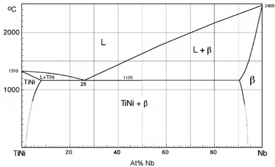
FIG. 1.14 – Estimation du diagramme de phase binaire du [NiTi]équiatomique-Nb (Grummon et al. 2006)
