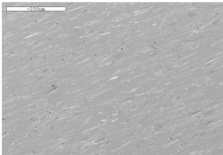
FIG. 2.2 – Micrographie du \text{Ni}_{47}\text{Ti}_{44}\text{Nb}_9 dans le sens longitudinal - Échelle 200 \mu\text{m}
