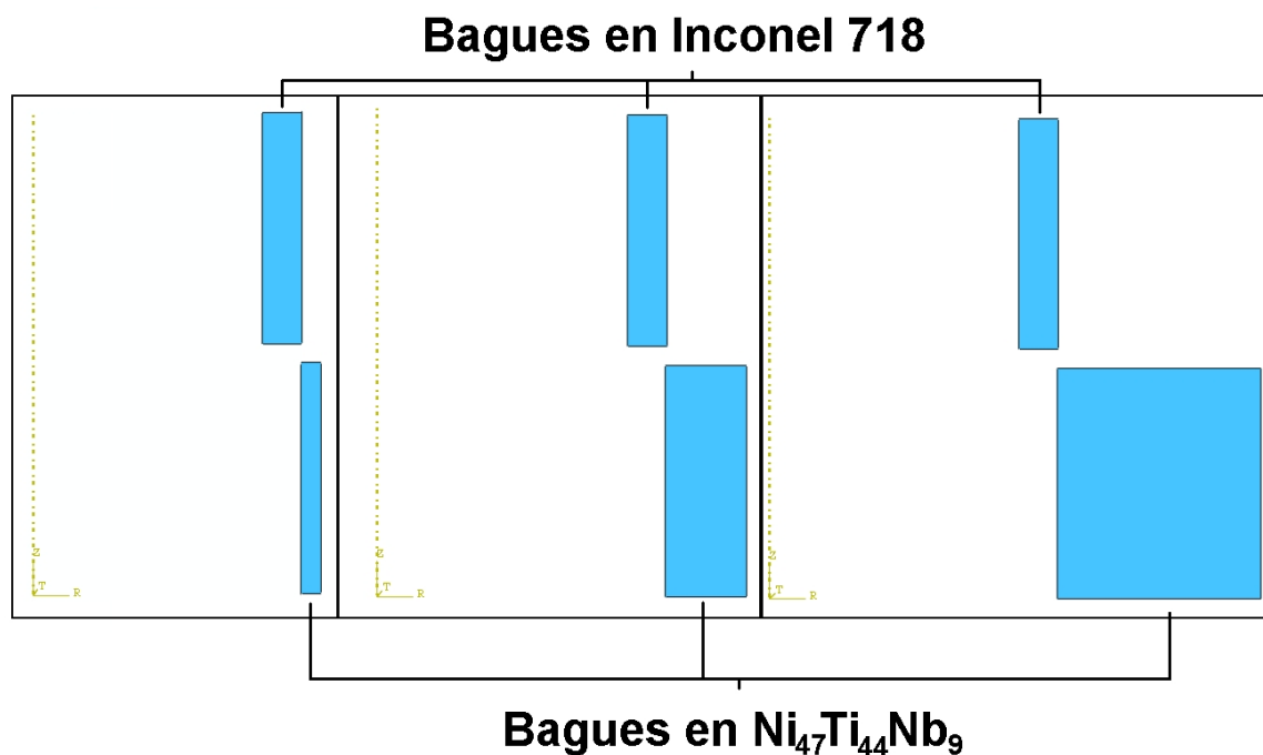
FIG. 4.16 – Géométrie des trois configurations simulées avec une bague en NiTiNb fine, moyenne et épaisse
