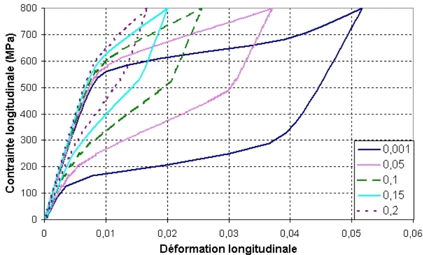
FIG. 5.1 – Simulation d'un composite avec une matrice de NiTi et des inclusions rigides ( E = 140 GPa)
