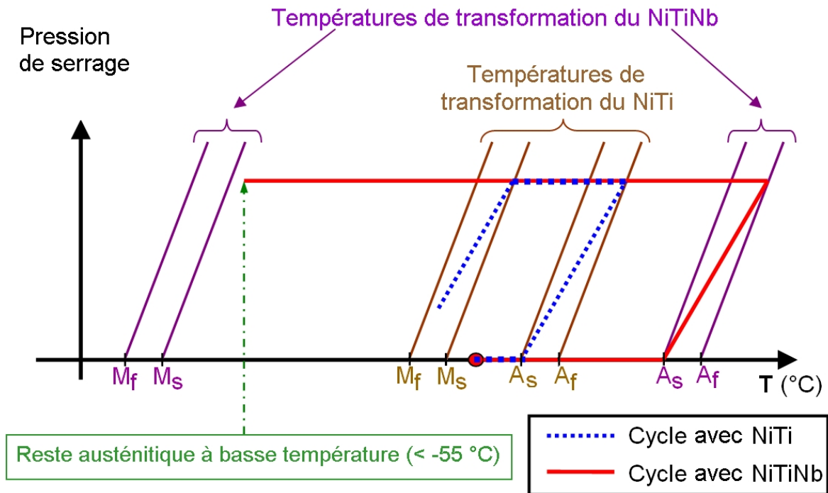
FIG. 1.12 – Évolution de la pression de serrage durant le cycle - Comparaison entre le NiTi et le NiTiNb
