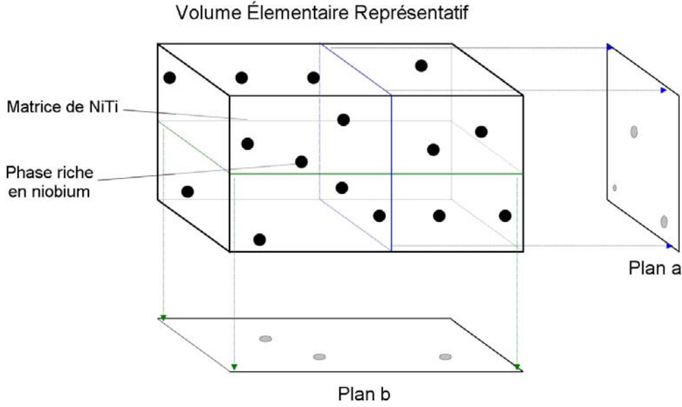
FIG. 3.2 – Volume Élémentaire Représentatif de la microstructure du \text{Ni}_{47}\text{Ti}_{44}\text{Nb}_9 composé d'une matrice en AMF et d'inclusions élastoplastiques sphériques
