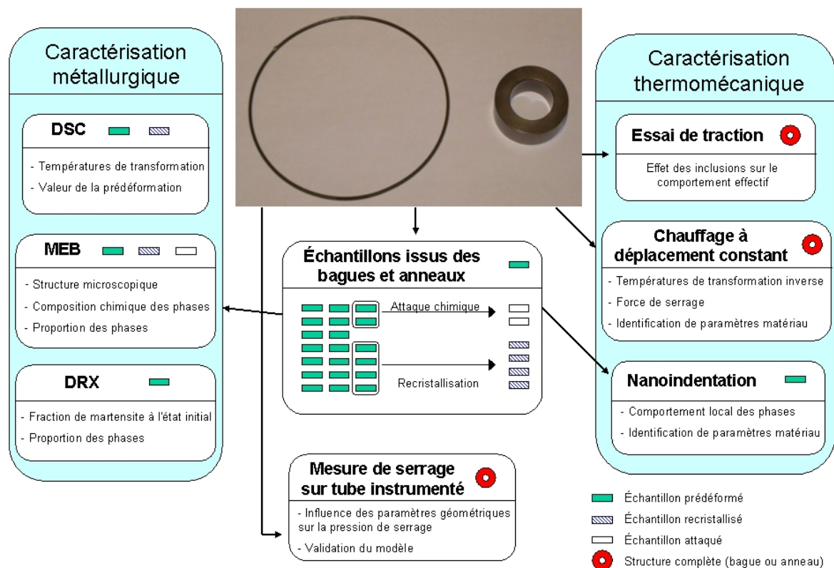
FIG. 2.1 – Synthèse des essais expérimentaux réalisés lors des travaux de thèse : essais de caractérisation métallurgique (DSC, MEB, DRX), essais de caractérisation thermomécanique (traction, chauffage à déplacement constant, nanoindentation) et essais sur le dispositif de serrage étudié
