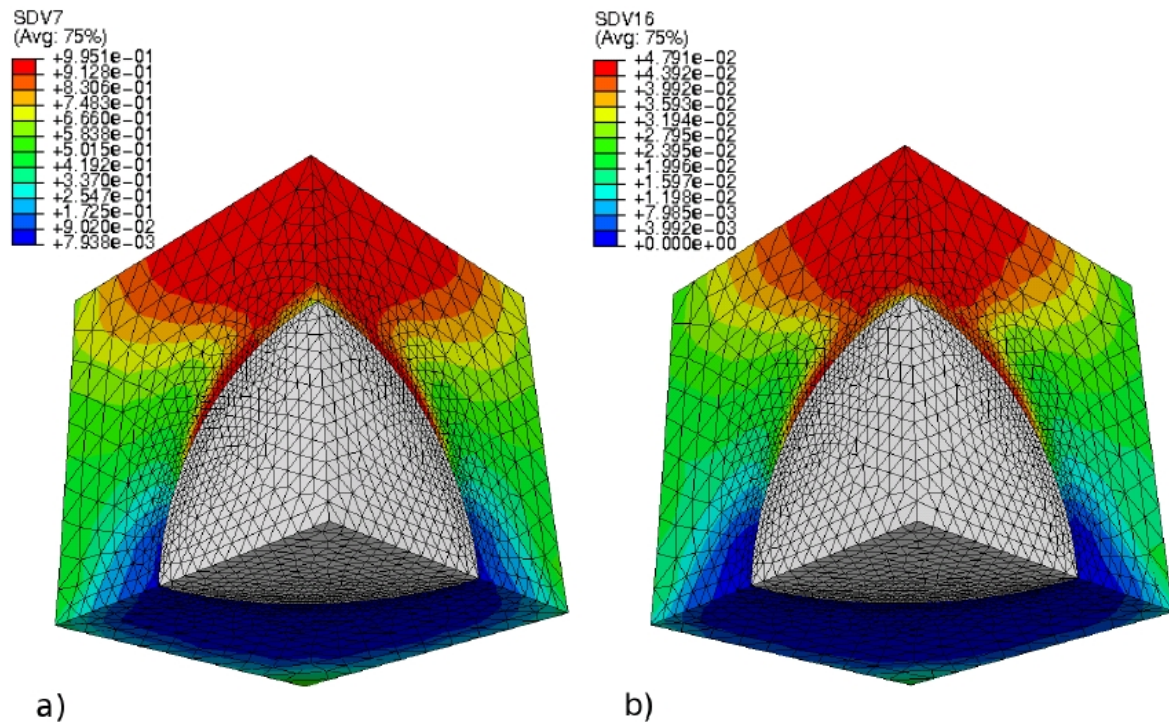
FIG. 5.8 – a) Répartition de la fraction volumique de martensite à 60 °C pour une déformation de 3 % - b) Répartition de la déformation de transformation à -20 °C pour une déformation de 3 % (Chemisky et al. 2009b)
