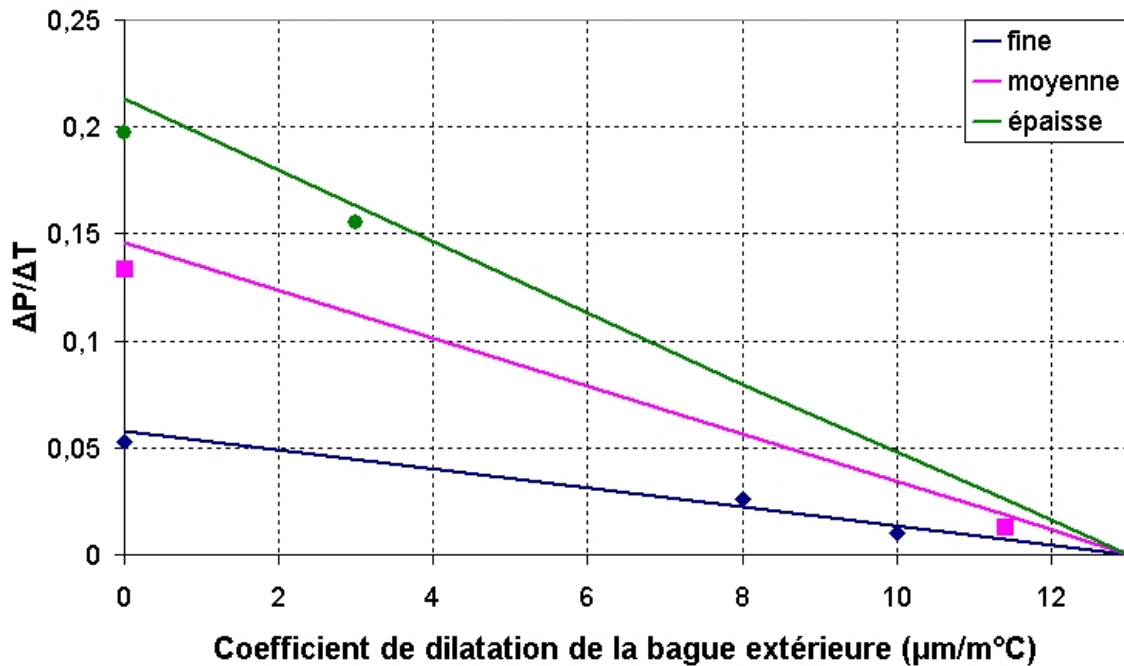
FIG. 4.25 – Simulation du serrage avec un comportement thermoélastique de la bague extérieure, pour différentes valeurs de son coefficient de dilatation - Comparaison avec le modèle de comportement du NiTiNb (marques rondes pour bague épaisse, carrées pour bague moyenne et losanges pour bague fine)
