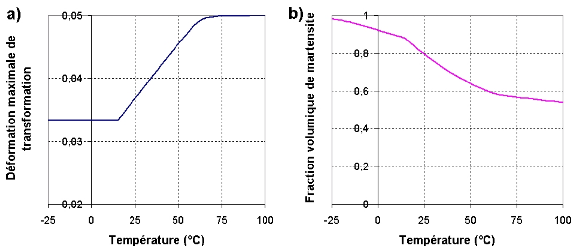
FIG. 4.28 – Variation de la déformation maximale de transformation (a) et de la fraction volumique de martensite (b) en fonction de la température pour un cycle de serrage avec un matériau dont la force critique d'orientation des variantes vaut 75 MPa.
