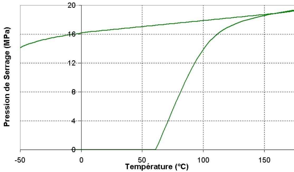
FIG. 4.18 – Simulation du dispositif avec une bague fine - Évolution de la pression de serrage en fonction de la température
