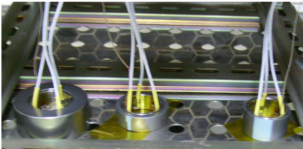
FIG. 4.6 – Photographie des trois dispositifs placés dans l'enceinte thermique avant le début de l'essai
