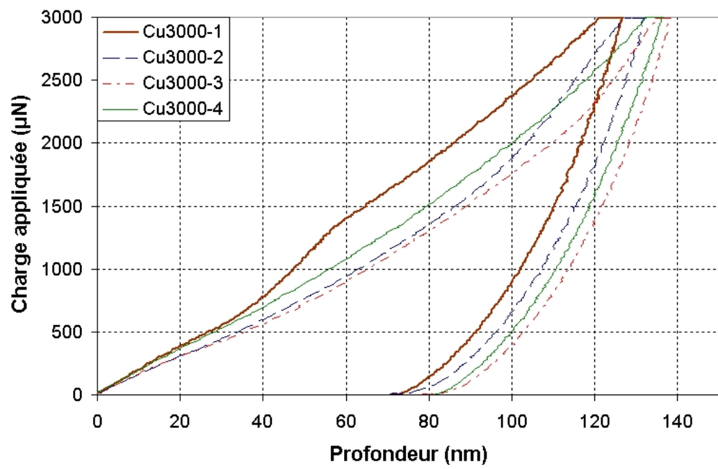
FIG. 2.33 – Résultats de nanoindentation sur des échantillons de CuAlBe (charge appliquée de 3000 µN)
