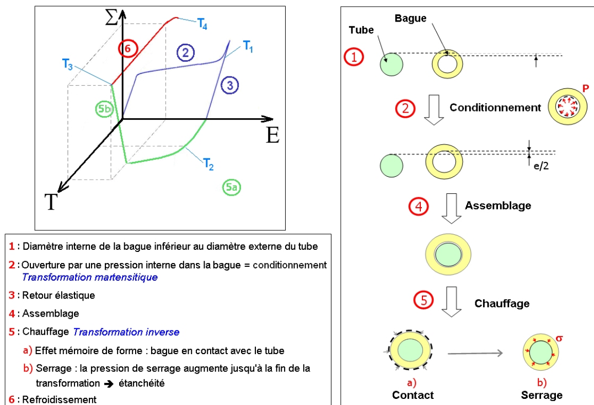
FIG. 1.11 – Cycle thermomécanique appliqué sur la bague à mémoire de forme - Conditionnement (1-3), assemblage (4) et chauffage jusqu'à serrage (5)
