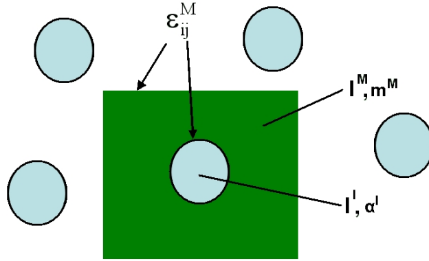
FIG. 3.3 – Représentation 2D de la solution inélastique de Mori-Tanaka
