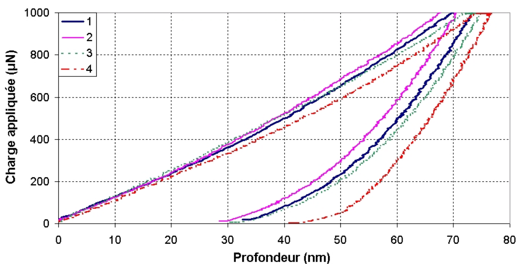
FIG. A.2 – Résultats de nanoindentation sur des échantillons de \text{Ni}_{47}\text{Ti}_{44}\text{Nb}_9 avec une charge appliquée de 1000\ \mu\text{N} et une vitesse de 200\ \mu\text{N/s}
