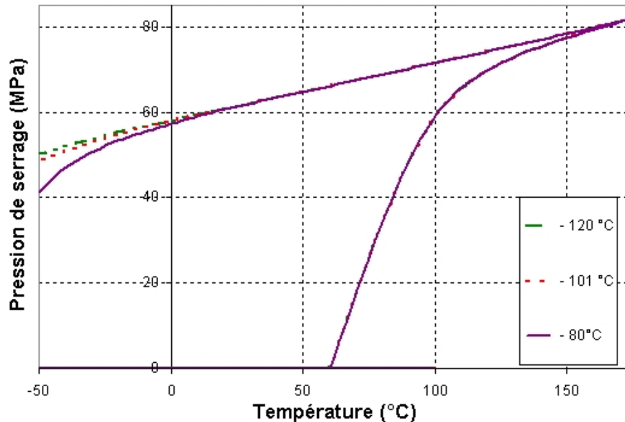
FIG. 3.9 – Influence de la température M_s sur la pression de serrage - M_s = -120 ; -101 et -80\text{ }^{\circ}\text{C}
