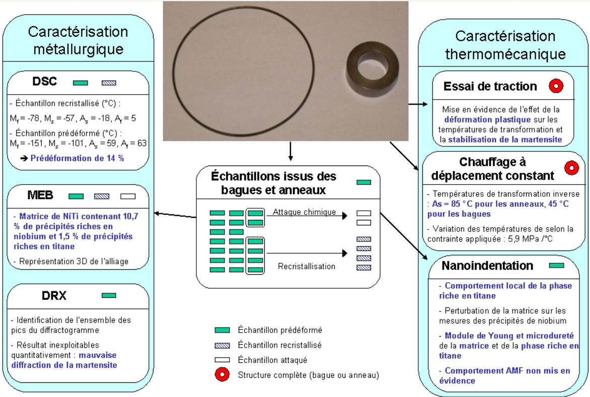
FIG. 2.35 – Synthèse des résultats expérimentaux présentés dans le chapitre 2 : essais de caractérisation métallurgique (DSC, MEB, DRX) et essais de caractérisation thermomécanique (traction, chauffage à déplacement constant, nanoindentation)
