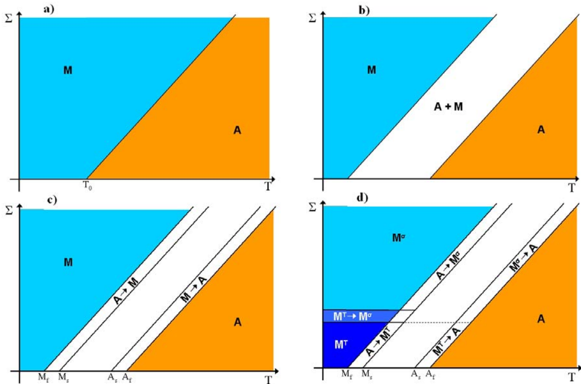
FIG. 1.2 – Construction du diagramme de transformation général d'un AMF - Représentation des deux phases stables suivant l'état thermomécanique a), tenant compte de l'hystérésis de transformation b), du décalage entre les températures de début et de fin de transformation c), de l'orientation des variantes de martensite d)
