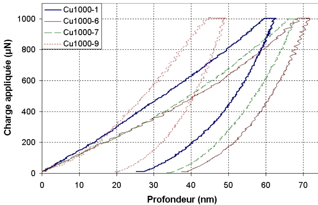
FIG. 2.32 – Résultats de nanoindentation sur des échantillons de \text{CuAlBe} (une charge appliquée de 1000 \mu\text{N} )
