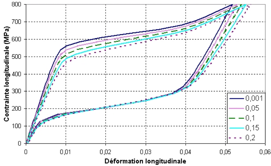
FIG. 5.2 – Simulation d'un composite avec une matrice de NiTi et des inclusions souples ( E = 10 GPa)
