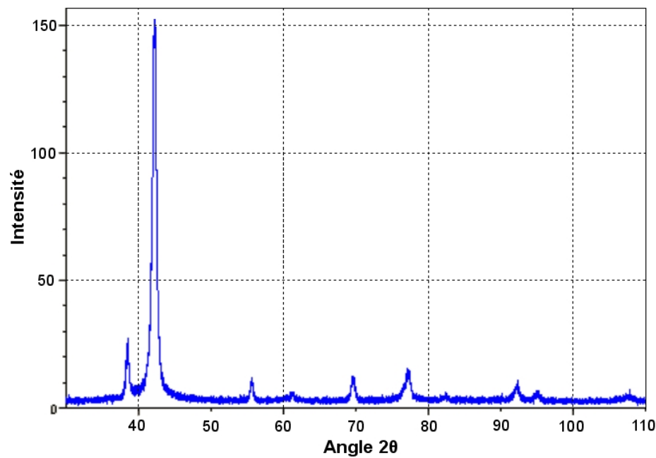
FIG. 2.15 – Diffractogramme obtenu lors de l’analyse par DRX d’un échantillon totalement austénitique
