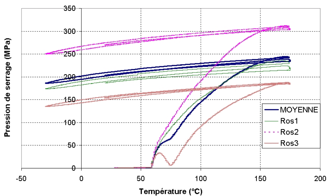
FIG. A.15 – Évolution de la pression de serrage obtenue via les trois rosettes sur la bague épaisse lors du cycle A2
