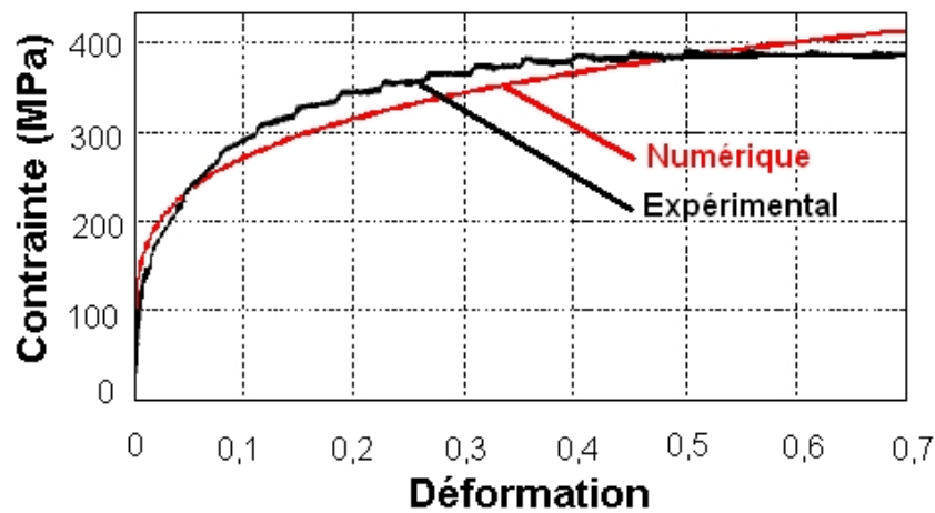
FIG. 3.5 – Comparaison entre un essai de traction sur du niobium pur et une simulation avec le modèle élastoplastique choisi - Recherche et identification des paramètres matériau.
