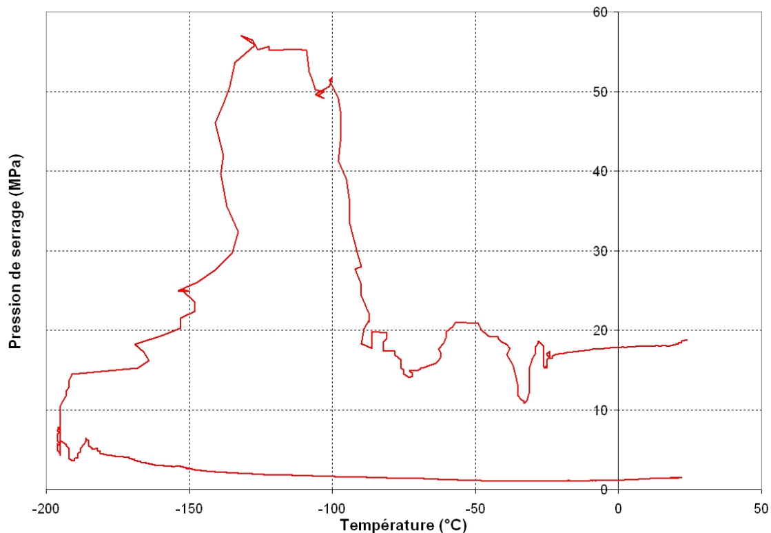
FIG. 4.13 – Évolution de la pression de serrage dans la bague fine lors de la trempe dans l'azote liquide
