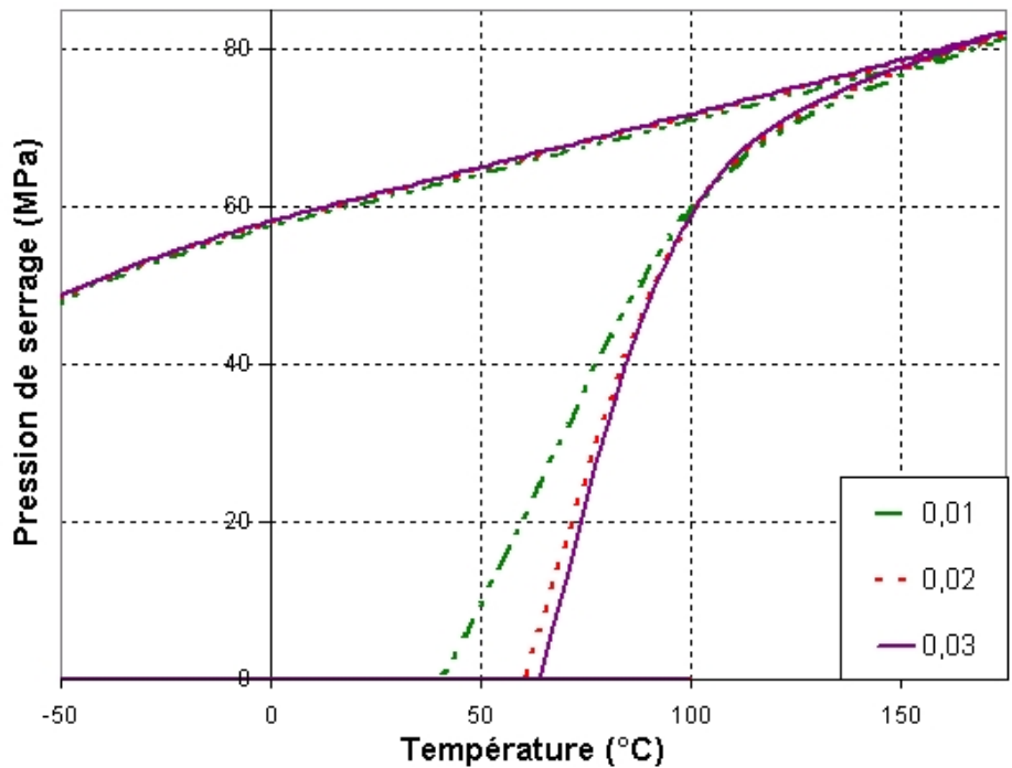
FIG. 3.8 – Influence de la déformation maximale de transformation sur la pression de serrage - \varepsilon_{max}^T = 0,01 ; 0,02 et 0,03
