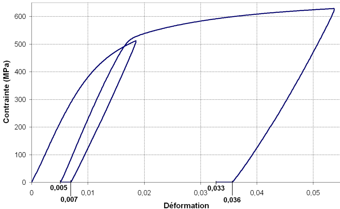
FIG. 2.23 – Essai de traction sur un échantillon de \text{Ni}_{47}\text{Ti}_{44}\text{Nb}_9 à 60^\circ\text{C}
