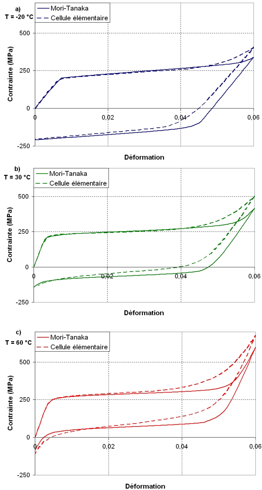
FIG. 5.9 – Comparaison de la réponse à un chargement homogène isotherme à -20 (a), 30 (b) et 60 °C (c) d'un matériau de type NiTiNb entre deux types de simulations : cellule élémentaire (pointillés) et schéma de Mori-Tanaka (traits pleins).
