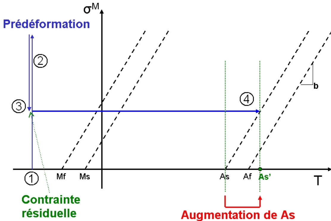
FIG. 5.5 – Comportement dans la matrice lors du cycle appliqué - Explication de l'augmentation de la température A_s
