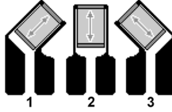
FIG. 4.3 – Numérotation des rosettes
