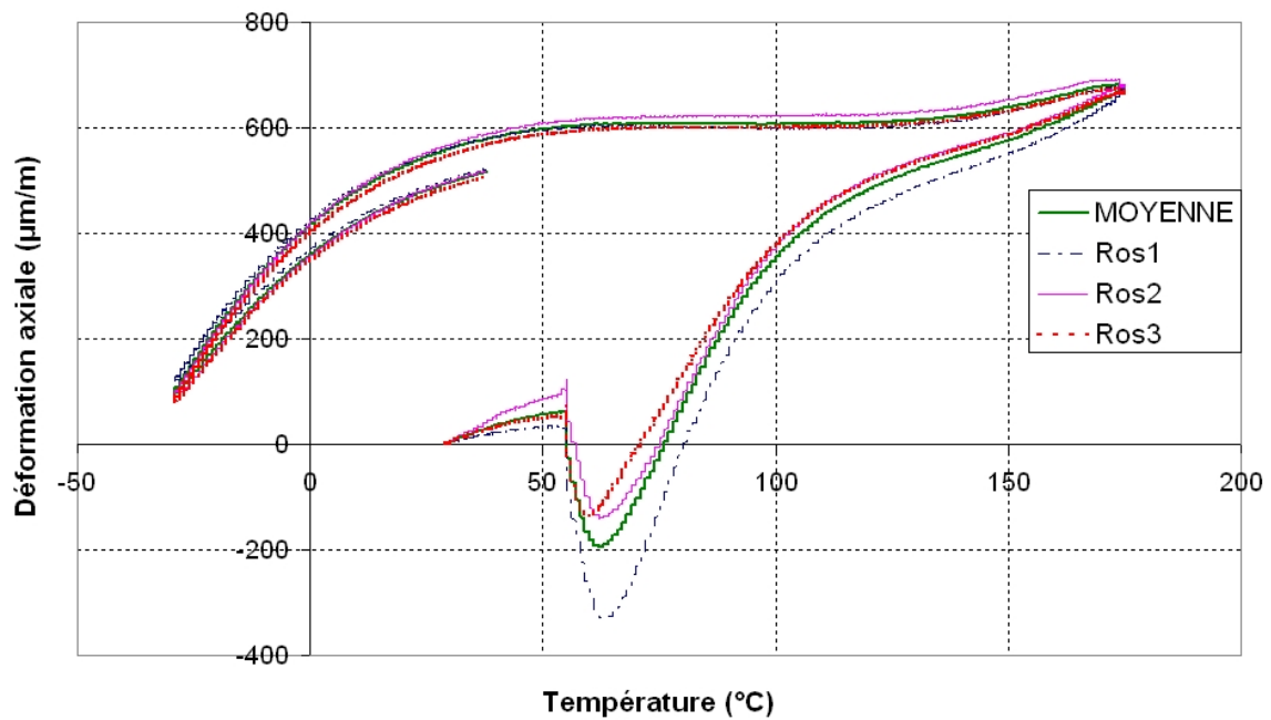
FIG. A.11 – Évolution des déformations axiales relevées sur les rosettes de la bague moyenne lors du cycle A2
