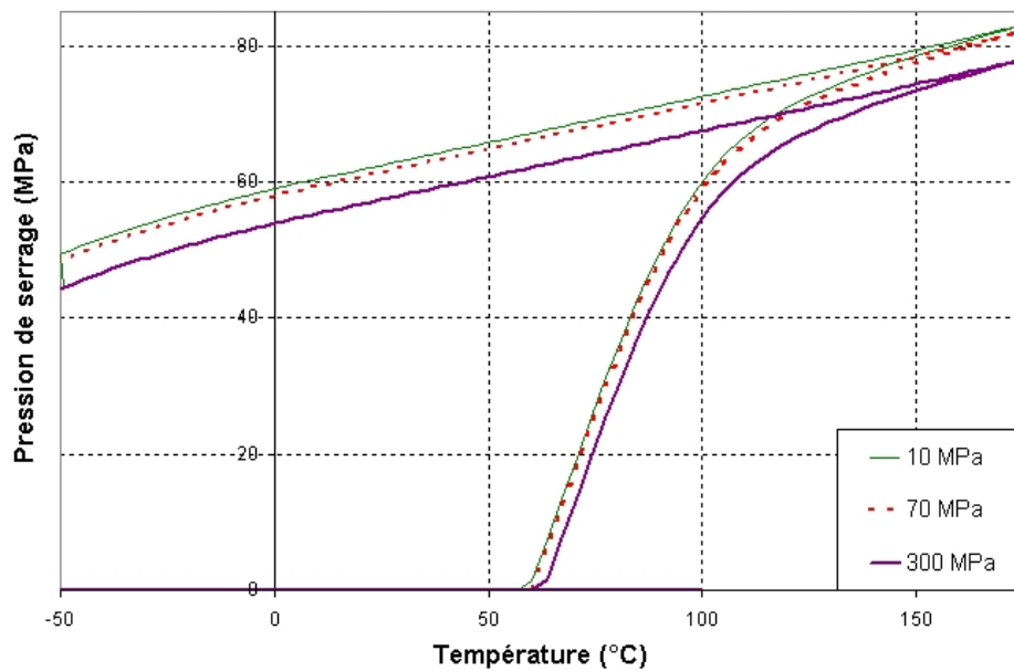
FIG. 3.15 – Influence de la limite élastique des inclusions sur la pression de serrage - \sigma_Y = 10 ; 70 et 300 MPa
