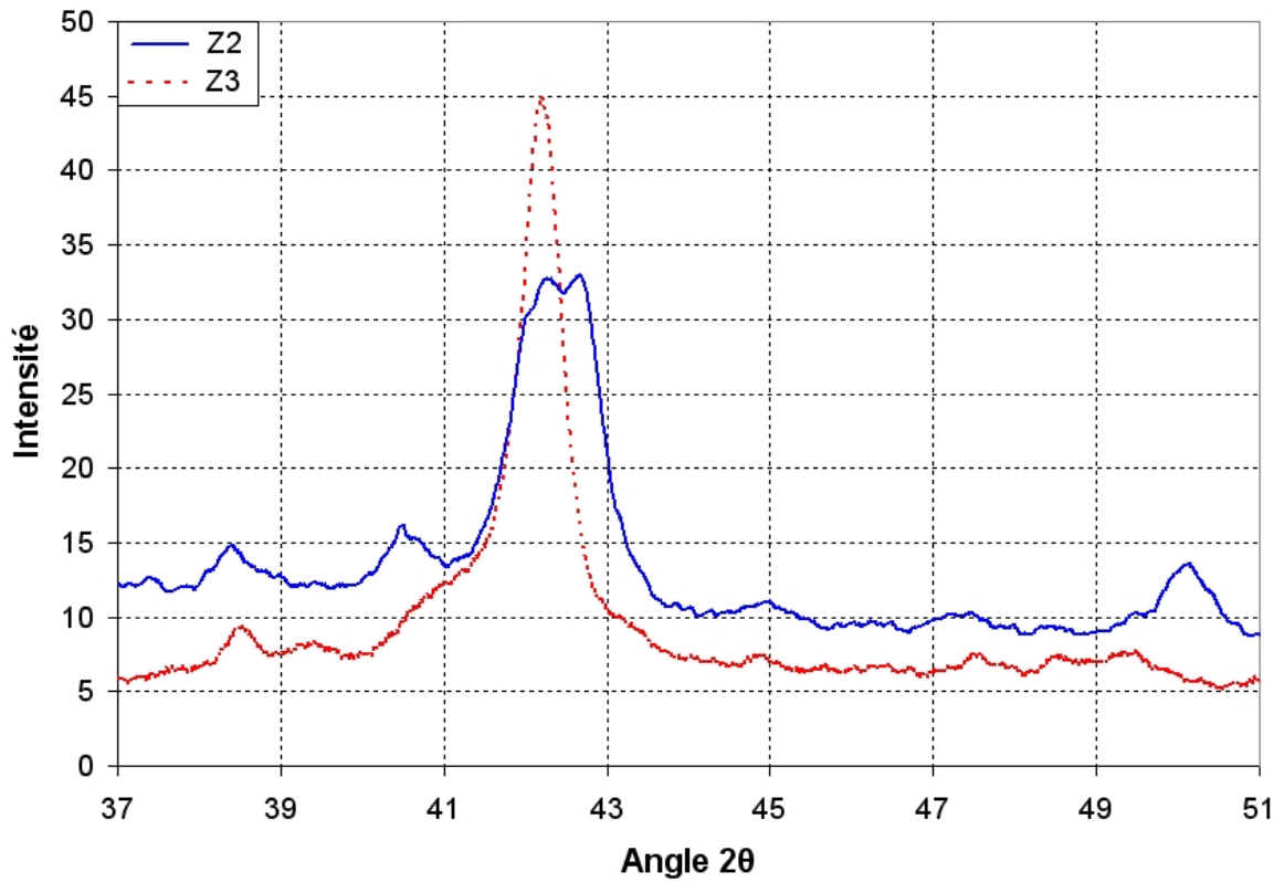
FIG. 2.18 – Comparaison de diffractogrammes d’un échantillon vierge (zone Z2) et d’un échantillon chauffé (zone Z3)
