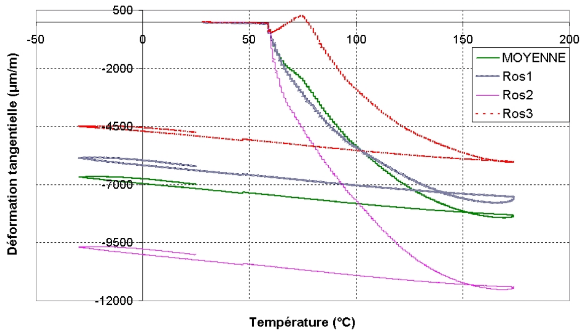
FIG. A.13 – Évolution des déformations tangentielles relevées sur les rosettes de la bague épaisse lors du cycle A2
