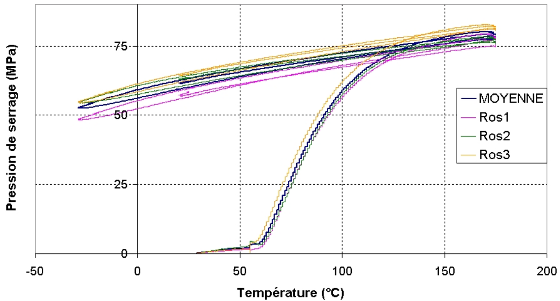
FIG. A.12 – Évolution de la pression de serrage obtenue via les trois rosettes sur la bague moyenne lors du cycle A2
