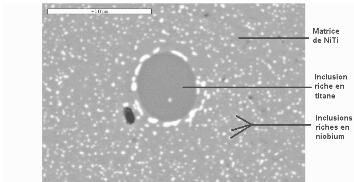
FIG. 2.7 – Micrographie du \text{Ni}_{47}\text{Ti}_{44}\text{Nb}_9 dans le sens transverse - Échelle 10 \mu\text{m}
