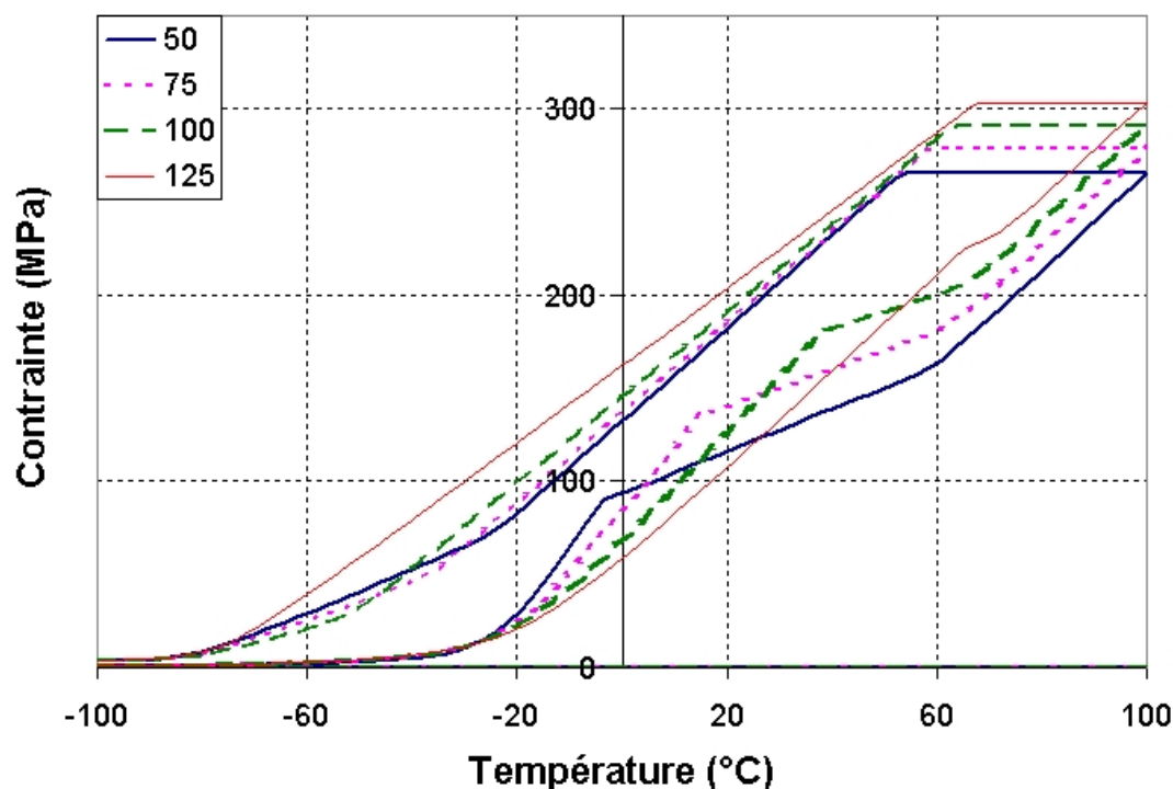
FIG. 4.27 – Simulations du cycle de serrage en faisant varier la force critique d'orientation de 50 à 125 MPa par pas de 25 MPa.
