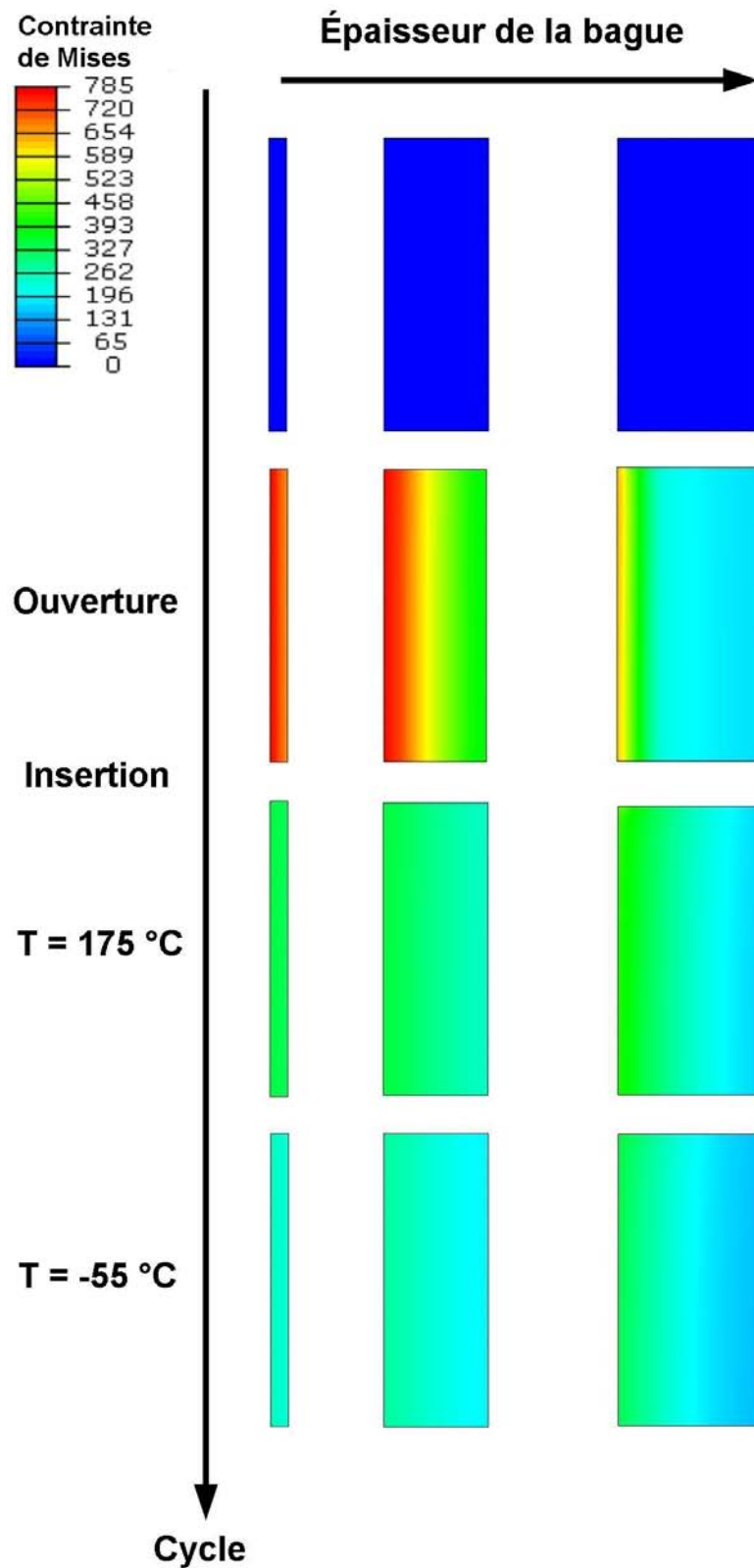
FIG. 4.22 – Évolution de la contrainte effective dans les bagues en NiTiNb pour les trois configurations : état initial, après ouverture, après chauffage à 175 °C, après refroidissement à - 55 °C
