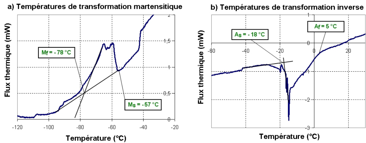
FIG. 2.13 – Résultats de l'analyse par DSC sur les échantillons recristallisés – a) Températures de transformation martensitique b) Températures de transformation inverse
