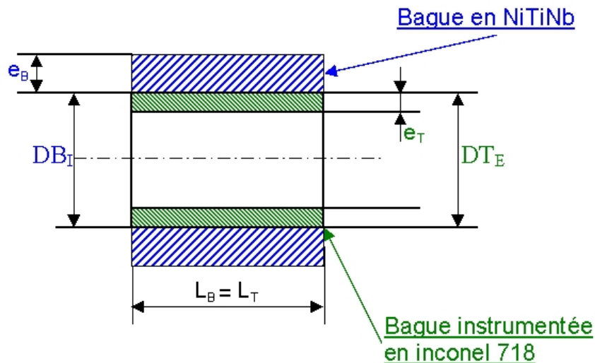
FIG. 4.1 – Dispositif de serrage d'une bague en NiTiNb sur une bague en Inconel 718 instrumentée de jauges d'extensométrie sur sa face intérieure
