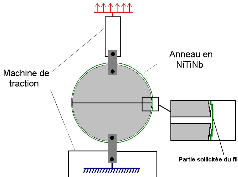
FIG. 2.24 – Schéma du dispositif de l'essai permettant de chauffer les bagues en maintenant le déplacement de leur face intérieure nul
