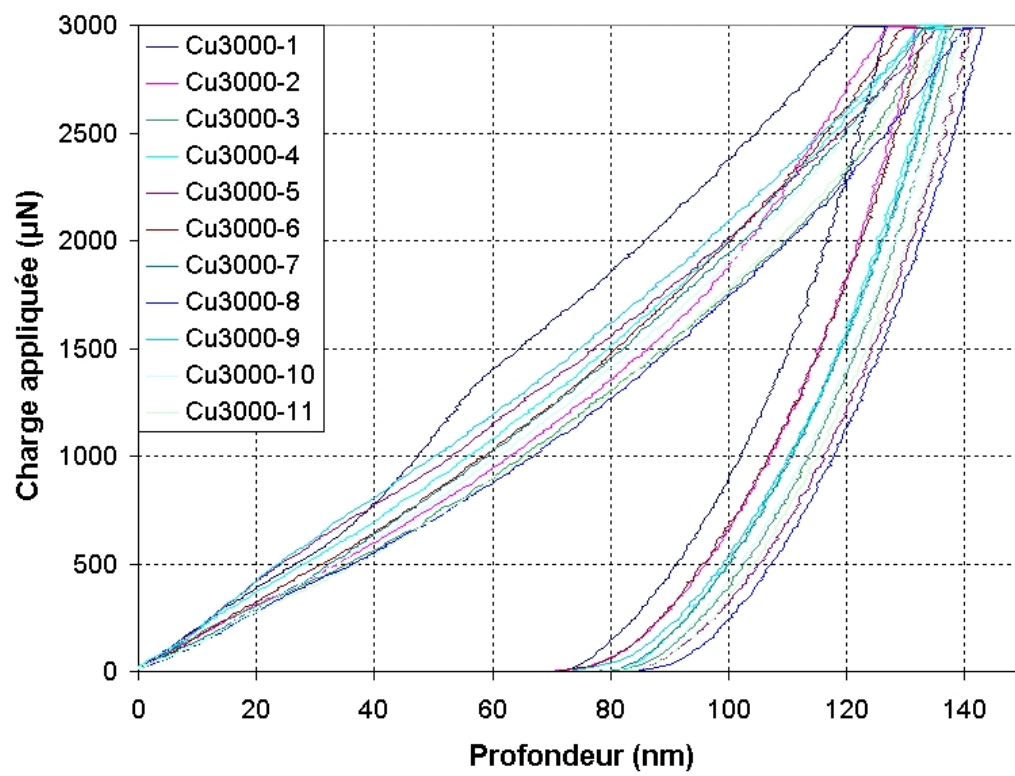
FIG. A.5 – Résultats de nanoindentation sur des échantillons de CuAlBe avec une charge appliquée de 3000 \mu\text{N}
