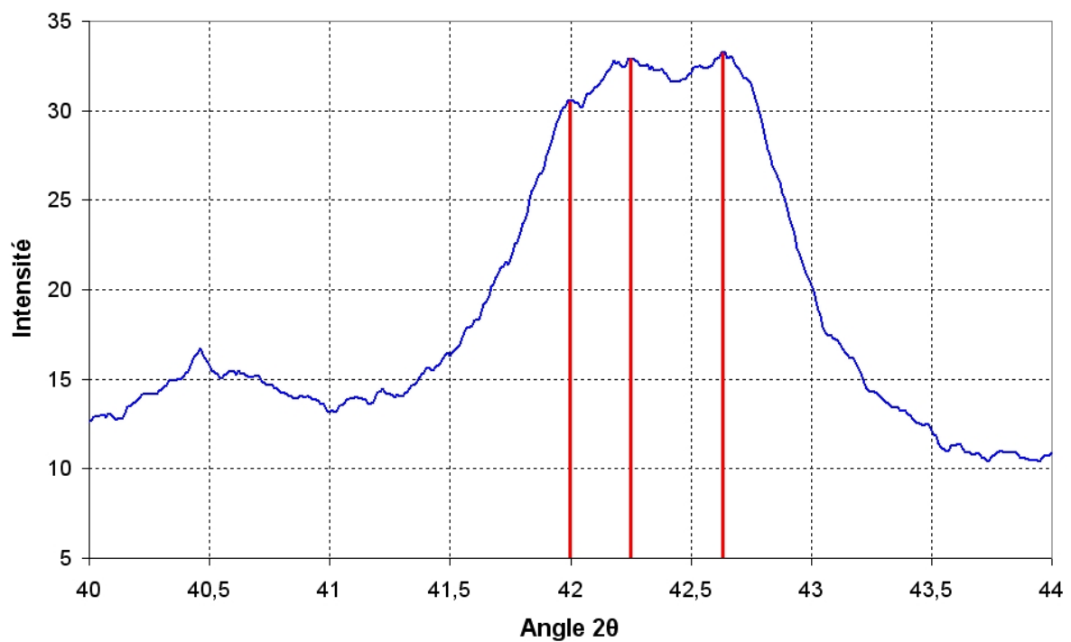
FIG. 2.17 – Zoom dans la région 2\theta = 42^\circ de la zone Z2
