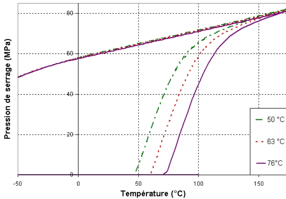
FIG. 3.10 – Influence de la température A_f sur la pression de serrage - A_f = 50 ; 63 et 76 °C
