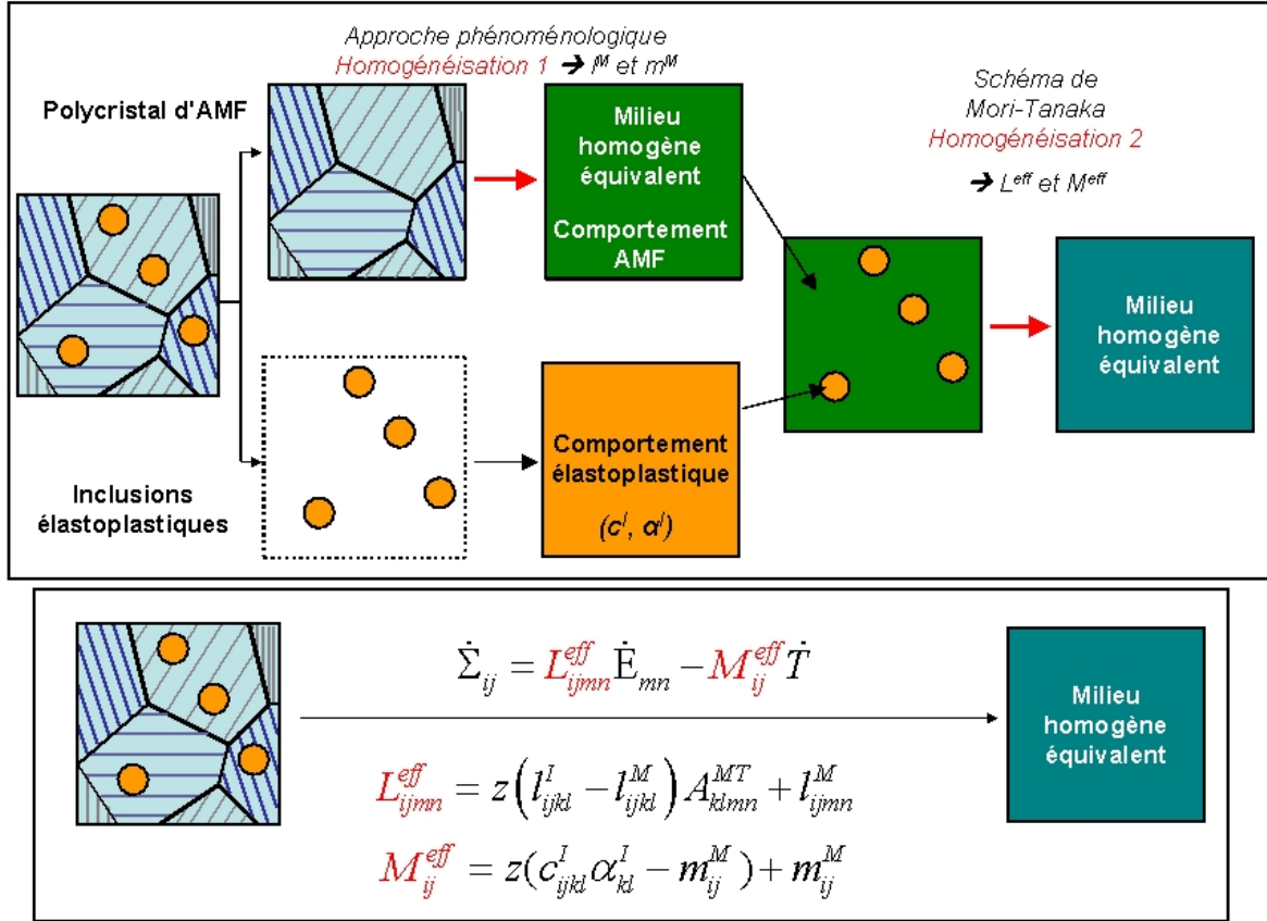
FIG. 3.1 – Stratégie d'homogénéisation permettant d'obtenir une loi de comportement macrohomogène depuis une microstructure hétérogène composée d'une matrice polycristalline en AMF et d'inclusions élastoplastiques sphériques
