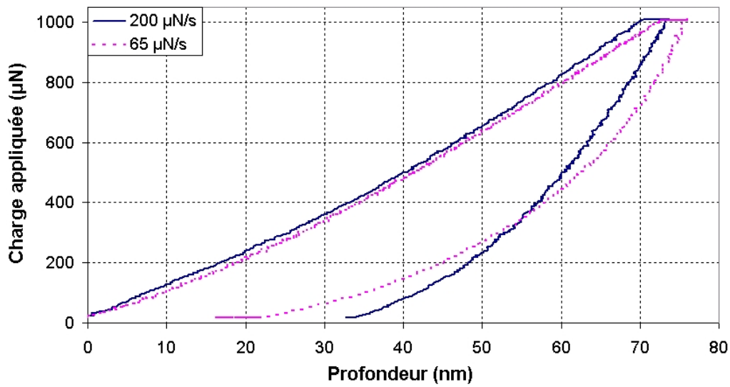
FIG. 2.31 – Résultats de nanoindentation sur des échantillons de \text{Ni}_{47}\text{Ti}_{44}\text{Nb}_9 avec une charge appliquée de 1000 \mu\text{N} et une vitesse de 65 et 200 \mu\text{N/s}
