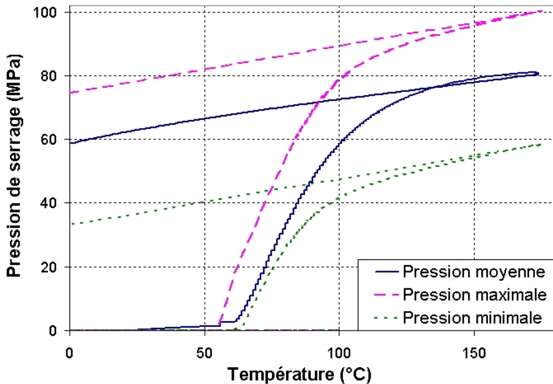
FIG. 4.31 – Évolution des pressions de serrage maximale et minimale - Comparaison avec la pression moyenne
