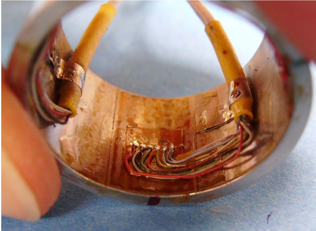
FIG. 4.4 – Photographie d'une rosette câblée en quart de pont
