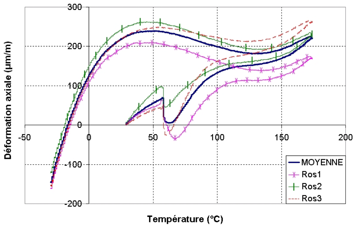
FIG. 4.8 – Évolution des déformations axiales relevées sur les rosettes de la bague fine lors du cycle A2
