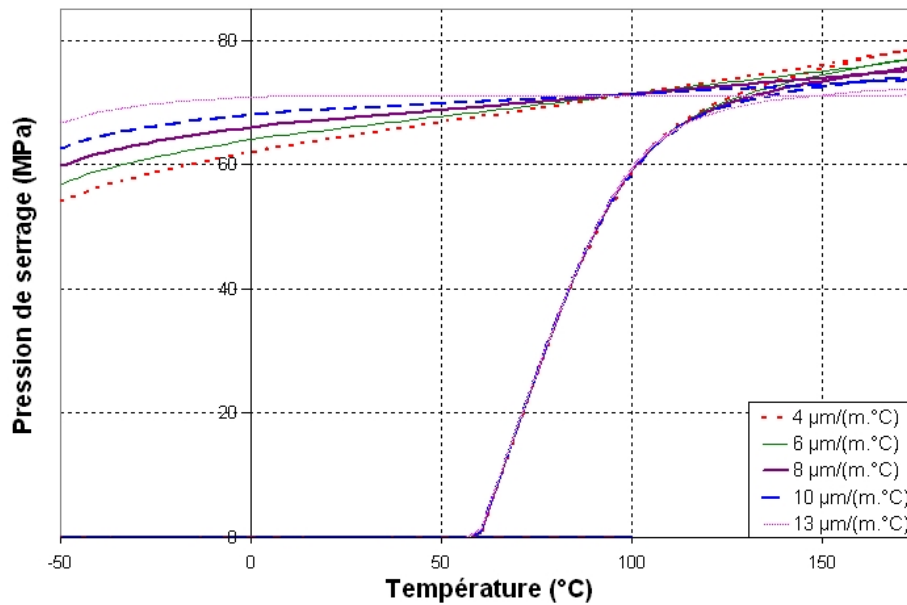
FIG. 3.7 – Influence du coefficient de dilatation sur la pression de serrage - \alpha^{AMF} = 4, 6, 8, 10 et 13 \mu\text{m}/(\text{m} \cdot ^\circ\text{C}) et \alpha^{Inconel} = 13 \mu\text{m}/(\text{m} \cdot ^\circ\text{C})
