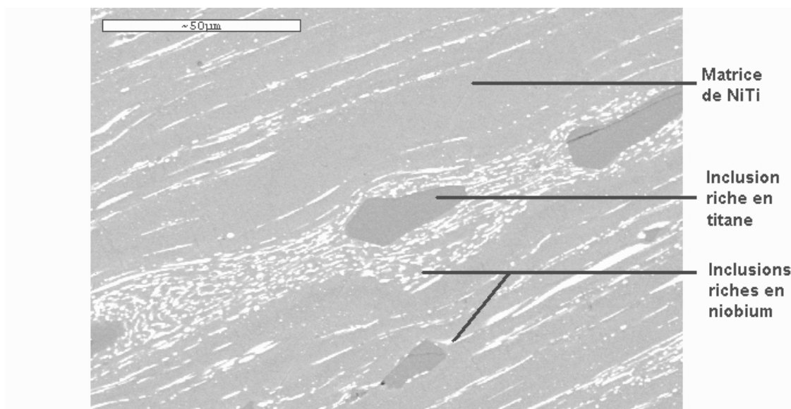
FIG. 2.4 – Micrographie du \text{Ni}_{47}\text{Ti}_{44}\text{Nb}_9 dans le sens longitudinal - Zoom sur une inclusion riche en titane - Échelle 50\ \mu\text{m}
