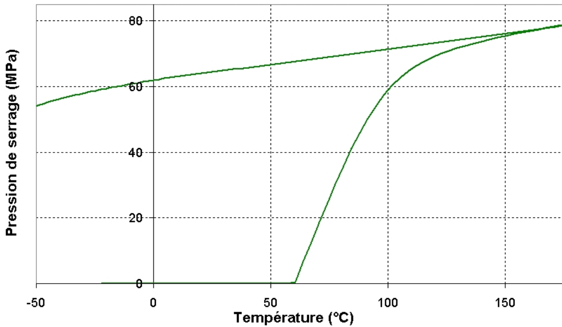
FIG. 4.19 – Simulation du dispositif avec une bague moyenne - Évolution de la pression de serrage en fonction de la température
