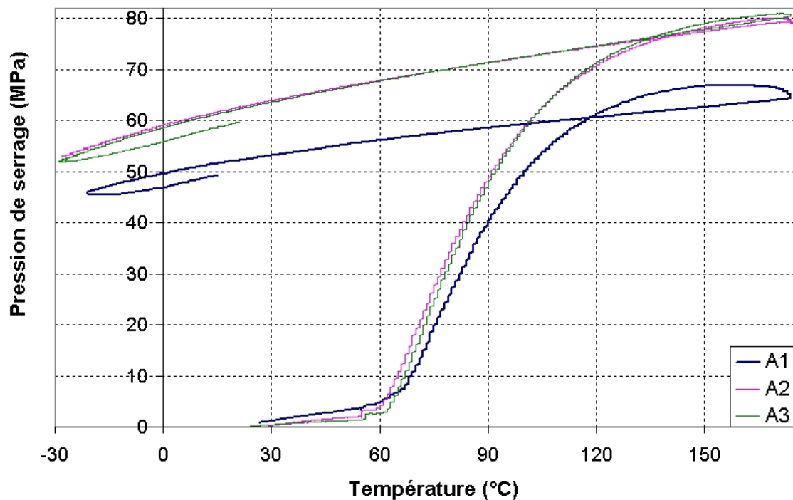
FIG. 4.11 – Évolution de la pression de serrage moyenne sur la bague moyenne lors des cycles A1, A2 et A3
