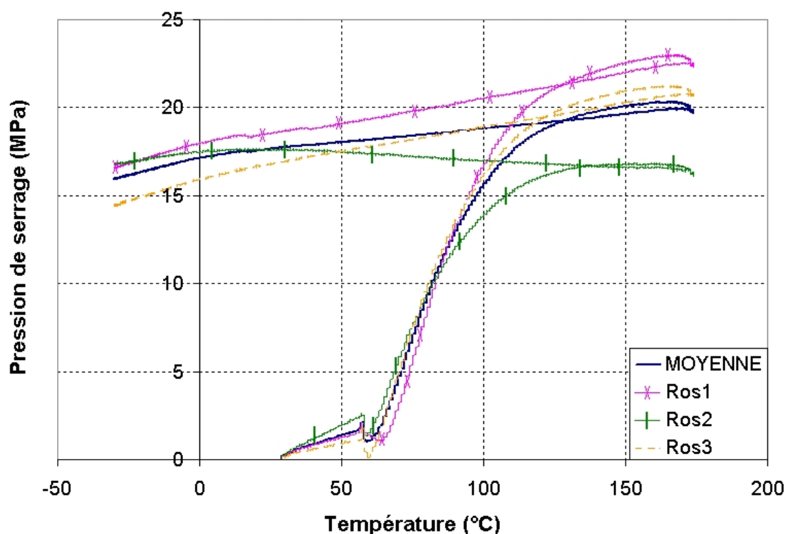
FIG. 4.9 – Évolution de la pression de serrage obtenue via les trois rosettes sur la bague fine lors du cycle A2
