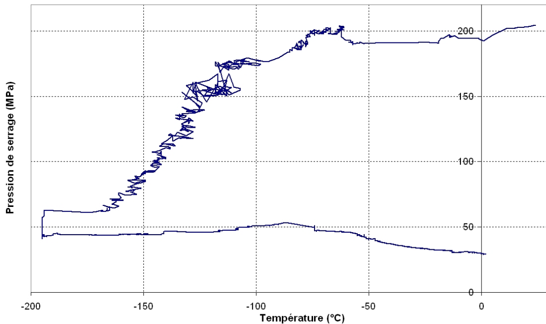
FIG. 4.14 – Évolution de la pression de serrage dans la bague épaisse lors de la trempe dans l'azote liquide
