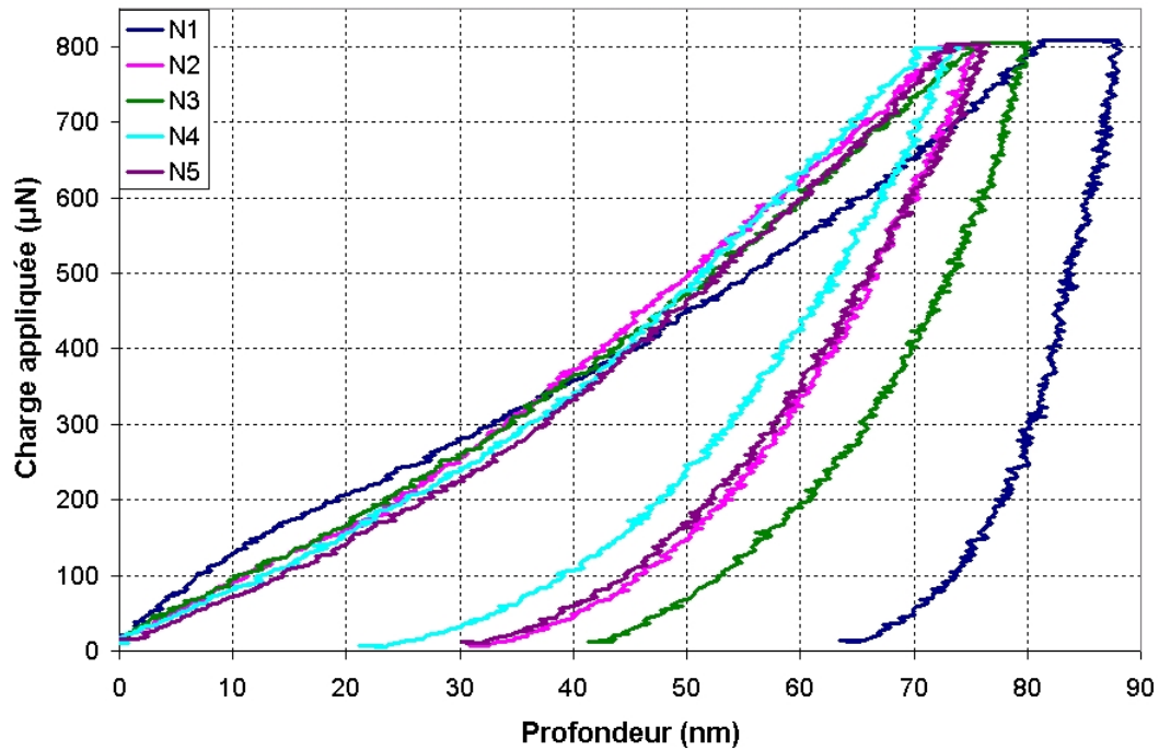
FIG. 2.27 – Résultats des essais de nanoindentation sur la matrice de NiTi
