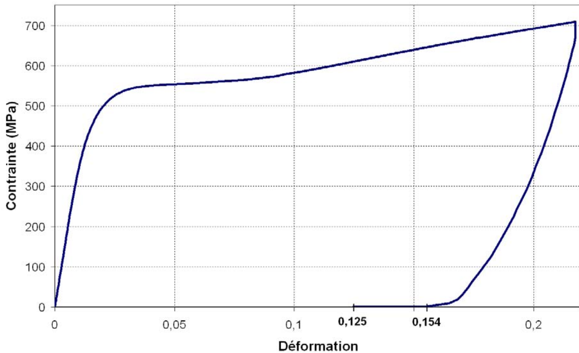
FIG. 2.20 – Essai de traction sur un échantillon de Ni_{47}Ti_{44}Nb_9 à 20°C
