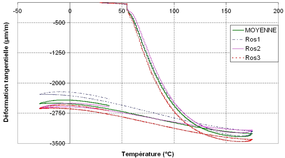
FIG. A.10 – Évolution des déformations tangentielle relevées sur les rosettes de la bague moyenne lors du cycle A2
