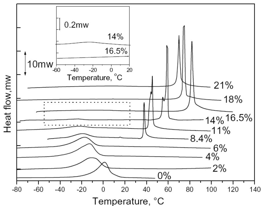
FIG. 1.17 – Caractérisation par DSC du \text{Ti}_{44}\text{Ni}_{47}\text{Nb}_9 sur des échantillons ayant subi différents niveaux de prédéformation, He et Rong (2004) - Mise en évidence de la stabilisation de la martensite
