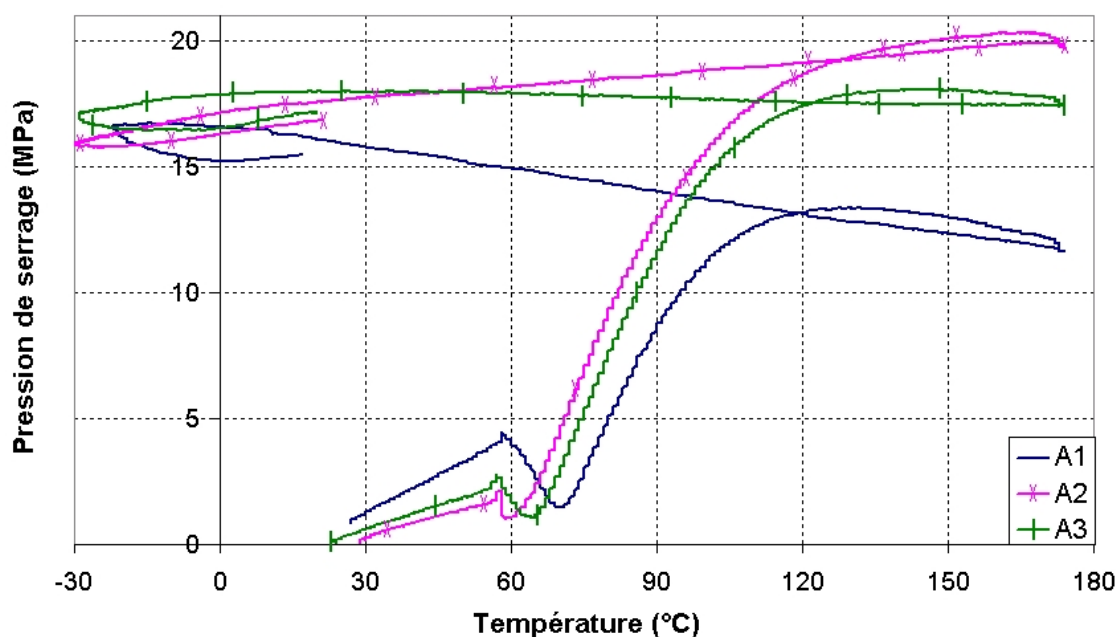
FIG. 4.10 – Évolution de la pression de serrage moyenne sur la bague fine lors des cycles A1, A2 et A3
