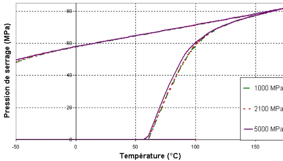
FIG. 3.13 – Influence du paramètre H_e sur la pression de serrage - H_e = 1000 ; 2100 et 5000 MPa
