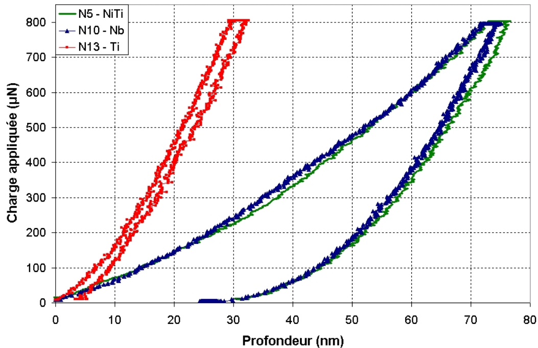
FIG. 2.30 – Comparaison des résultats moyens pour les différentes phases étudiées
