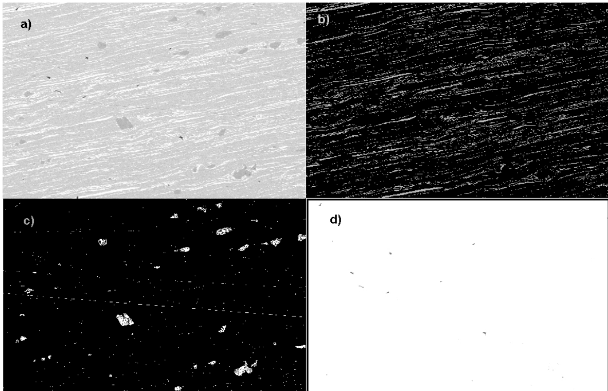
FIG. 2.11 – Analyse d'images effectuée sur une micrographie de \text{Ni}_{47}\text{Ti}_{44}\text{Nb}_9 - a) Micrographie de base ; b) Inclusions riches en niobium ; c) Inclusions riches en titane ; d) Carbures de silicium induits durant le polissage
