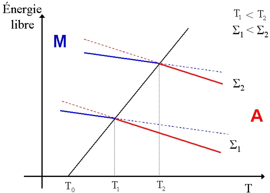
FIG. 1.1 – Évolution de l'énergie libre de la martensite et de l'austénite en fonction de la température et variation de la température d'équilibre selon la contrainte appliquée
