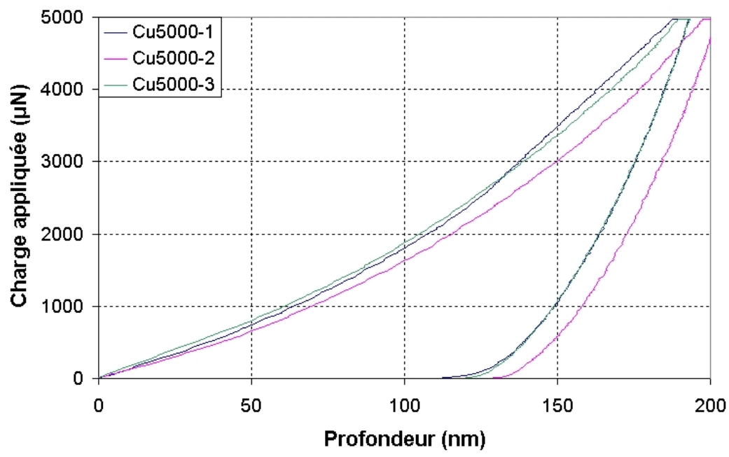
FIG. 2.34 – Résultats de nanoindentation sur des échantillons de CuAlBe (charge appliquée de 5000 µN)
