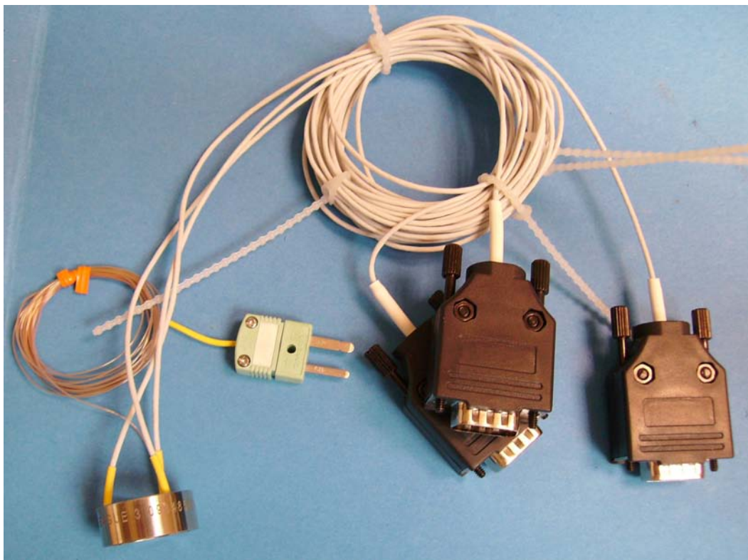
FIG. 4.5 – Photographie d'une bague instrumentée d'un thermocouple (à gauche) et de trois rosettes régulièrement collées à 120 °C
