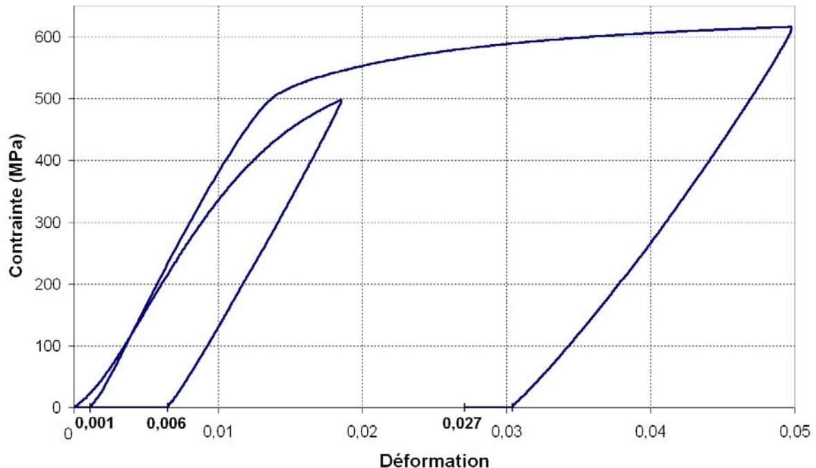
FIG. 2.22 – Essai de traction sur un échantillon de \text{Ni}_{47}\text{Ti}_{44}\text{Nb}_9 à 45^\circ\text{C}
