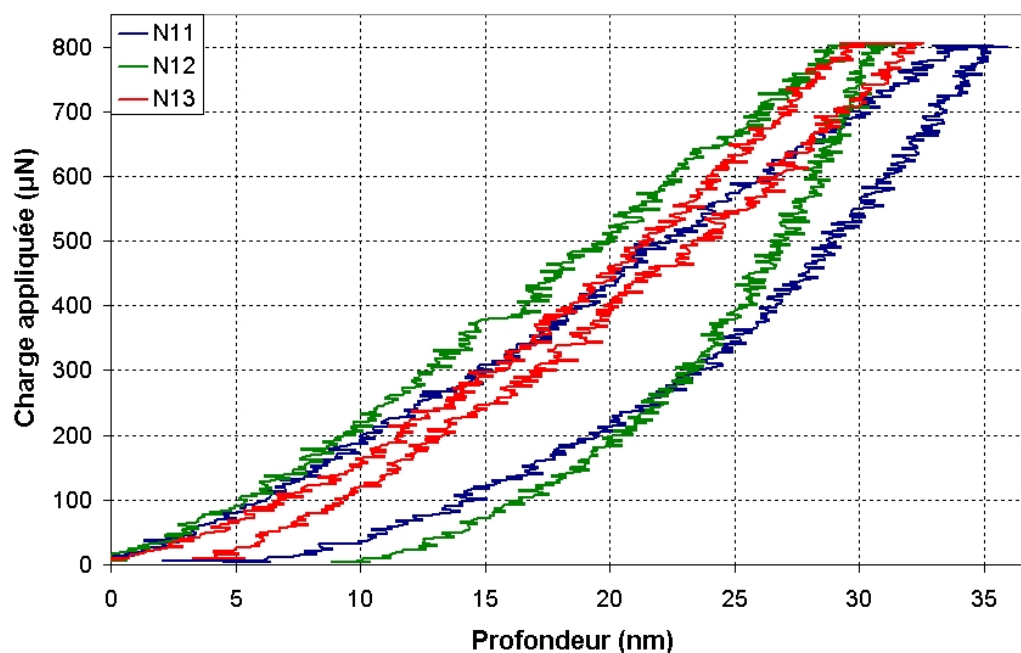
FIG. 2.29 – Résultats des essais de nanoindentation sur la phase riche en titane
