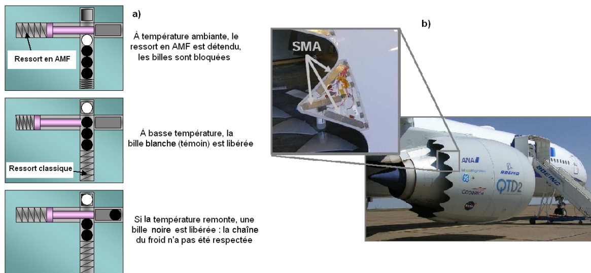
FIG. 1.8 – Exemples d'utilisation de l'effet mémoire double sens des AMF - a) Thermomarqueur Imago ® (Raymond et Weynant 1991) ; b) Chevrons développés par Boeing ® (Calkins et Butler 2004)
