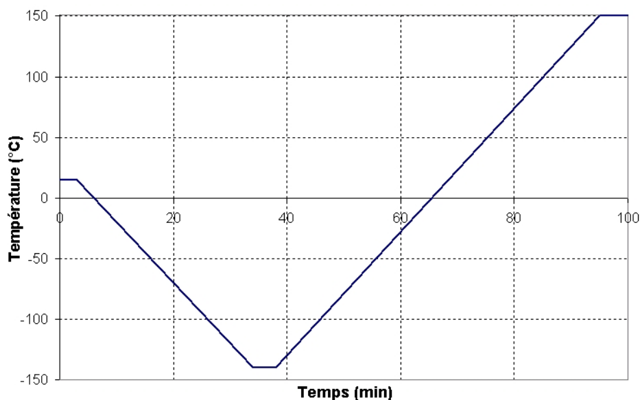
FIG. 2.12 – Cycle thermique imposé lors des analyses de DSC composé d'un refroidissement suivi d'un chauffage, à 5 °C/min
