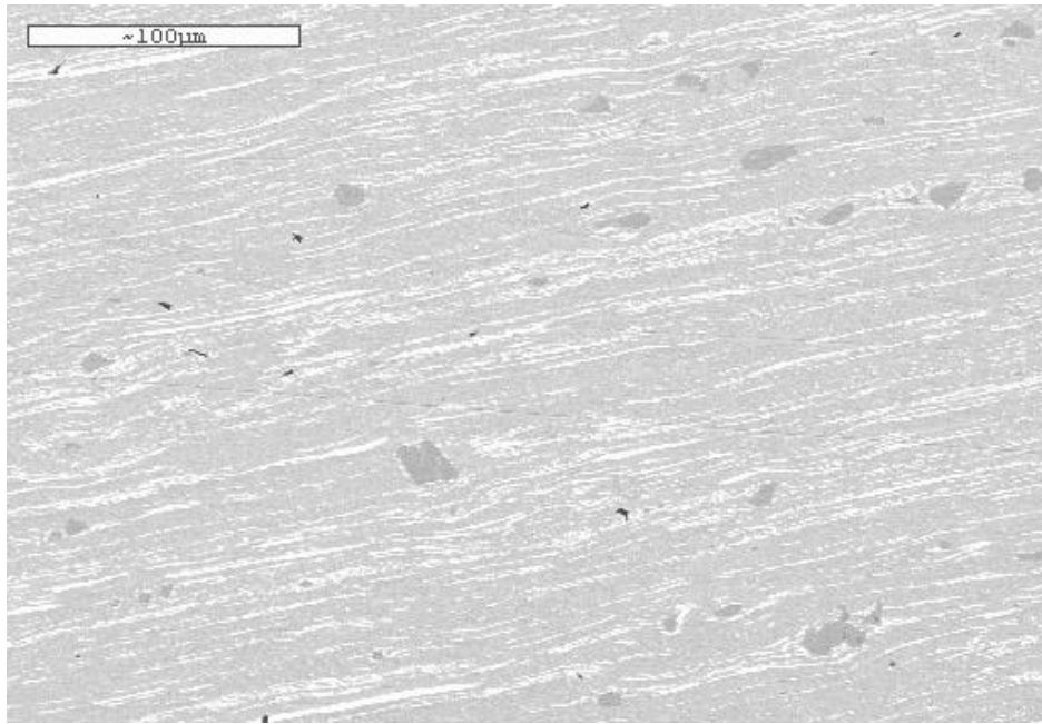
FIG. 2.3 – Micrographie du \text{Ni}_{47}\text{Ti}_{44}\text{Nb}_9 dans le sens longitudinal - Échelle 100\ \mu\text{m}
