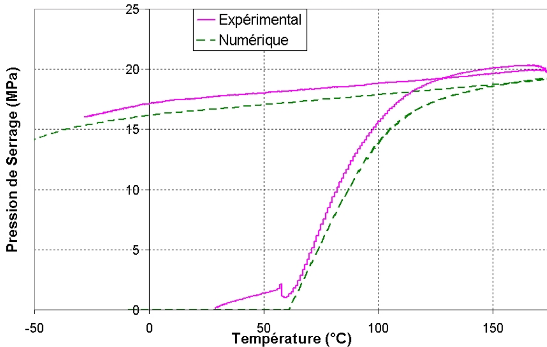
FIG. 4.24 – Comparaison expérimental/numérique de la simulation de la bague fine
