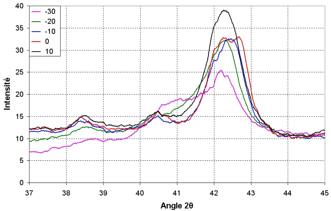
FIG. 2.19 – Disparition du pic de martensite en modifiant l'angle \chi
