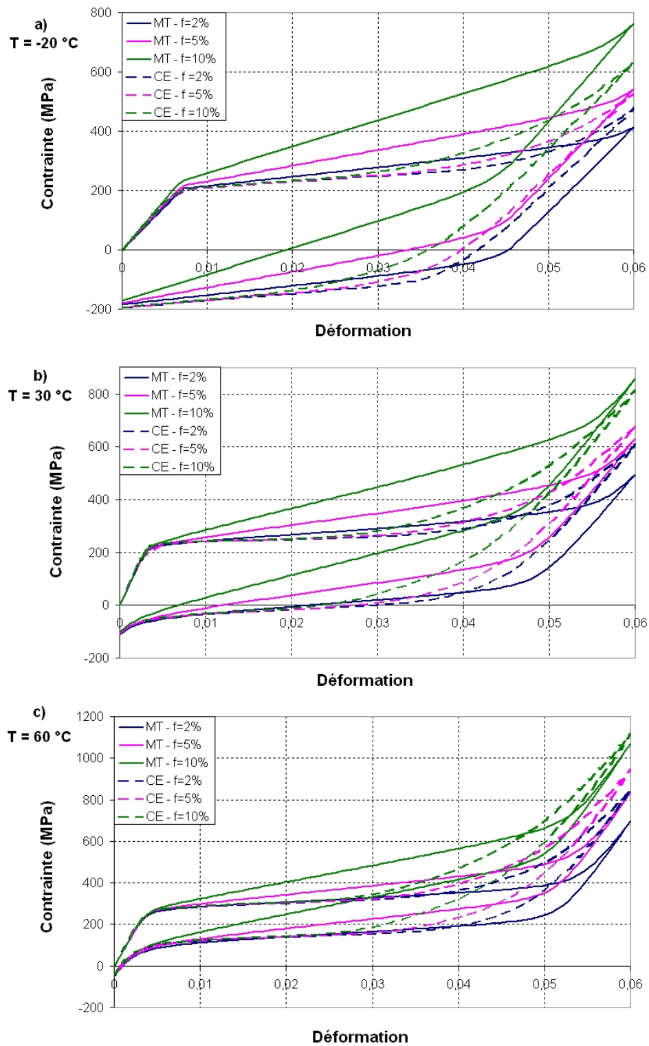
FIG. 5.7 – Comparaison de la réponse à un chargement homogène isotherme à -20 (a), 30 (b) et 60 °C (c) d'un matériau de type NiTi avec des précipités Ni_4Ti_3 , pour trois fractions d'inclusion ( f = 2, 5 et 10\% ), entre deux types de simulations : cellule élémentaire ("CE", en pointillés) et schéma de Mori-Tanaka ("MT", en traits pleins).
