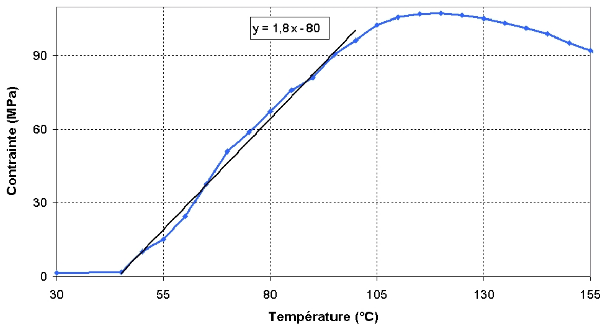
FIG. 2.26 – Évolution de la contrainte en fonction de la déformation lors du chauffage d'une bague S2, en bloquant le déplacement de son diamètre interne
