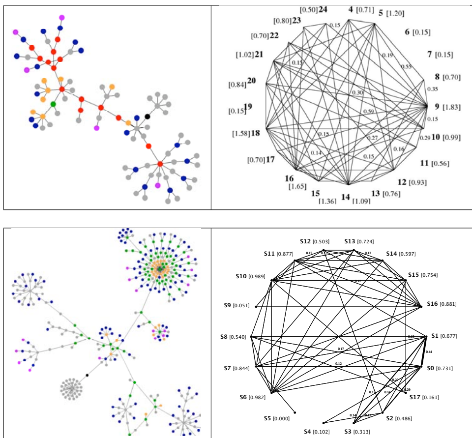
FIGURE 3.7 – Comparaison entre graphes de sites Web et graphes des documents. En haut à gauche le graphe du site Web sur l'ouragan Gilbert publié par le National Hurricane Center ( www.nhc.noaa.gov/1988gilbert.html ). En haut à droite, le graphe d'un document traitant aussi sur l'ouragan Gilbert (voir les annexes, section A.2). En bas à gauche le graphe d'un site Web sur l'actualité au Tibet ( www.tibet-info.net/www/index.php ). En bas à droite le graphe d'un cluster de trois articles journalistiques sur le même sujet (voir le document dans les annexes A.3).
