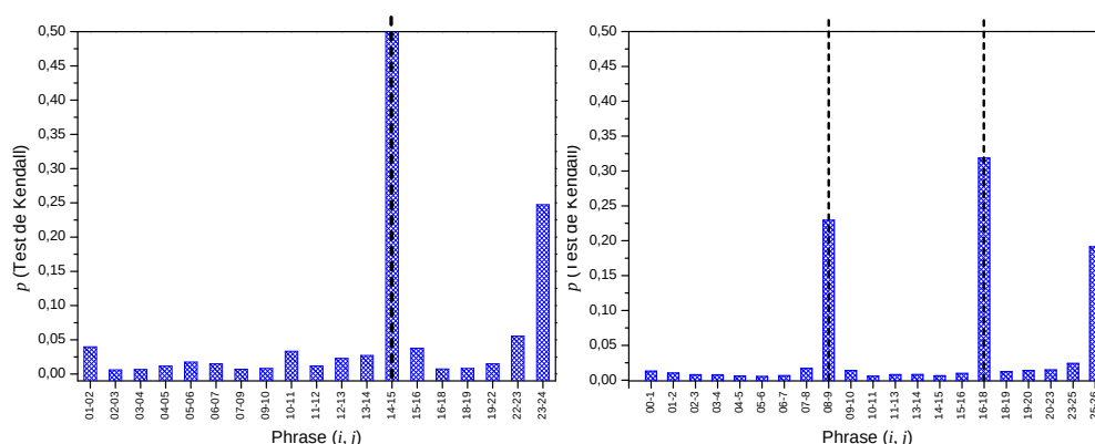
FIGURE 5.2 – Détection des frontières pour le texte 2-mélanges (deux thématiques, à gauche) et 3-mélanges (trois thématiques, à droite). Une p -value > 0,1 indique la présence d'une rupture thématique.
