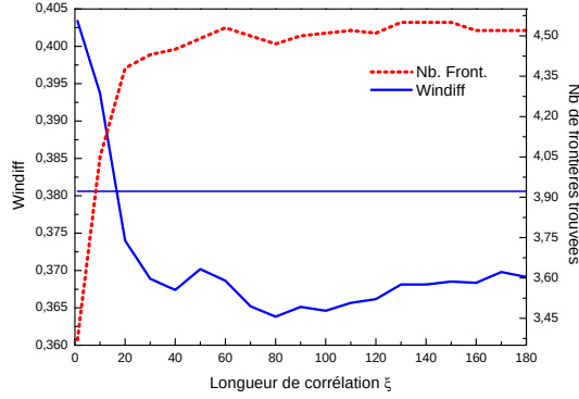
FIGURE 5.8 – Évolution de WD et du nombre de frontières en fonction de \xi . La ligne horizontale représente la valeur de WD à longueur de corrélation infinie. Taille des segments entre 6 et 8 phrases pour le corpus en français.
