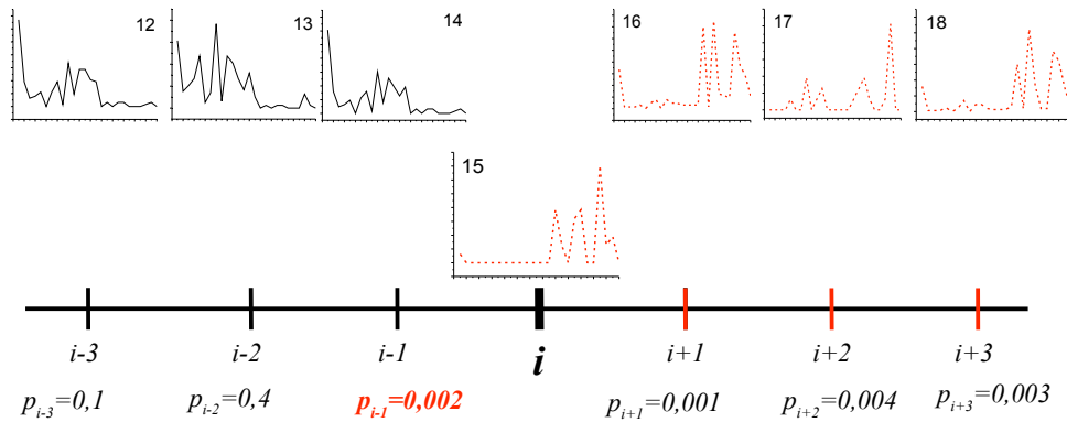
FIGURE 5.4 – Test \tau -Kendall en fenêtre ; p_{i \pm k} = probabilité de se tromper avec l'hypothèse que i \pm k et i appartient au même segment thématique (c'est à dire d'accepter H_1 quand H_0 est vraie) ; pred = nombre de phrases parmi les 3 qui précèdent à i qui ne sont pas concordants avec elle ( p > 0,01 ), et succ = nombre de phrases parmi les 3 suivants à i qui sont concordants avec elle ( p < 0,01 ). Si pred(i) > 2/3 et succ(i) > 2/3 , alors i est une frontière.
