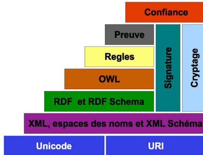
FIG. 2.9 – Le gâteau du Web sémantique
