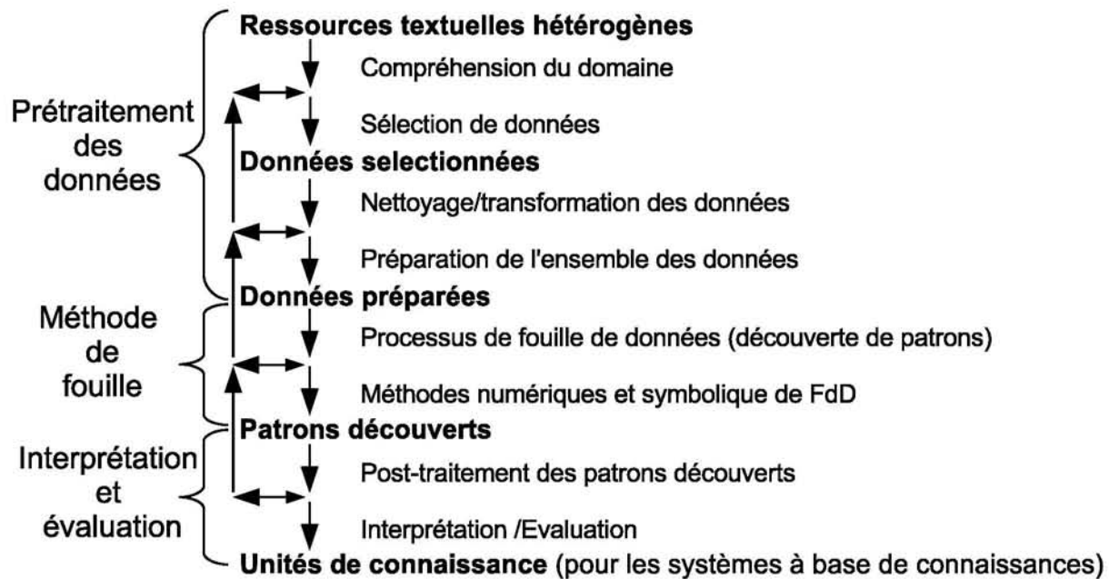
FIG. 3.1 – Le processus d'extraction de connaissances à partir de données : des données aux connaissances
