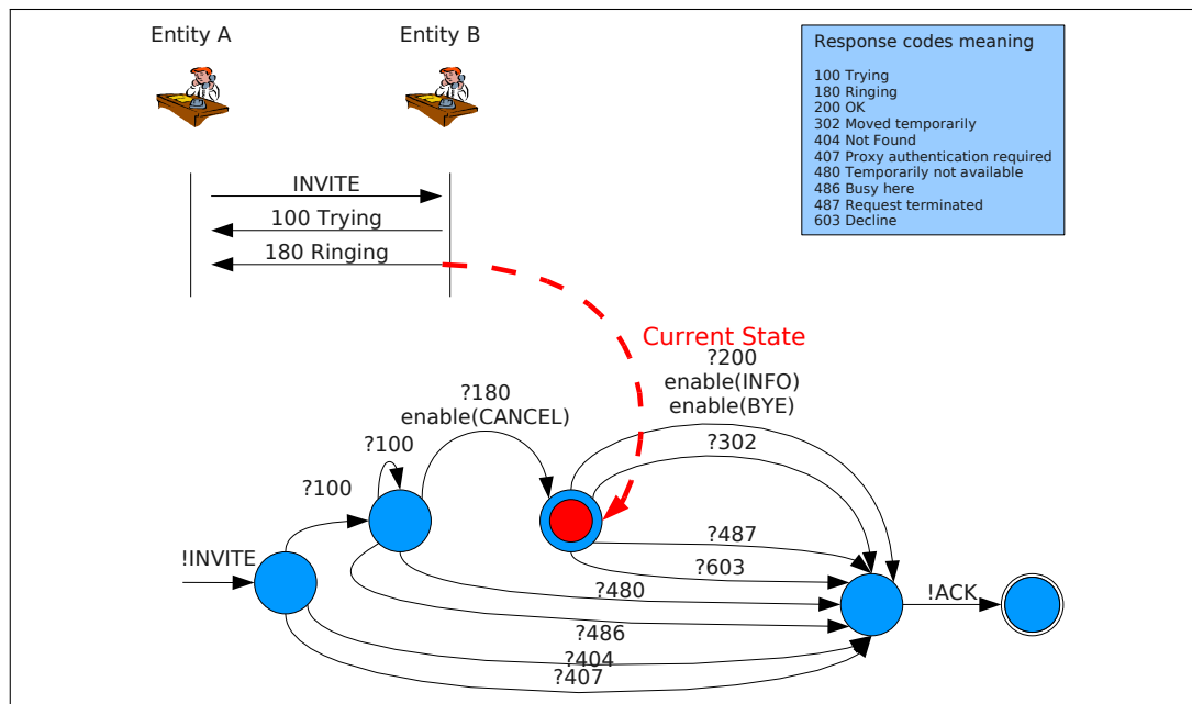
Figure 5: Automate de fonctionnement appris à partir d'un message INVITE Les transitions marquées (?) indiquent que les messages correspondent à l'entité qui répond. Le marquage (!) indique que les messages proviennent de l'entité cliente.
