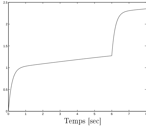
FIG. 2.27: Entrée u_1(t)
