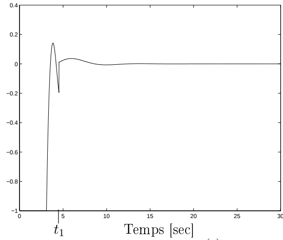
FIG. 3.33: Entrée u(t)
