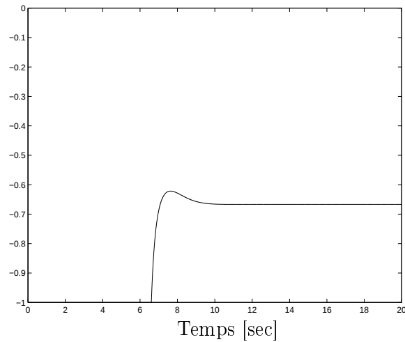
FIG. 3.20: Entrée u(t) : \delta = 10
