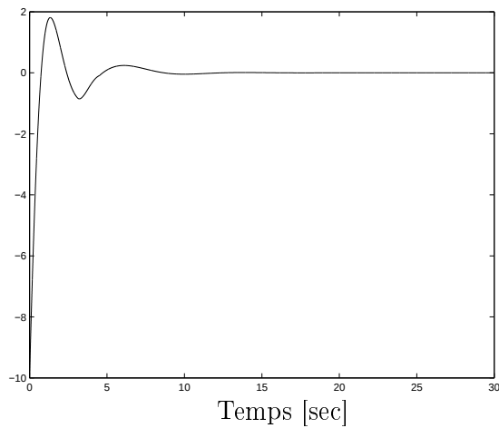
FIG. 3.37: Etats x_2(t)
