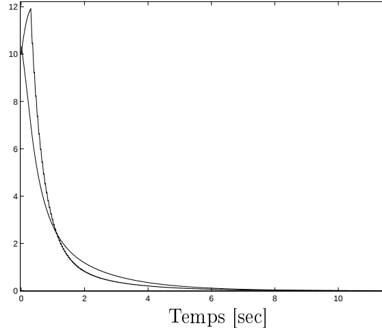
FIG. 3.19: Etats x_1(t) et x_2(t)
