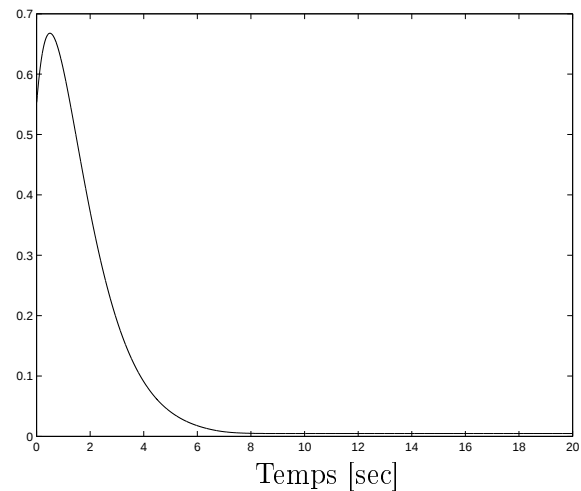
FIG. 3.21: Erreur d'observation e_1(t) : \delta = 10
