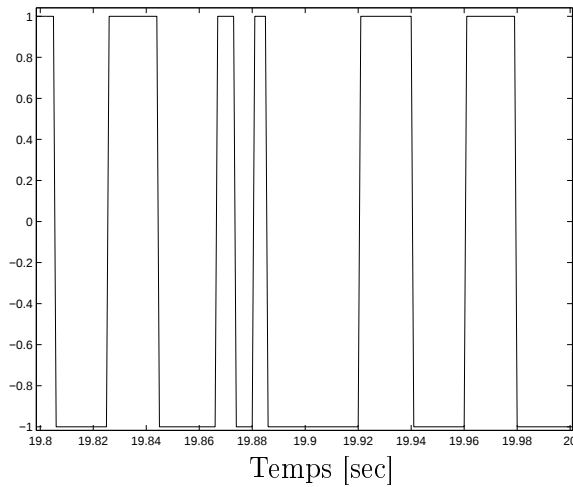
FIG. 3.17: Entrée u_2(t)
