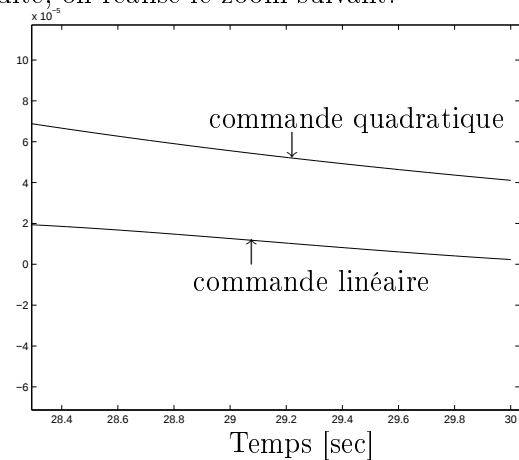
FIG. 3.42: Etats x_2(t)
