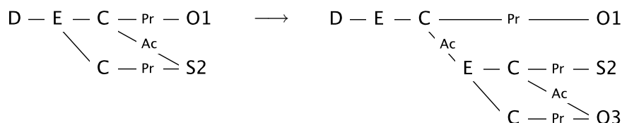
FIG. 8.18 – otherReject après O_3
