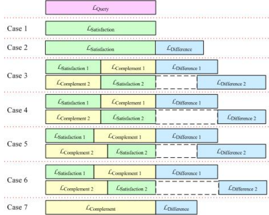
FIG. 9 – Cas d’une réponse composée limitée à deux fragments de réponse
