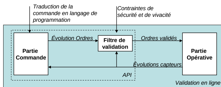
Figure 41 Filtre de sécurité, schéma de principe (Marangé et al, 2007)
