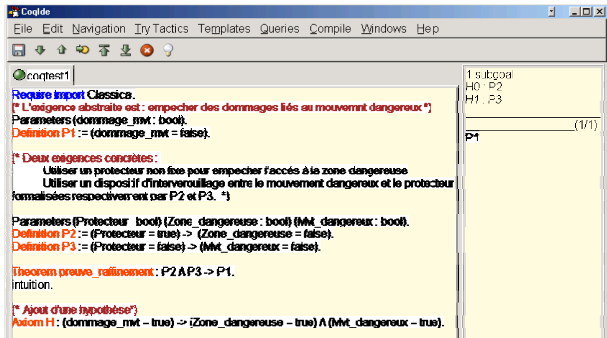
Figure 38 Preuve réalisée avec l'assistant de preuve COQ
