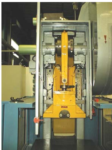
Vue de face du coulisseau/bielle
