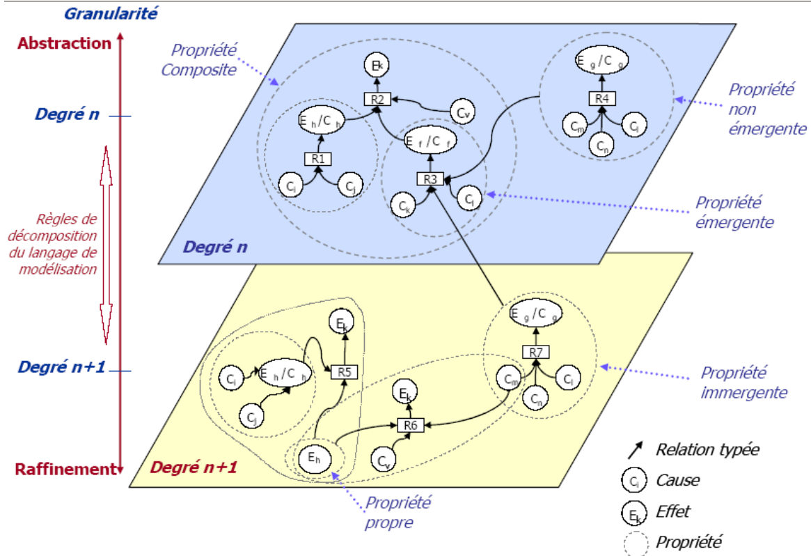
Figure 25 Types de propriétés définis par le modèle CREDI (Chapurlat, 2007)
