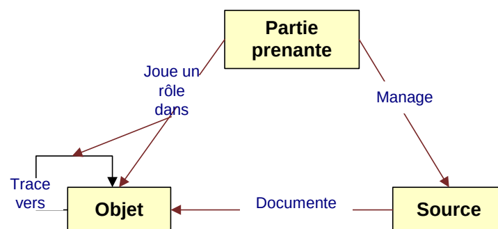
Figure 29 Méta modèle de la traçabilité (Ramesh et Jarke, 2001)
