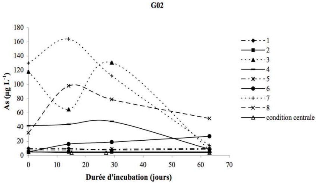
Figure 184 : Cinétiques de solubilisation de As pour G02 en fonction des 8 expériences non centrales et des 3 expériences en conditions centrales.
