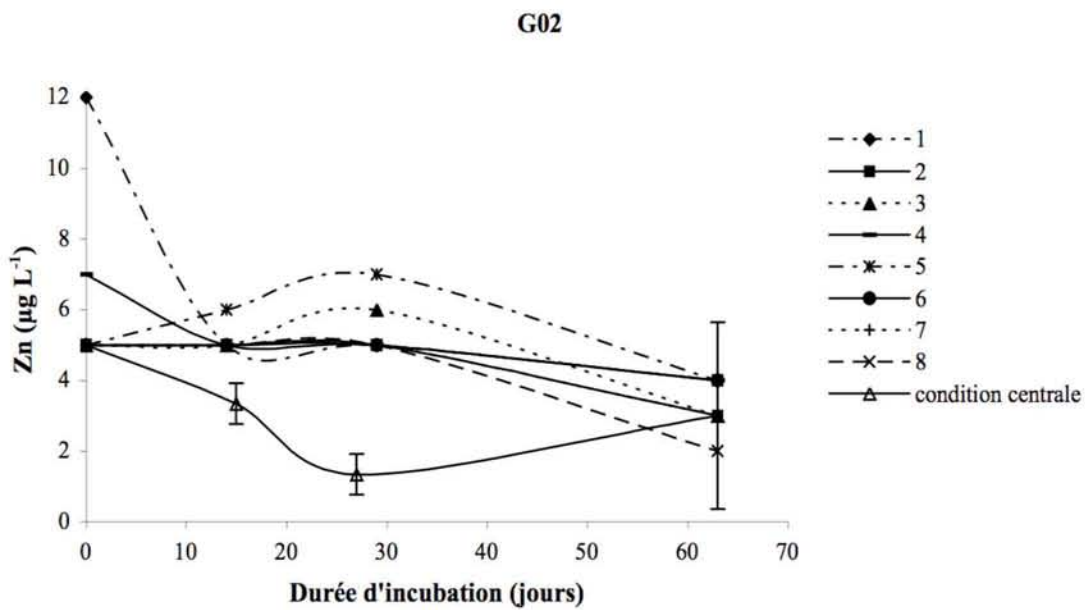
Figure 185 : Cinétiques de solubilisation de Zn pour G02 en fonction des 8 expériences non centrales et des 3 expériences en conditions centrales.
