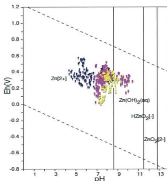
Figure 99 : Estimation de la spéciation de Zn dans le système Zn-O-H ( 10^{-10} \text{ mol.kg}^{-1} et conditions standards de température et pression, Takeno, 2005) d'après le pH et Eh mesurés pour les échantillons De Plateaux-Hageven (bleu), Flémalle (rose) et Gallego (jaune).
