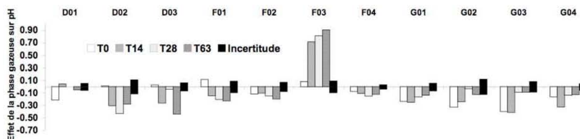
Figure 92 : Effets de la « Composition de la phase gazeuse » sur pH.
