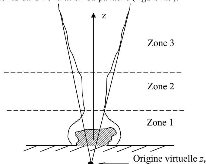
Figure 2.5 : Description en trois zones d'un panache développé au-dessus d'une source non ponctuelle et notion de l'origine virtuelle (d'après Kofoed et Nielsen [10])
