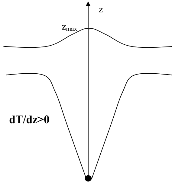
Figure 2.4 : Schéma d'un panache dans un milieu à variation linéaire de température (D'après Kofoed et Nielsen [10]).
