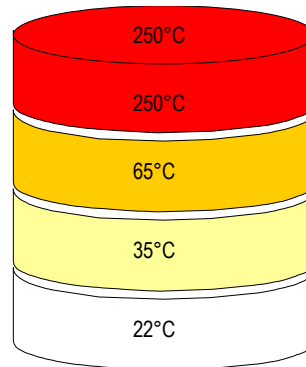
Figure 4.4 : configuration de la source pour le cas 2
