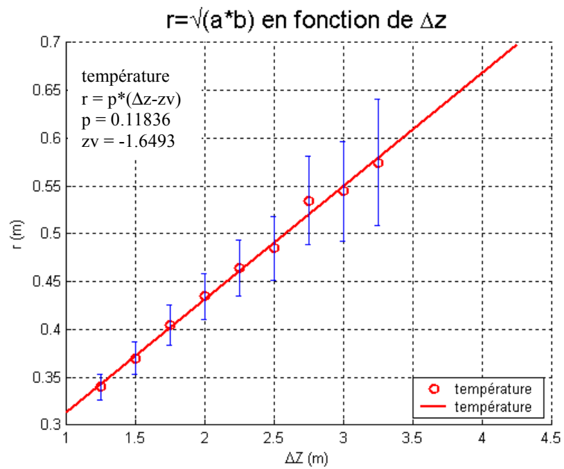
Figure 5.22 : Evolution des rayons thermiques - Comparaison des origine virtuelles : cas 3
