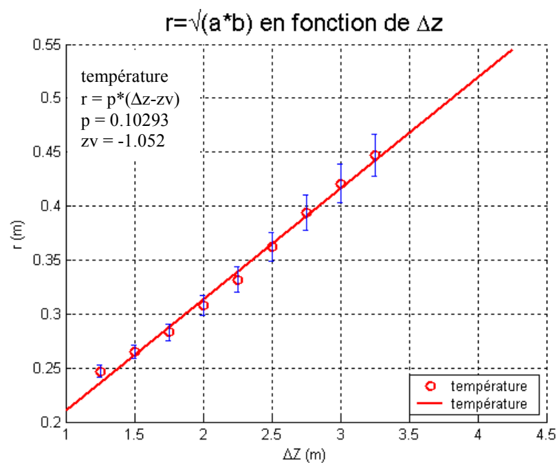
Figure 5.20 : Evolution des rayons thermiques - Comparaison des origines virtuelles : cas 1
