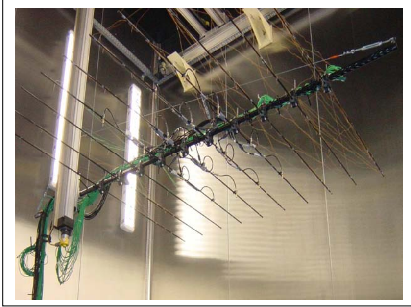
figure 3.8 : matrice de capteurs
