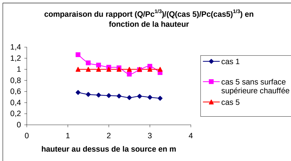
figure 5.17 : comparaison du rapport débit/puissance convectée entre un cas étudié et le cas référence pour plusieurs cas de sources rectangulaires
