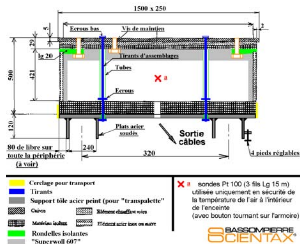
figure 3.6 : schéma d'un des quatre modules constituant la source rectangulaire
