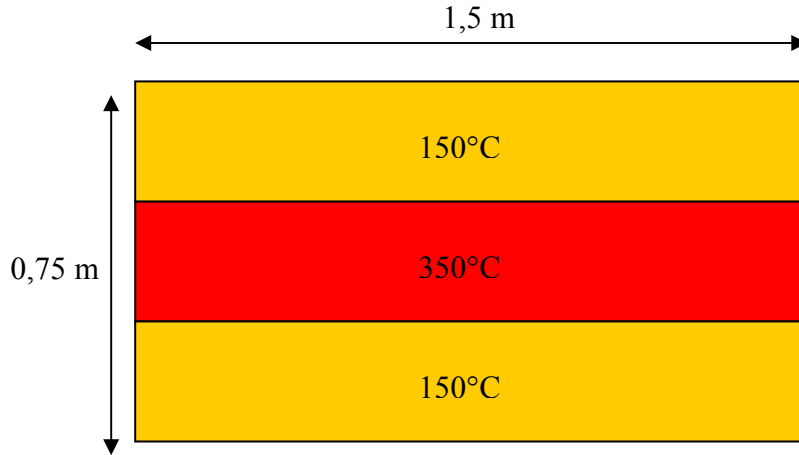
figure 5.65 : configuration de 3 sources rectangulaires (vue de dessus) : T=150^{\circ}\text{C} , T=350^{\circ}\text{C} , T=150^{\circ}\text{C} .
