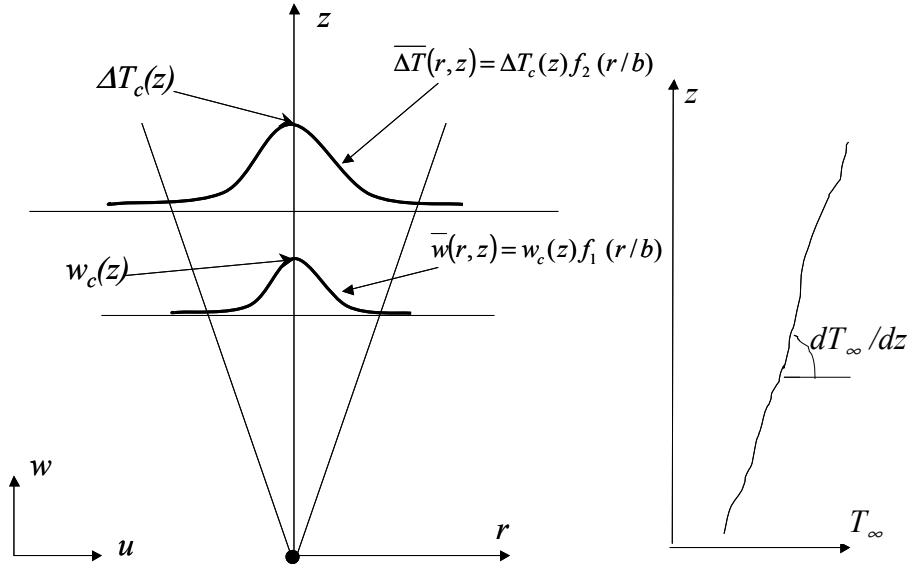
Figure 2.2 : Représentation schématique d'un panache axisymétrique
