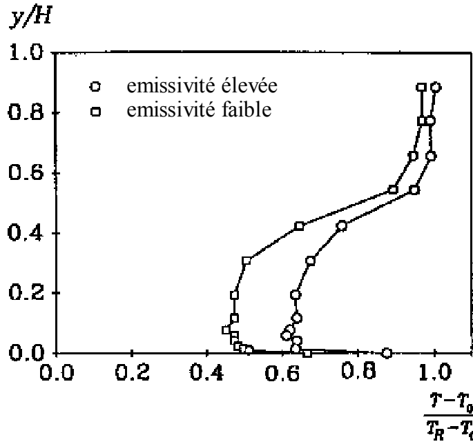
Figure 2.6 : Influence de l'émissivité de la source sur le profil vertical de température (d'après Nielsen [24])
