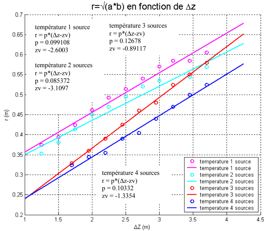
Figure 5.44 : Evolution des rayons thermiques en fonction de z - Comparaison des origine virtuelles
