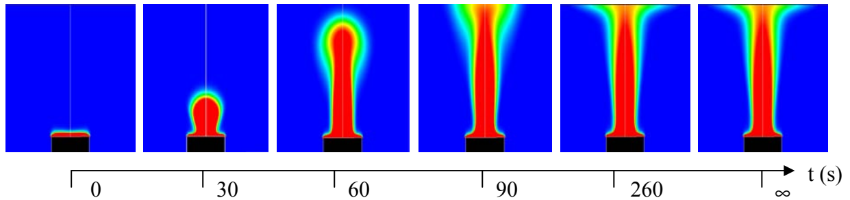
Figure 2.15 : Evolutions du champ de température de l'air environnant dans une enceinte ventilée ( Q_v=10000\text{m}^3/\text{h} ) cylindrique ( R=2.5\text{m} et H=5\text{m} ) avec une source thermique de 1.54\text{m} de diamètre à 200^\circ\text{C}
