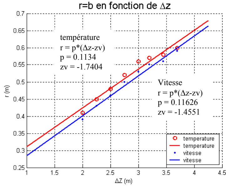
Figure 5.48 : Evolution des rayons thermiques et dynamiques en fonction de z > 2m - Comparaison des origine virtuelles : 1 source
