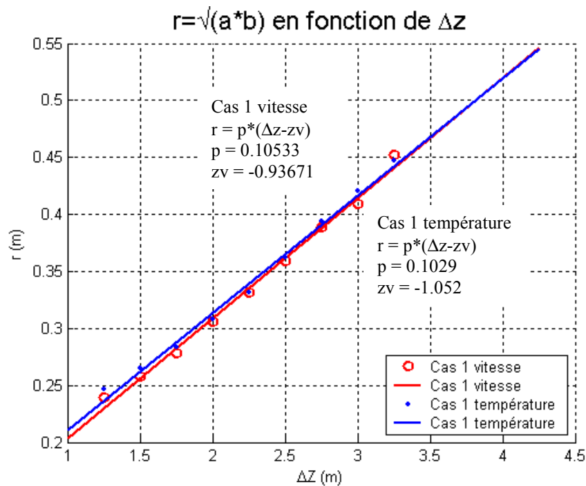
Figure 5.6 : Evolution des rayons thermiques et dynamiques en fonction de z - Comparaison des origine virtuelles : cas 1
