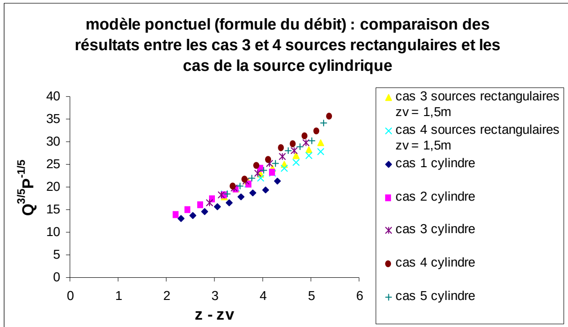
figure 5.72 : modèle ponctuel : comparaison des résultats entre les cas 3 et 4 sources rectangulaires et les cas de la source cylindrique à partir de la formule du débit Q(z) = 0,005 \cdot P_c^{1/3} (z - z_v)^{5/3}
