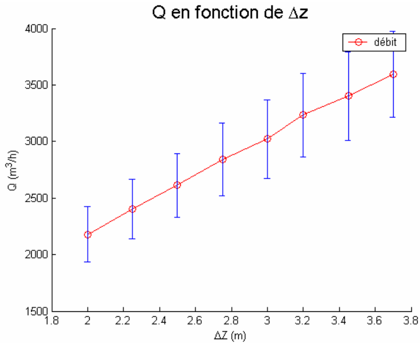
figure 5.60 : débit en fonction de la hauteur z – barres d'erreur : cas 1 source
