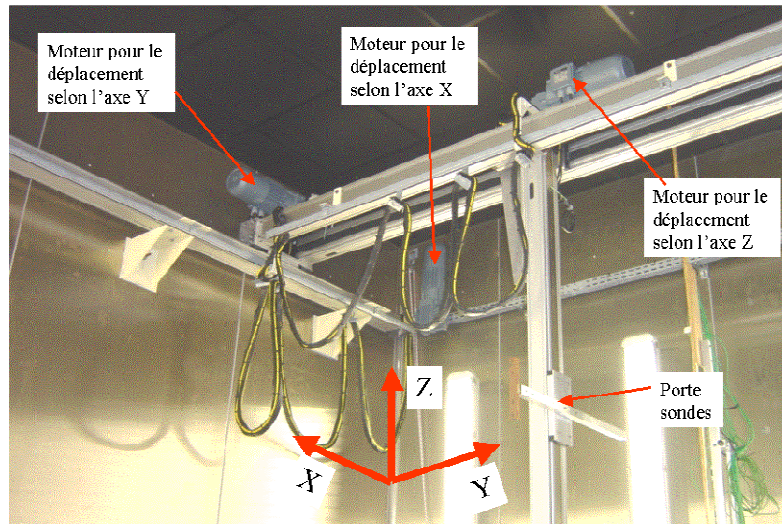
Figure 3.4 : Système de déplacement 3D installé dans la chambre d'essai
