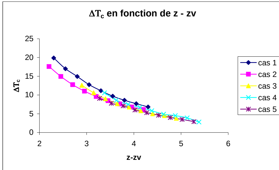
figure 5.13 : Evolution de la température au centre du panache en fonction de z-z_v pour les cinq cas étudiés
