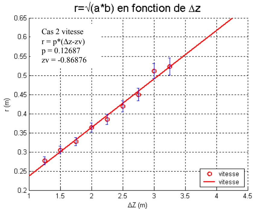
Figure 5.26 : Evolution des rayons dynamiques - Comparaison des origine virtuelles : cas 2
