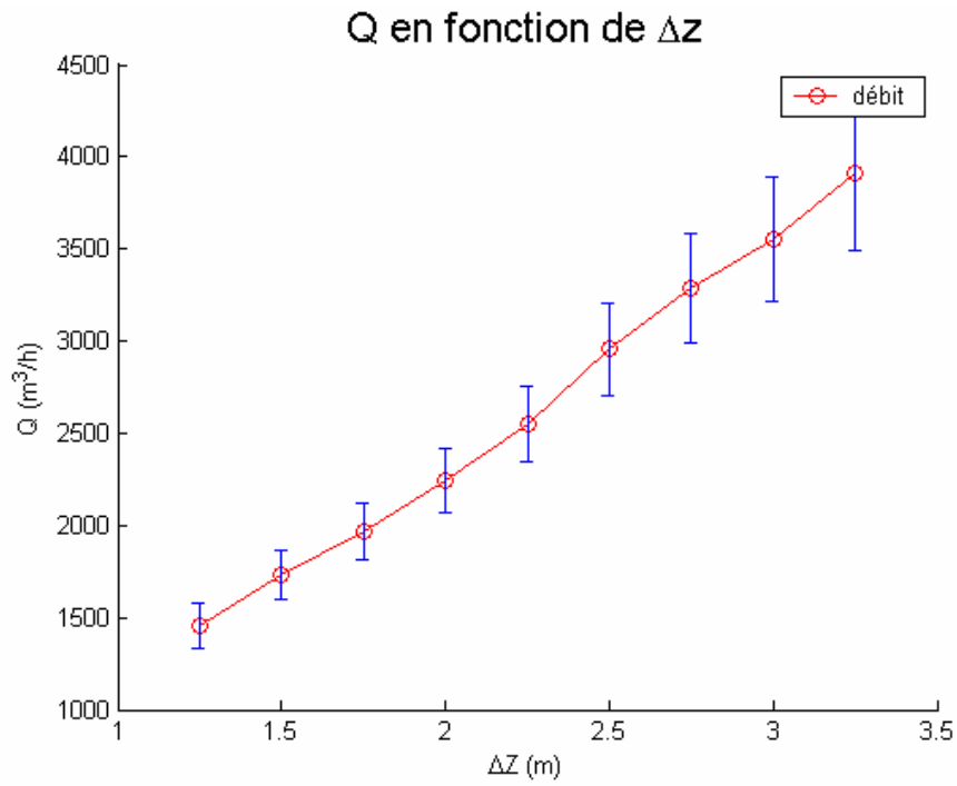
figure 5.32 : débit expérimental en fonction de \Delta z - incertitude pour le cas 3
