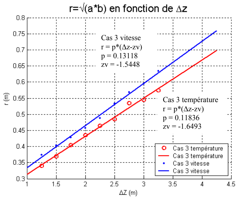
Figure 5.8 : Evolution des rayons thermiques et dynamiques en fonction de z - Comparaison des origine virtuelles : cas 3
