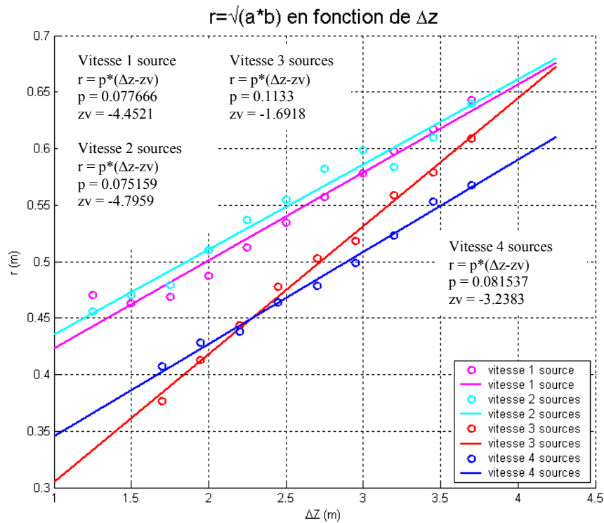
Figure 5.45 : Evolution des rayons dynamiques en fonction de z - Comparaison des origine virtuelles
