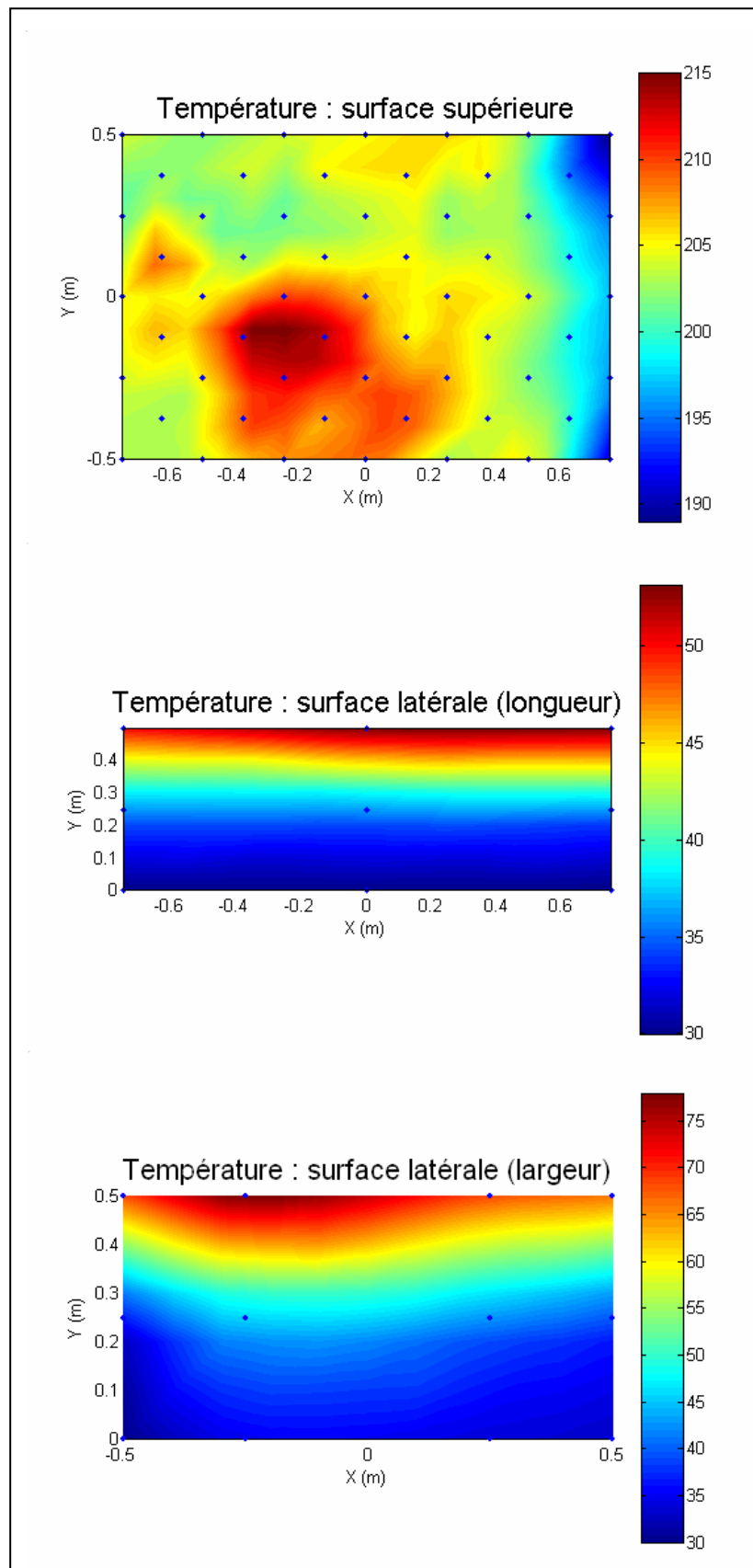
Figure 4.8 : Températures de surfaces de la source rectangulaire Distribution de température sur la surface supérieure de la source rectangulaire et sur les parois latérales selon un plan.
