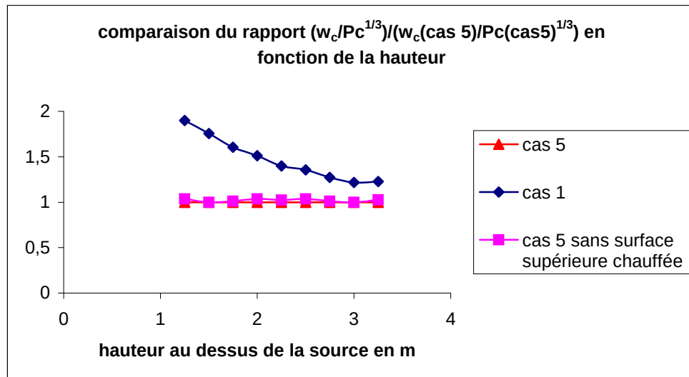
figure 5.19 : comparaison du rapport w_c /puissance convectée entre un cas étudié et le cas référence pour plusieurs cas de sources rectangulaires
