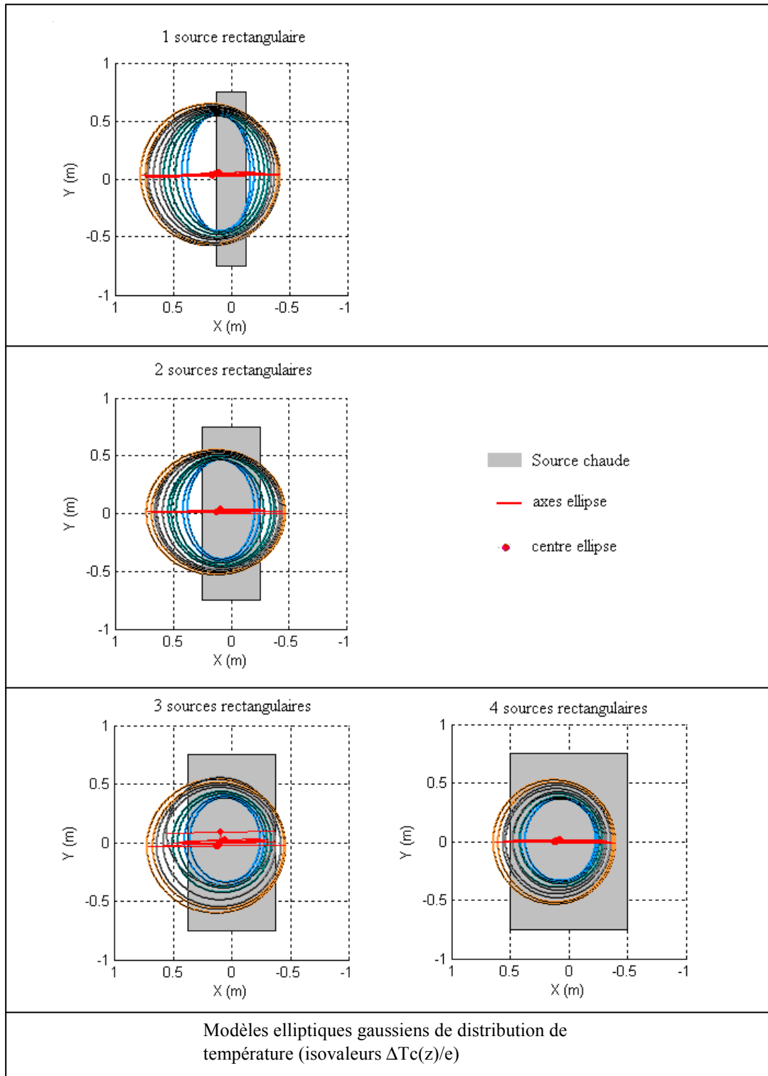
Figure 5.40 : modèles elliptiques (isothermes \Delta T_c(z)/e ) obtenus pour 1, 2, 3 et 4 sources rectangulaires
