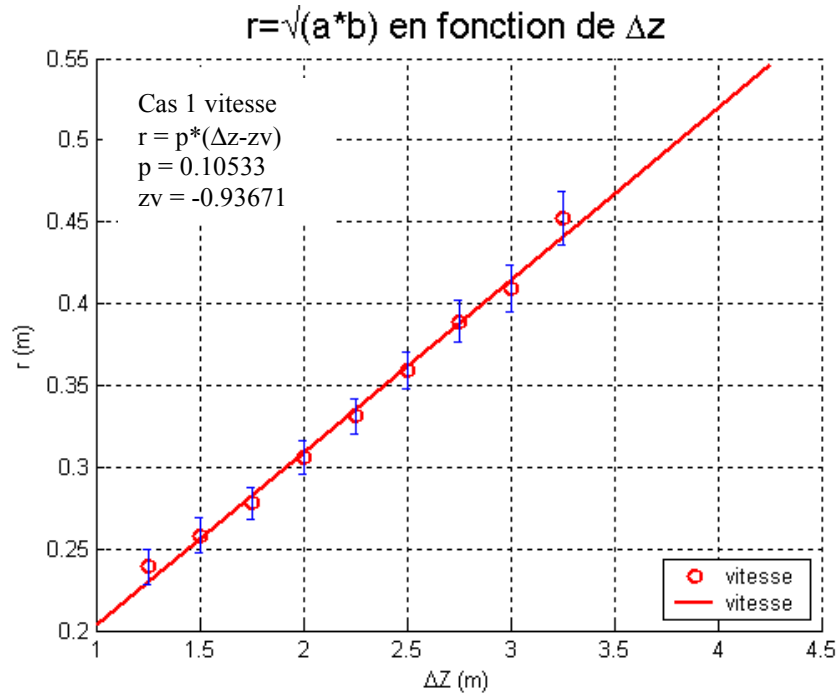
Figure 5.25 : Evolution des rayons dynamiques - Comparaison des origine virtuelles : cas 1
