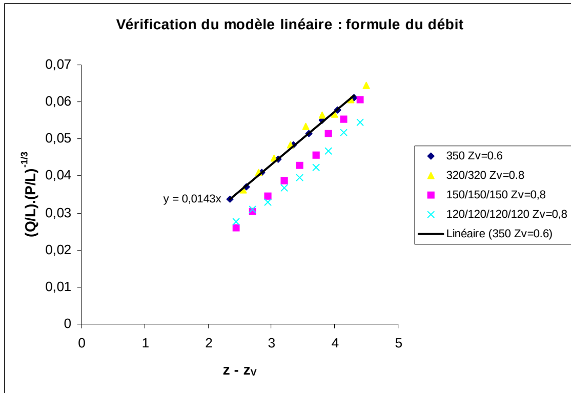
figure 5.50 : vérification du modèle linéaire à partir de la formule du débit
