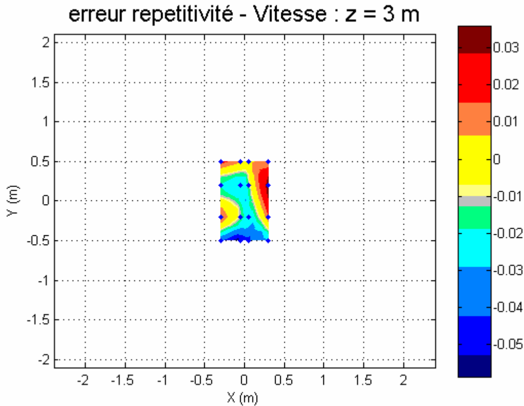
figure 7 : différence de vitesse entre deux séries de mesures à z = 3 m – 1 source
