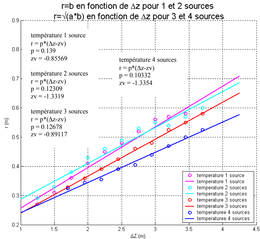
Figure 5.46 : Evolution des rayons thermiques en fonction de z ( r = b pour 1 et 2 sources et r = \sqrt{ab} pour 3 et 4 sources) - Comparaison des origine virtuelles
