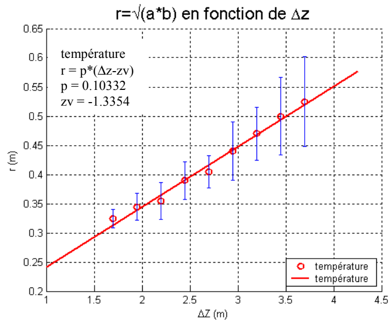
Figure 5.55 : Erreur de mesure sur le rayon thermique en fonction de z : cas 4 sources
