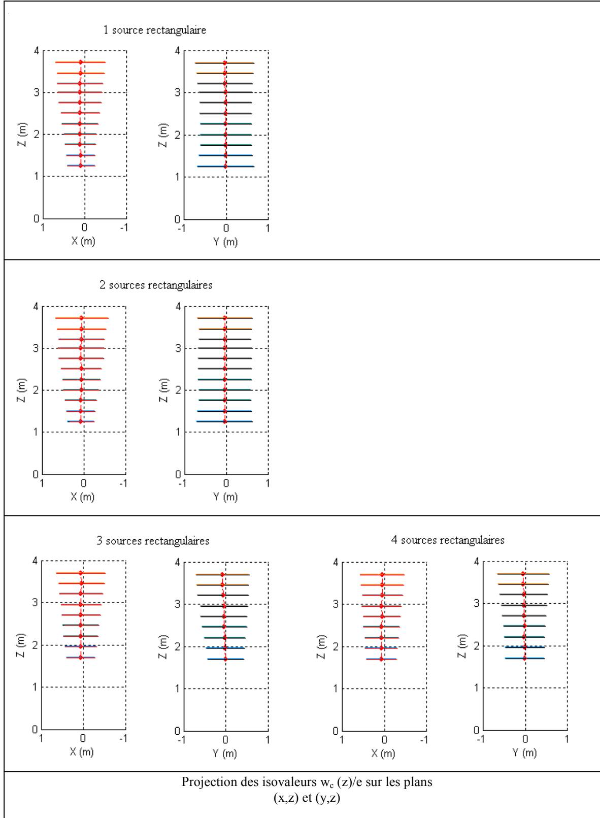
Figure 5.43 : projection des isovitesse w_c(z)/e sur les plans (x, z) et (y, z) obtenus pour 1, 2, 3 et 4 sources rectangulaires
