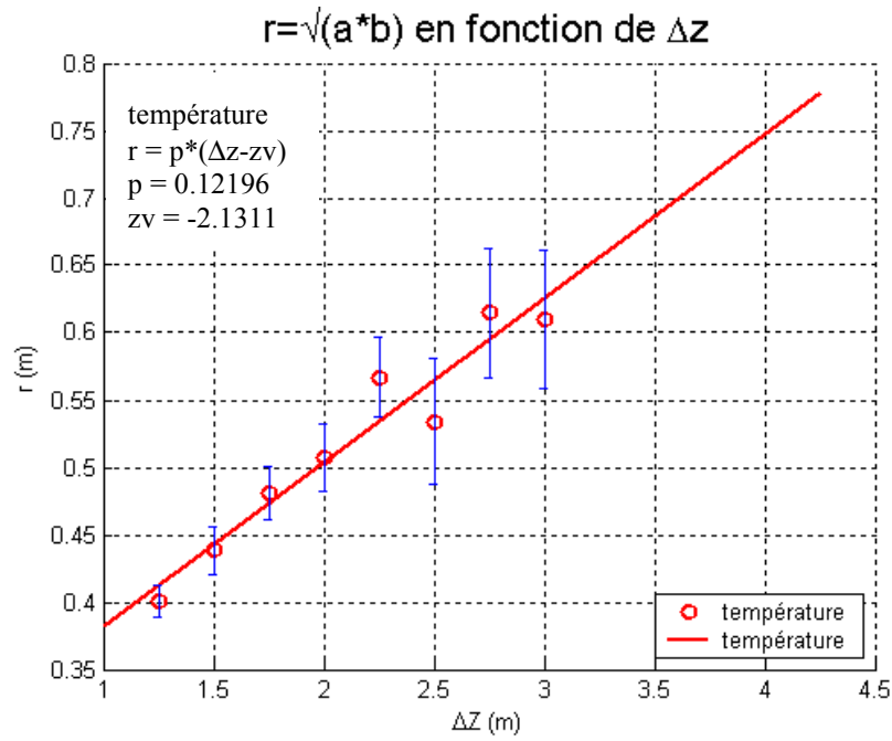
Figure 5.23 : Evolution des rayons thermiques - Comparaison des origine virtuelles : cas 4
