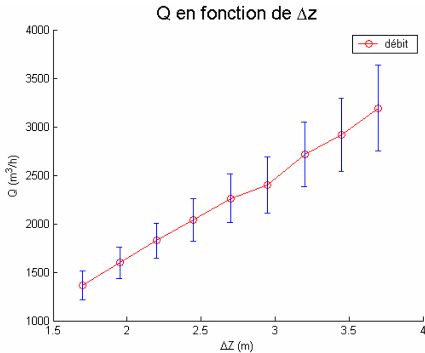
figure 5.62 : débit en fonction de la hauteur z – barres d'erreur : cas 3 sources
