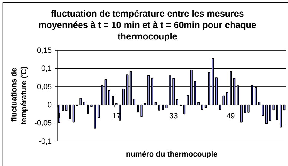
figure 1 : fluctuation de température entre les mesures moyennées à t = 10 min et à t = 60 min pour chaque thermocouple
