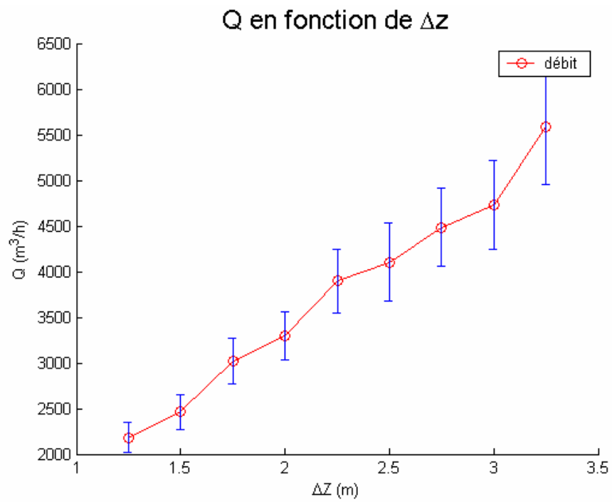
figure 5.33 : débit expérimental en fonction de \Delta z - incertitude pour le cas 4
