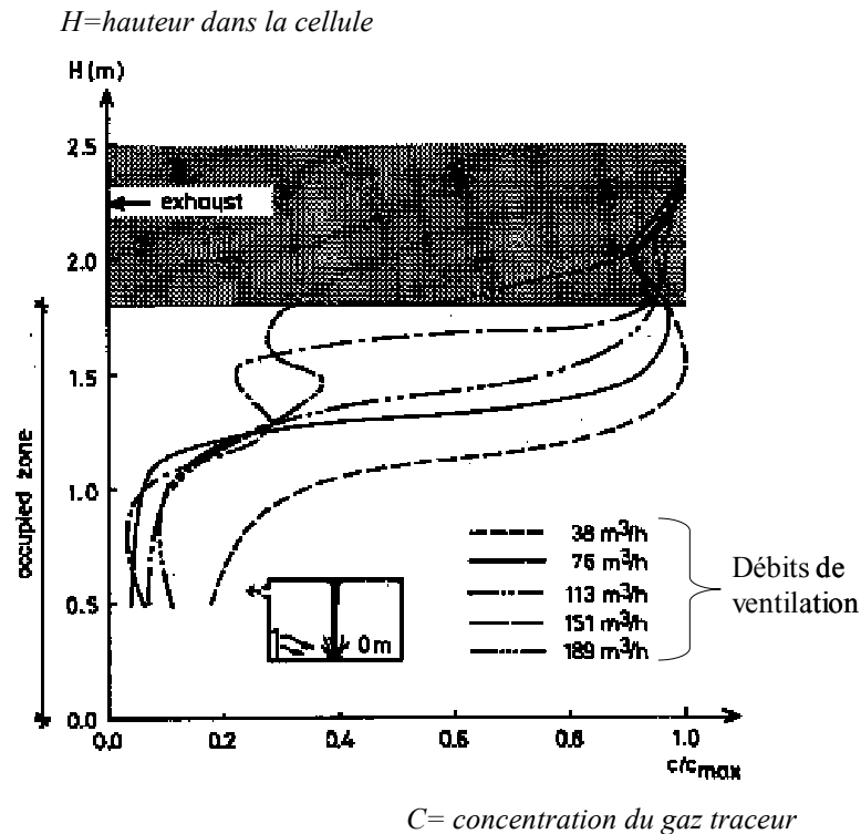
Figure 2.10 : Exemples de profils verticaux de concentration d'un gaz traceur mesurée en enceinte aéraulique pour différents débits de ventilation dans le cas d'un cylindre chauffé (d'après Heiselberg et Sandberg [31]).
