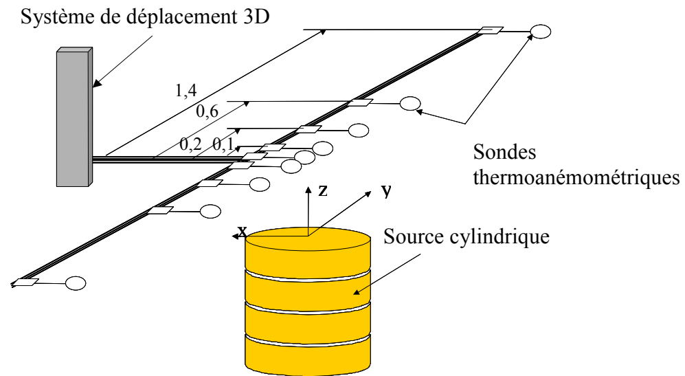
Figure 4.2 : Disposition des sondes thermoanémométriques
