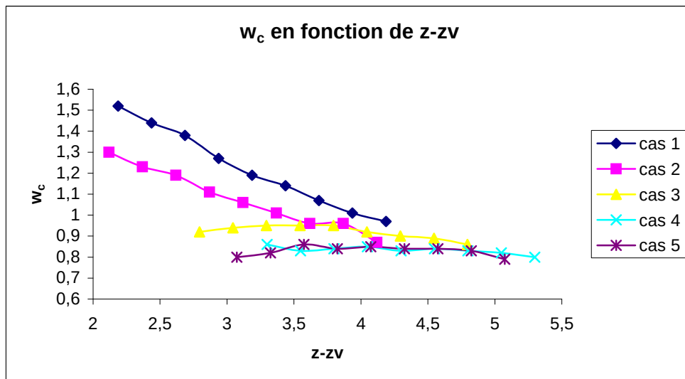
figure 5.14 : Evolution de la vitesse au centre du panache en fonction de z-z_v pour les cinq cas étudiés
