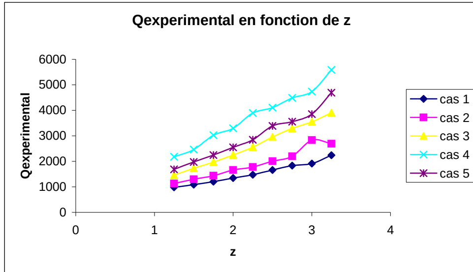
figure 5.12 : Evolution du débit d'air emporté par le panache en fonction de z pour les cinq cas étudiés
