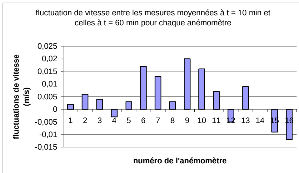
figure 2 : fluctuation de vitesse entre les mesures moyennées à t = 10 min et à t = 60 min pour chaque sonde de vitesse
