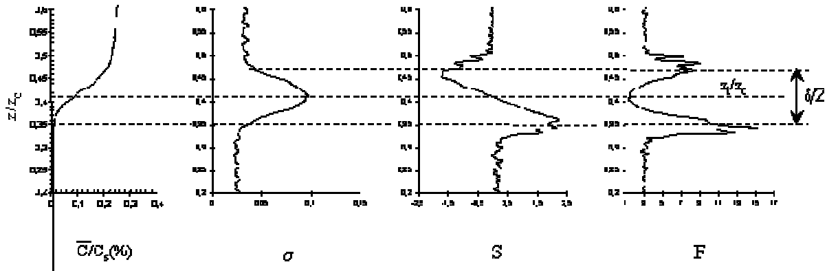
Figure 2.13 : Profils verticaux de concentration moyenne, d'écart type et des facteurs de dissymétrie et d'aplatissement des fluctuations de concentration du traceur fluorescent (d'après Auban [11] ; Auban et al. [42]).
