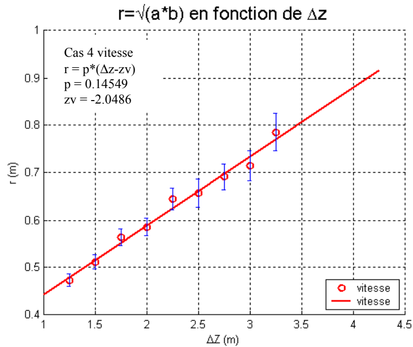
Figure 5.28 : Evolution des rayons dynamiques - Comparaison des origine virtuelles : cas 4
