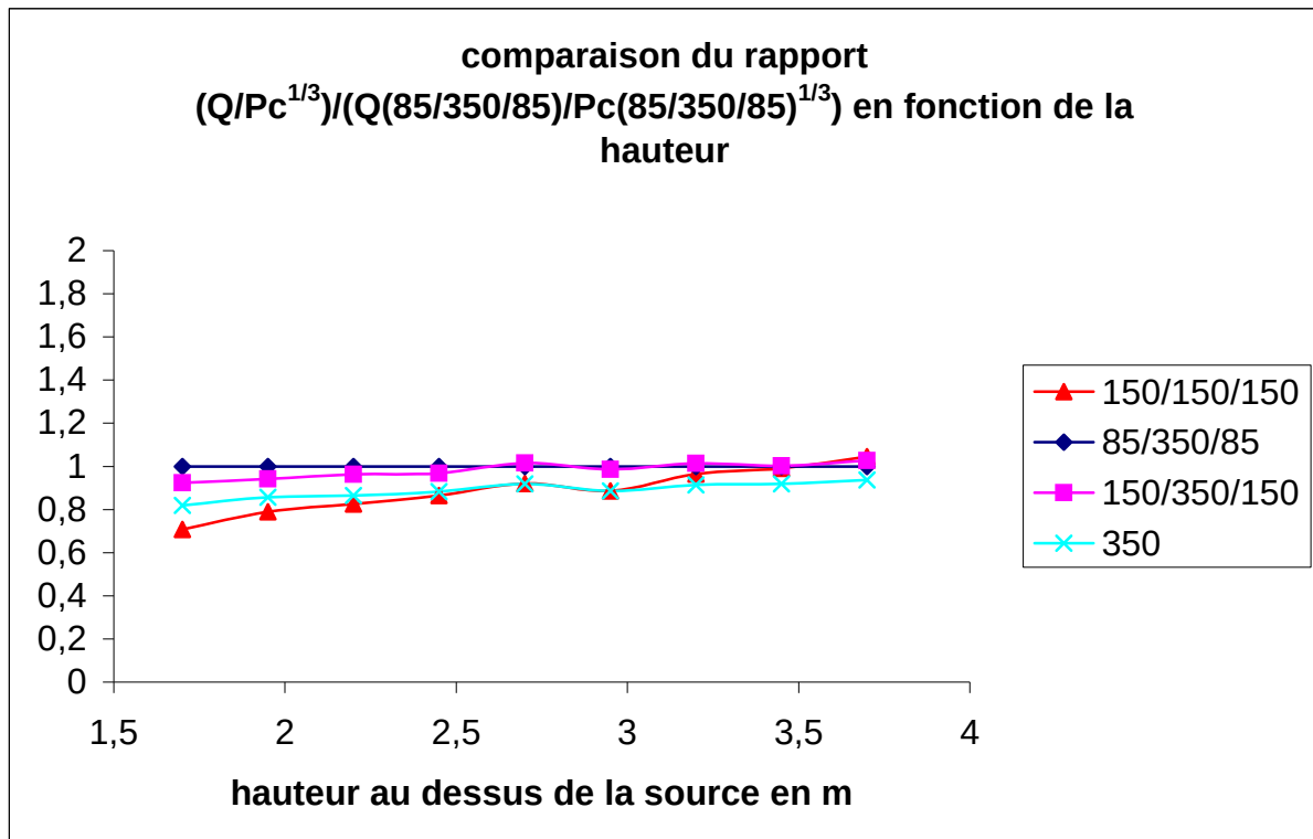
figure 5.68 : comparaison du rapport débit/puissance convectée entre un cas étudié et le cas référence pour plusieurs cas de sources rectangulaires référencés par leur température
