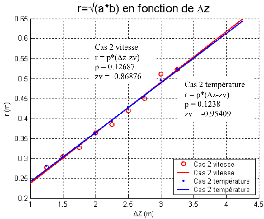
Figure 5.7 : Evolution des rayons thermiques et dynamiques en fonction de z - Comparaison des origine virtuelles : cas 2
