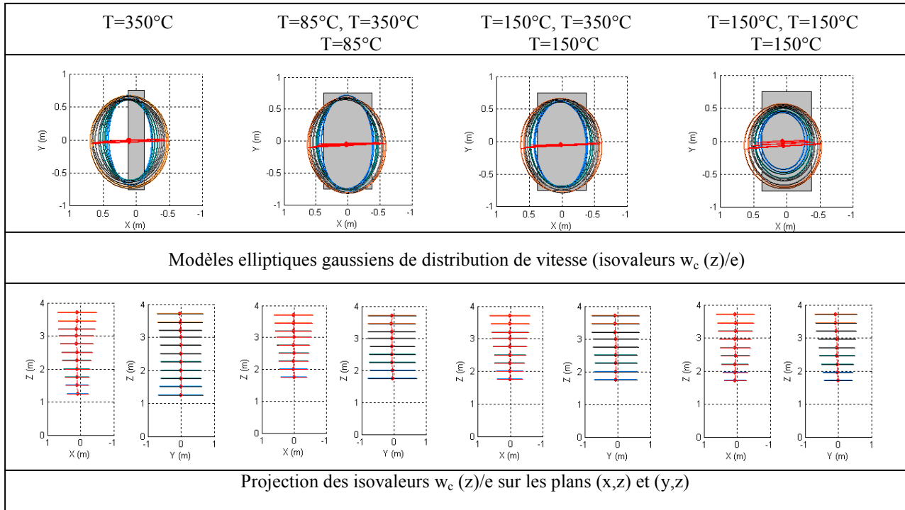
Figure 5.67: comparaison des modèles elliptiques (isovitesse w_c(z)/e ) sur les plans (x, y), (x, z) et (y, z) entre les quatre configurations
