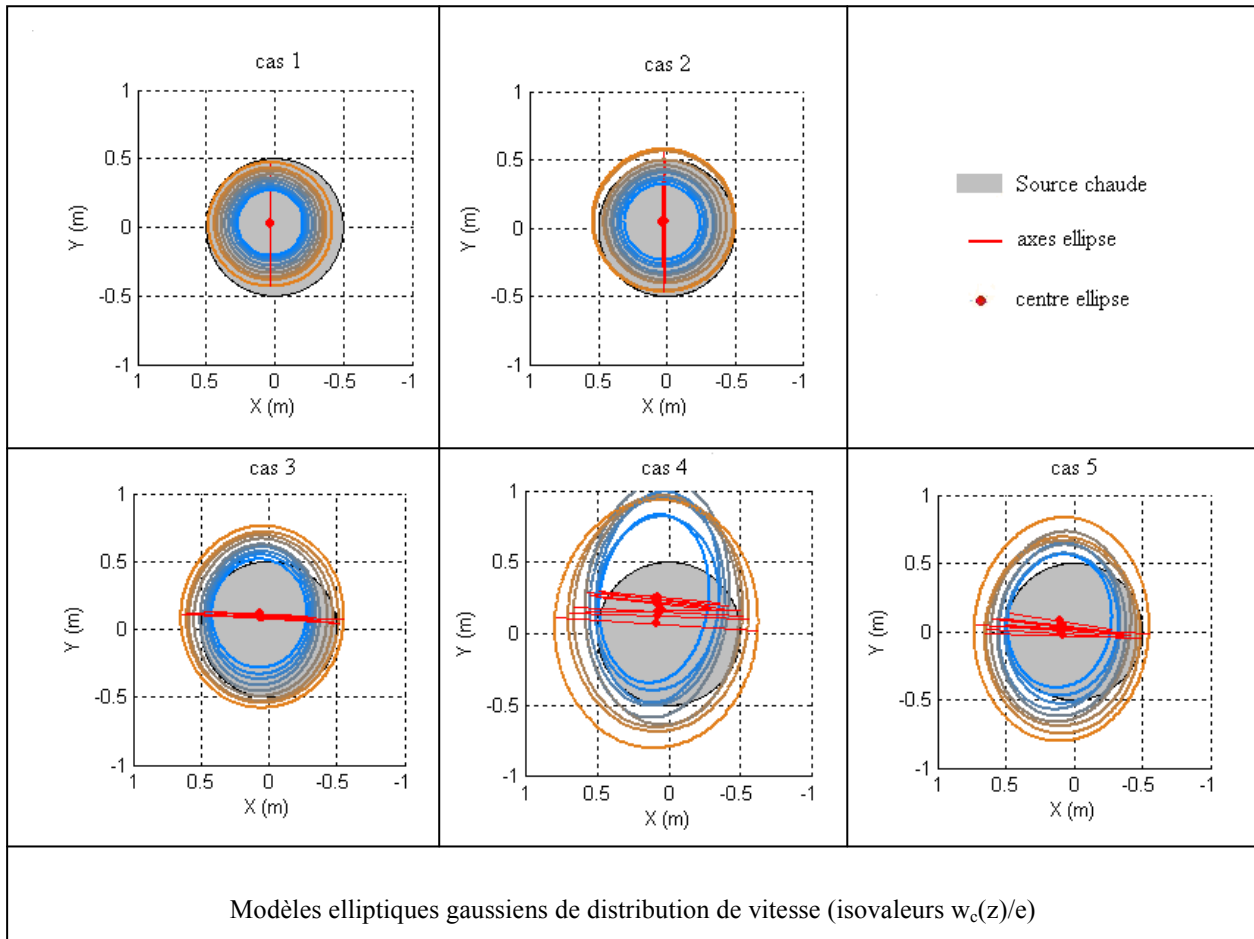
Figure 5.4 : Comparaison des modèles elliptiques (isovaleurs w_c(z)/e ) entre les cinq séries de mesure à z = 1,25, 1,50, 1,75, 2,25, 2,75 et 3,25 m
