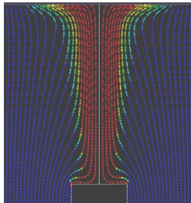
Figure 2.16 : Ligne de courant colorée en fonction de la température, alimentation du panache tout au long de son développement dans l'enceinte
