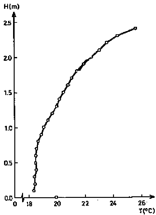
Figure 2.9 : Exemple de profil vertical de température mesurée en enceinte aéraulique dans le cas d'un cylindre chauffé (d'après Heiselberg et Sandberg [31])
