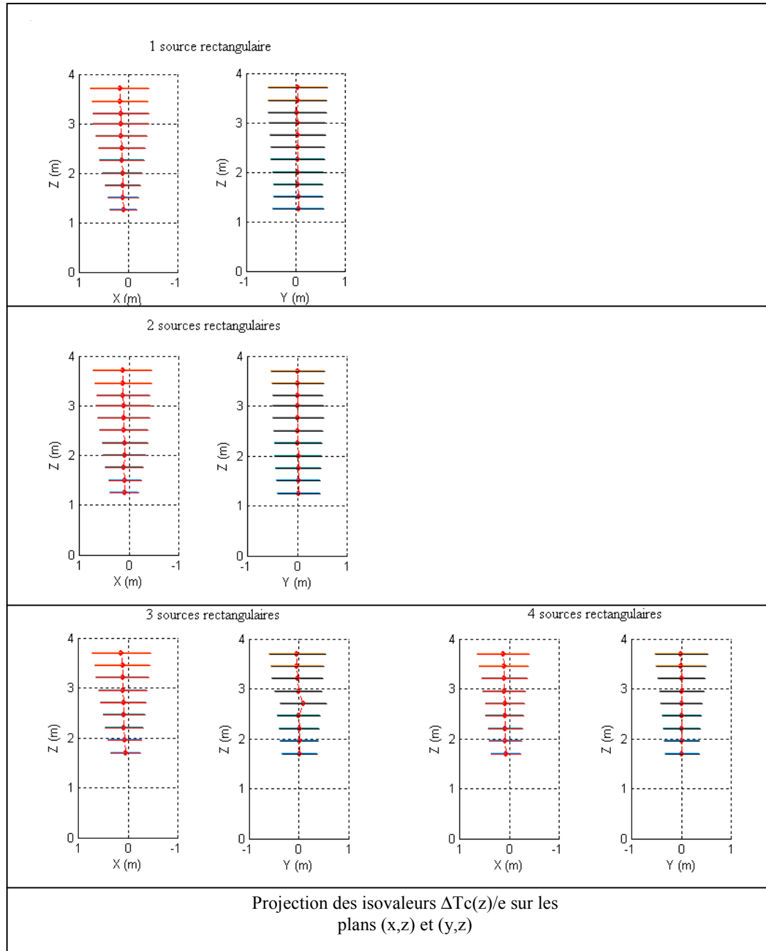
Figure 5.41 : projection des isothermes \Delta T_c(z)/e sur les plans (x, z) et (y, z) obtenus pour 1, 2, 3 et 4 sources rectangulaires
