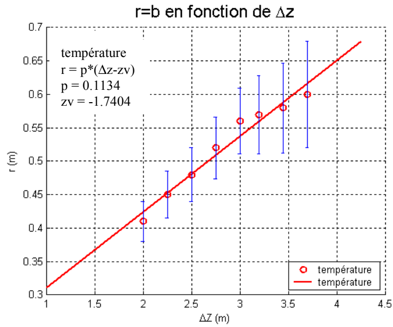
Figure 5.52 : Erreur de mesure sur le rayon thermique en fonction de z : cas 1 source
