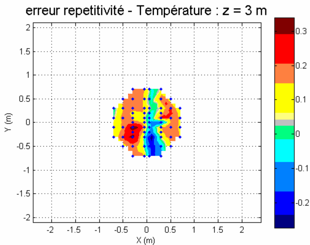
figure 5 : différence de température entre deux séries de mesures à z = 3 \text{ m} - 1 \text{ source}
