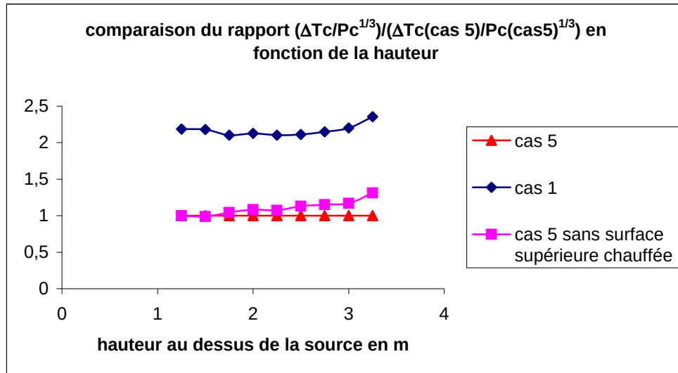
figure 5.18 : comparaison du rapport \Delta T_c /puissance convectée entre un cas étudié et le cas référence pour plusieurs cas de sources rectangulaires
