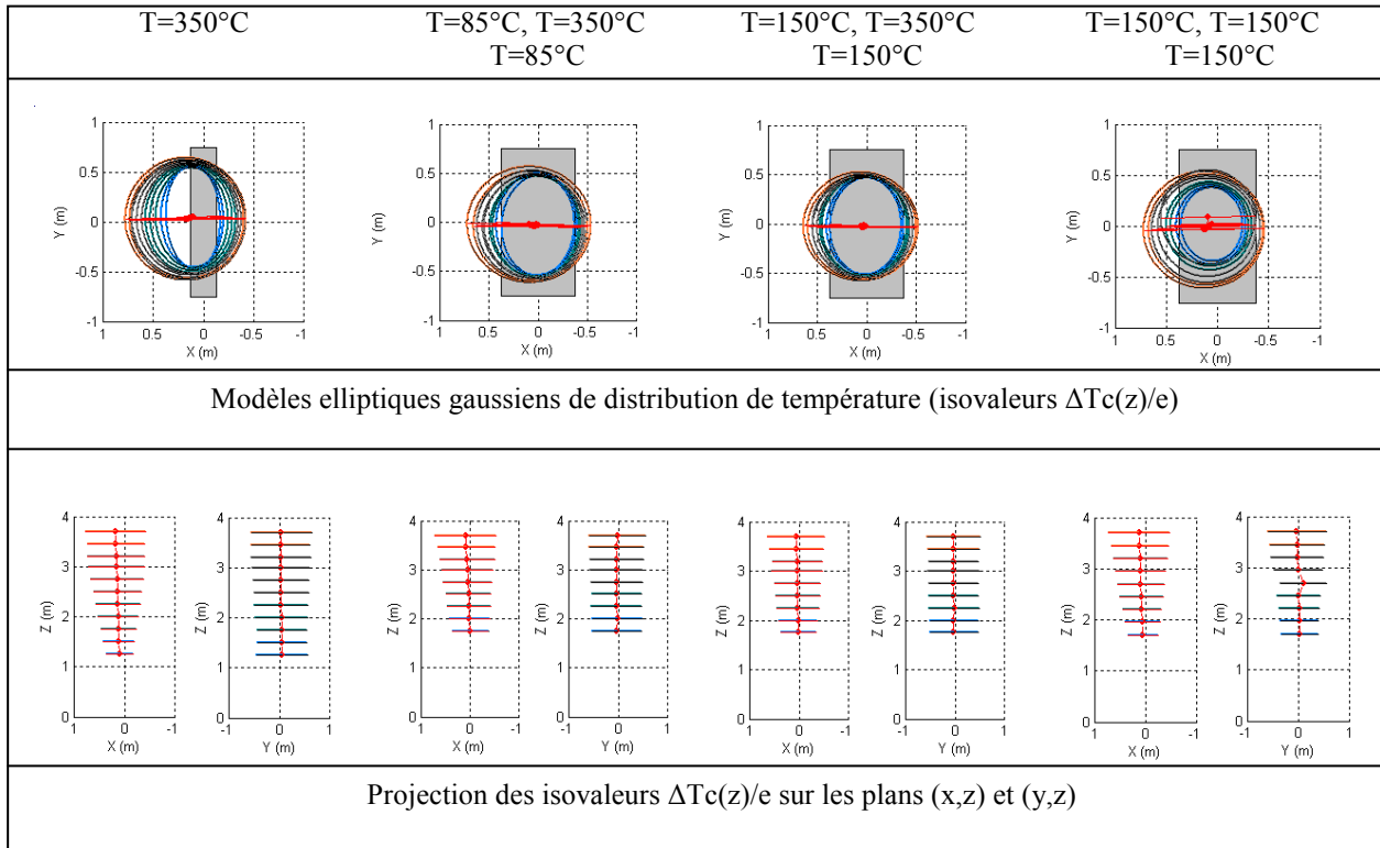
Figure 5.66 : comparaison des modèles elliptiques (isothermes \Delta T_c(z)/e ) sur les plans (x, y), (x, z) et (y, z) entre les quatre configurations
