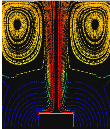
Figure 2.18 : Ligne de courant colorée en fonction de la température, stratification du milieu environnant
