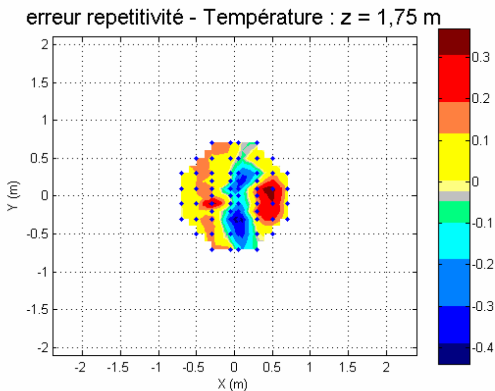
figure 4 : différence de température entre deux séries de mesures à z = 1,75 \text{ m} - 1 \text{ source}
