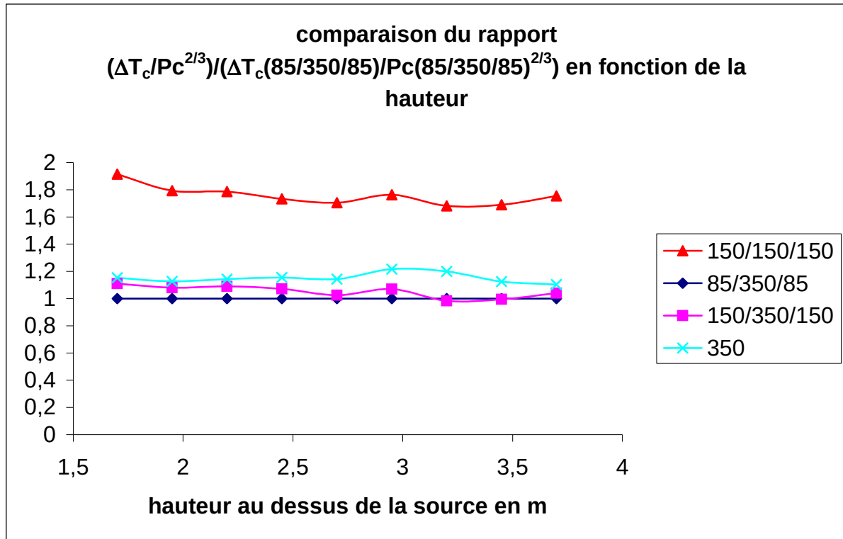
figure 5.69 : comparaison du rapport \Delta T_c /puissance convectée entre un cas étudié et le cas référence pour plusieurs cas de sources rectangulaires référencés par leur température
