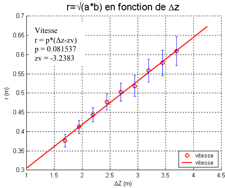
Figure 5.58 : Erreur de mesure sur le rayon dynamique en fonction de z : cas 3 sources
