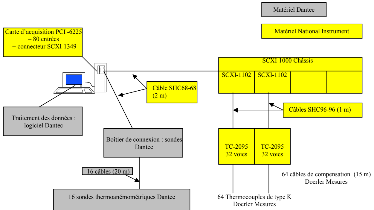
Figure 3.7 : Schéma simplifié du nouveau système de mesure simultanée de 64 thermocouples et de 16 sondes thermoanémométriques
