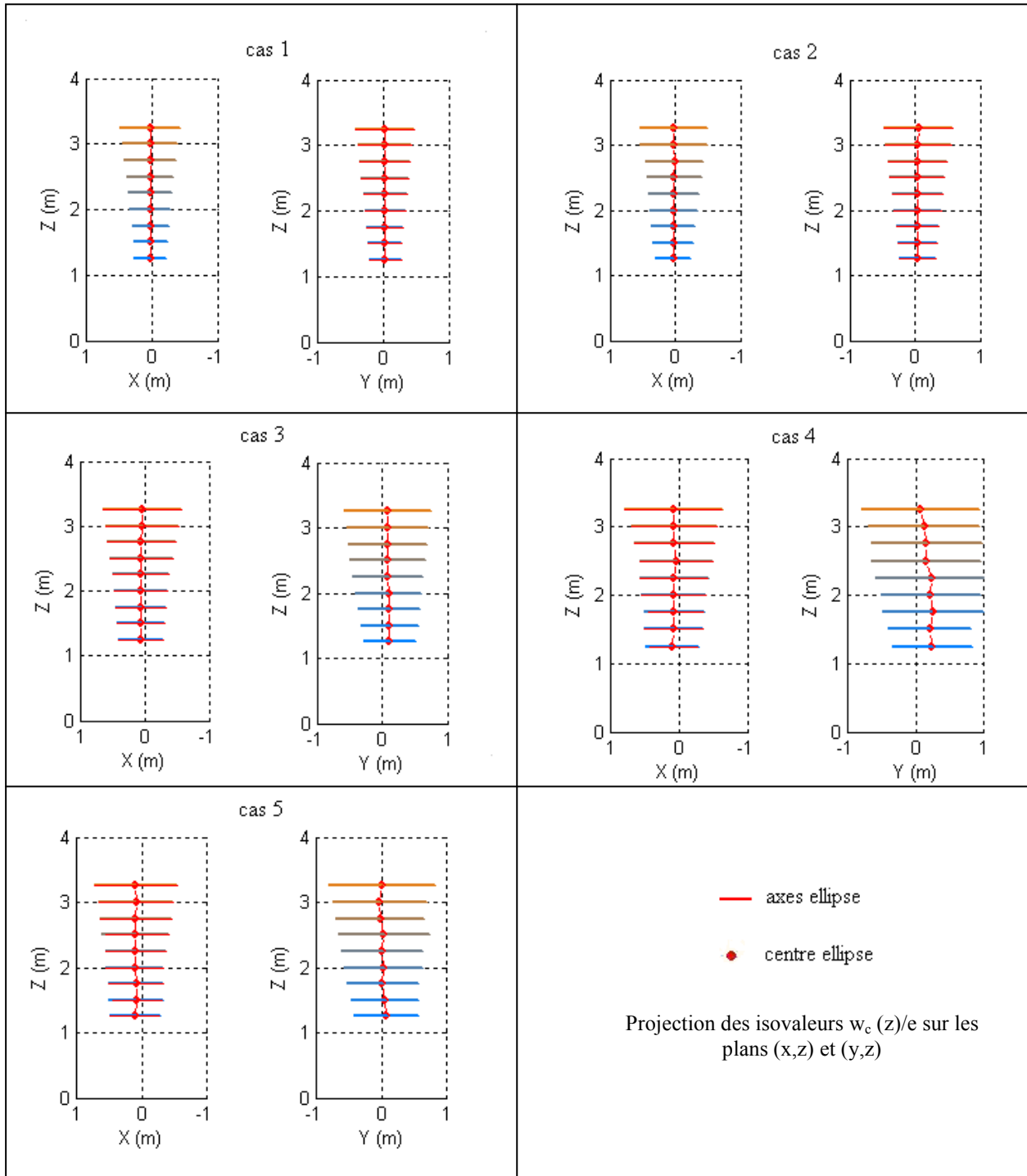
Figure 5.5 : Comparaison des coordonnées x_0 et y_0 du centre entre les cinq séries de mesure à différentes hauteurs
