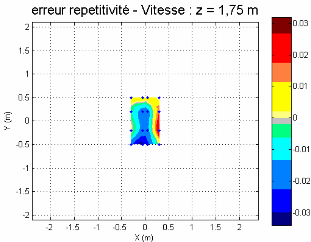
figure 6 : différence de vitesse entre deux séries de mesures à z = 1,75\text{ m} – 1 source
