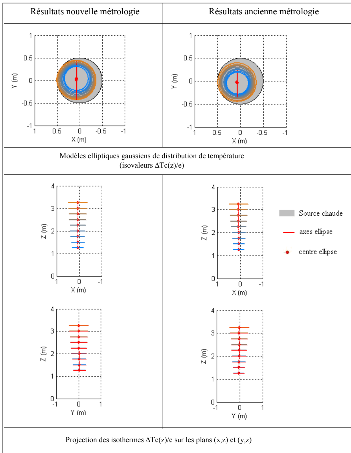
Figure 4.5 : Comparaison des modèles elliptiques (isothermes \Delta T_c(z)/e ) et des coordonnées x_0 et y_0 du centre entre les deux séries de mesure pour le cas 2 à différentes hauteurs
