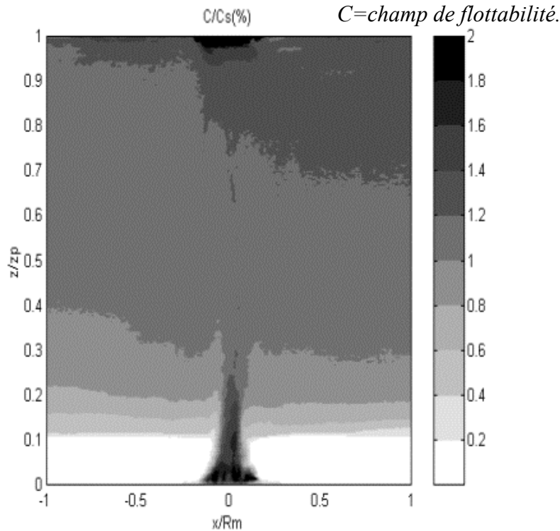
Figure 2.12 : Exemple de champ de concentration mesuré en simulation hydraulique par fluorescence induite par plan laser (d'après Auban [11] ; Auban et al. [42]).
