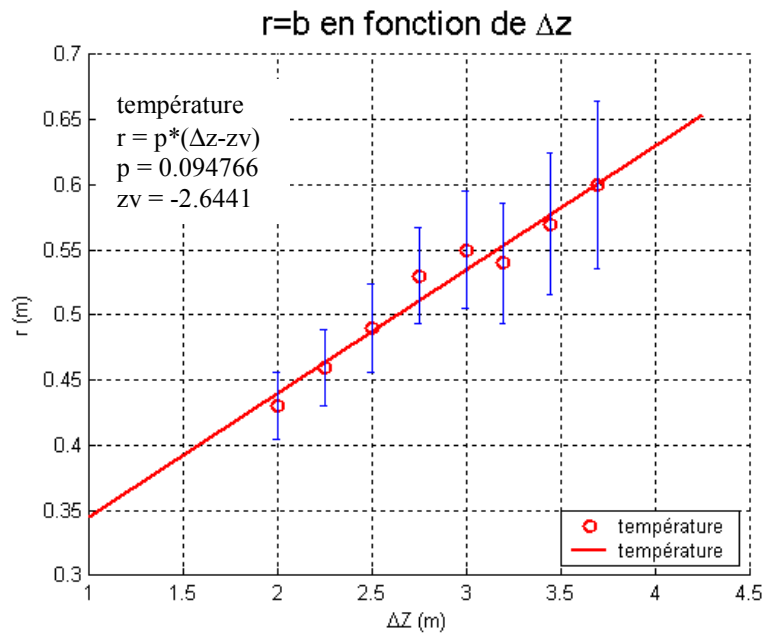
Figure 5.53 : Erreur de mesure sur le rayon thermique en fonction de z : cas 2 sources
