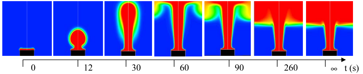
Figure 2.17 : Evolutions du champ de température de l'air environnant dans une enceinte ventilée ( Q_v=1500\text{m}^3/\text{h} ) cylindrique ( R=2.5\text{m} et H=5\text{m} ) avec une source thermique de 1.54\text{m} de diamètre à 200^\circ\text{C}
