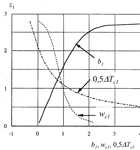
Figure 2.3 : Solutions adimensionnées pour un panache développé en milieu stratifié (d'après Morton et al. [12]).
