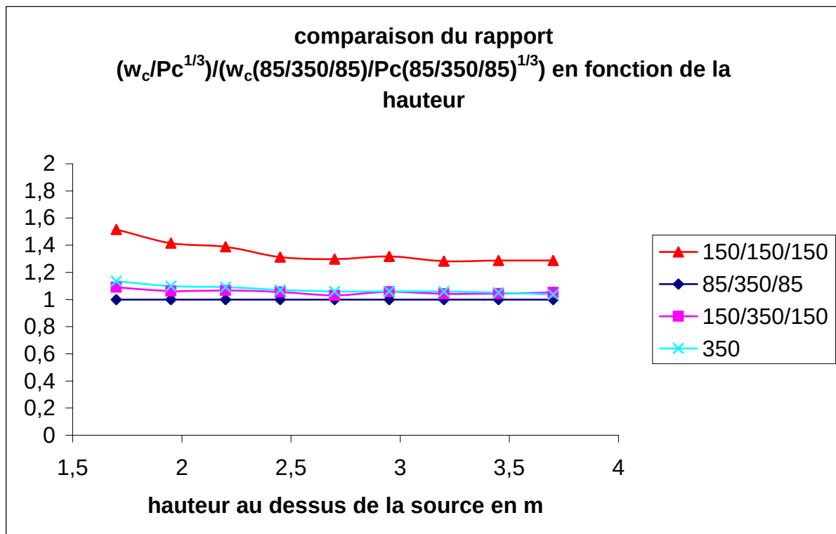
figure 5.70 : comparaison du rapport w_c /puissance convectée entre un cas étudié et le cas référence pour plusieurs cas de sources rectangulaires référencés par leur température
