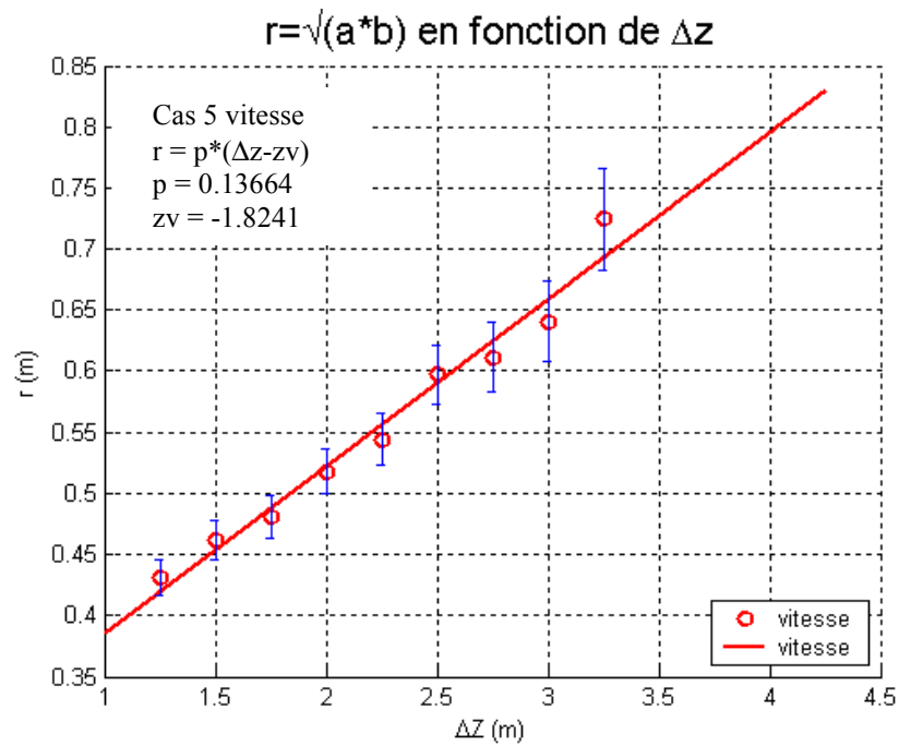
Figure 5.29 : Evolution des rayons dynamiques - Comparaison des origine virtuelles : cas 5
