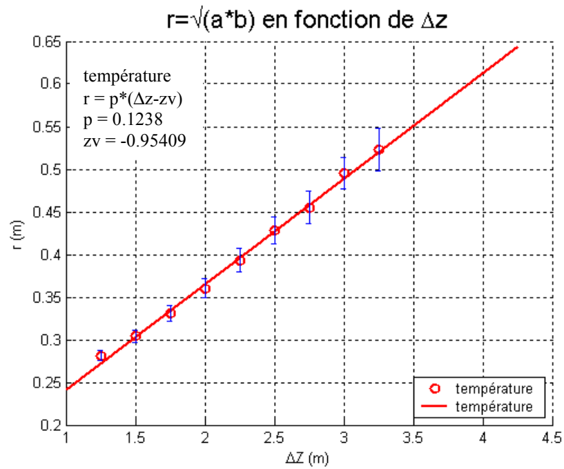
Figure 5.21 : Evolution des rayons thermiques - Comparaison des origine virtuelles : cas 2
