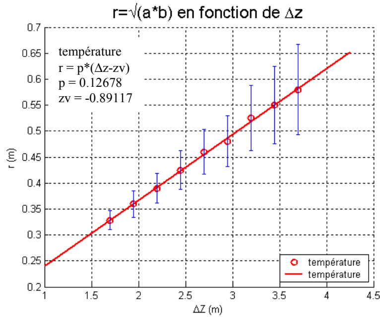
Figure 5.54 : Erreur de mesure sur le rayon thermique en fonction de z : cas 3 sources
