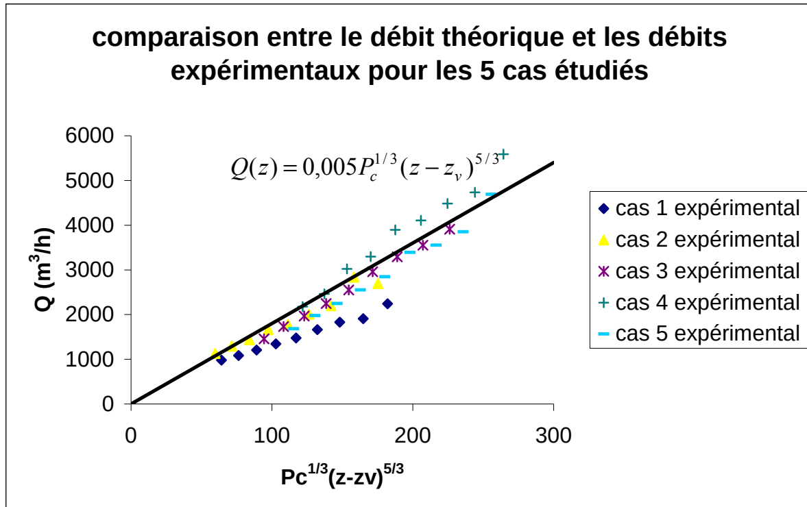
Figure 5.16 : Comparaison entre les débits expérimentaux et théoriques pour les 5 cas étudiés
