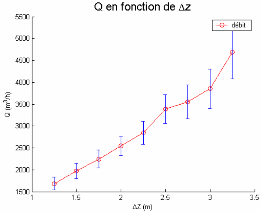
figure 5.34 : débit expérimental en fonction de \Delta z - incertitude pour le cas 5
