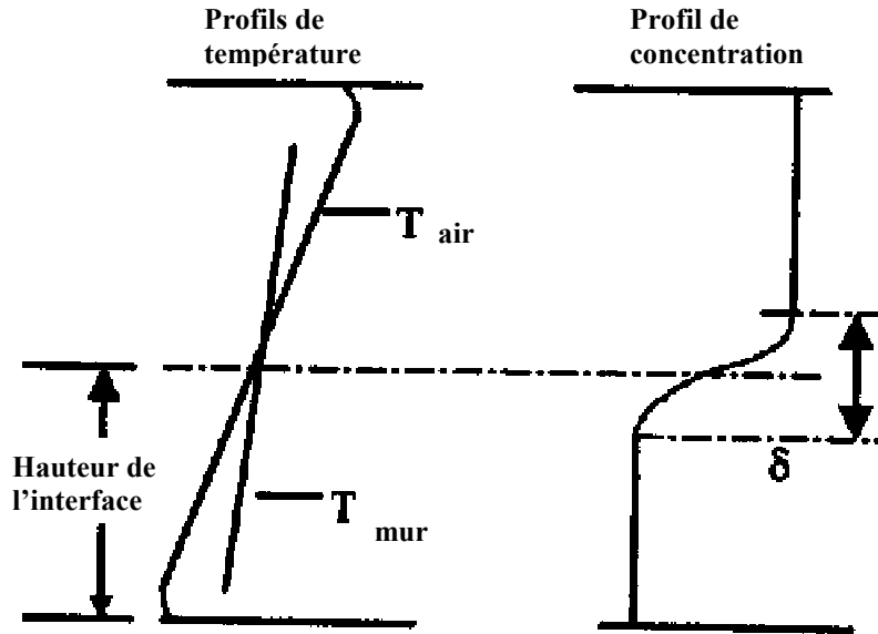
Figure 2.11 : Critères adoptés par Xing et Awbi ([38] et [39]) et Stymne et al. [41] pour localiser la thermocline en enceinte aéraulique.
