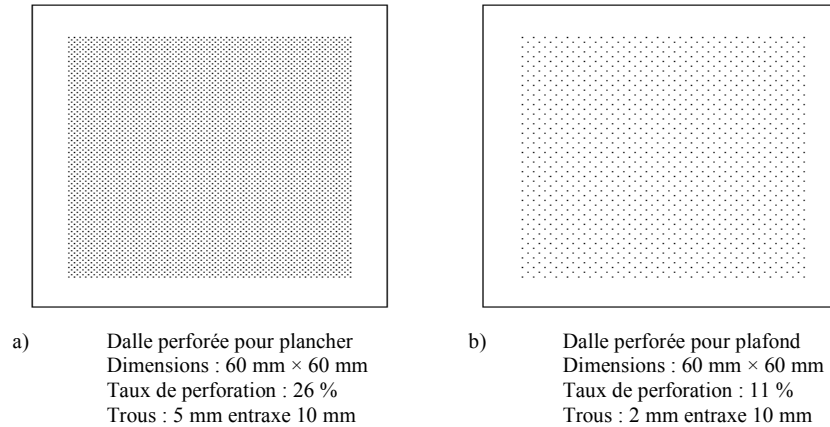
Figure 3.2 : Dalles utilisées pour construire le plancher et le plafond de la chambre d'essai
