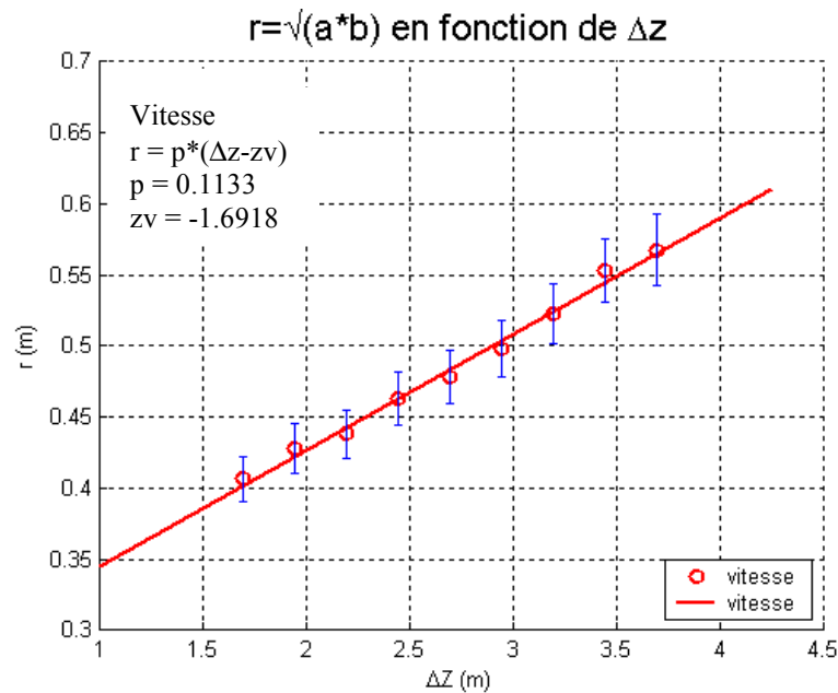
Figure 5.59 : Erreur de mesure sur le rayon dynamique en fonction de z : cas 4 sources
