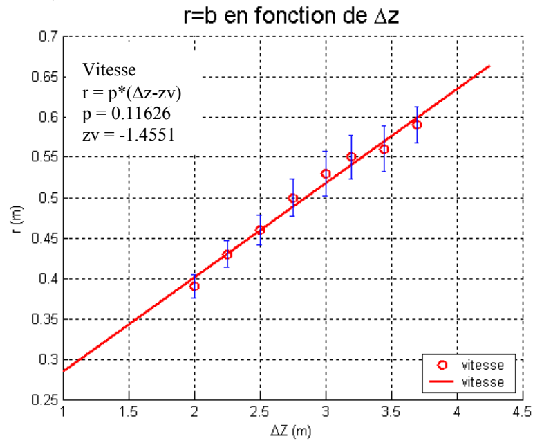
Figure 5.56 : Erreur de mesure sur le rayon dynamique en fonction de z : cas 1 source
