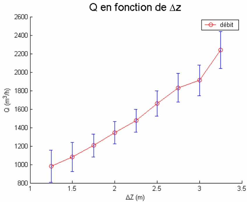
figure 5.30 : débit expérimental en fonction de \Delta z - incertitude pour le cas 1
