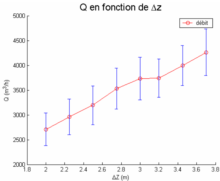
figure 5.61 : débit en fonction de la hauteur z – barres d'erreur : cas 2 sources
