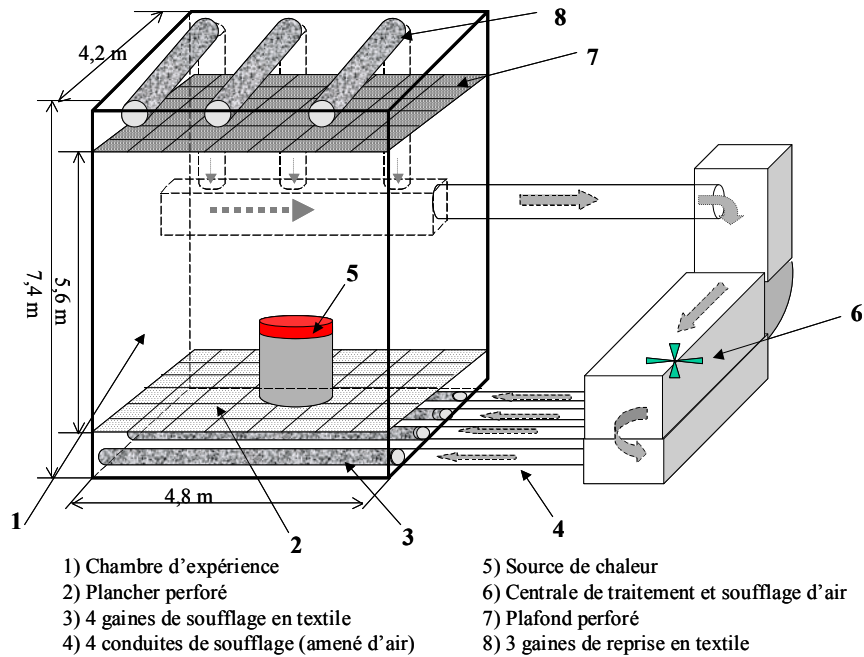
Figure 3.1 : Schéma de la cellule aéraulique installée à l'INRS
