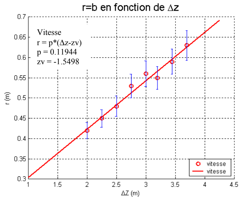
Figure 5.57 : Erreur de mesure sur le rayon dynamique en fonction de z : cas 2 sources
