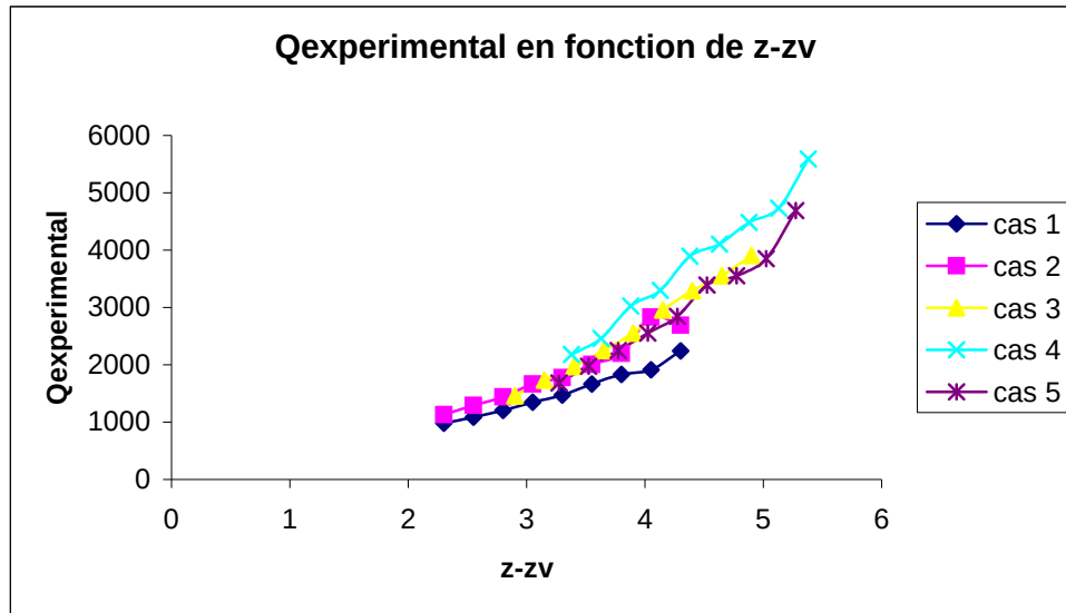
figure 5.15 : Evolution du débit d'air emporté par le panache en fonction de z-z_v pour les cinq cas étudiés
