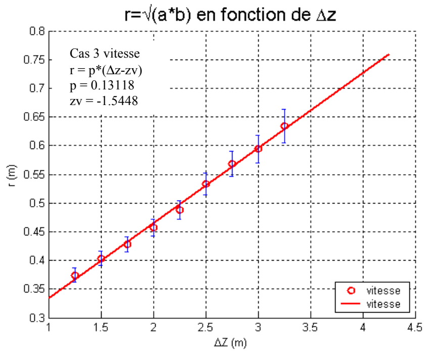
Figure 5.27 : Evolution des rayons dynamiques - Comparaison des origine virtuelles : cas 3
