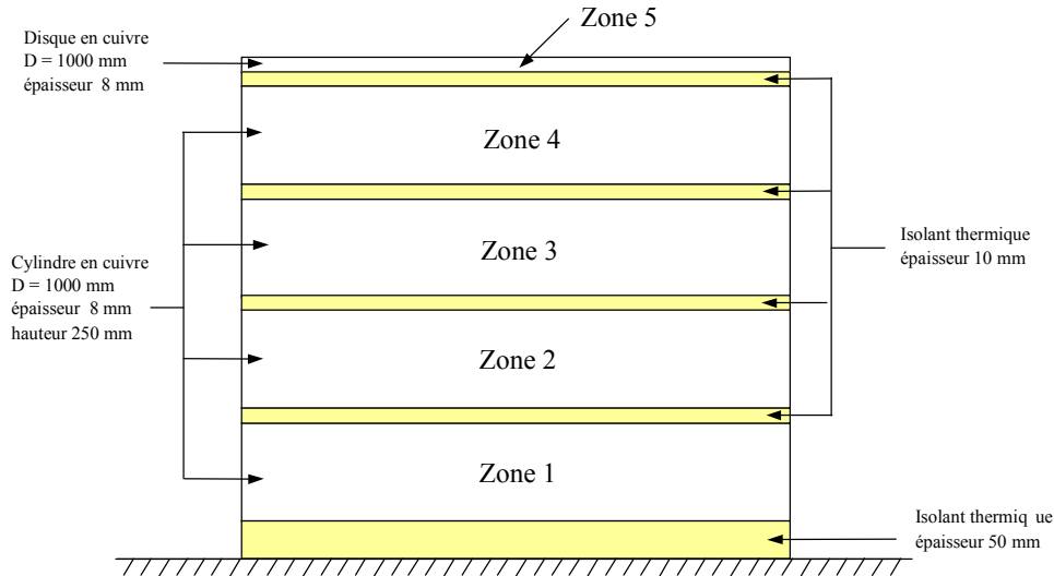
Figure 3.5 : Schéma de la source cylindrique utilisée
