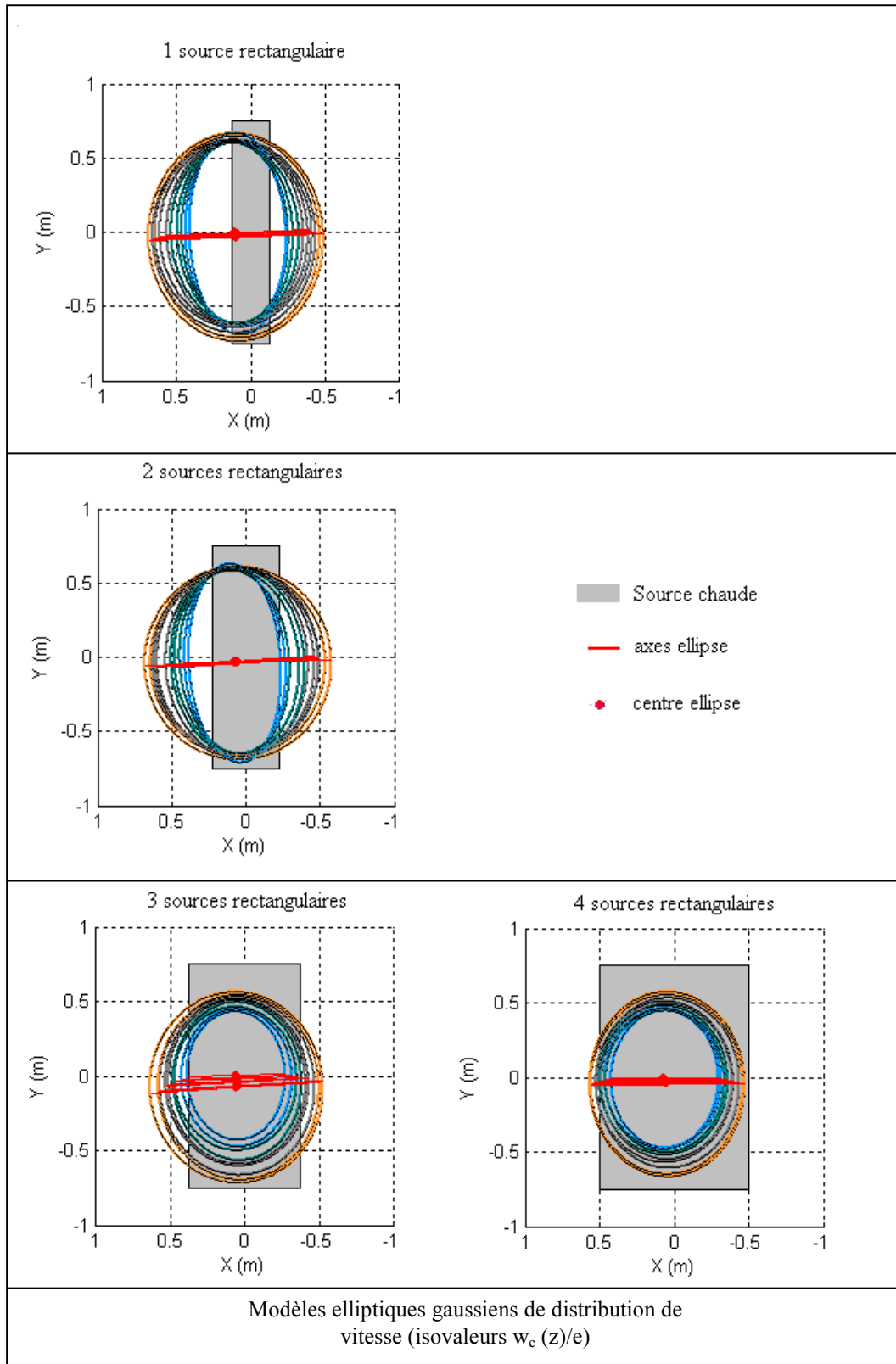
Figure 5.42 : modèles elliptiques (isovitesse w_c(z)/e ) obtenus pour 1, 2, 3 et 4 sources rectangulaires
