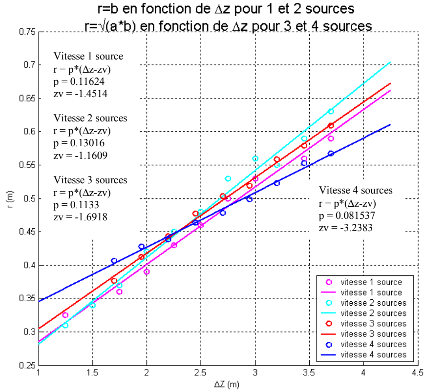
Figure 5.47 : Evolution des rayons dynamiques en fonction de z ( r = b pour 1 et 2 sources et r = \sqrt{ab} pour 3 et 4 sources) - Comparaison des origine virtuelles
