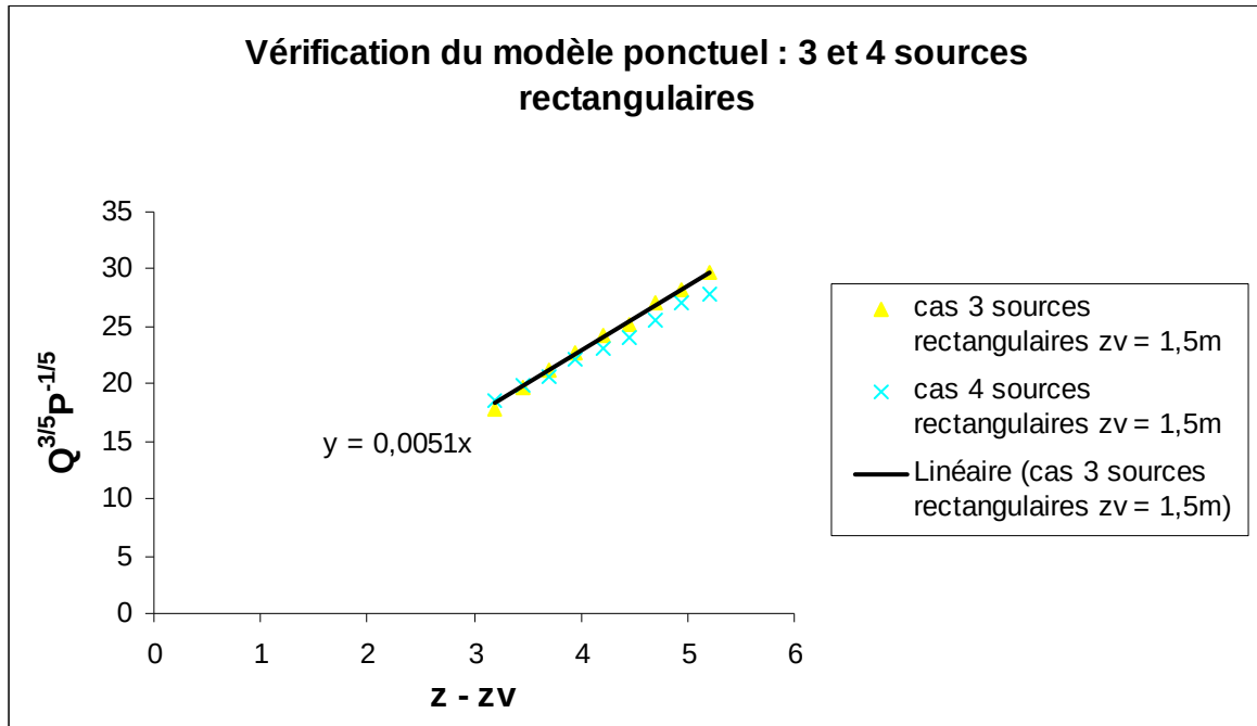
figure 5.51 : vérification du modèle ponctuel à partir de la formule du débit Q(z) = 0,005 \cdot P_c^{1/3} (z - z_v)^{5/3} : 3 et 4 sources rectangulaires
