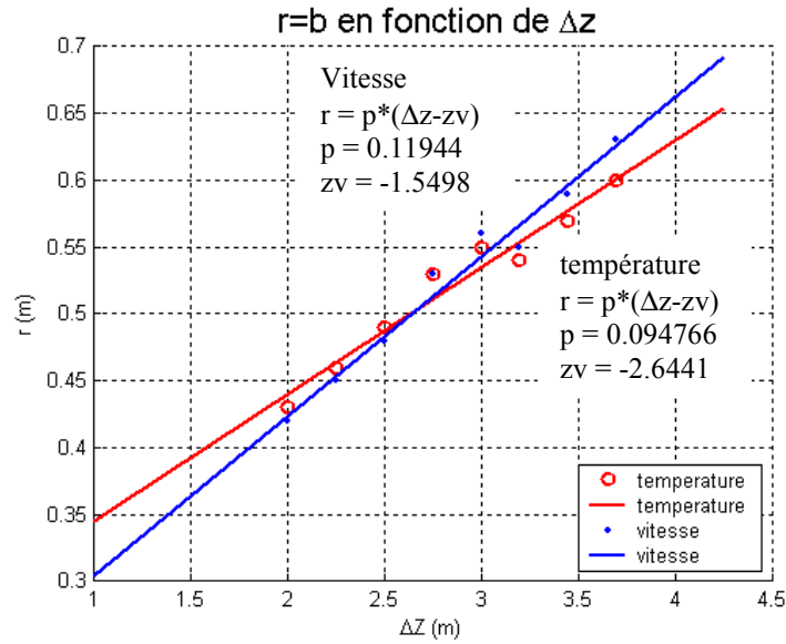
Figure 5.49 : Evolution des rayons thermiques et dynamiques en fonction de z > 2m - Comparaison des origine virtuelles : 2 sources
