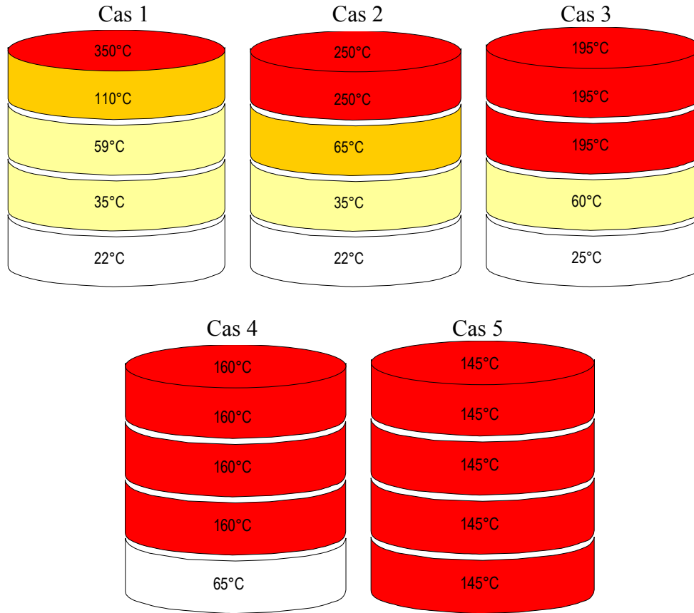
figure 5.1 : configuration de la source pour les cas 1, 2, 3, 4, 5
