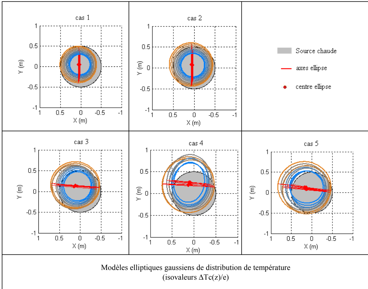
Figure 5.2 : Comparaison des modèles elliptiques (isothermes \Delta T_c(z)/e ) entre les cinq séries de mesure à z = 1,25, 1,50, 1,75, 2,25, 2,75 et 3,25 m
