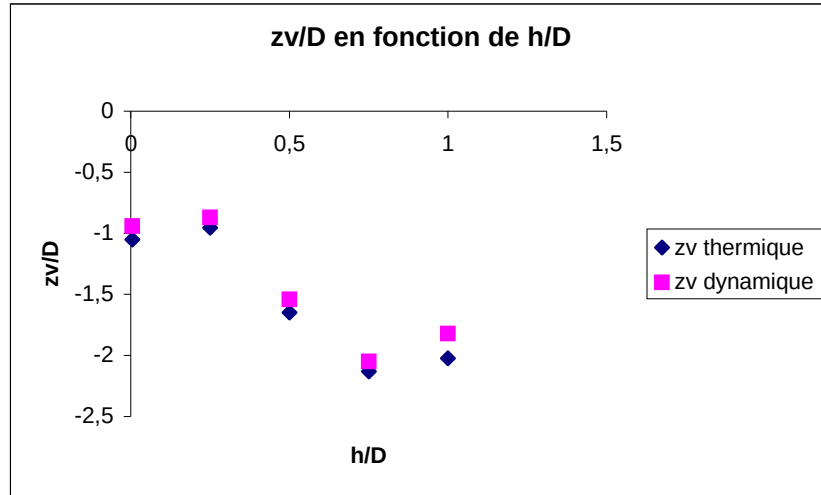
Figure 5.11 : z_v/D en fonction de hauteur de chauffe/D obtenus avec z_v thermique et z_v dynamique
