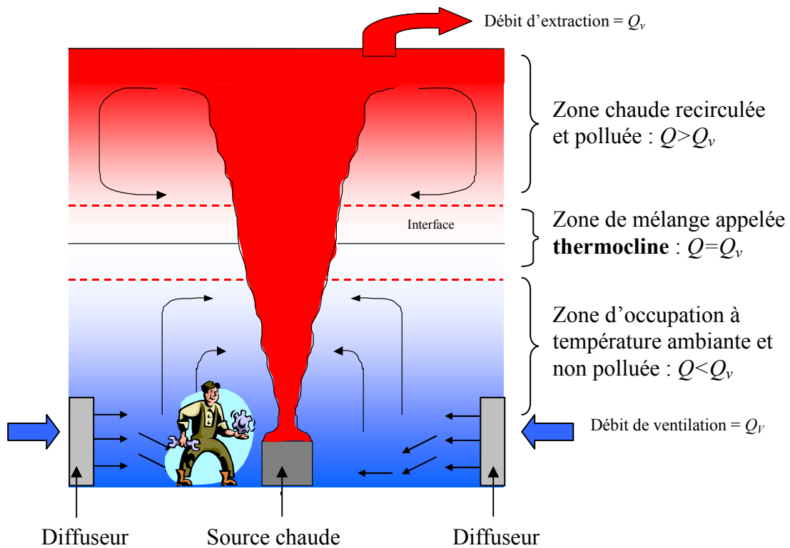
Figure 2.1 : Principe de la ventilation par déplacement
