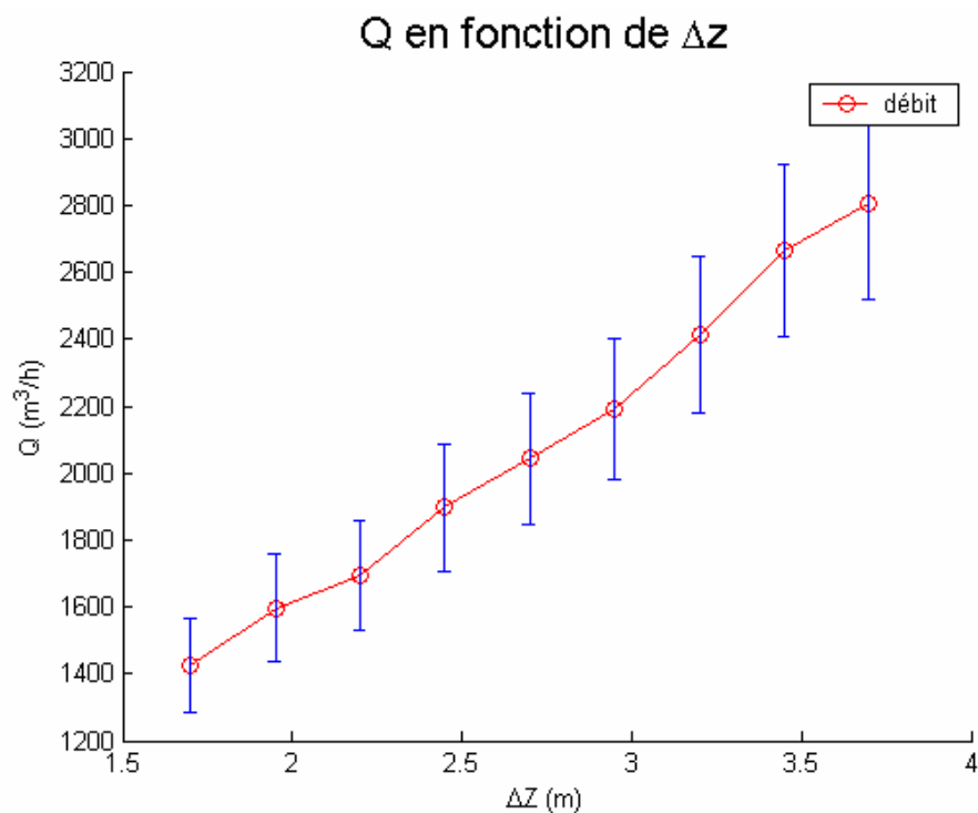
figure 5.63 : débit en fonction de la hauteur z – barres d'erreur : cas 4 sources
