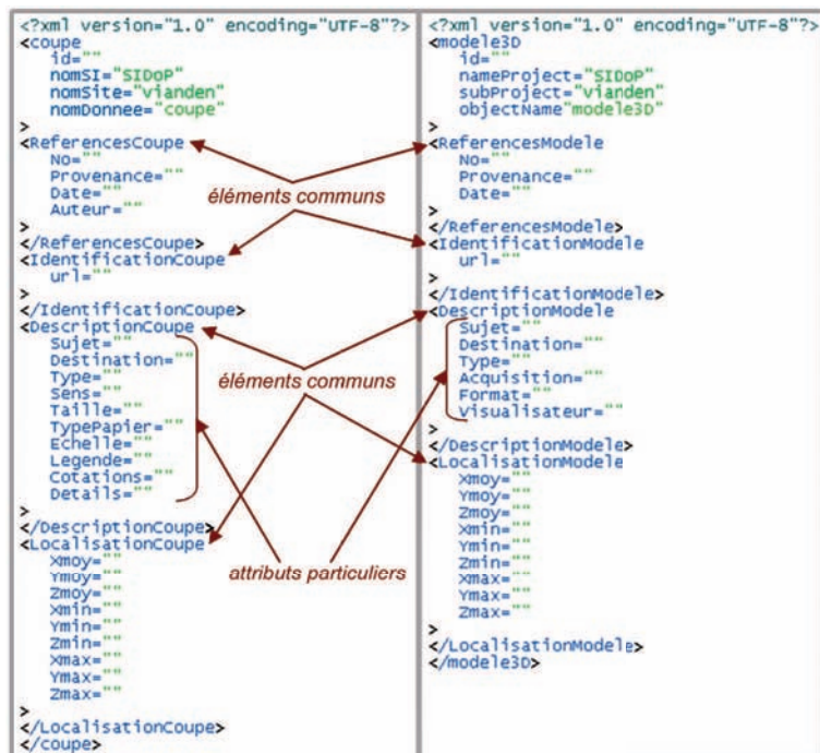
FIG. 7.4 – Schéma XML pour les données de type coupe et modele3D
