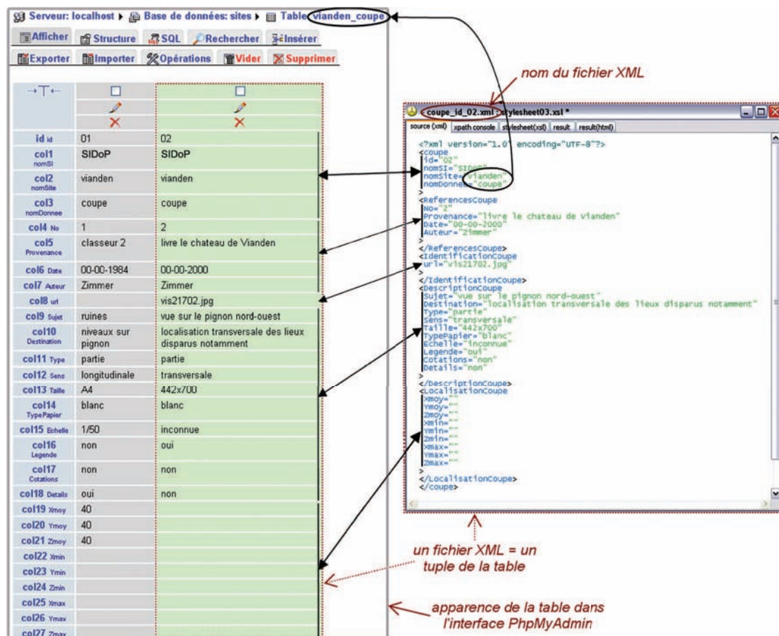
FIG. 7.6 – Correspondance entre un tuple d'une table MySQL et un fichier de donnée XML
