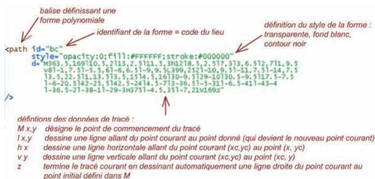
FIG. 8.12 – Géométrie d'un polygone en SVG
