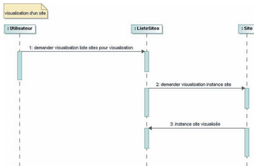
FIG. 10.9 – Diagramme de séquence décrivant la visualisation d'un site
