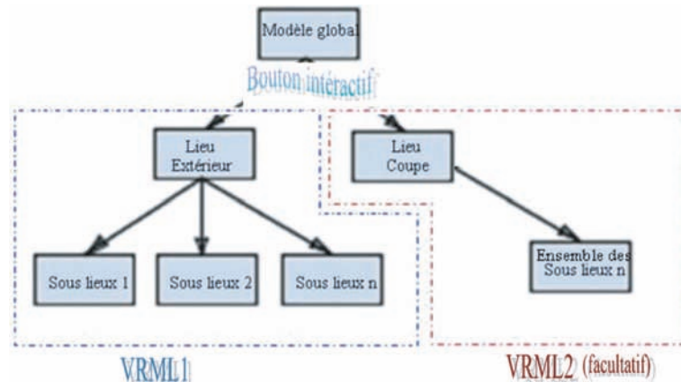
Figure 6 - Structure hiérarchique du VRML final représentant une entité lieu et sous-lieux
