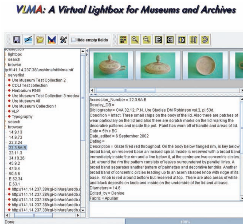
FIG. 2.5 – L'outil VLMA pour la visualisation de collections de musées [ http://lkws1.rdg.ac.uk/ure/js/test2.html ] [réf. du 01 mai 2007]
