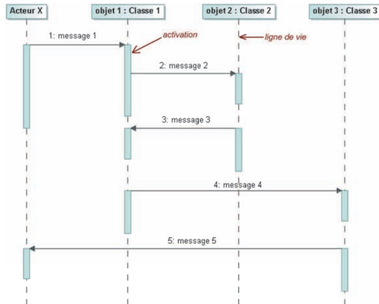
FIG. 10.2 – Formalisme du diagramme de séquence
