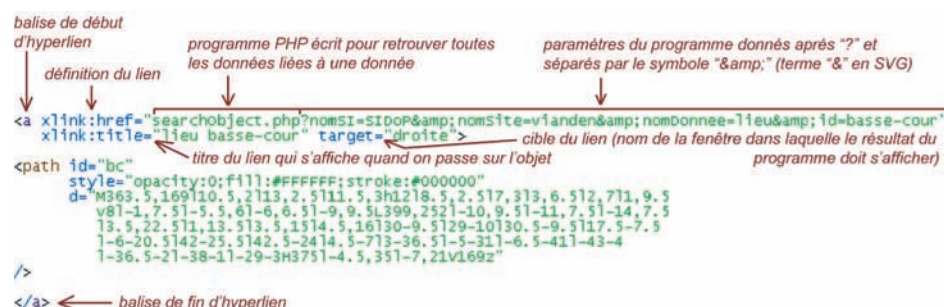
FIG. 8.14 – Ajout d'un hyperlien sur une zone pour retrouver toutes les données liées au lieu représenté
