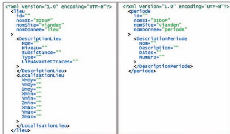
FIG. 7.3 – Schémas XML pour les données de types lieu (à gauche) et période (à droite)
