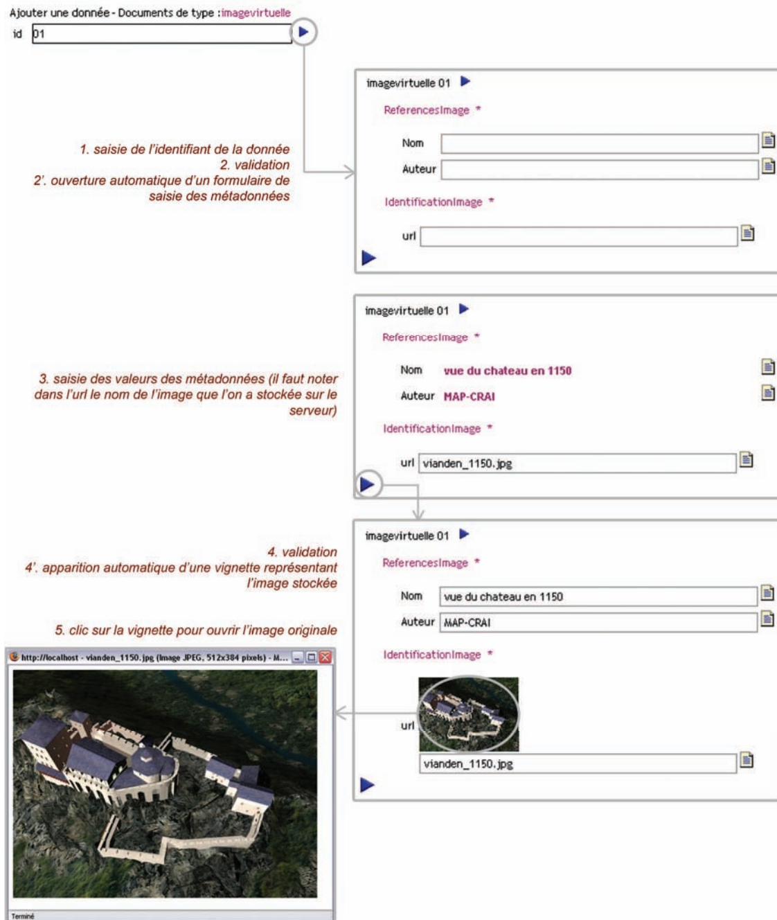
FIG. 7.11 – Procédure pour l'ajout d'une donnée de type imagevirtuelle
