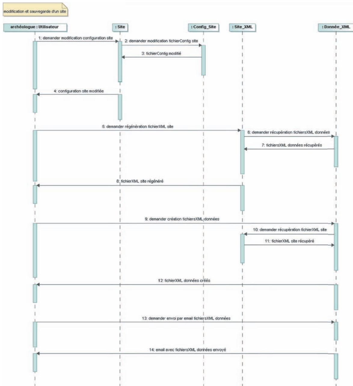
FIG. 10.8 – Diagramme de séquence décrivant la modification et la sauvegarde d'un site
