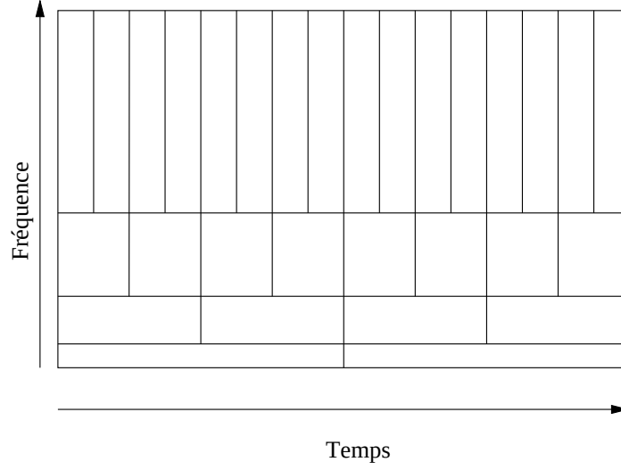
FIG. 3.4 – Décomposition temps-fréquence du signal. Une décomposition dyadique est appliquée à la fois sur l'axe du temps et l'axe des fréquences.
