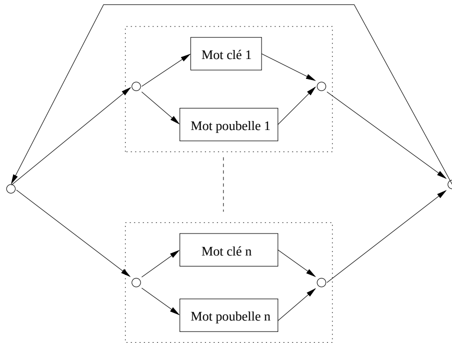
FIG. 6.1 – Description d'un système de détection de mots clés basé sur l'utilisation d'un réseau de mots clés et de modèles poubelles.
