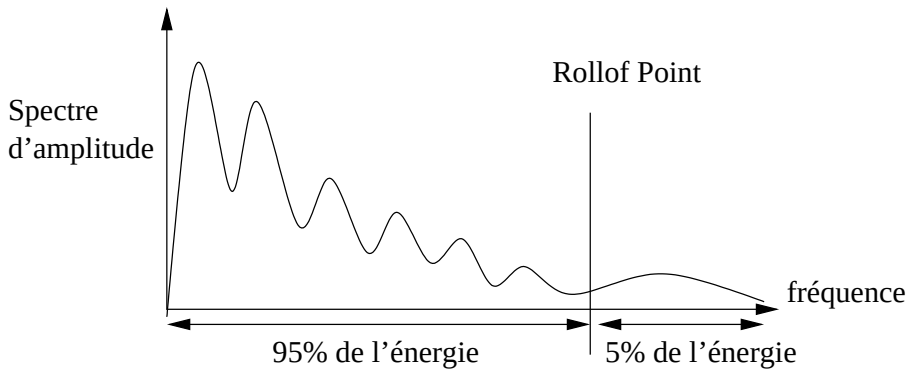
FIG. 1.5 – Définition du “ Spectral Rolloff Point ”
