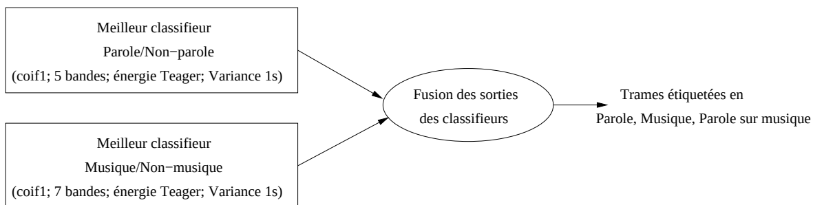
FIG. 5.5 – Fusion de classifieurs consistant à regrouper la sortie du meilleur classifieur parole/non-parole et la sortie du meilleur classifieur musique/non-musique. (Fusion 1PNP-1MNM).
