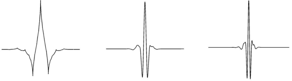
FIG. 3.10 – Exemples de Coiflets : de gauche à droite nous avons 'coif1', 'coif3' et 'coif5'.
