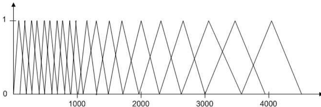
FIG. 1.3 – Filtres triangulaires à échelle Mel (20 bandes).
