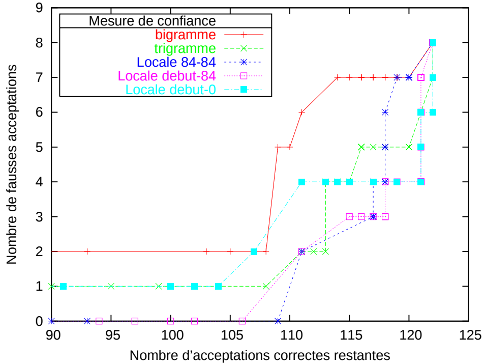
FIG. 6.1 – Evolution du nombre de fausses acceptations et du nombre de bons mots clés restant en fonction du seuil de décision (corpus de développement).
