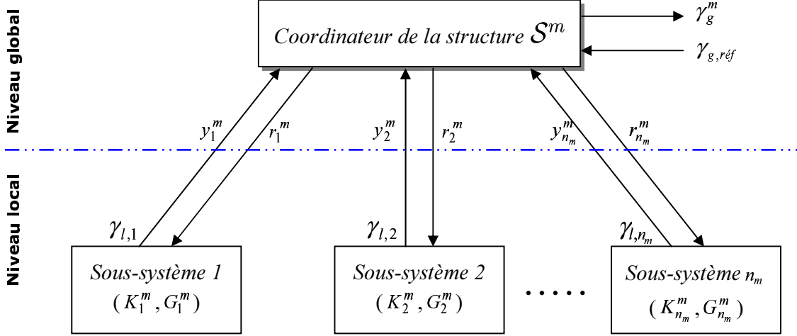
FIG. 3.3 – L'architecture du système sous une structure \mathcal{S}^m
