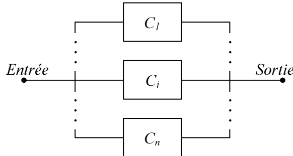
FIG. 1.12 – Système avec n composants en parallèles
