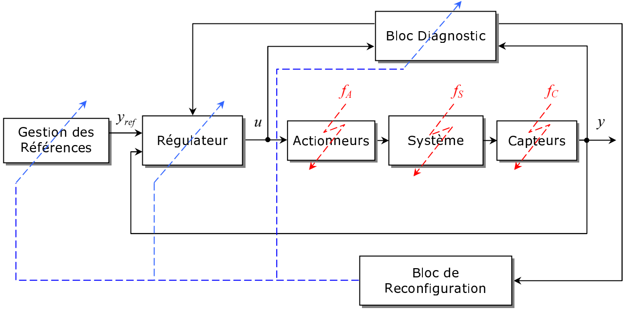
FIG. 1.4 – Structure générale des systèmes tolérants aux défauts
