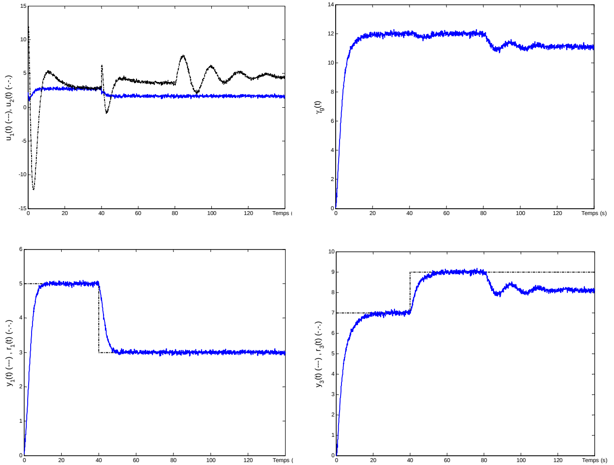
FIG. 3.7 – Évolution dynamique des variables de commande et de sortie du système défaillant ( \beta = 30\% )
