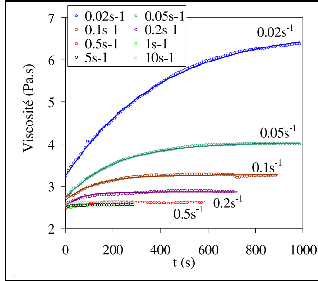
Fig. 11.25 Variation de viscosité lors de l'orientation des bâtonnets PF60 (20,3%) pour différents gradients de vitesse. Les lignes continues sont les modélisations obtenues avec les courbes de type exponentiel.
