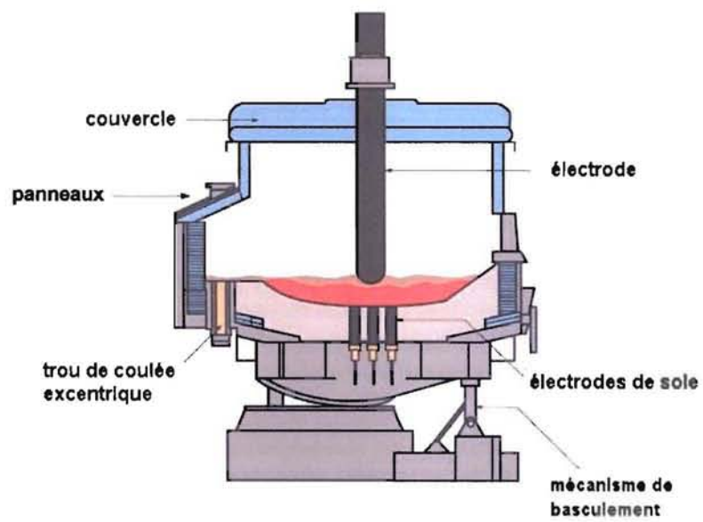
FIG. 1.2 – Vue détaillée du four
