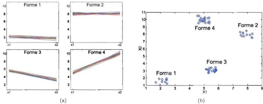
FIG. B.1 – Représentation du corpus artificiel avec ses quatre classes de formes 2D (a) Le corpus est représenté dans l'espace des signaux (b) Le même corpus dans l'espace des variables (chaque point représente une forme 2D)
