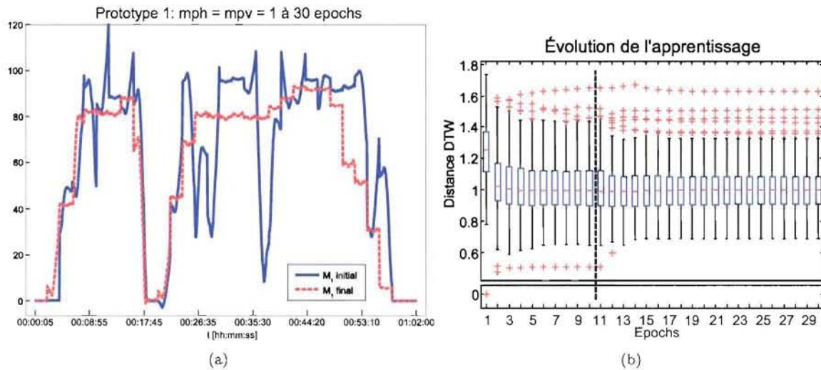
FIG. 3.41 – Résultat de l'apprentissage des prototypes sur les données du four :
