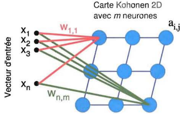
FIG. 2.1 – Carte auto-organisatrice de Kohonen (SOM) 2D avec le vecteur d'entrée \vec{x} = \{x_1, \dots, x_n\} et les vecteurs de référence représentés par \vec{w}_k = \{w_{1,k}, \dots, w_{n,k}\}
