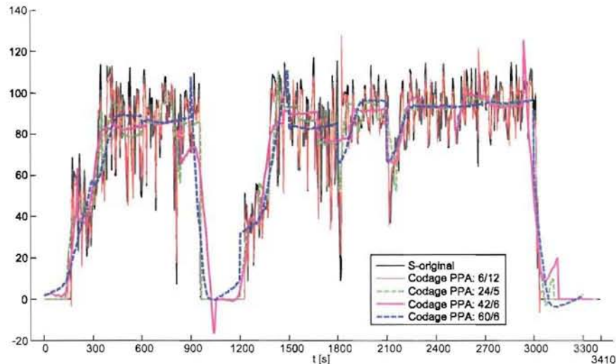
FIG. 4.20 – Ex. 2 - Nr-Ref. 41 : Représentation du signal original avec les reconstructions basées sur les quatres codages
