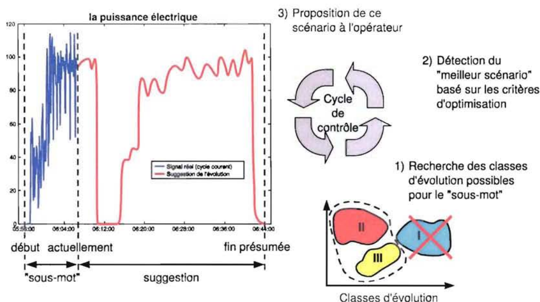
FIG. 4.1 – Le contrôle prédictif en ligne
