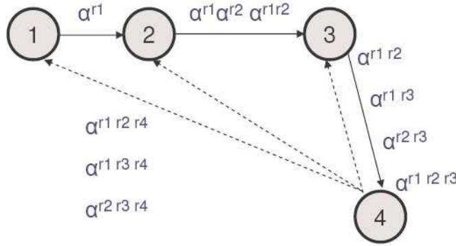
FIG. 2.5 – Exemple de génération de la clé de groupe dans GDH (avec 4 participants)
